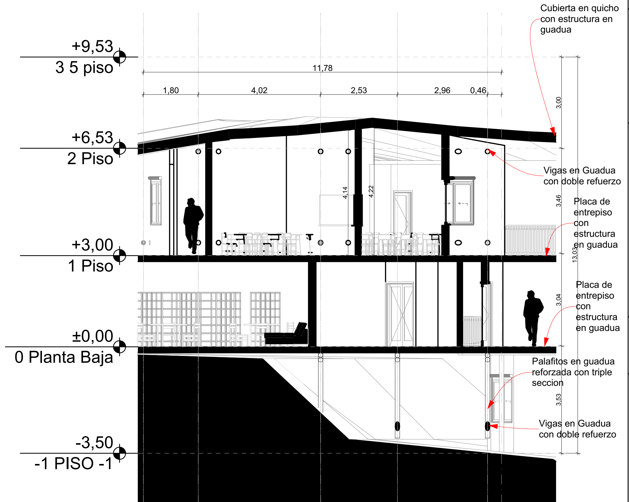
D Corte 7 esc: 1_50
