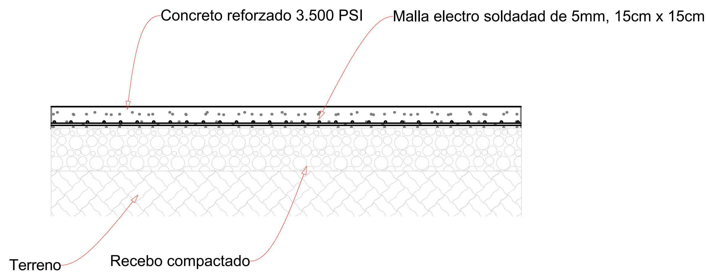
D10 Detalle constructivo placa en concreto esc: 1_20
