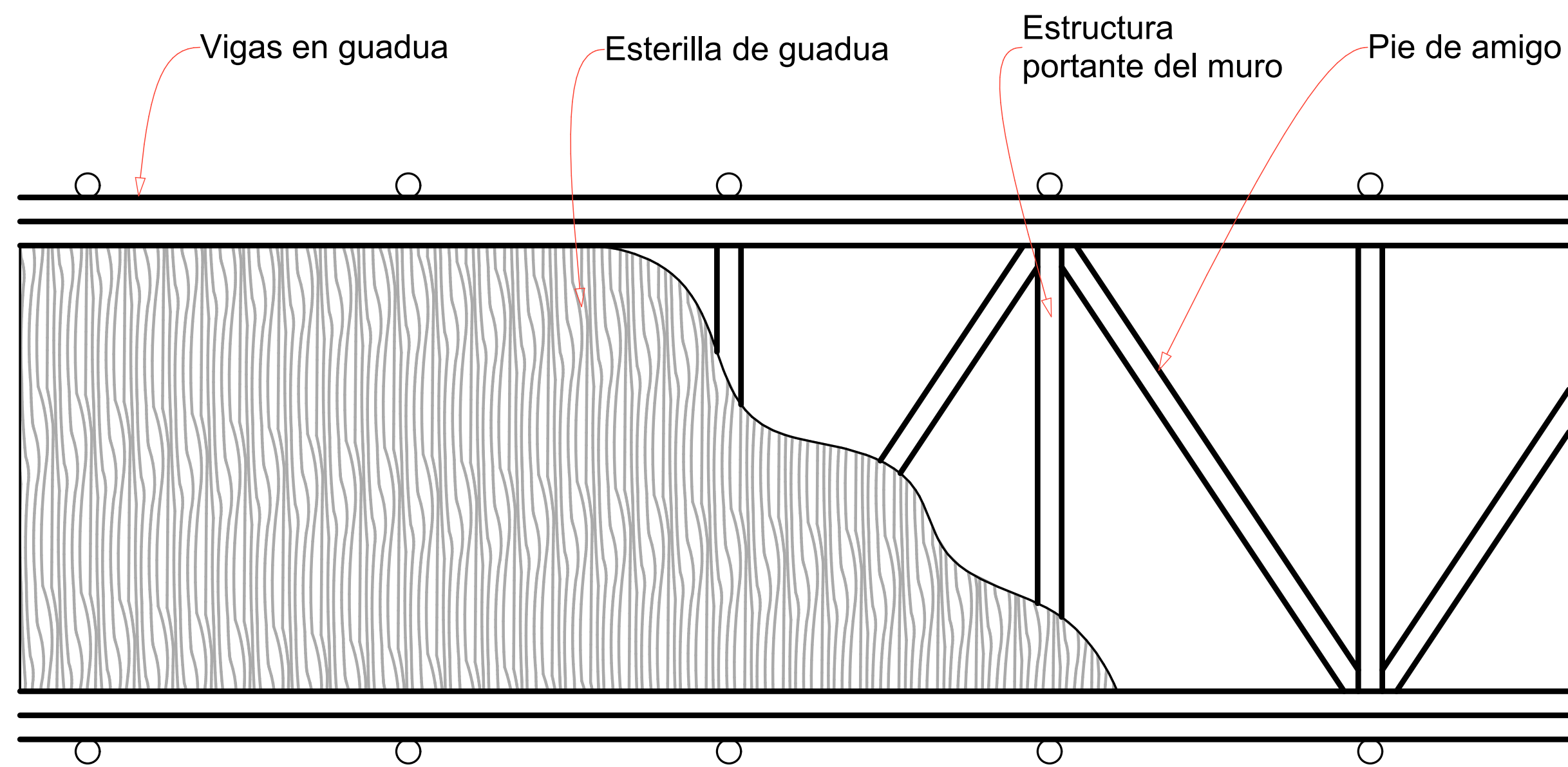
D09 Detalle constructivo muros esc: 1_30
