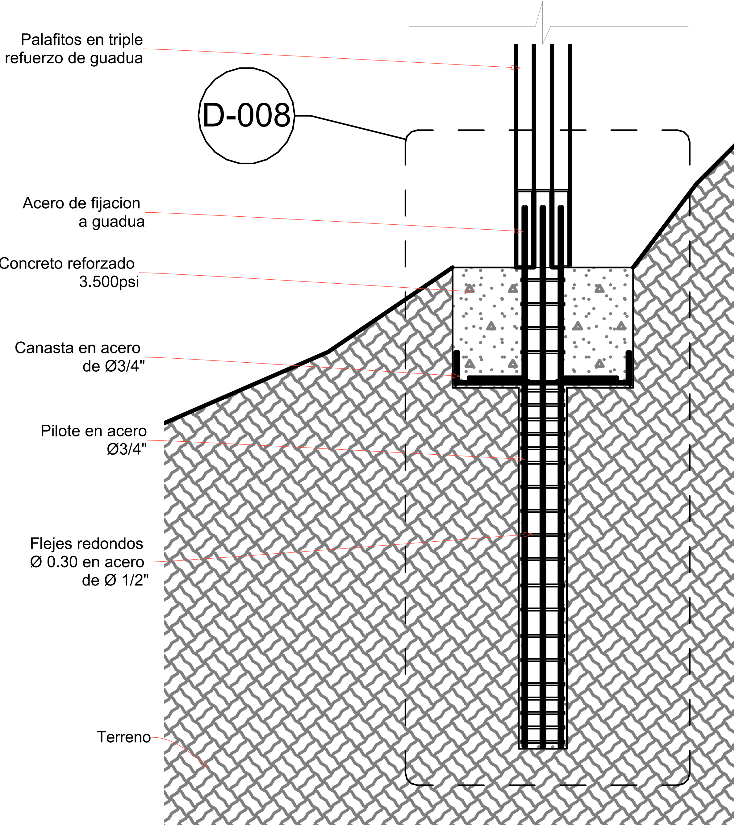
D08 Detalle constructivo esc: 1_20
