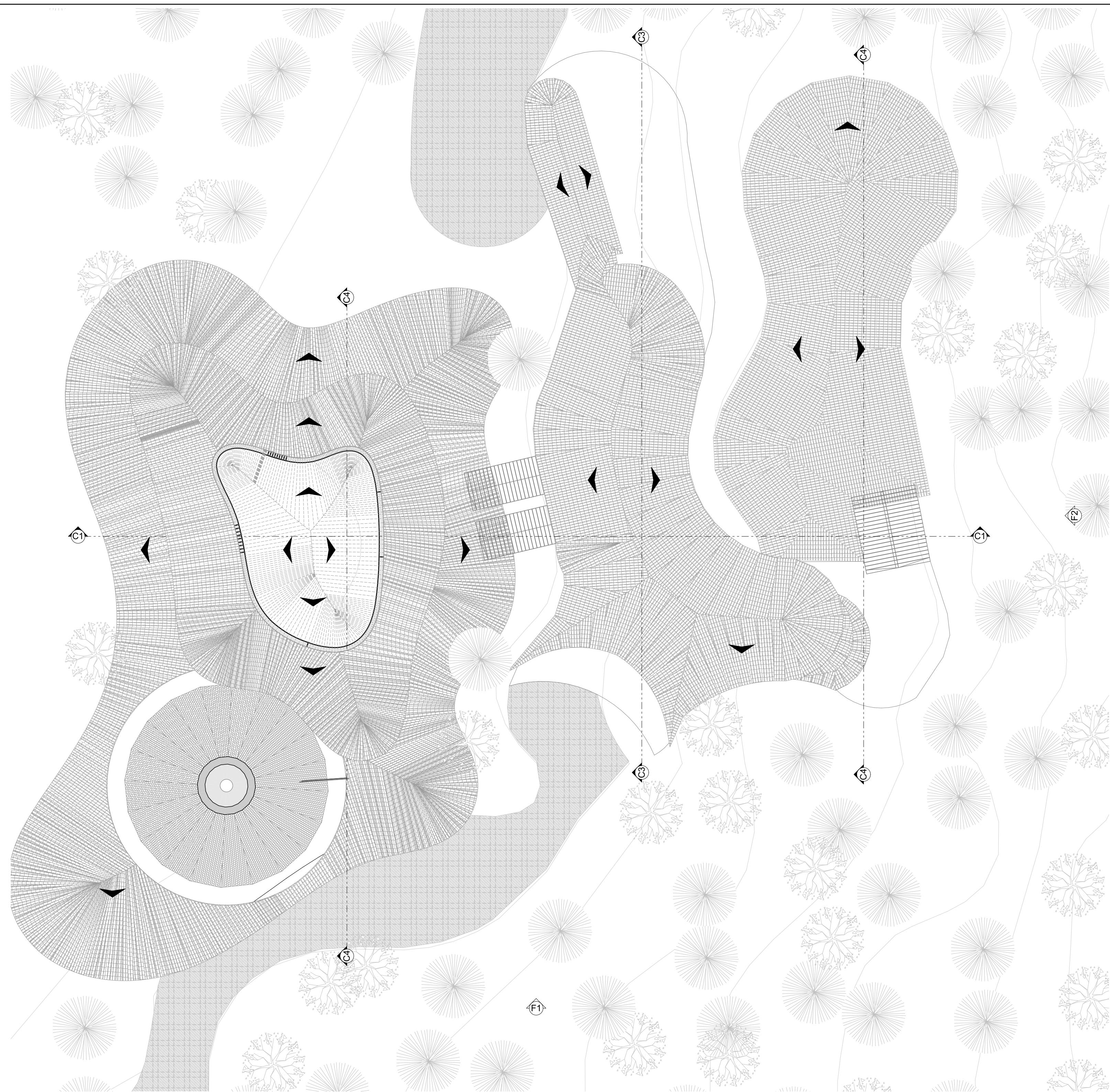
A Planta de cubiertas esc: 1_200
