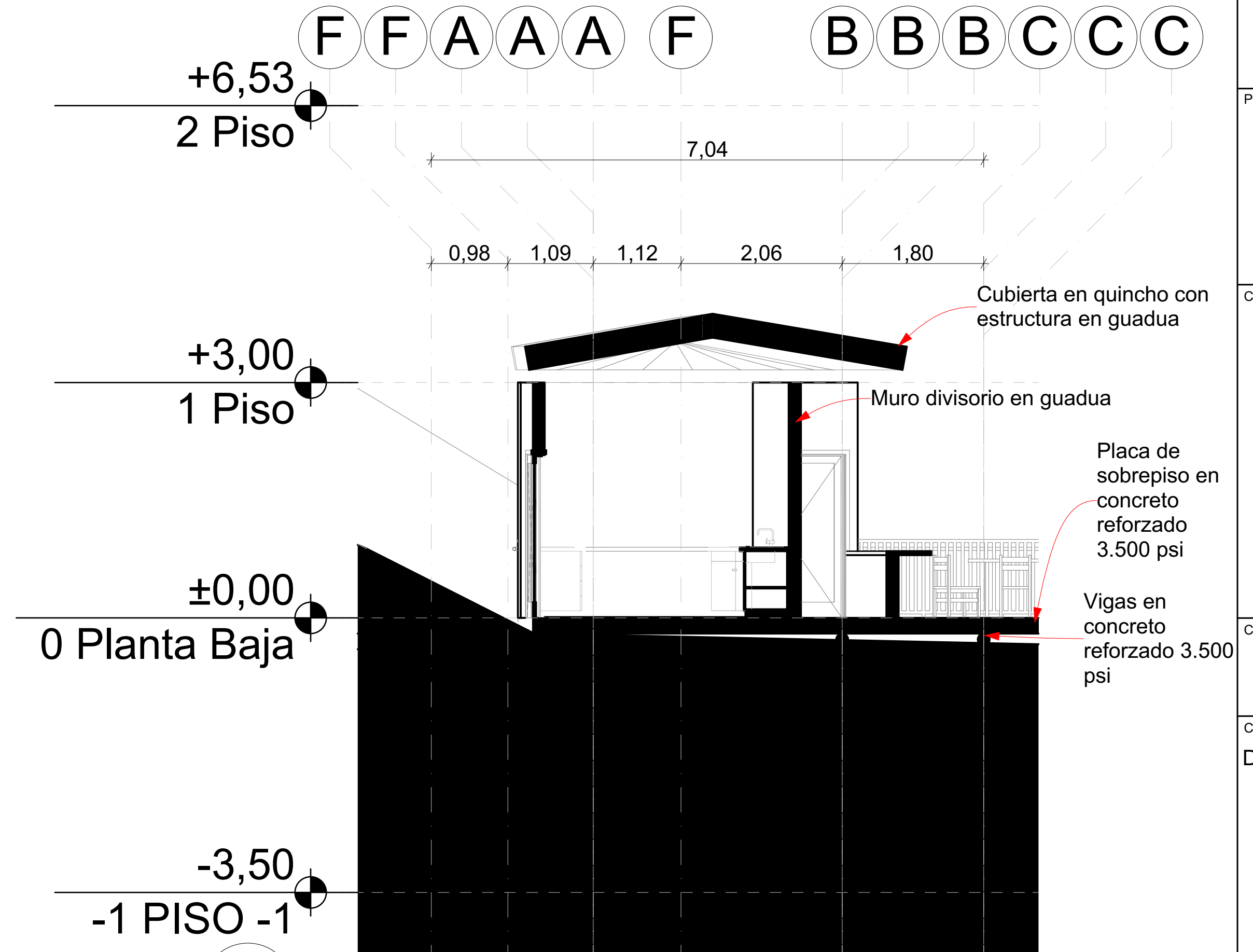
D Corte 5 esc: 1_50
