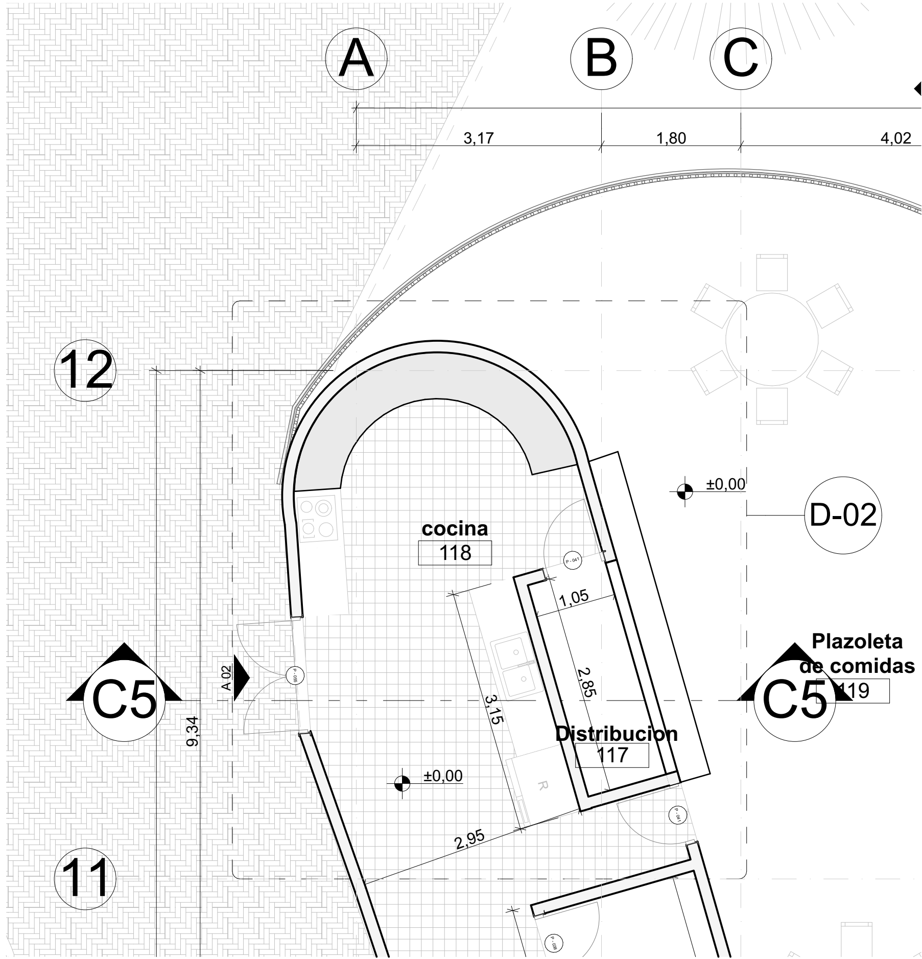
D Detalle 02 esc: 1_50
