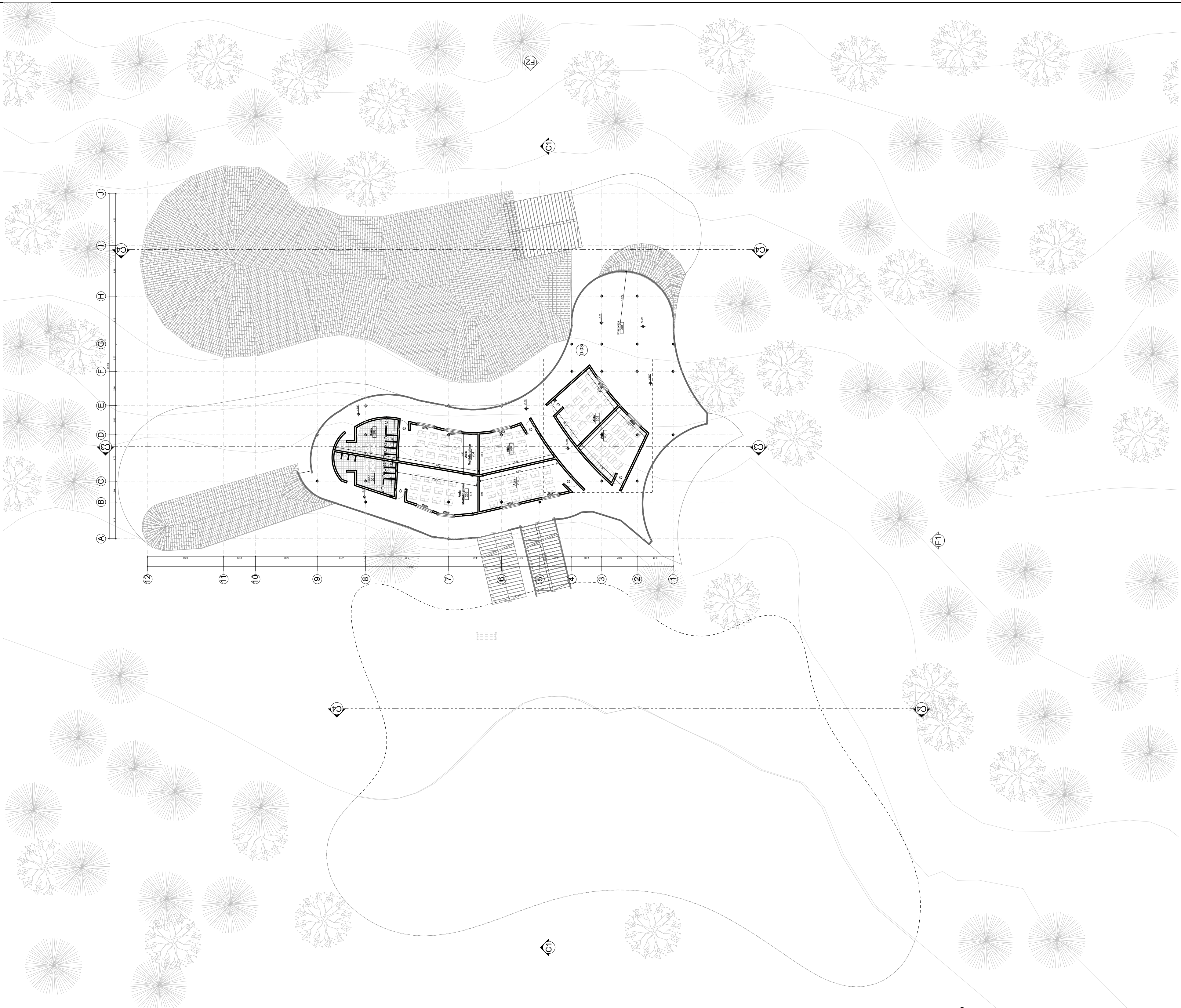
A Implantacion planta 2 esc: 1_200
