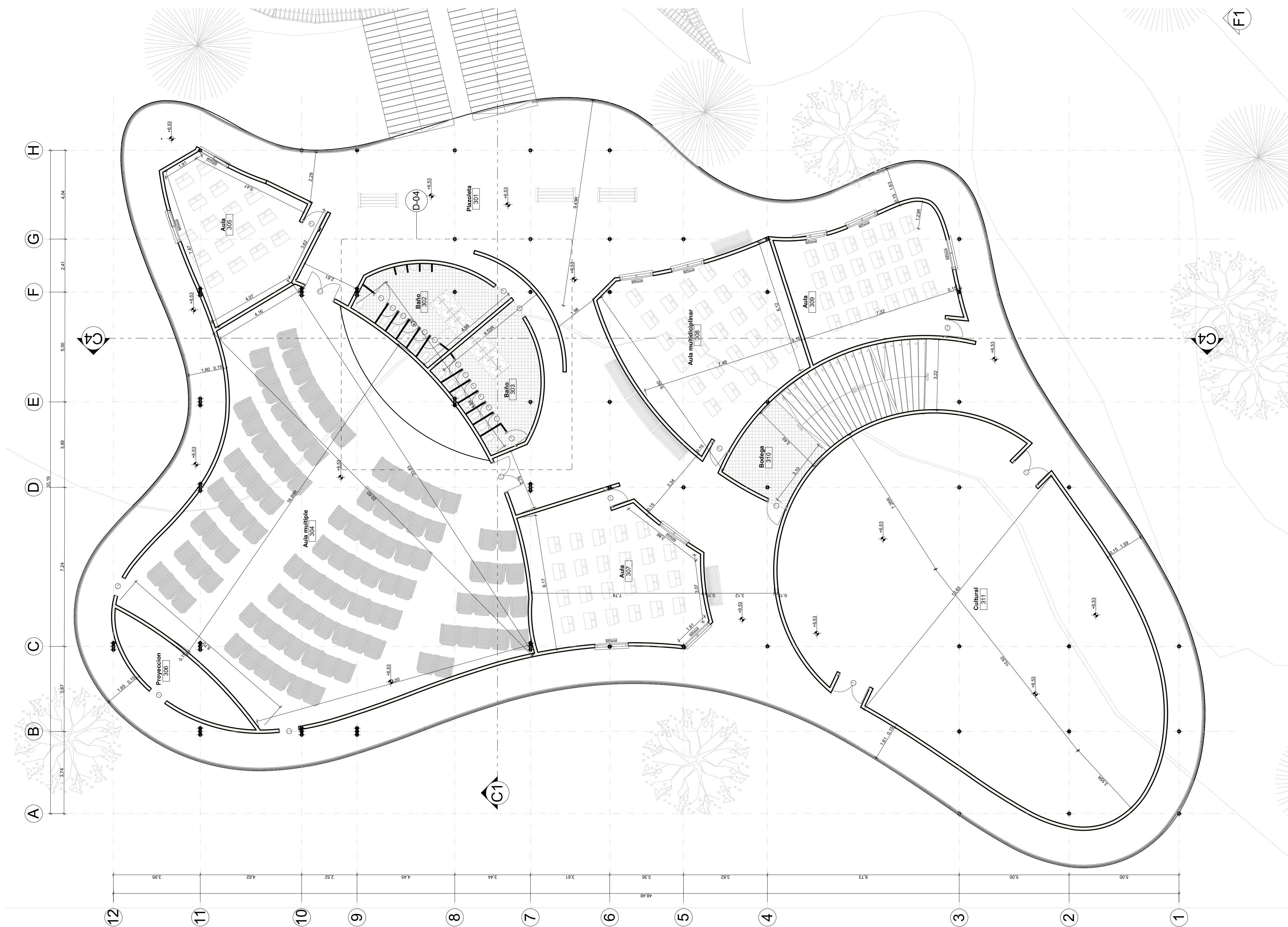
Planta arquitectonica 3 esc: 1_100
