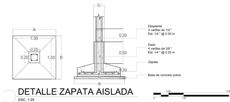
Figura 28 Detalle zapata aislada.
