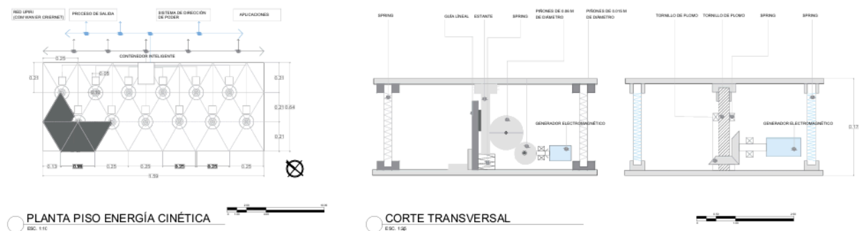
Figura 39 Piso energía cinética.
