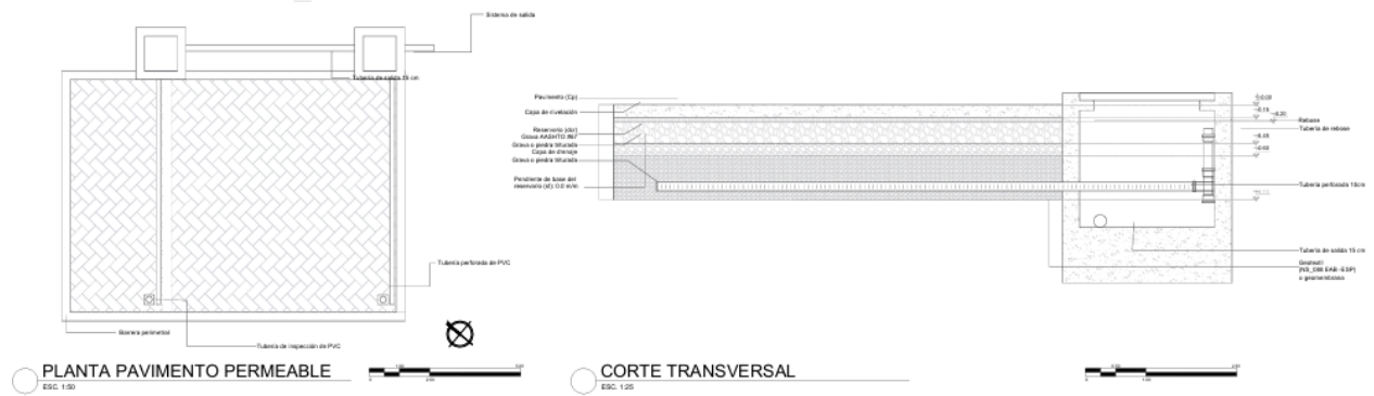
Figura 38 Pavimento permeable
