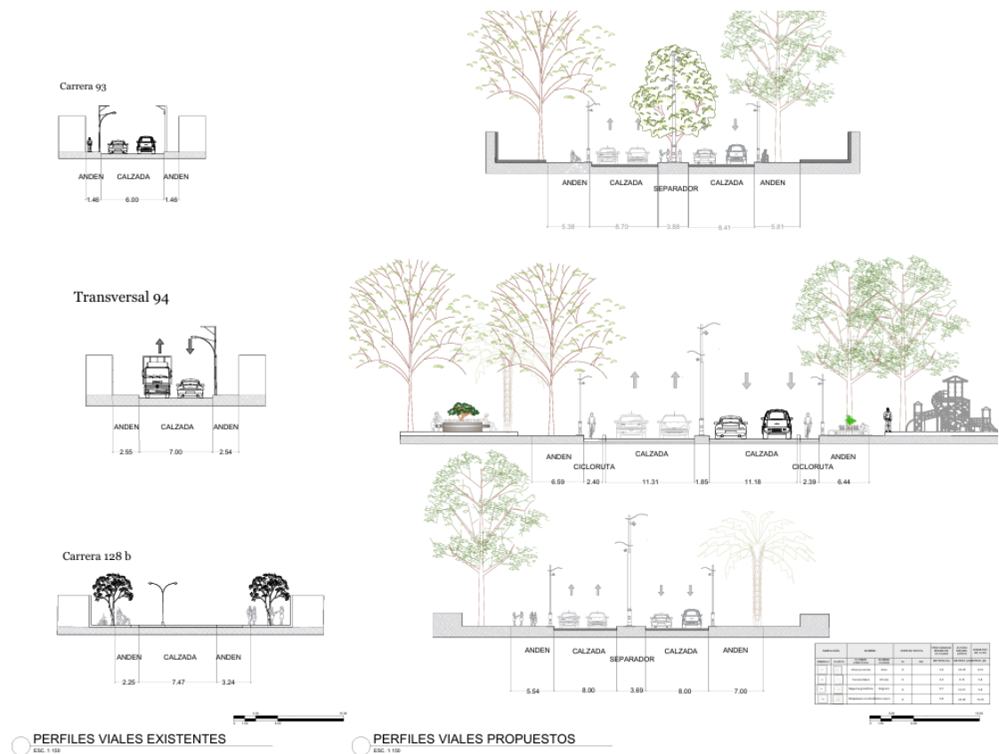
Figura 22 Comparativo de los perfiles viales existentes y los propuestos Nota. Elaboración propia. 2025
