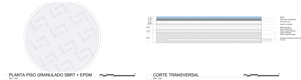
Figura 42 Detalle piso SBRT + EPDM.
