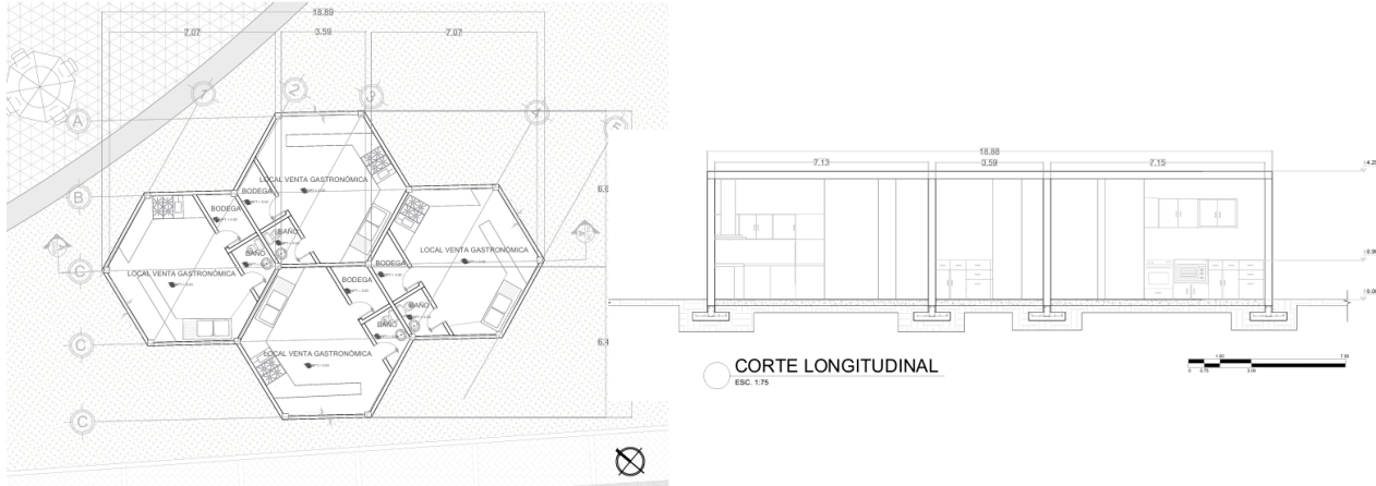
Figura 27 Módulo comercial tipo 3
