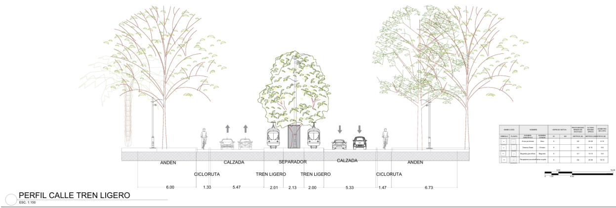
Figura 23 Perfil vial tren ligero.
