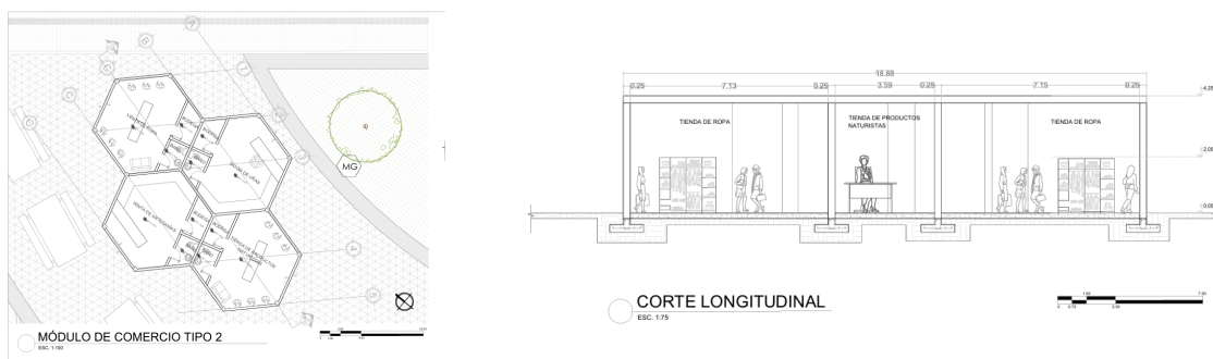
Figura 26 Módulo comercial tipo 2
