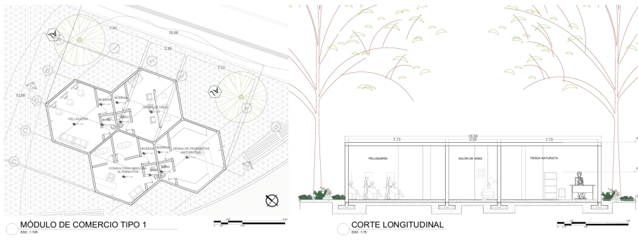
Figura 25 Módulo comercial tipo 1
