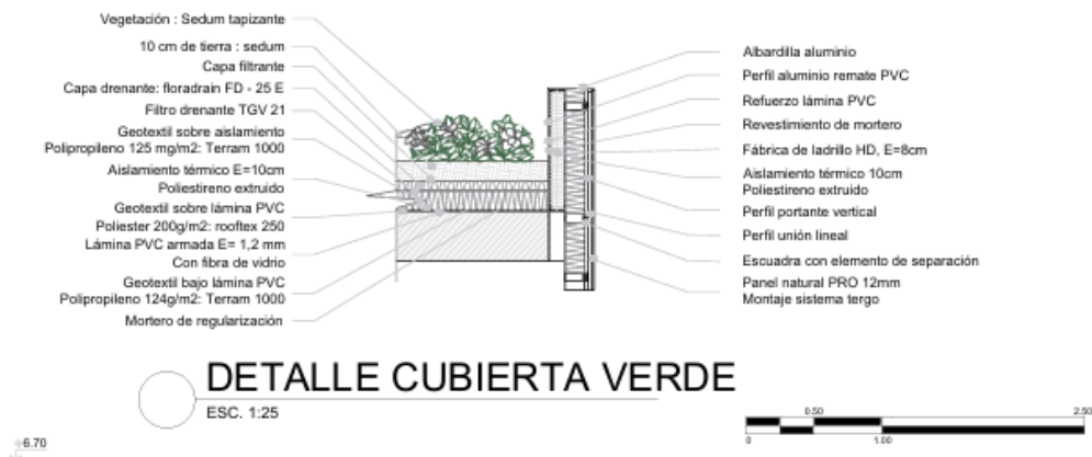
Figura 35 Detalle de cubierta verde
