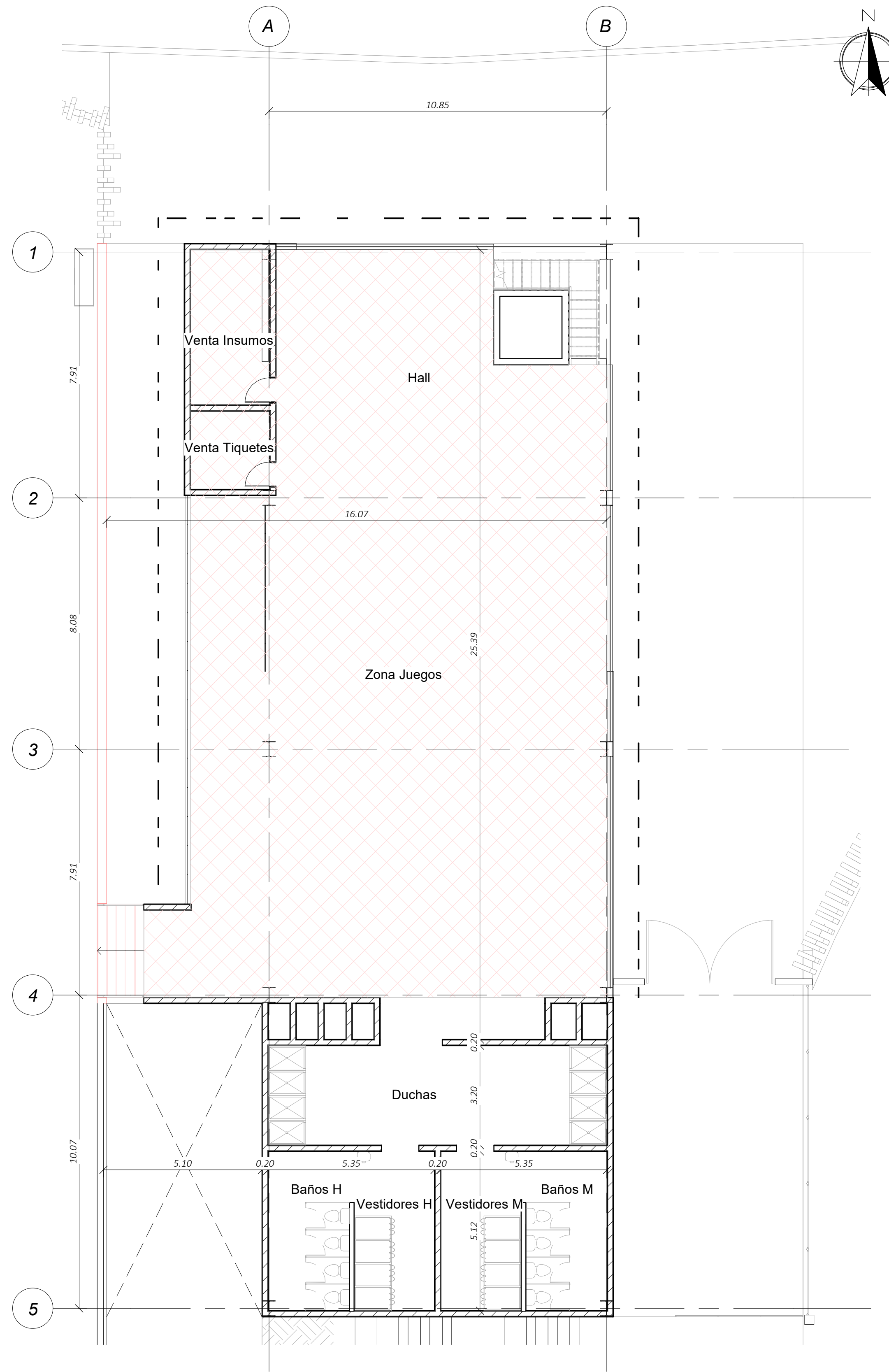
2 Planta Piscina Nivel 1 A100 1 : 100
