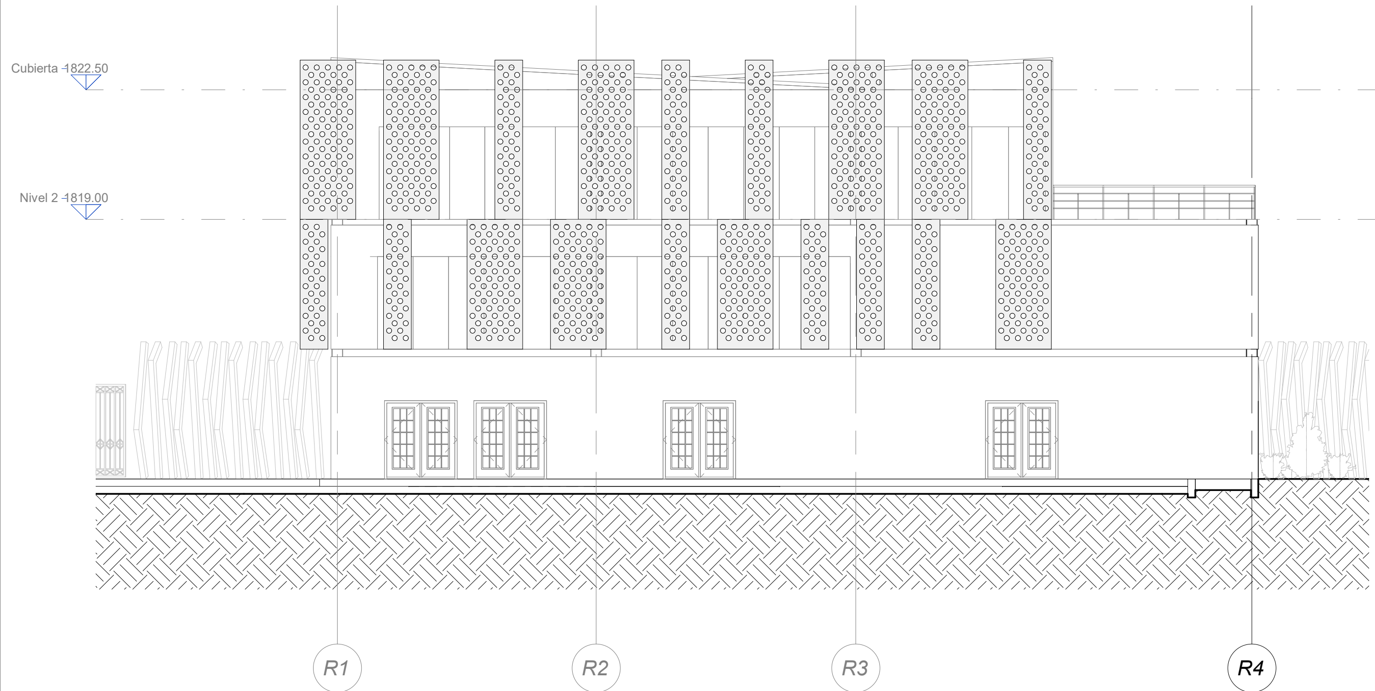
1 Fachada Principal Gimnasio A107 1 : 100
