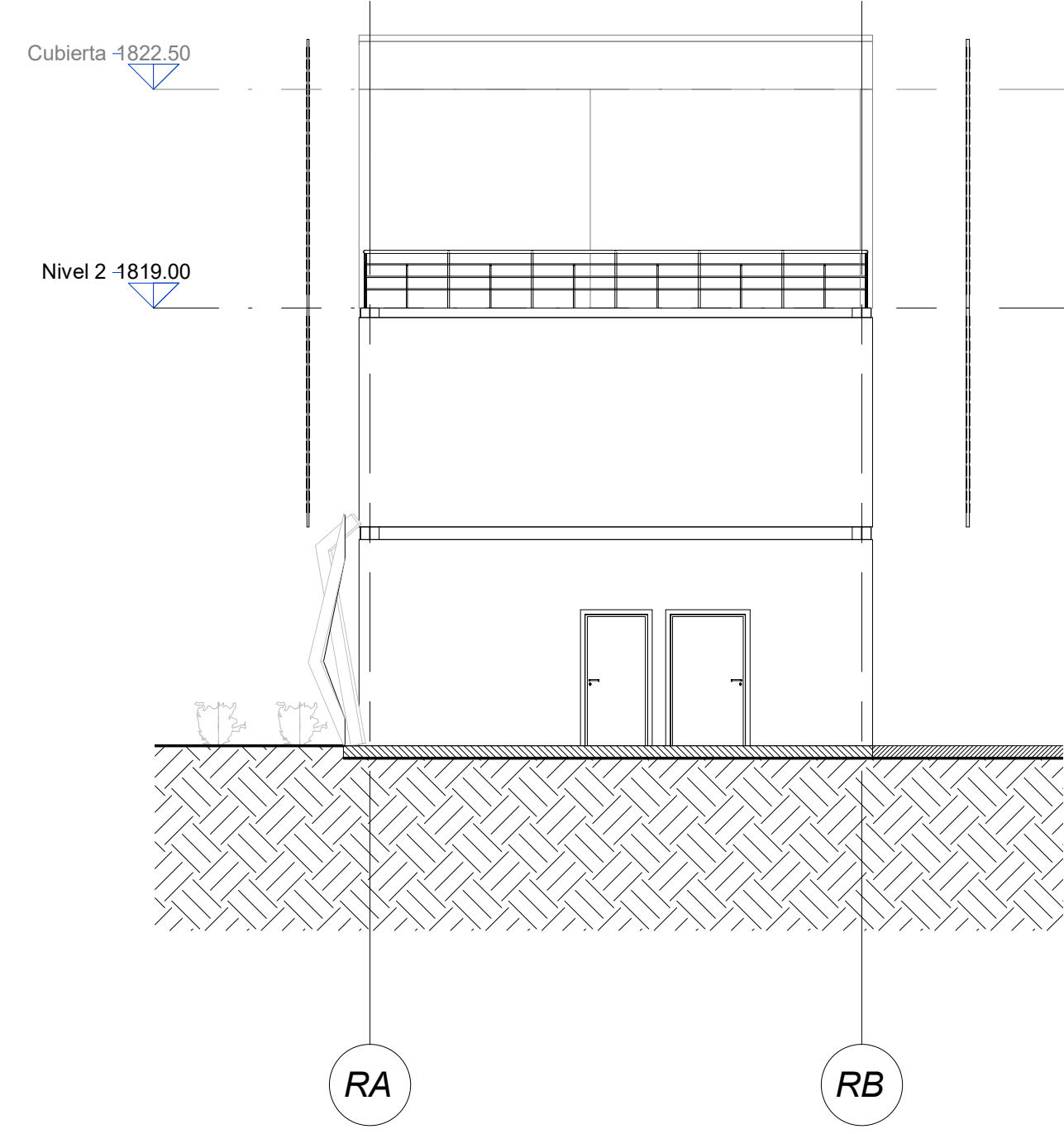
2 Fachada Late. Izquierda Gimnasio A107 1 : 100
