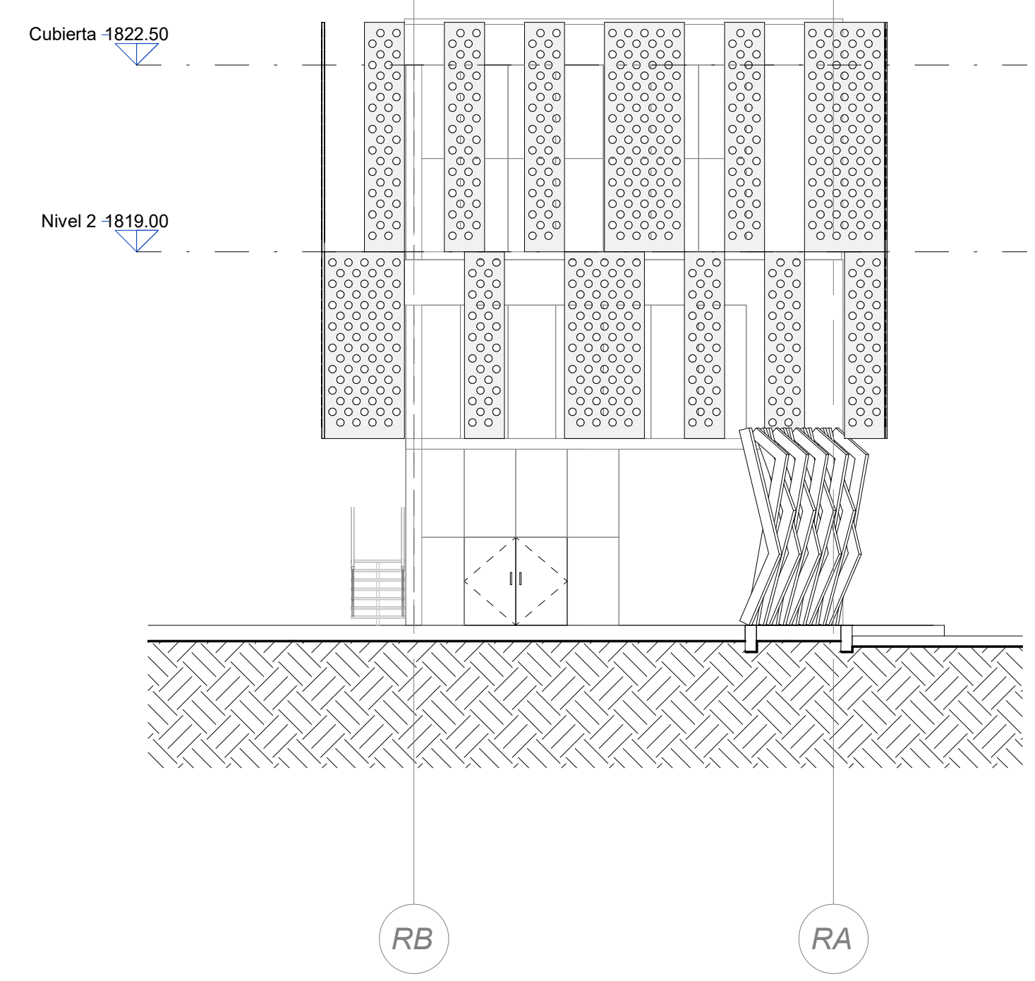
4 Fachada Late. Derecha Gimnasio A107 1 : 100
