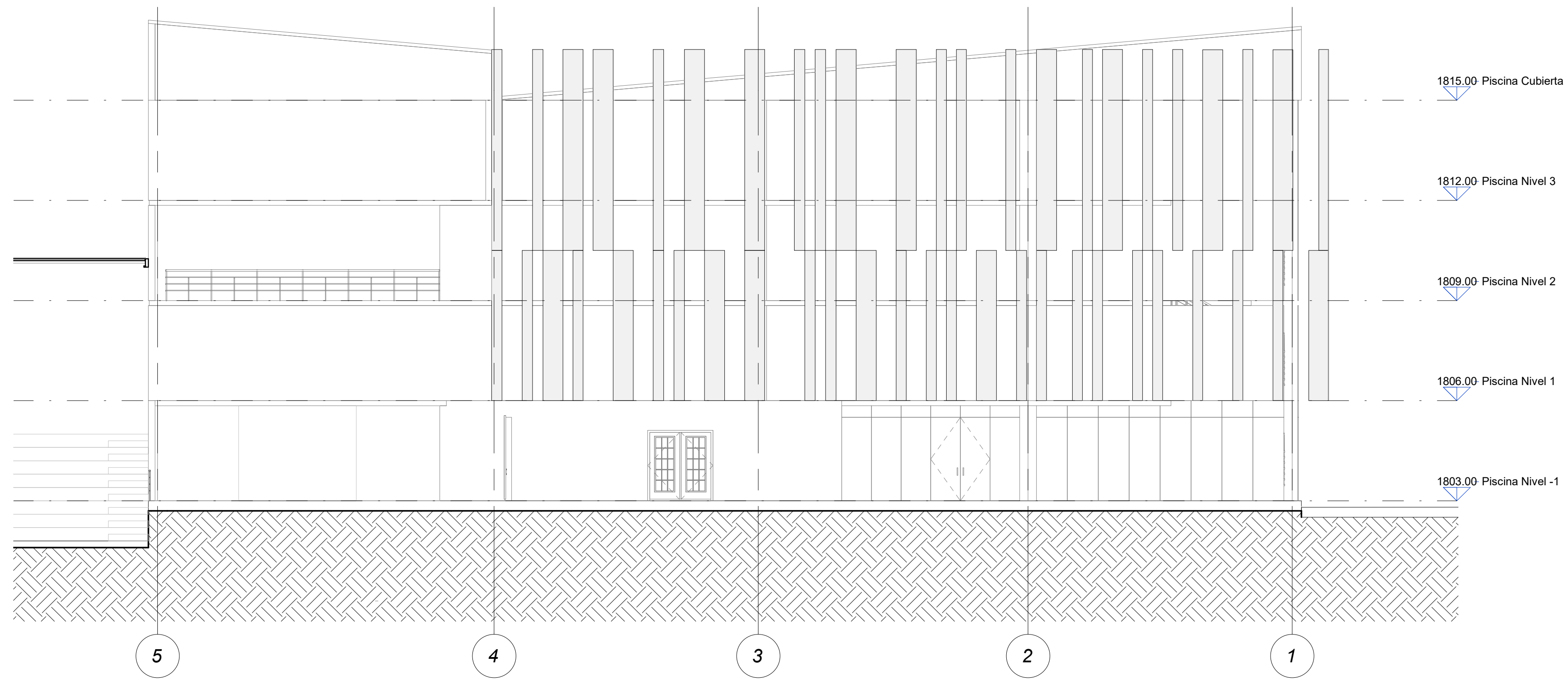
1 Fachada Principal Administración A102 1 : 100
