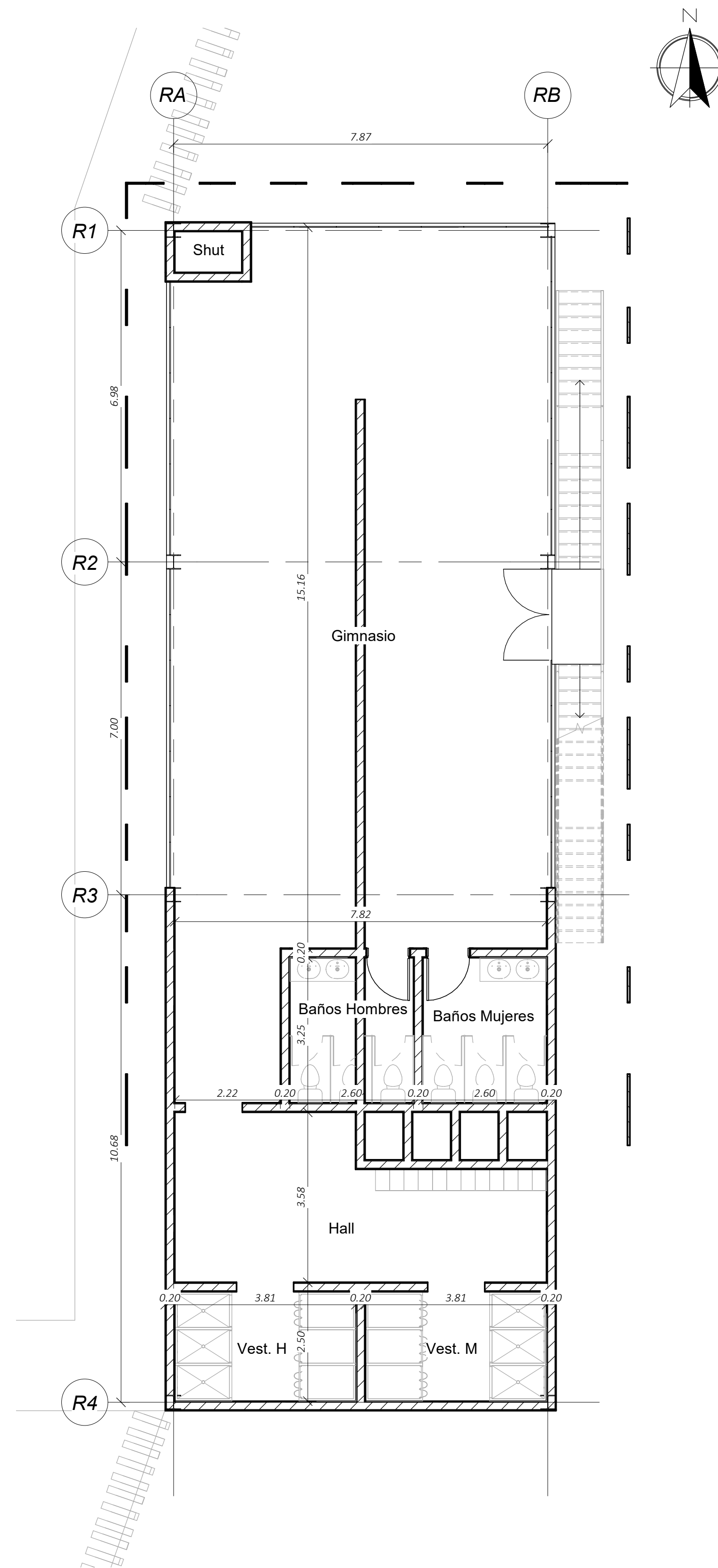
2 Planta Gimnasio Nivel 1 A105 1 : 75
