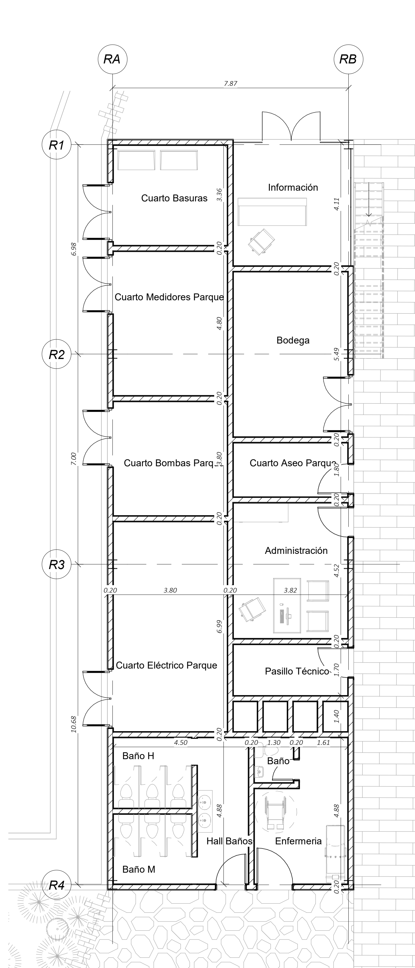
1 Planta Gimnasio Nivel 0 A105 1 : 75
