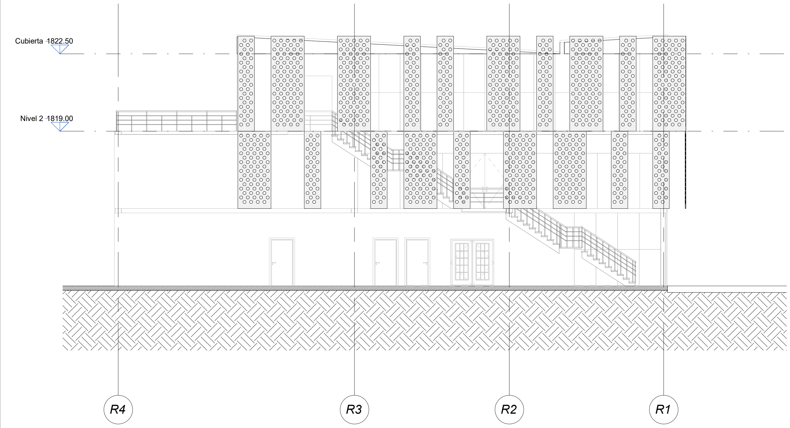
3 Fachada Posterior Gimnasio A107 1 : 100
