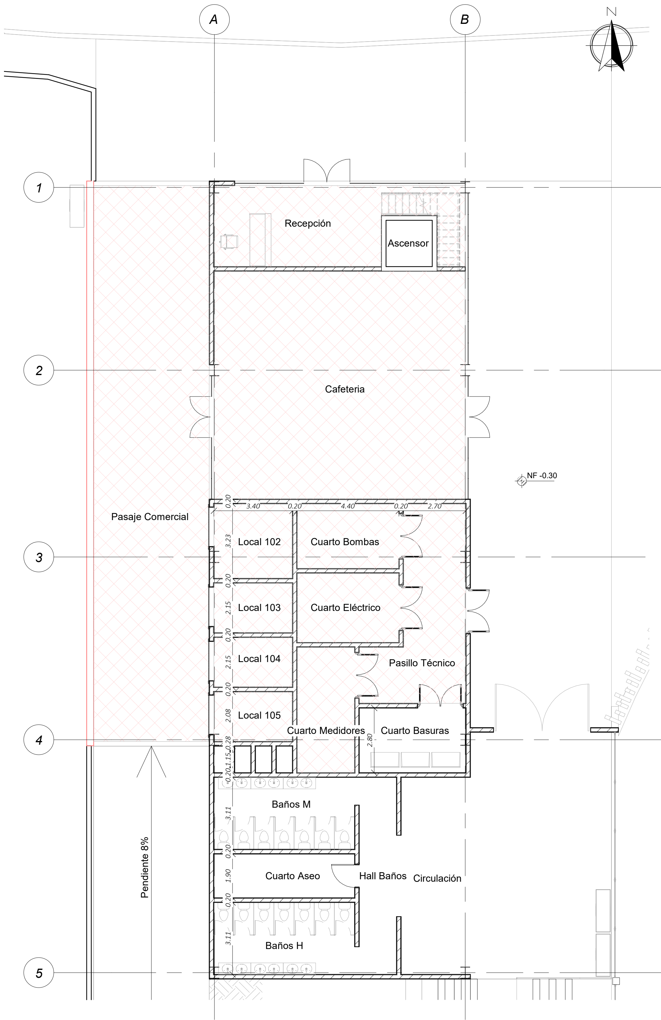
1 Planta Piscina Nivel -1 A100 1 : 100
