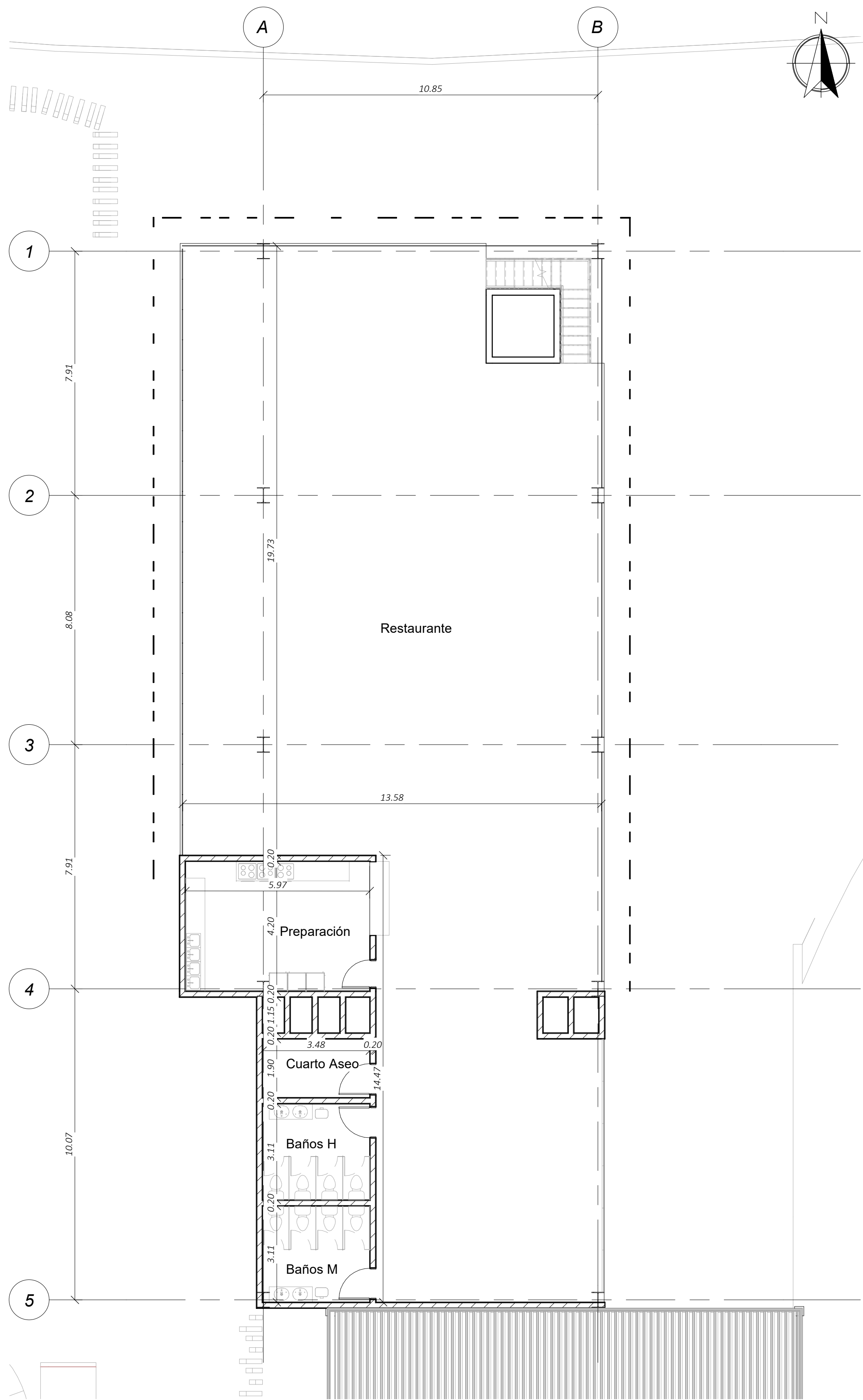
1 A101 Planta Piscina Nivel 2 1 : 100
