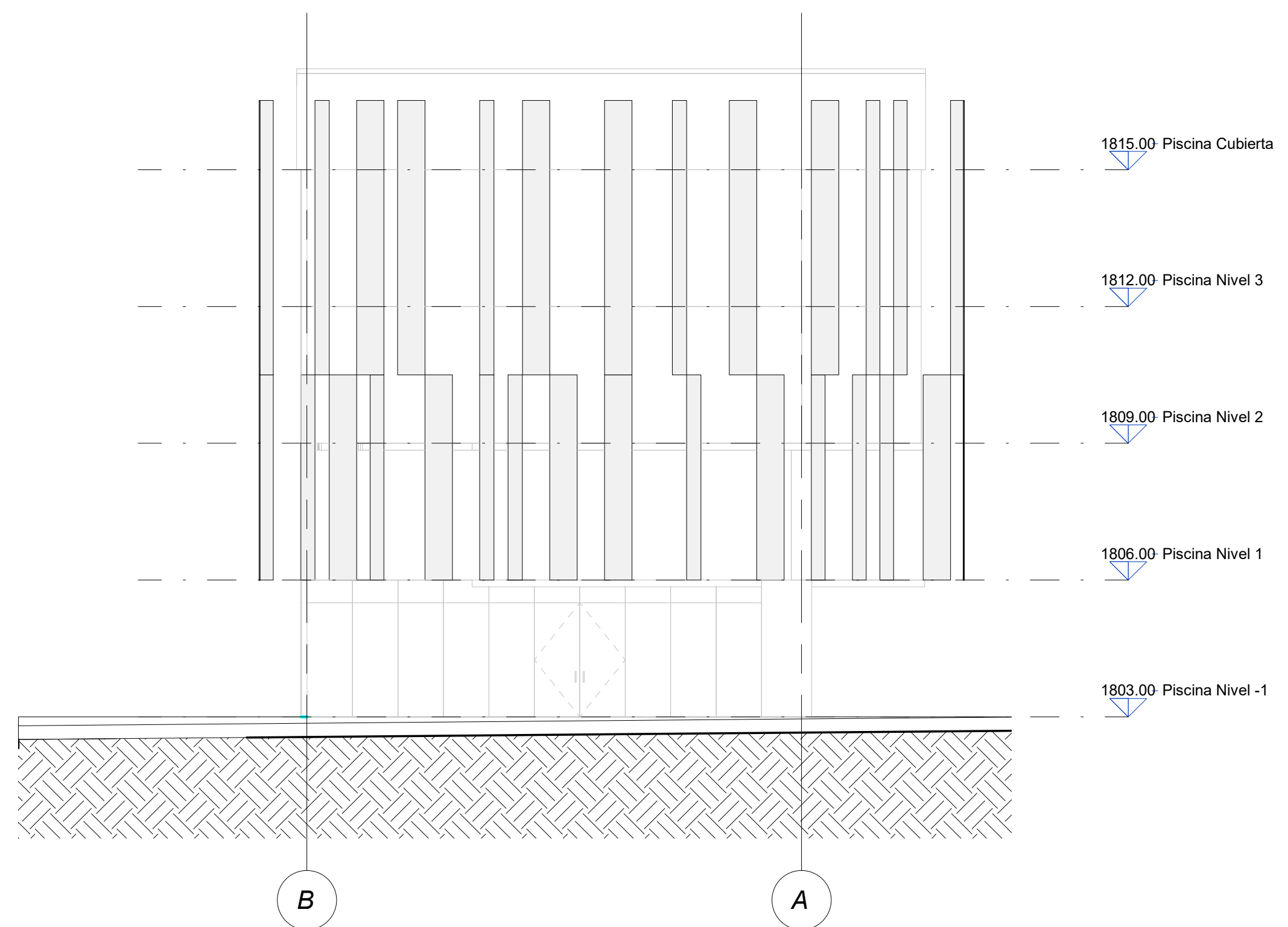
2 Fachada Late. Derecha Administración A102 1 : 100
