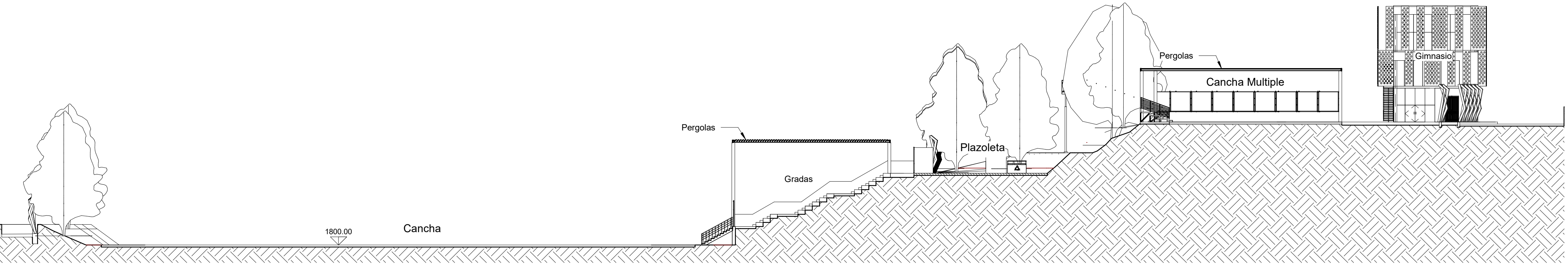
1 Sección Transversal 1 U107 1 : 250
