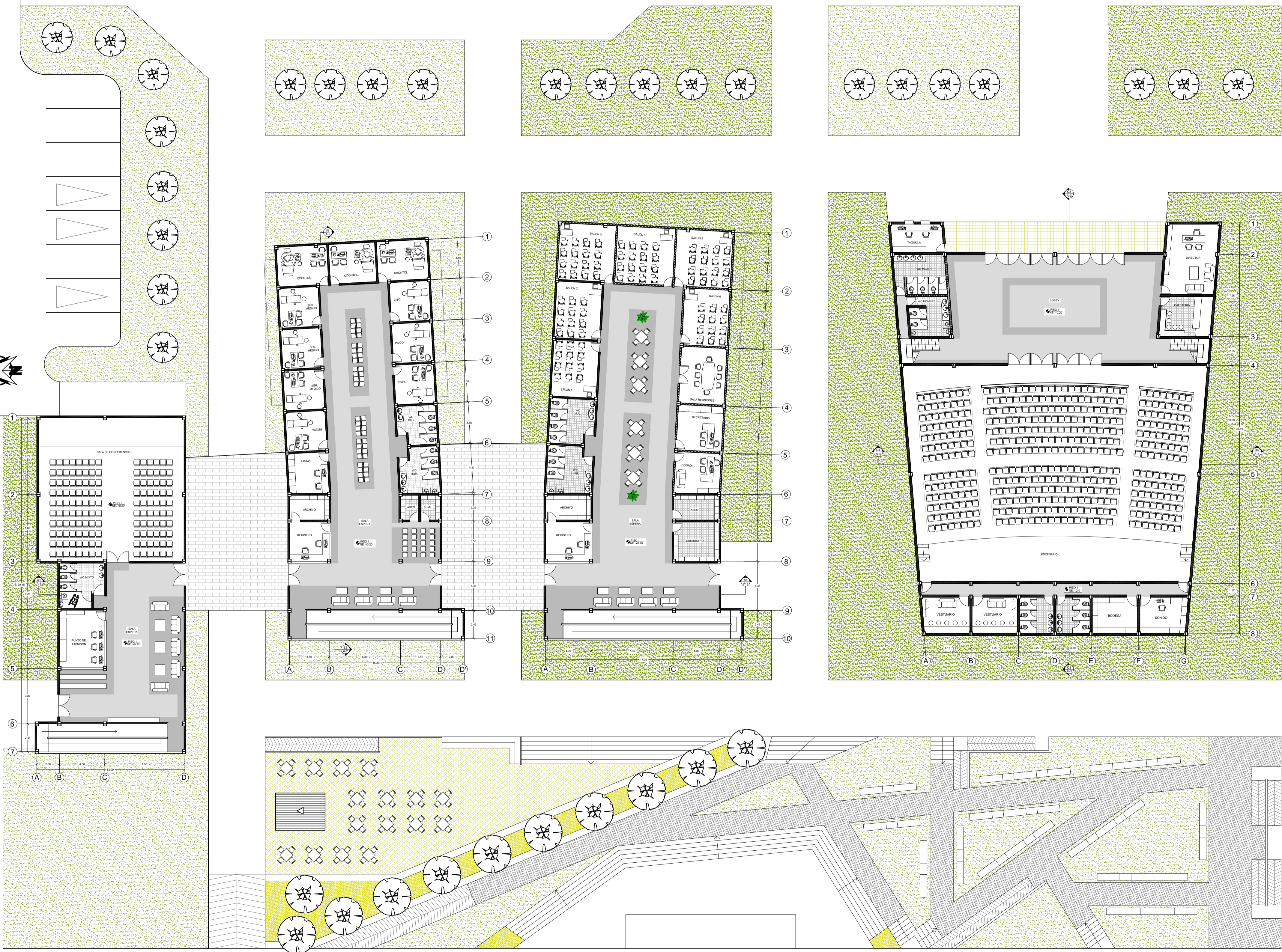
PRIMERA PLANTA, ESC 1:200
