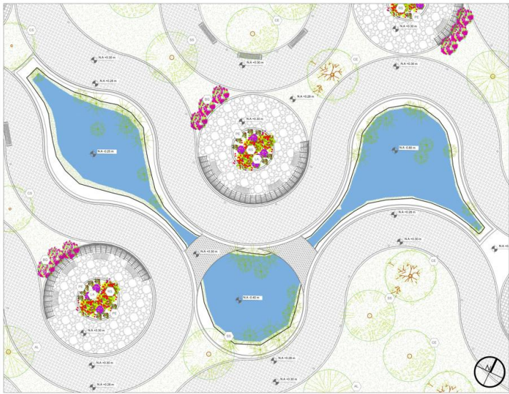
P1 PLANTA GENERAL PONDAJE HÚMEDO ESCALA 1:200 0 4.00 8.00 20.00
