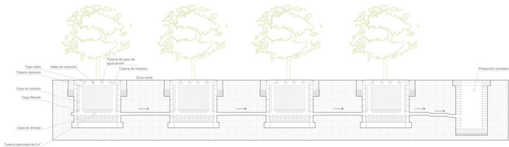
C1 DETALLE CONSTRUCTIVO - ALCORQUE
