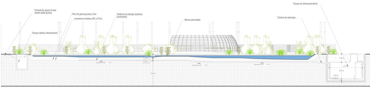
C1 DETALLE CONSTRUCTIVO PONDAJE HÚMEDO ESCALA 1:50 0 0.50 1.00 7.00
