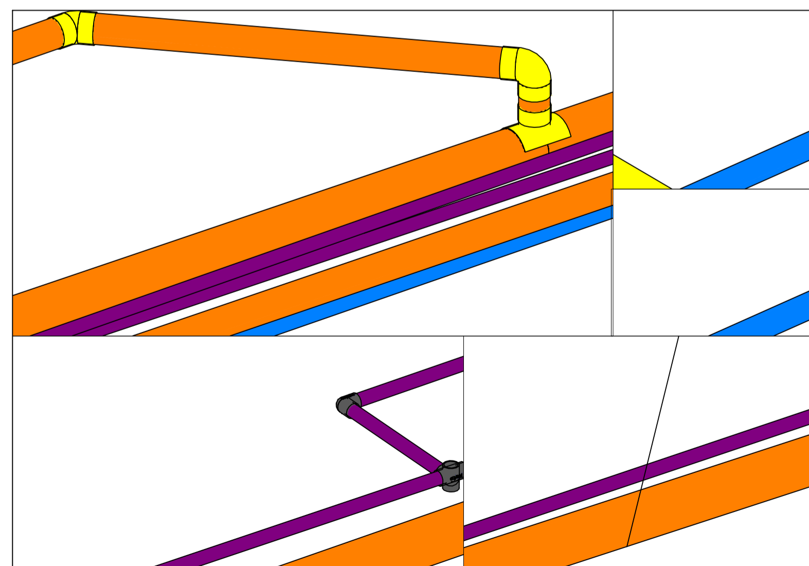
D2 DETALLE CONEXIONES HIDRAULICAS ESCALA 1:20 0 0.4 0.8 1.2 1.6 2.0 m ESCALA A 120
