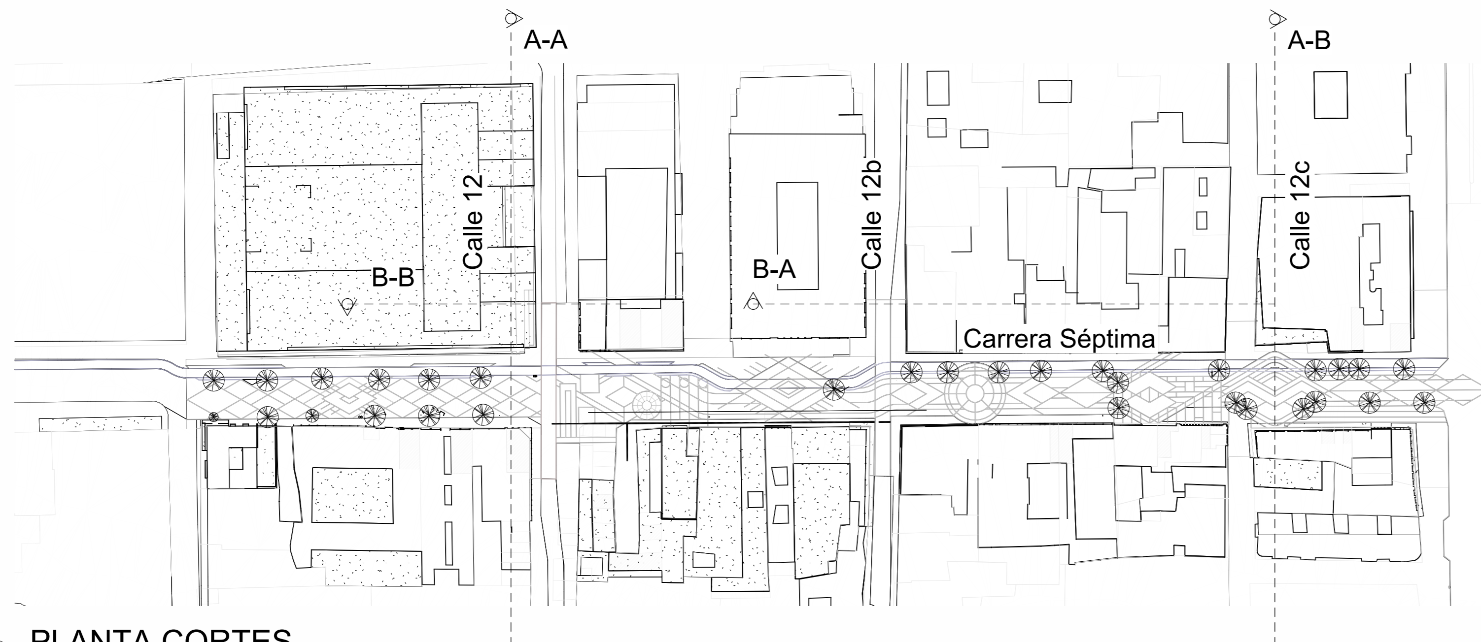
7 PLANTA CORTES 1 : 1200
