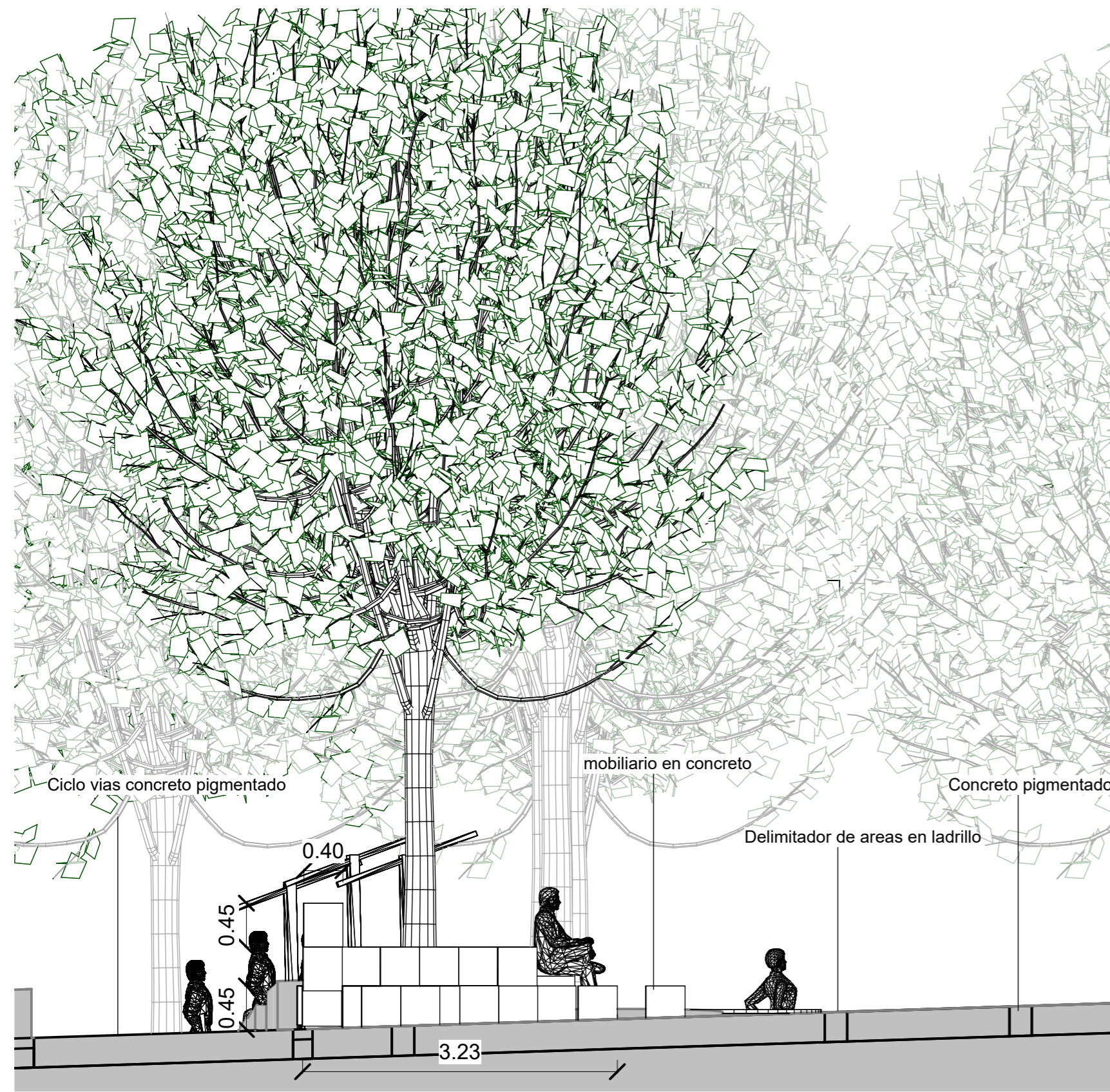
1 Mobiliario fijo calle 12 1 : 50
