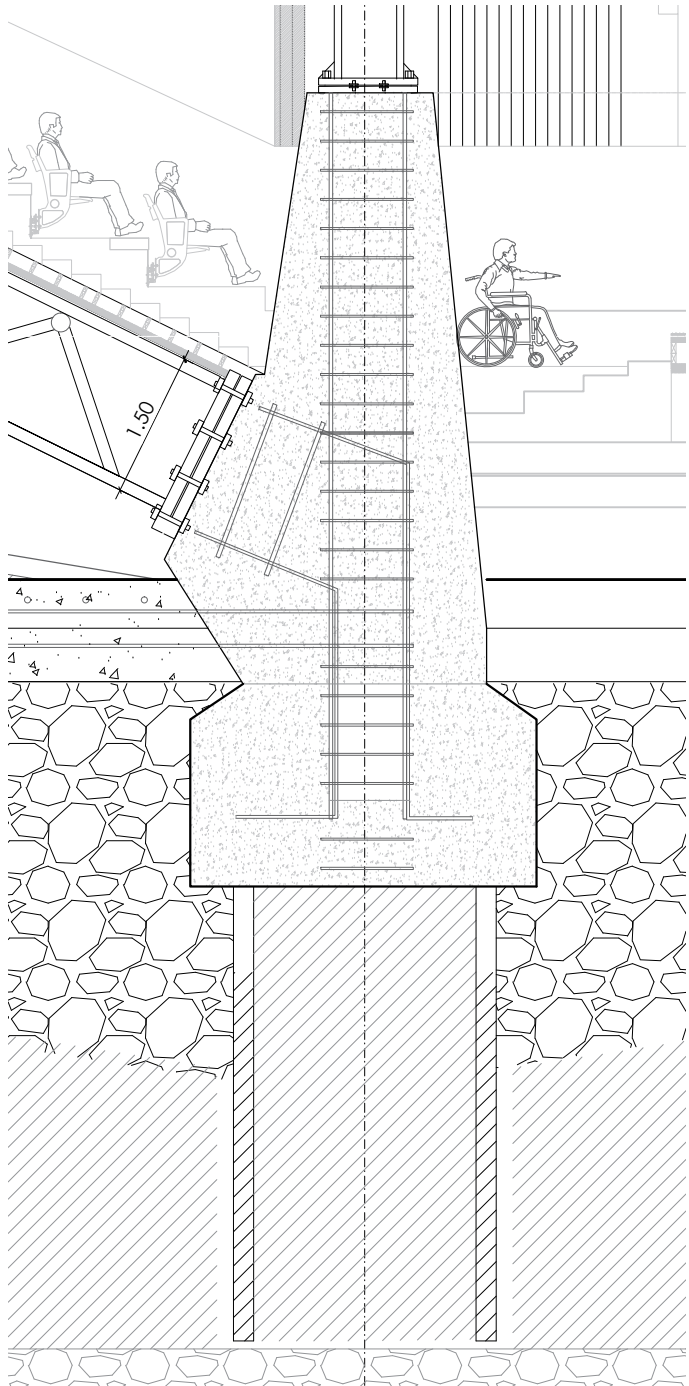
DETALLE 4 - DE PEDESTAL
