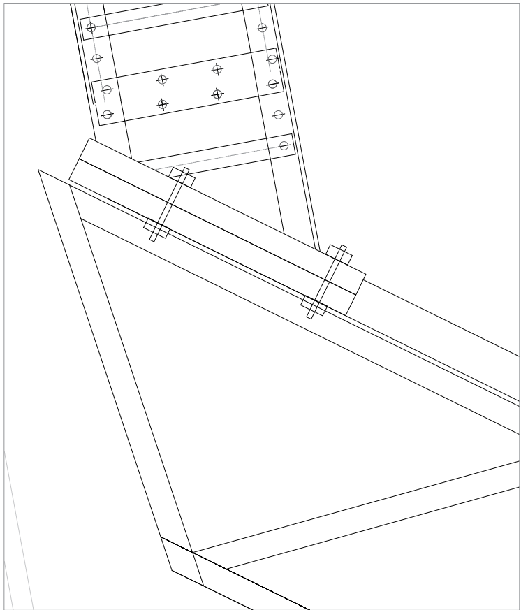
DETALLE 3-ANCLAJE VIGA VIERENDEL
