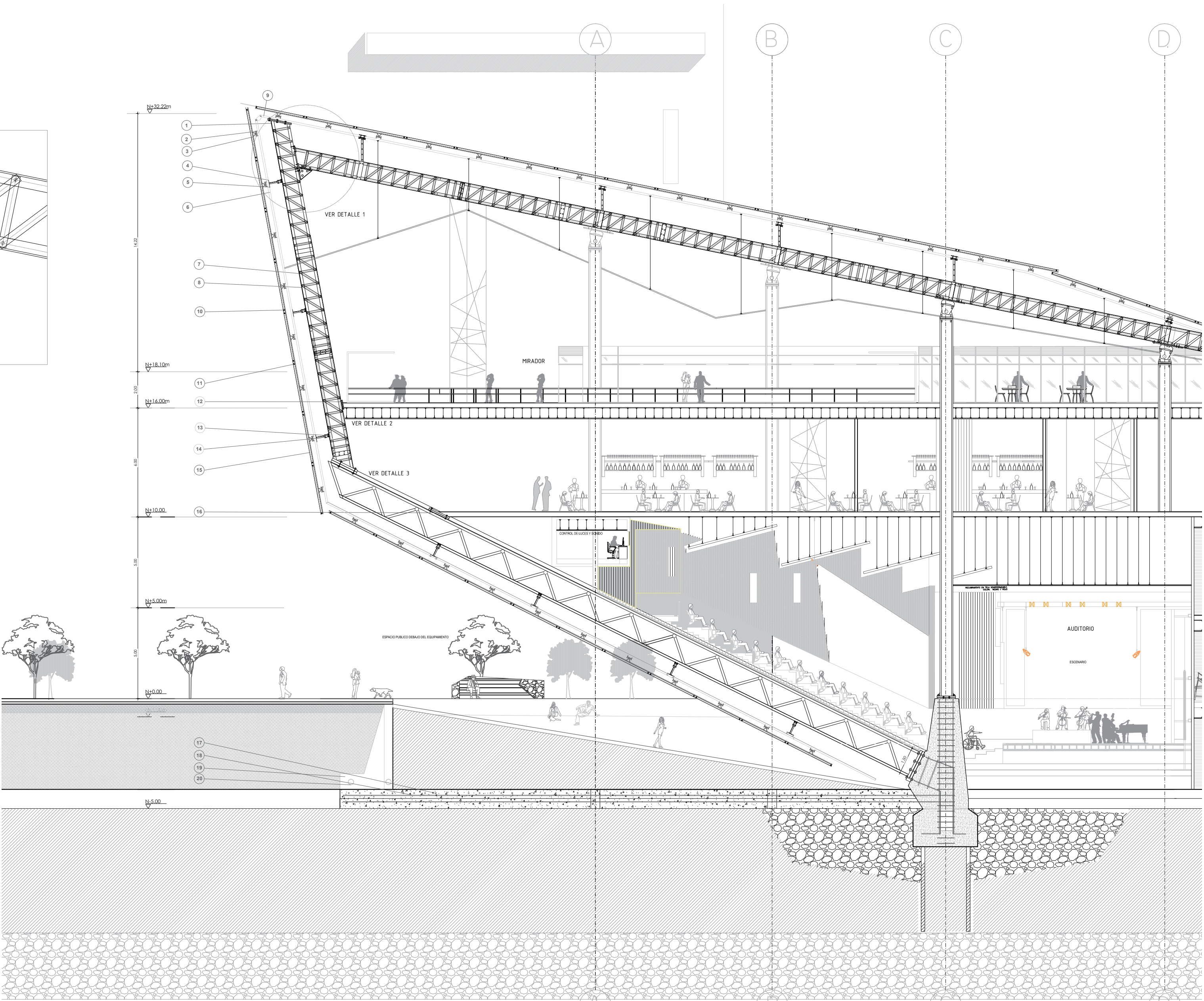
CORTE B-B
