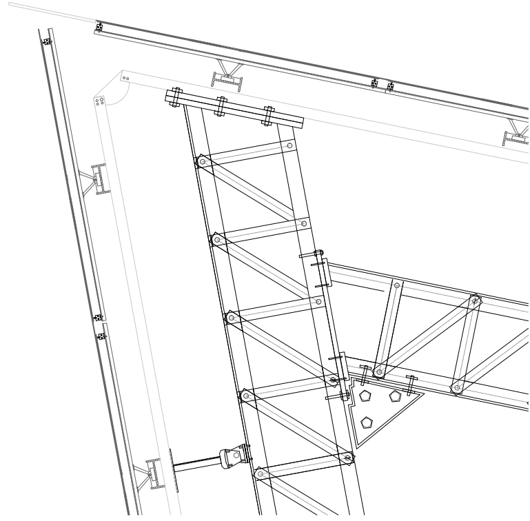
DETALLE 1 -CUMBRERA
