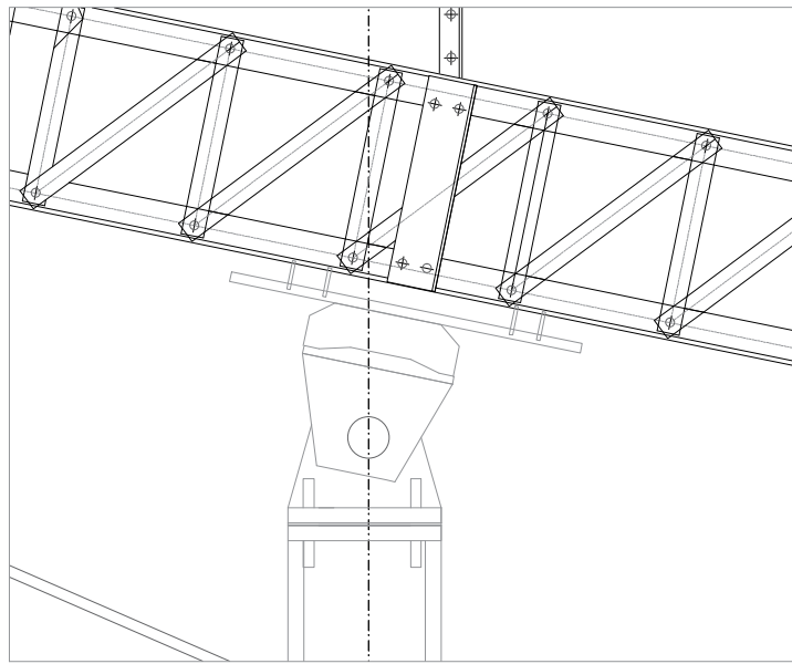
DETALLE 5 - DE ANCLAJE CUBIERTA
