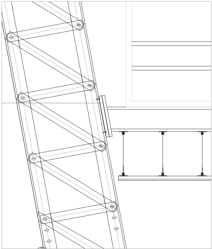
DETALLE 2-ANCLAJE ENTREPISO
