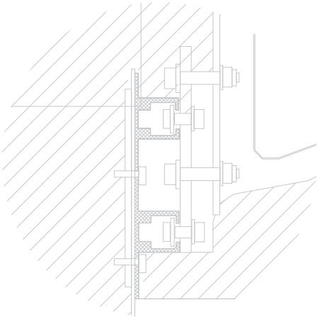
DETALLE 6 -ANCLAJE DE SILLA
