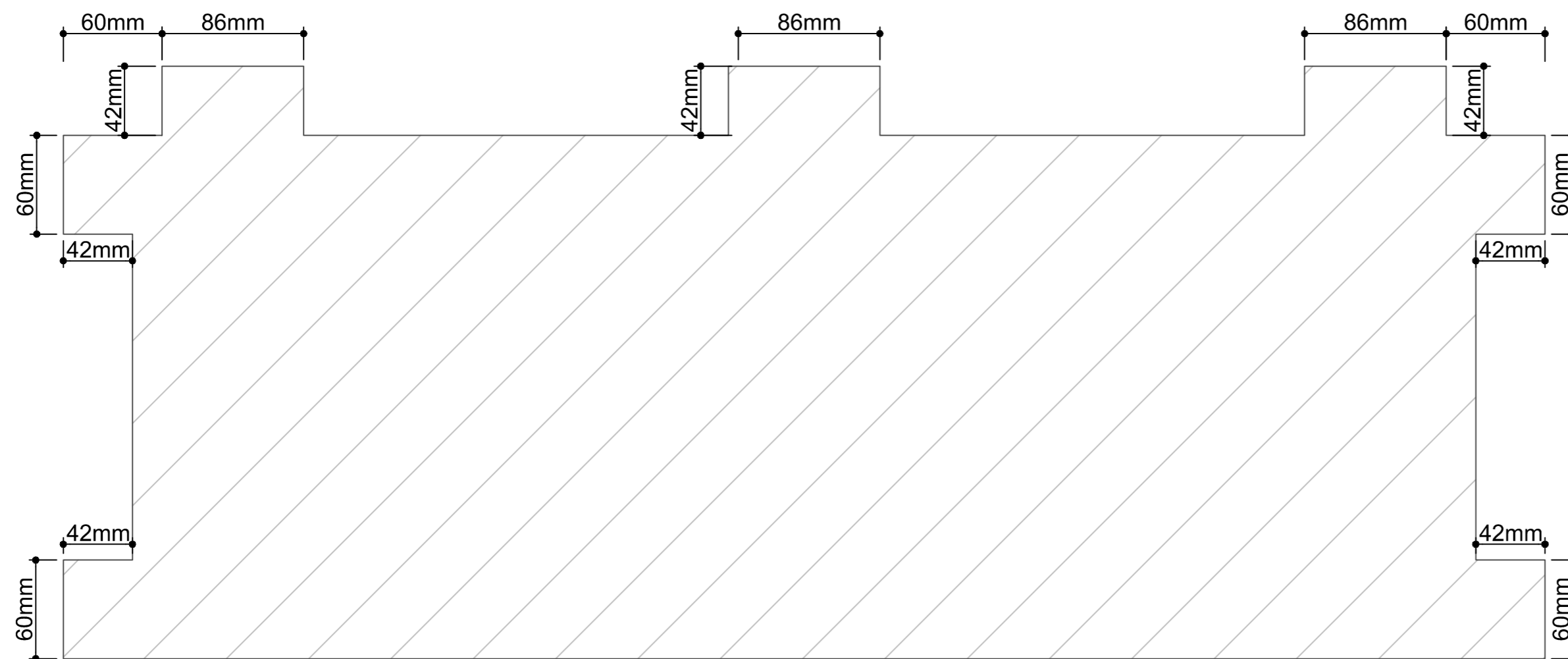
DIMENCIONES DE DETALLE CASETÓN PLEGABLE PROTOTIPO A1 Esc 1 : 5
