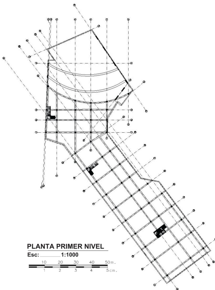
Ilustración 32 Planta Estructural Primer Piso Volumen 1°
