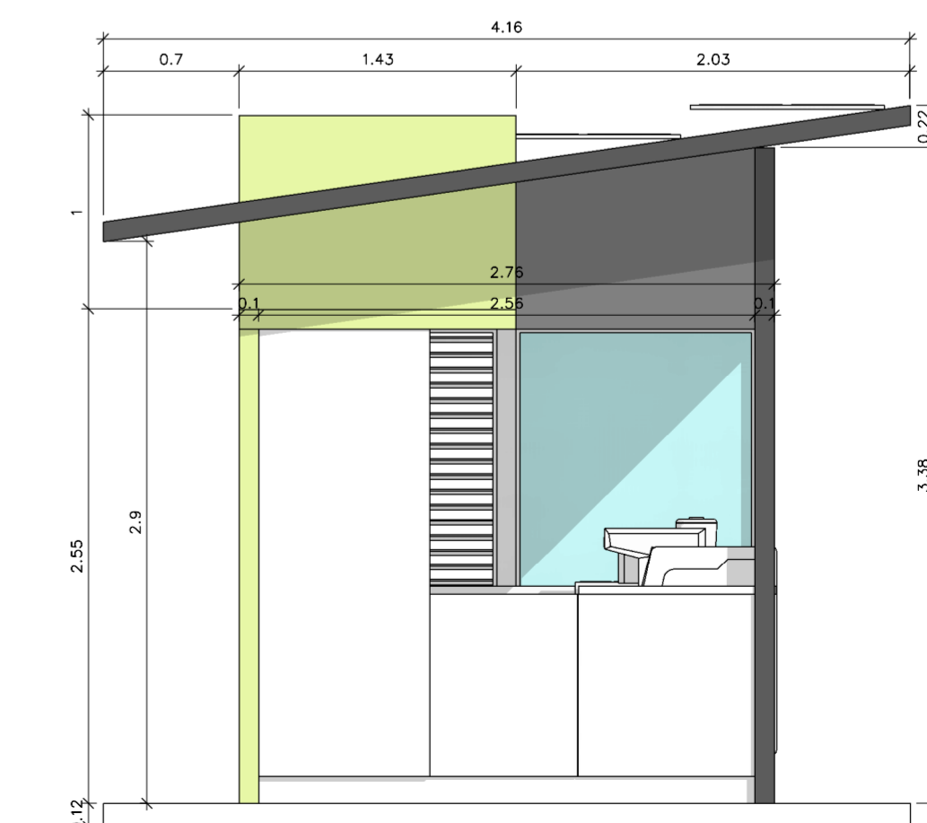
FACHADA LATERAL IZQUIERDA
