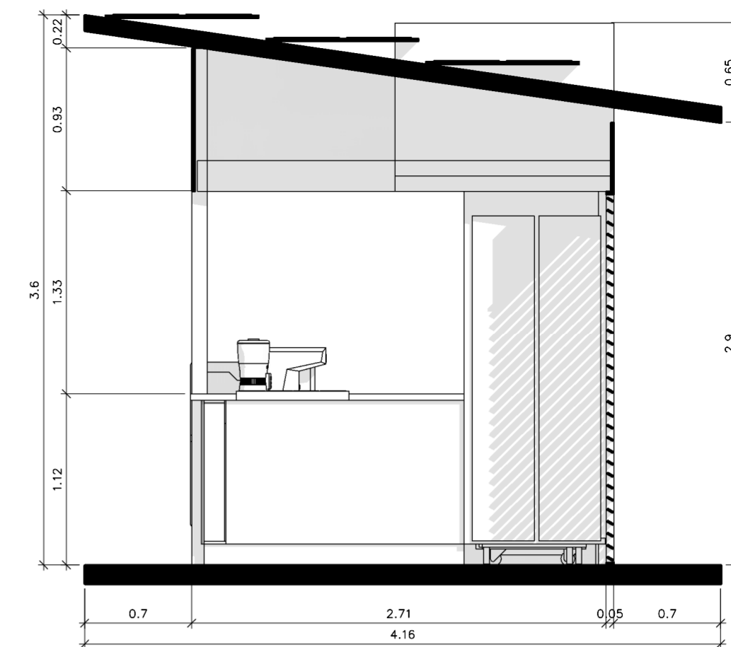
CORTE TRANSVERSAL
