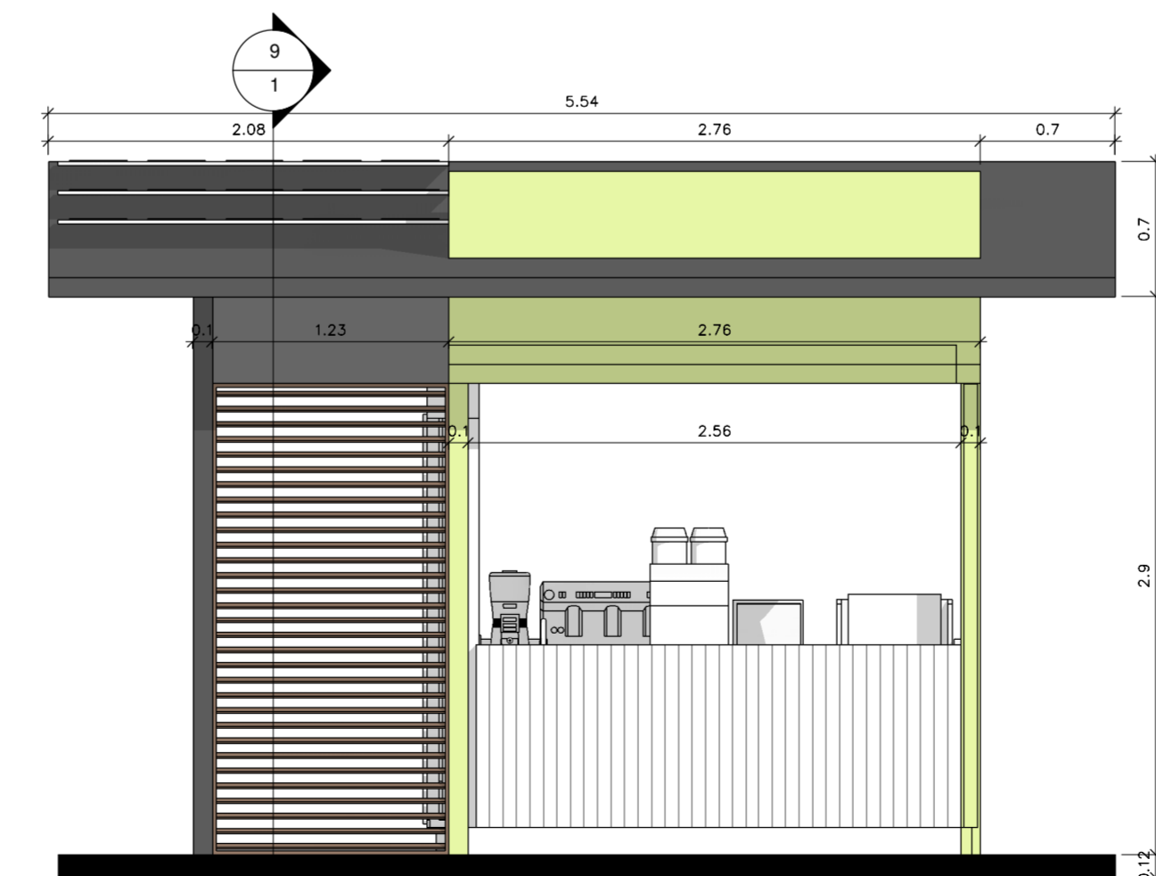
FACHADA POSTERIOR
