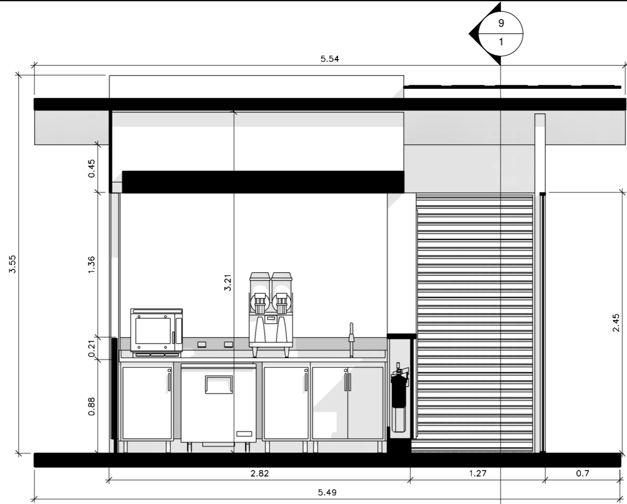
CORTE LONGITUDINAL
