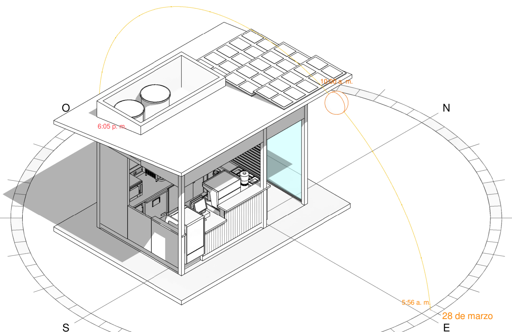
ISOMETRICO ASOLEACION
