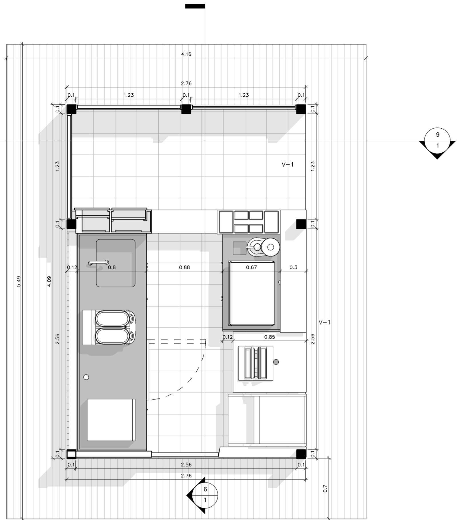
PLANTA GENERAL
