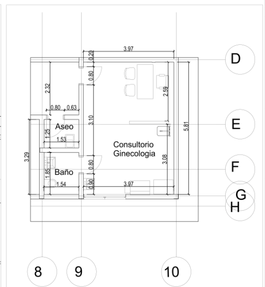
PG AMPLIACION 1 ESCALA 1:50
