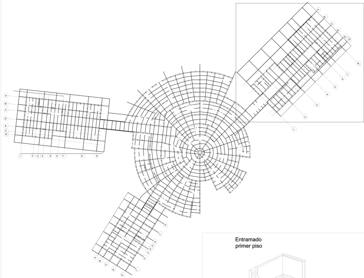
PG ENTRAMADO LIGERO EN MADERA ESCALA 1:2000
