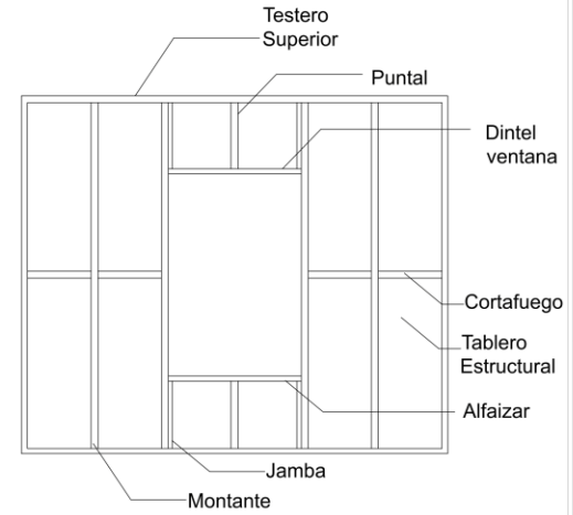
PG ENTRAMADO MURO ESCALA 1:1
