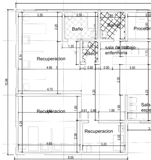
PG AMPLIACION ESCALA 1:100
