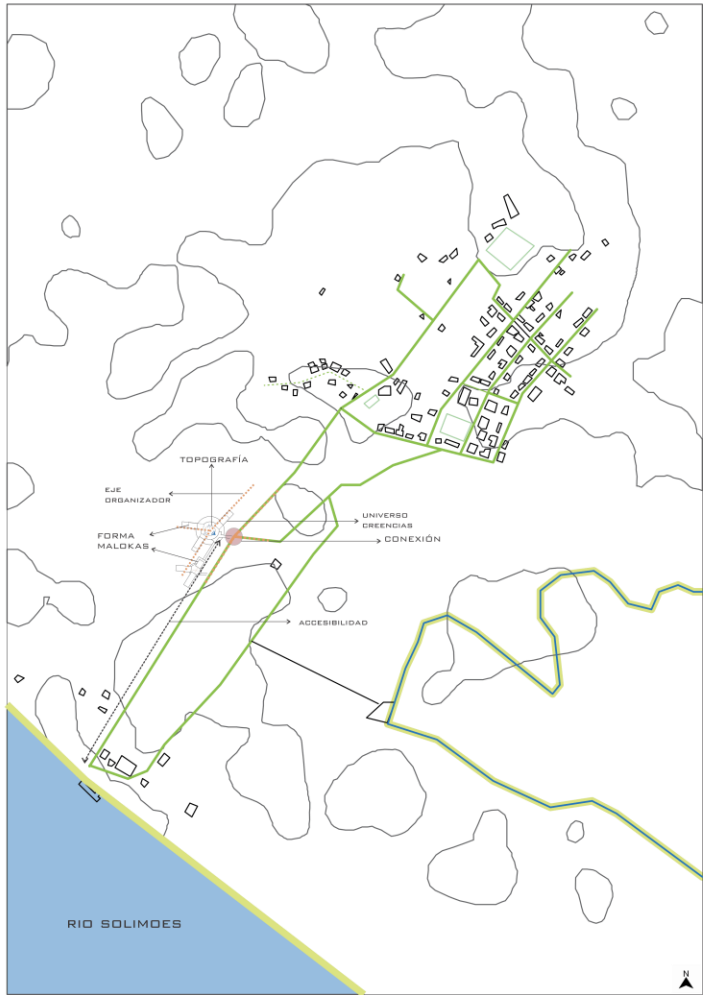
PG CRITERIOS LOCALIZACION ESCALA 1:500
