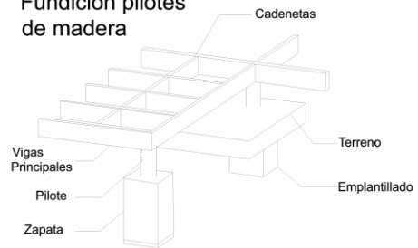
DT DETALLES PILOTES ESCALA 1
