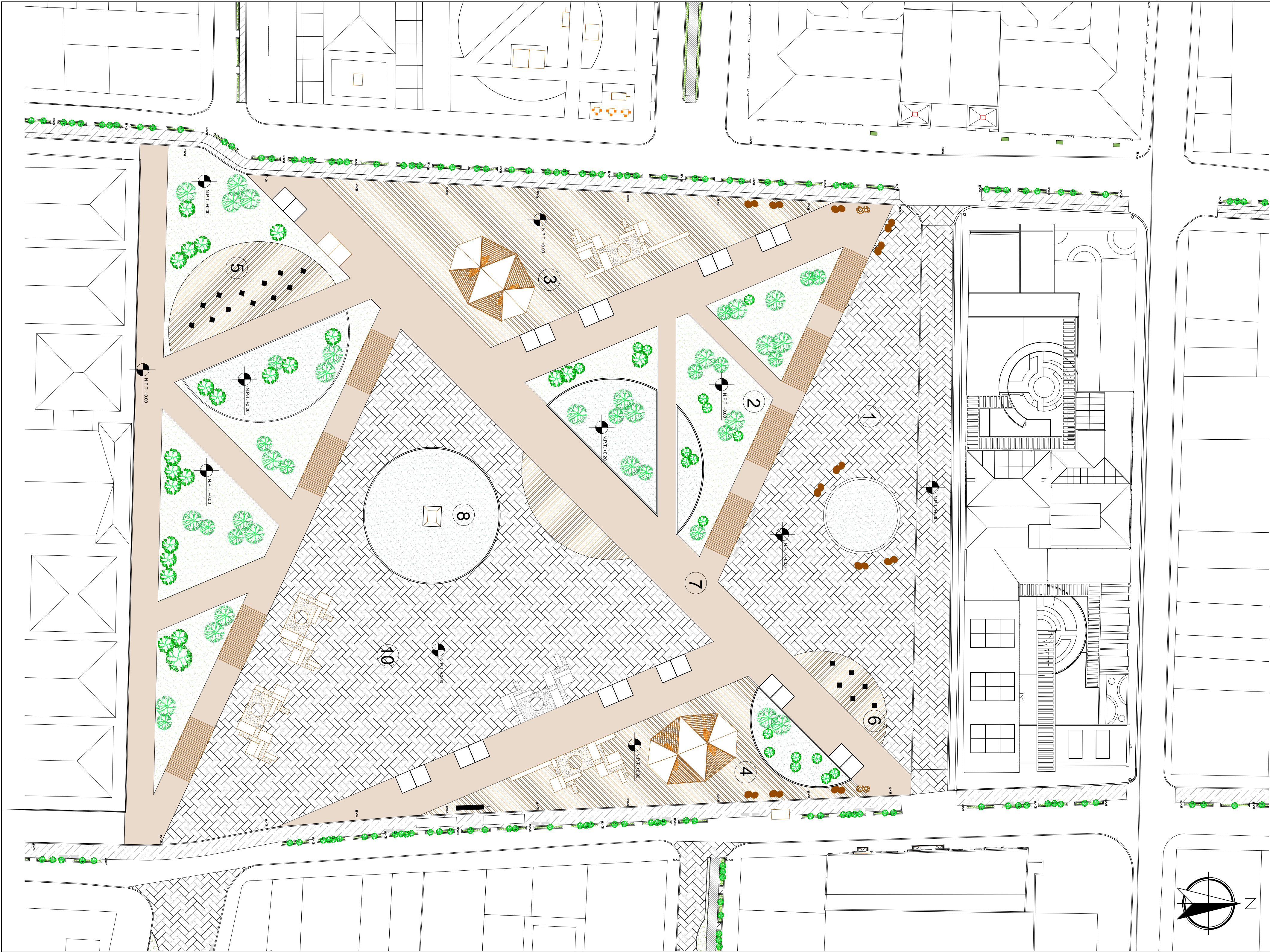
1 PLANTA URBANA PLAZA ESPAÑA ESC 1:500 0 5 10m ESCALA GRAFICA
