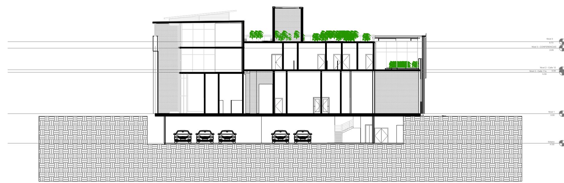
1 CORTE A-A ESC 1:300 0 5 10m ESCALA GRAFICA
