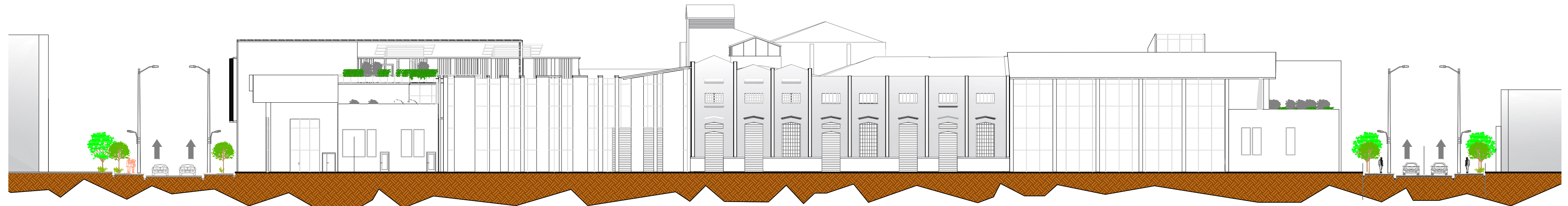
2 FACHADA CALLE 12 ESC 1:300 0 5 10m ESCALA GRAFICA
