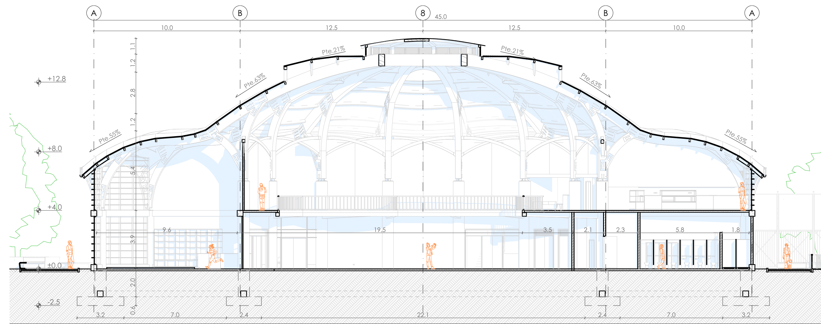
SC2 Sección Escala 1:150
