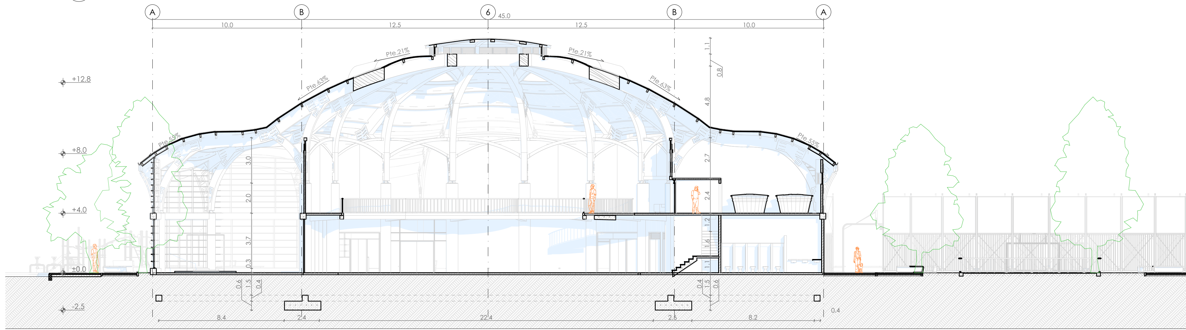
SC2 Sección Escala 1:150
