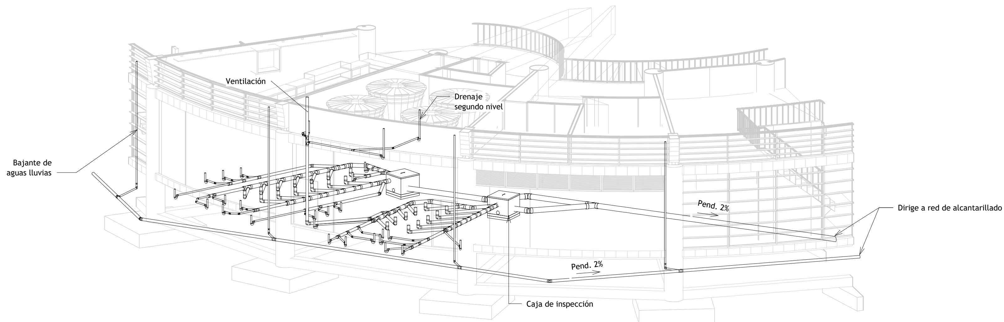
3 Axonometría
