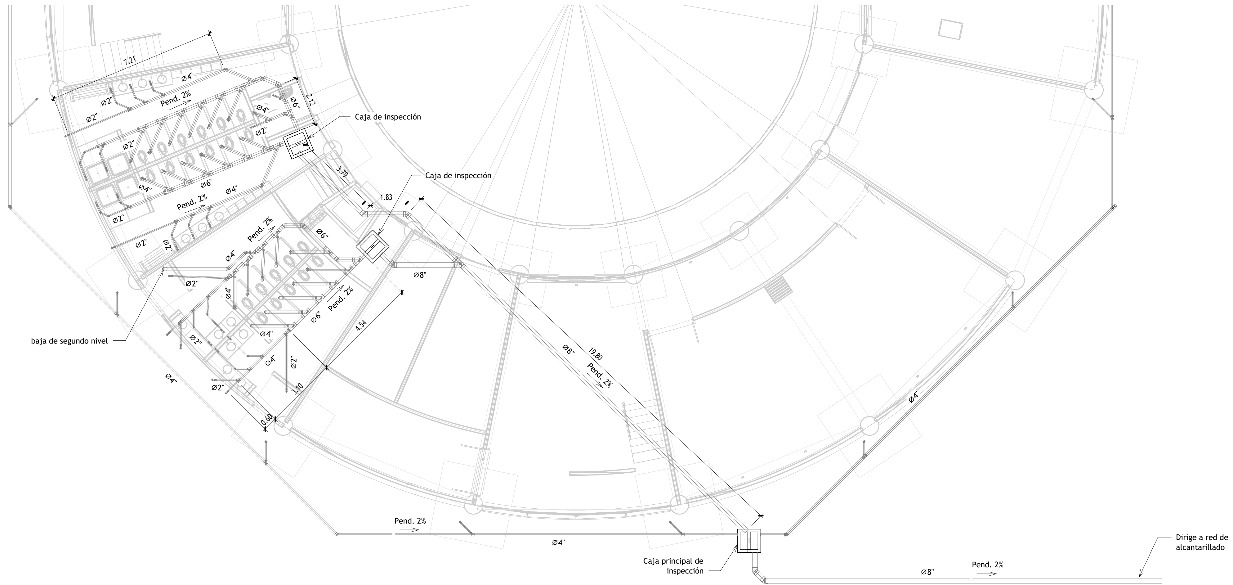
1 Planta Primer Nivel 1 : 100
