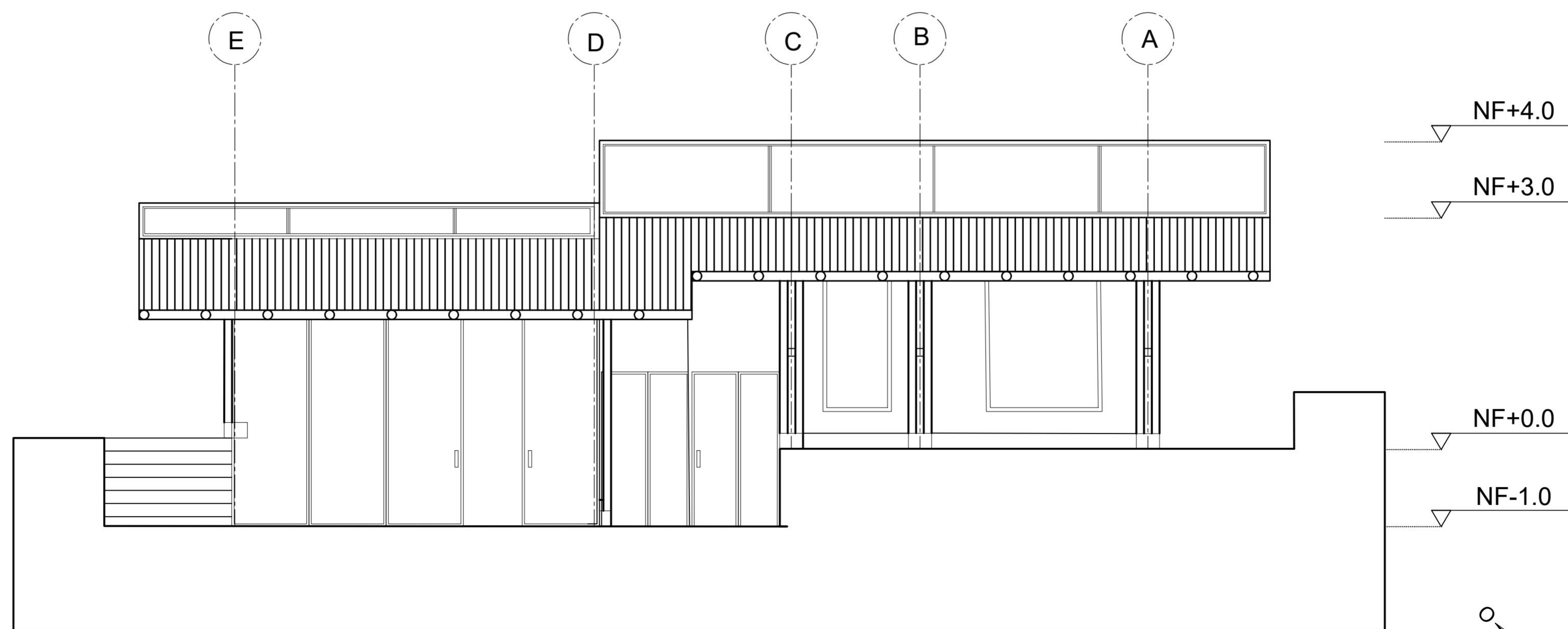
F FACHADA POSTERIOR ESC:1:50
