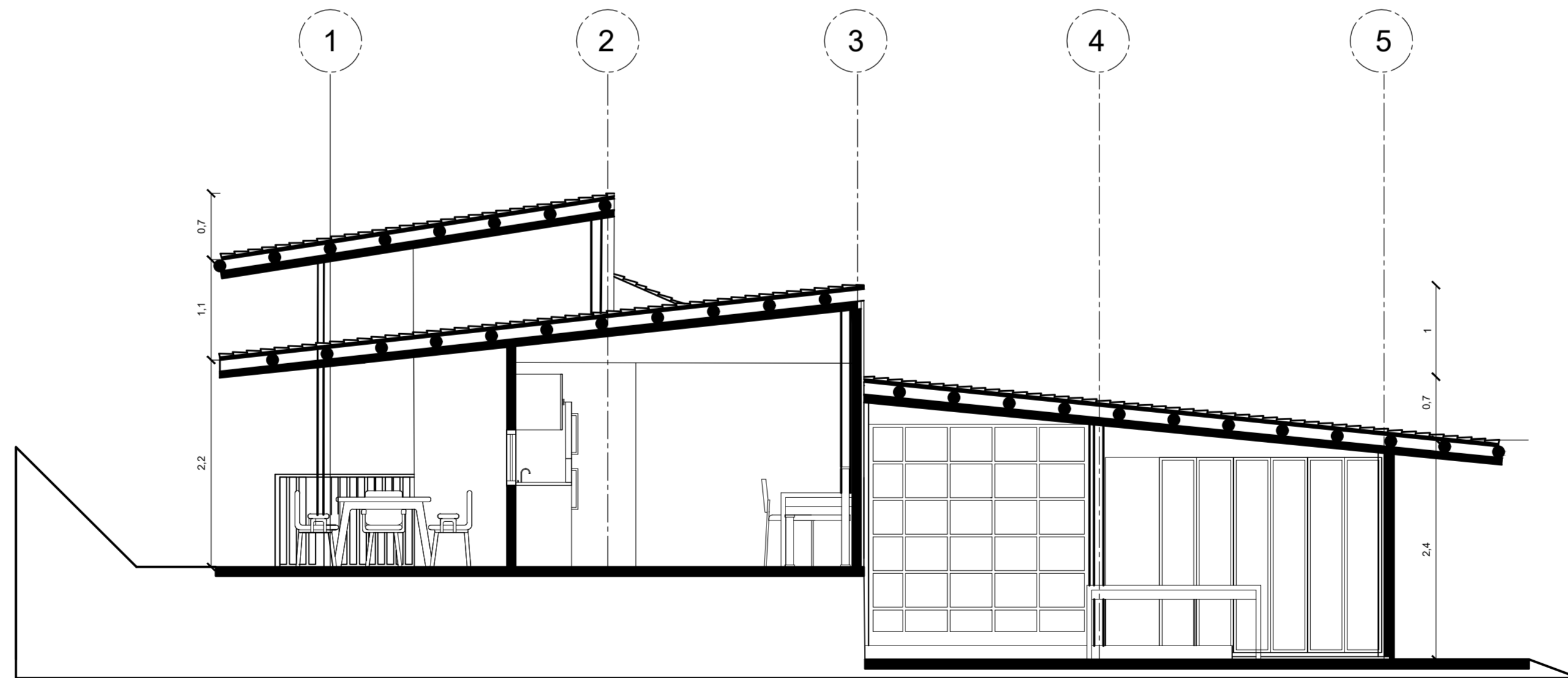
C CORTE A-A' ESC:1:50
