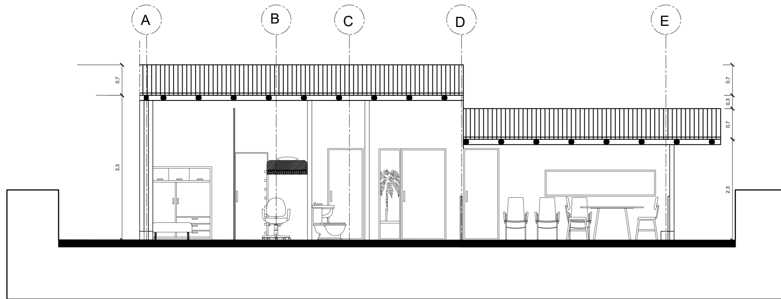
C CORTE B-B ESC:1:50
