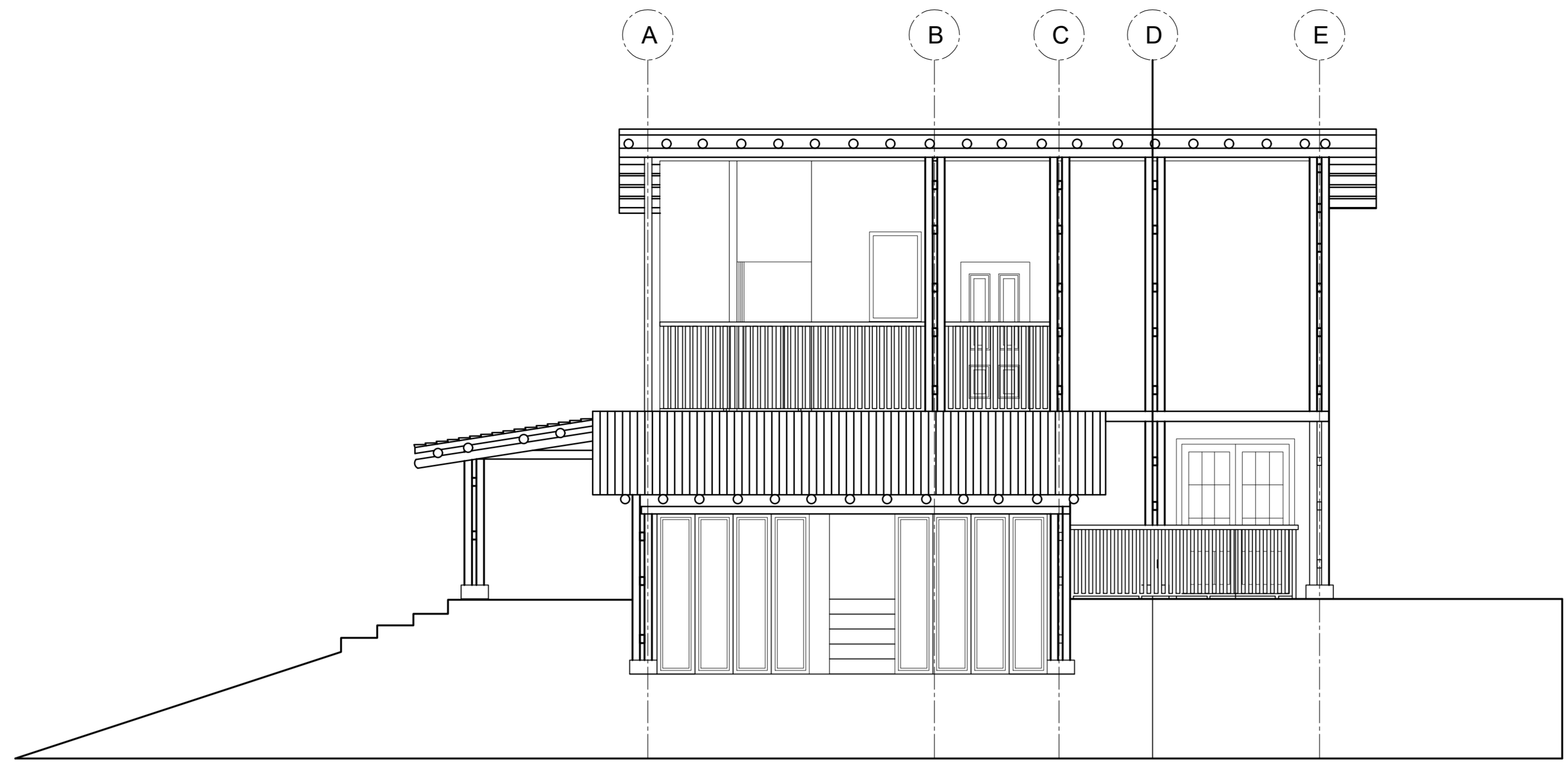
F FACHADA LATERAL DERECHA ESC:1:50
