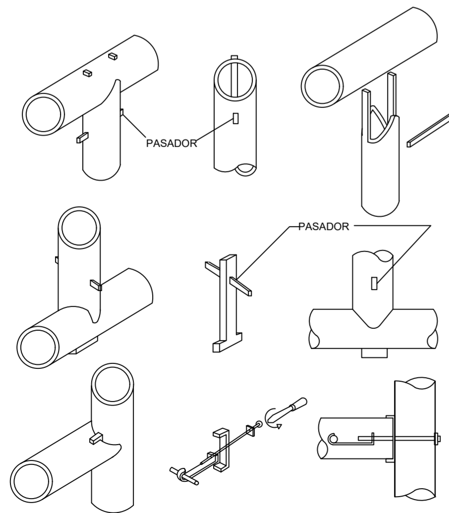
DT DETALLE UNIONES EN GUADUA ESC:1:10
