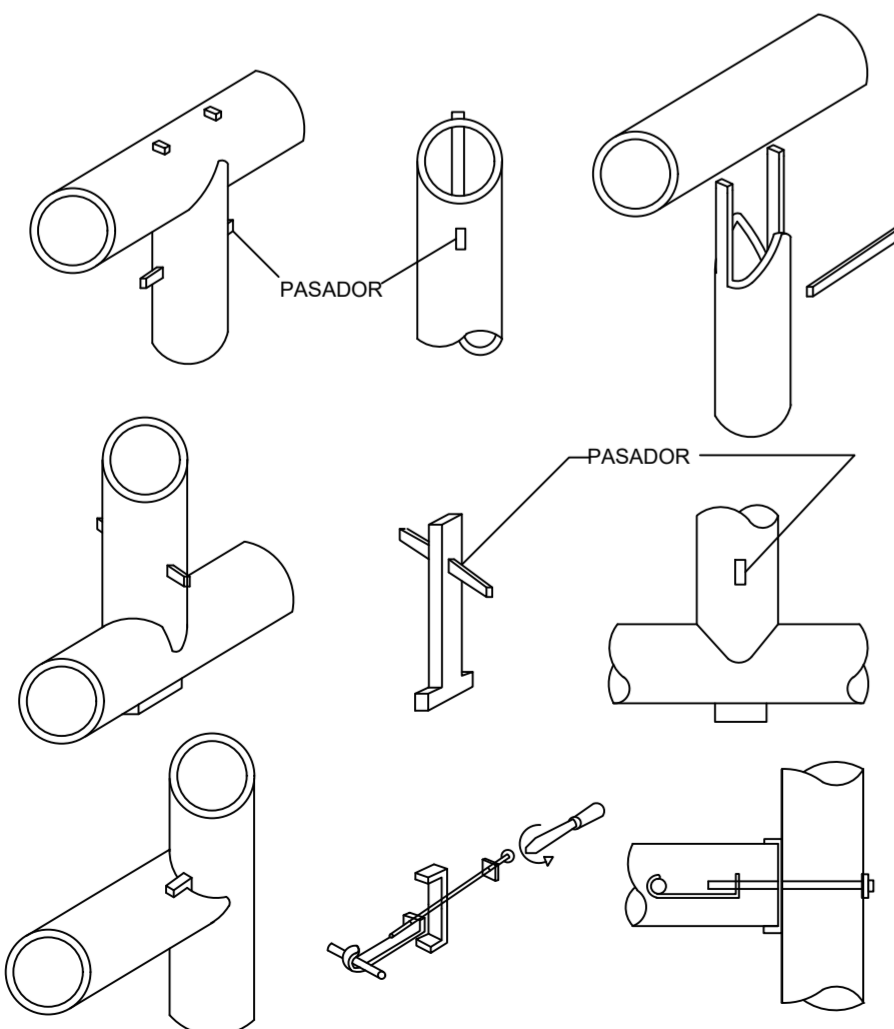
DT DETALLE UNIONES EN GUADUA ESC:1:10
