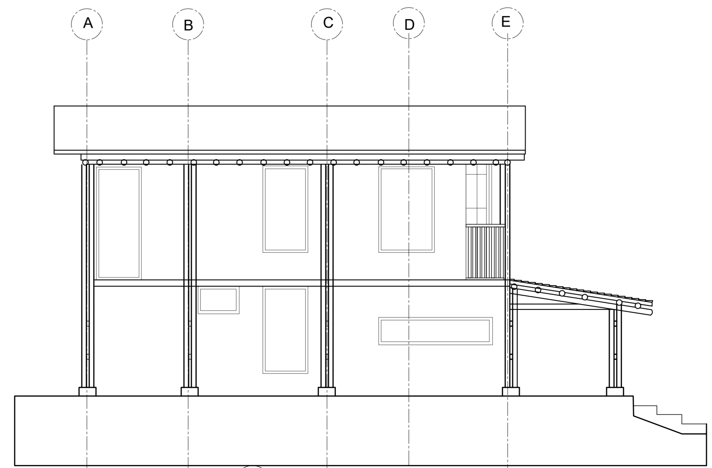
F FACHADA LATERAL IZQUIERDA ESC:1:50
