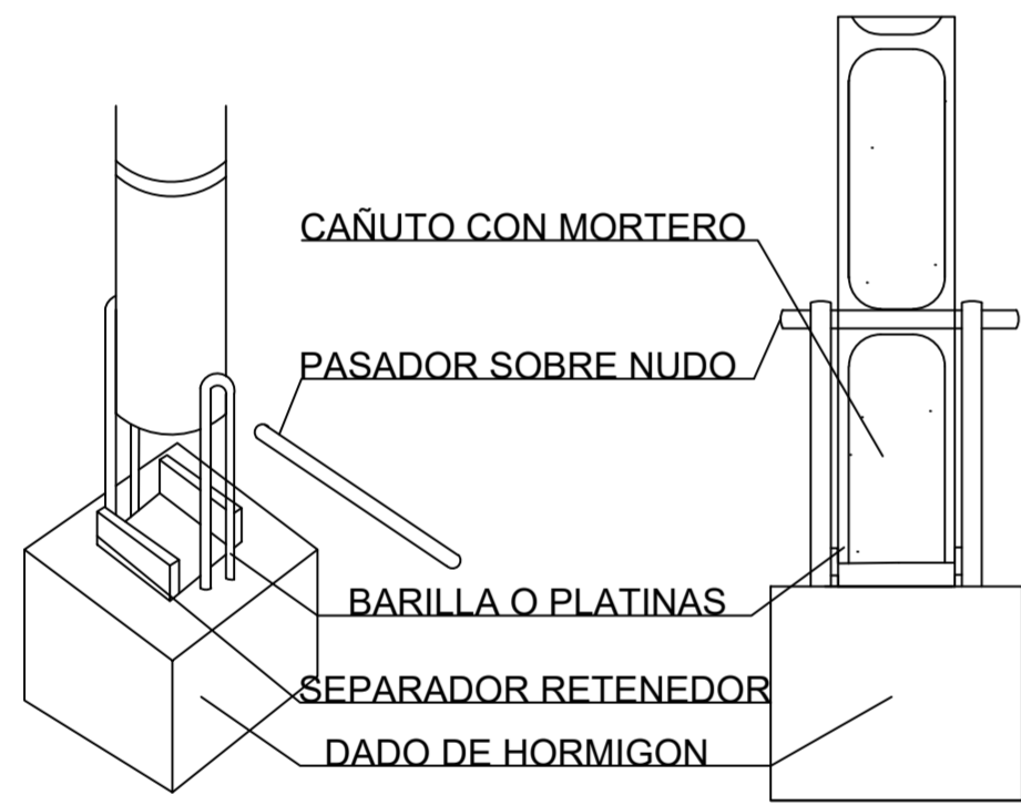
DT DETALLE BASE COLUMNA ESC:1:10
