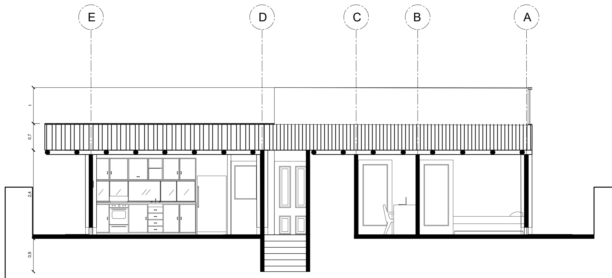
C CORTE B. B' ESC:1:50
