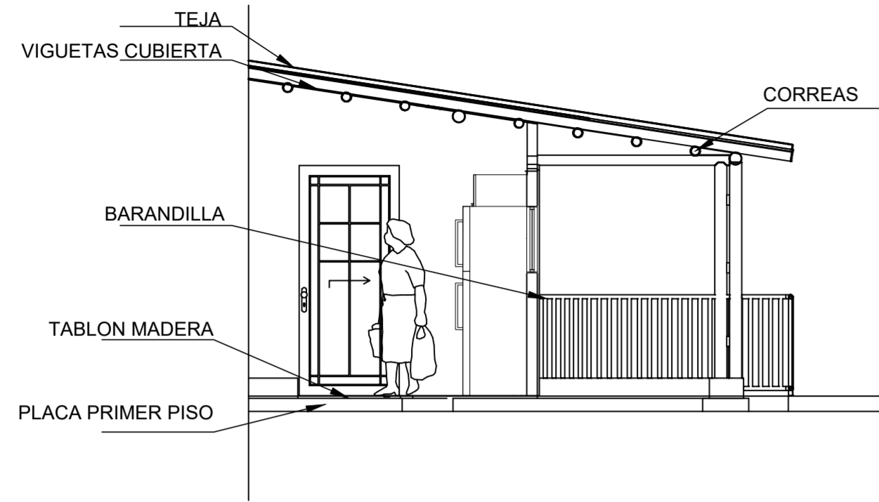
DT CORTE FACHADA ESC:1:50
