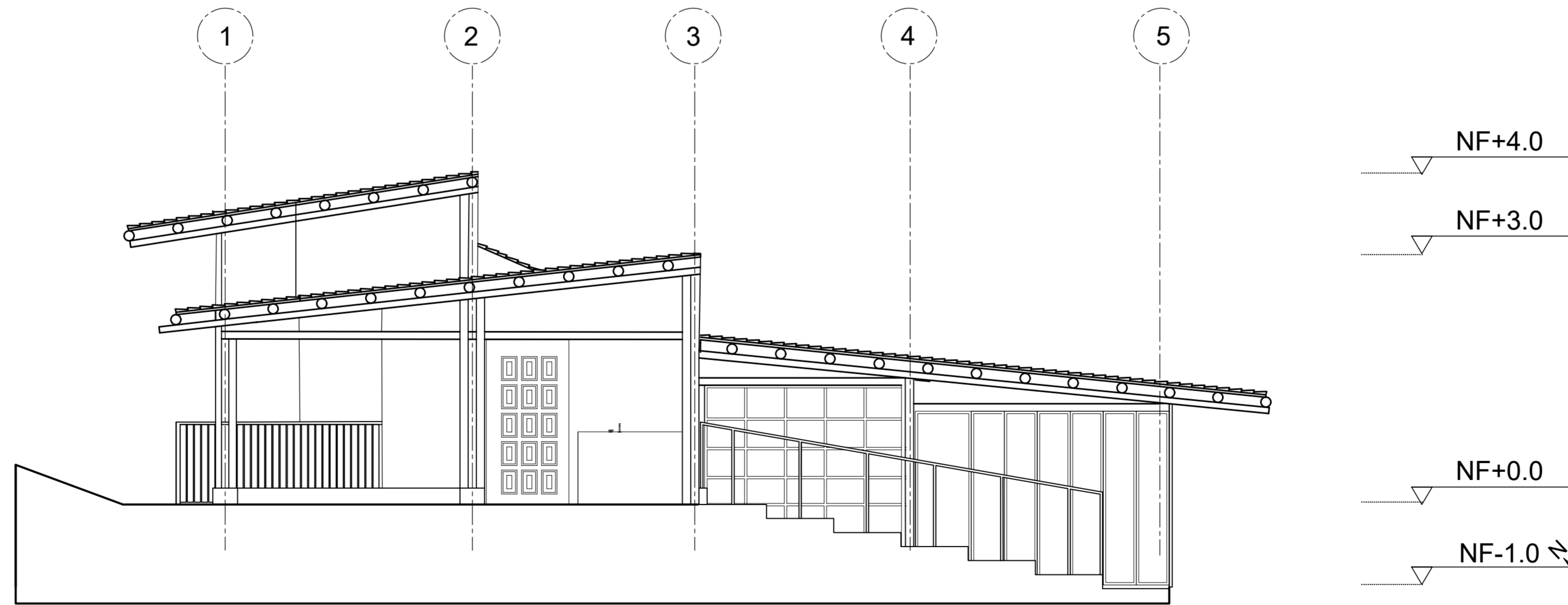
A FACHADA LATERAL IZQUIERDA ESC:1:50
