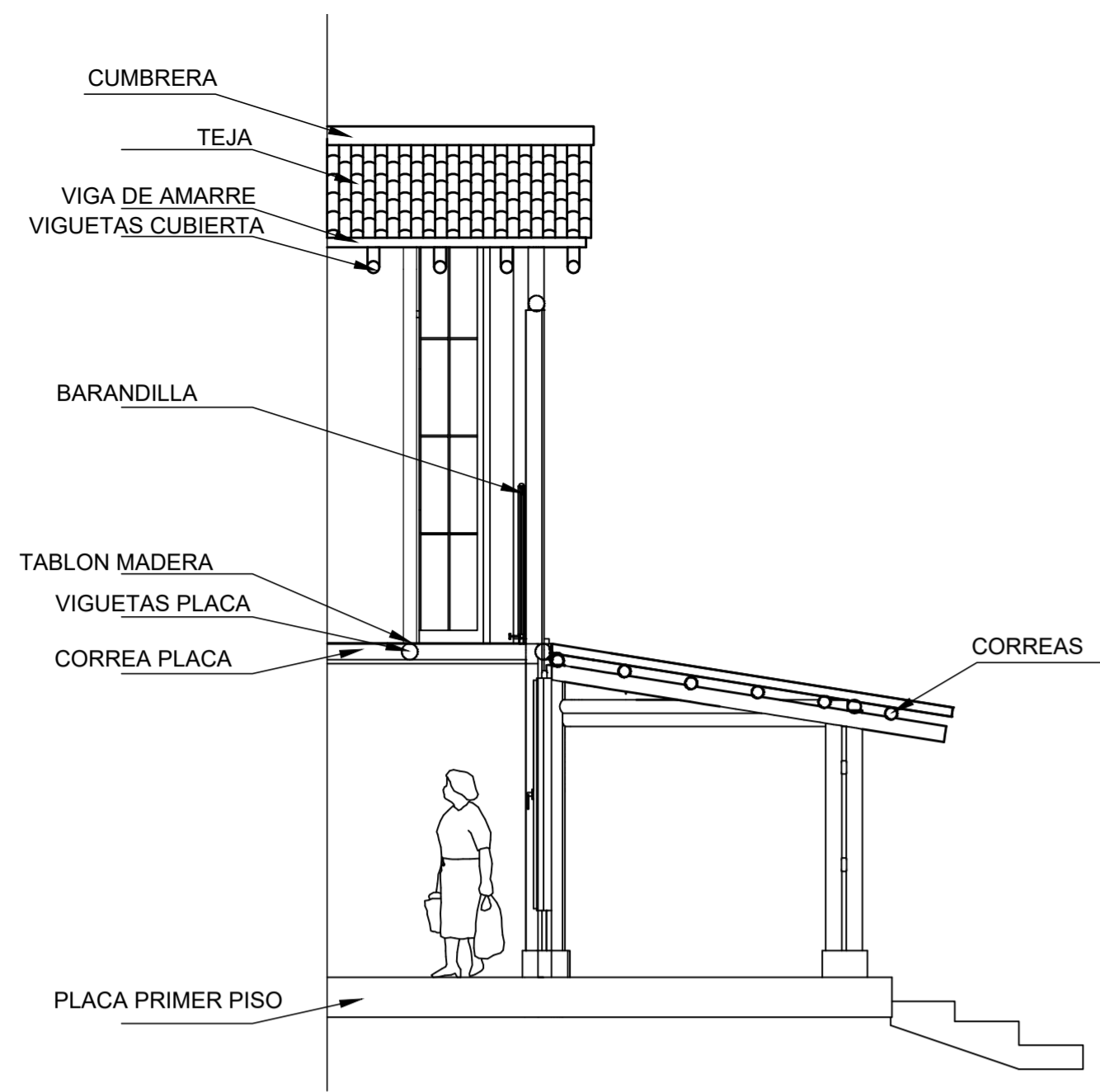
DT CORTE FACHADA ESC:1:50
