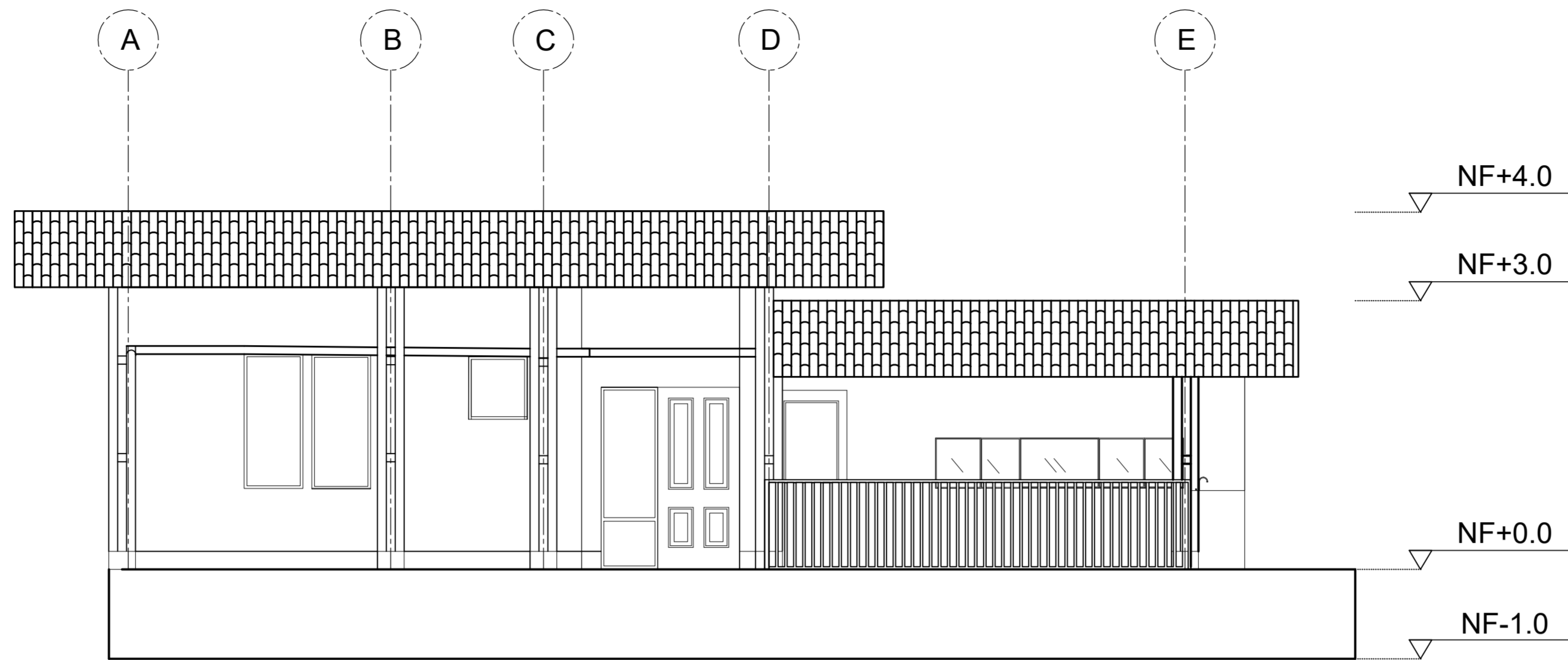
F FACHADA PRINCIPAL ESC:1:50
