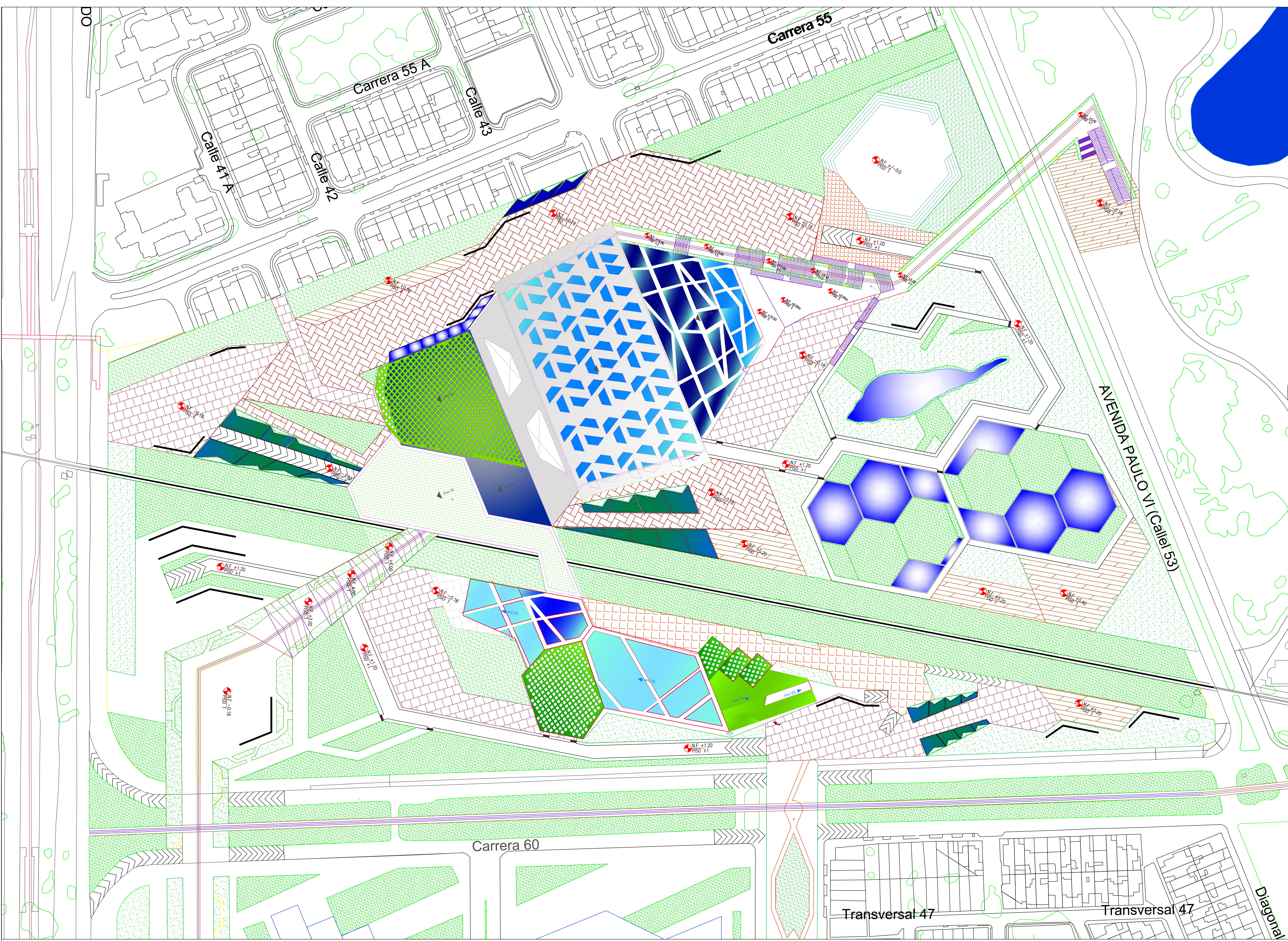
U4 PLANO IMPLANTACIÓN - CUBIERTAS ESCALA 1 : 1000
