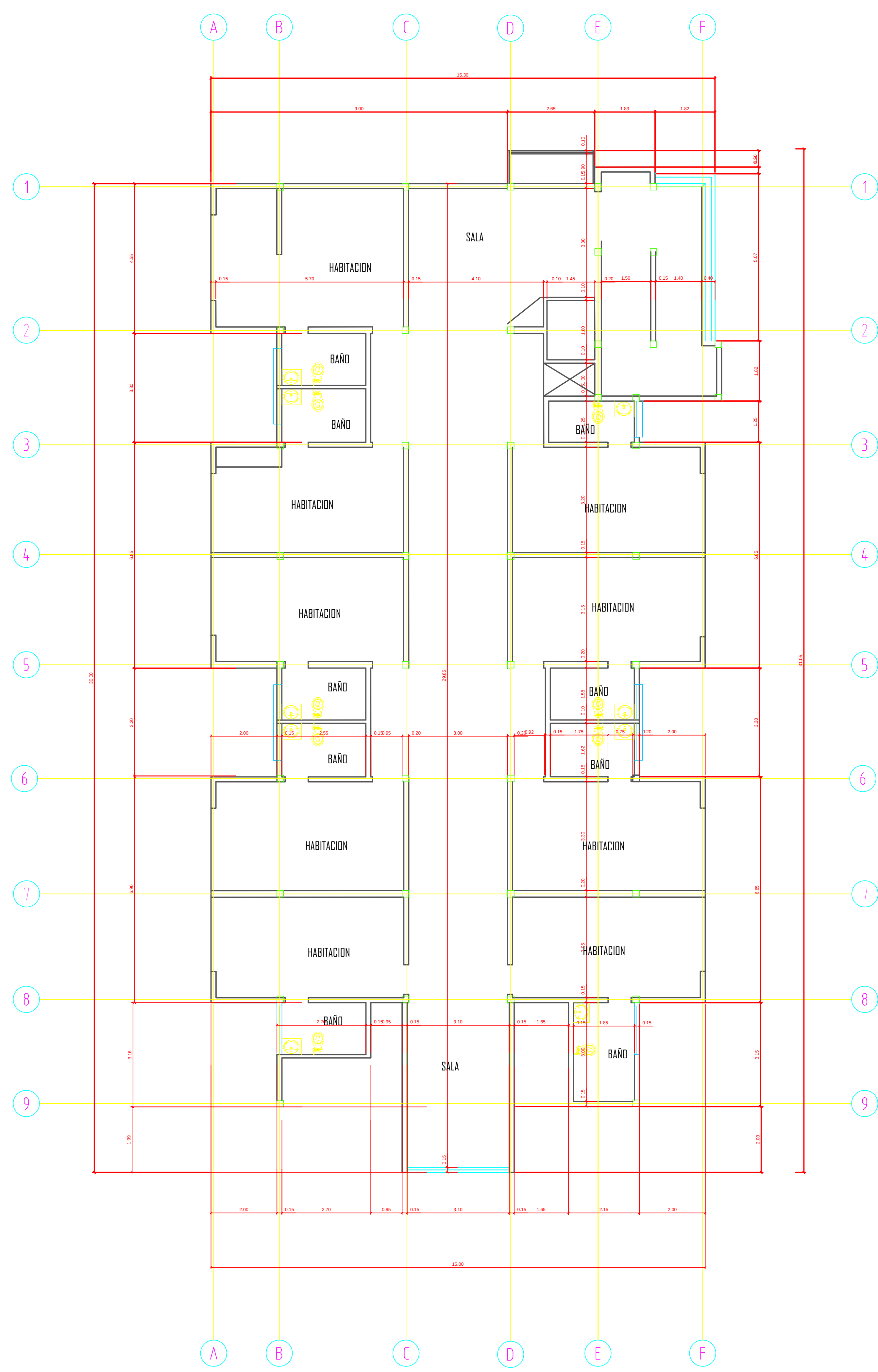
PLANTA TERCER PISO
