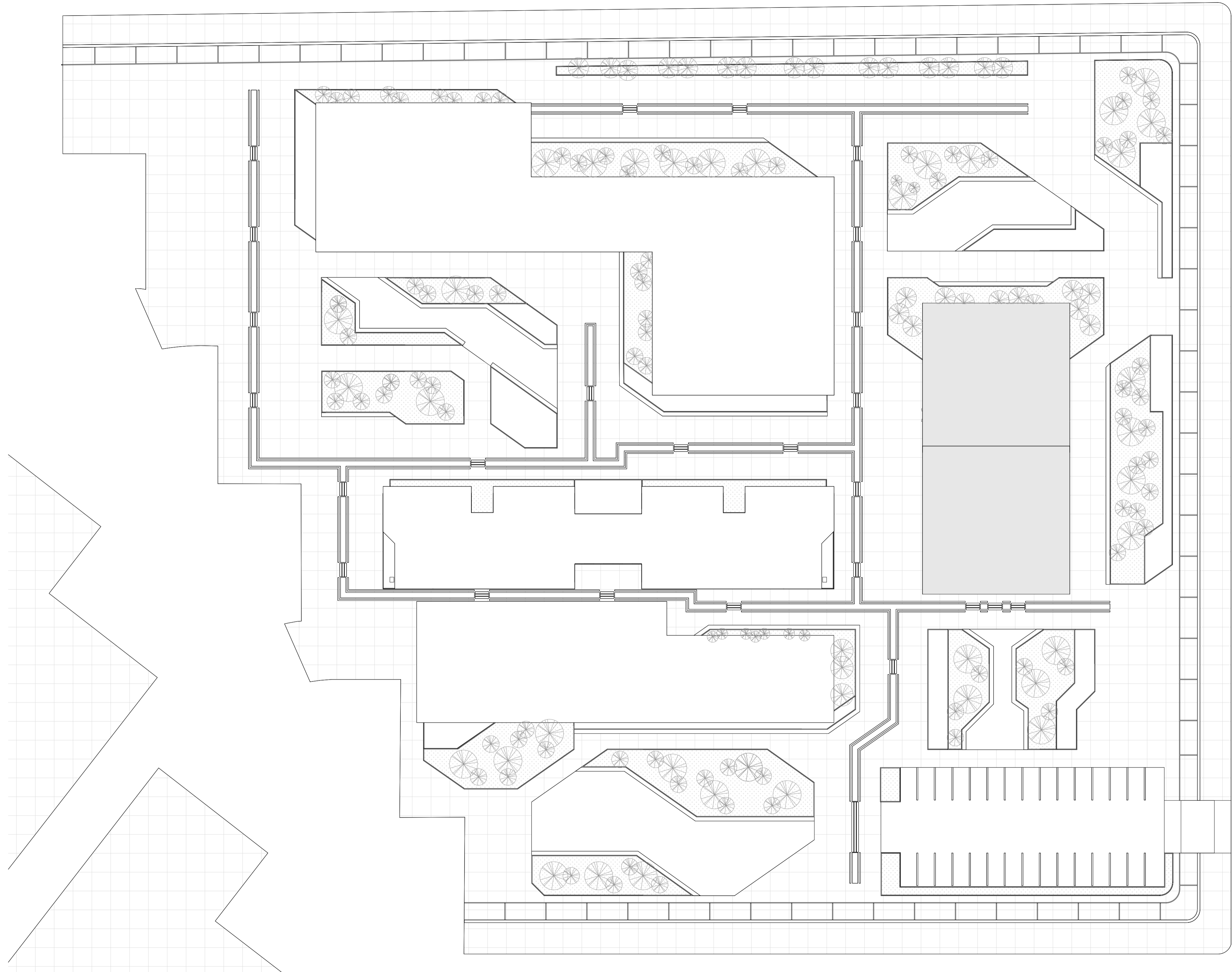
1 Cubierta A105 1:350
