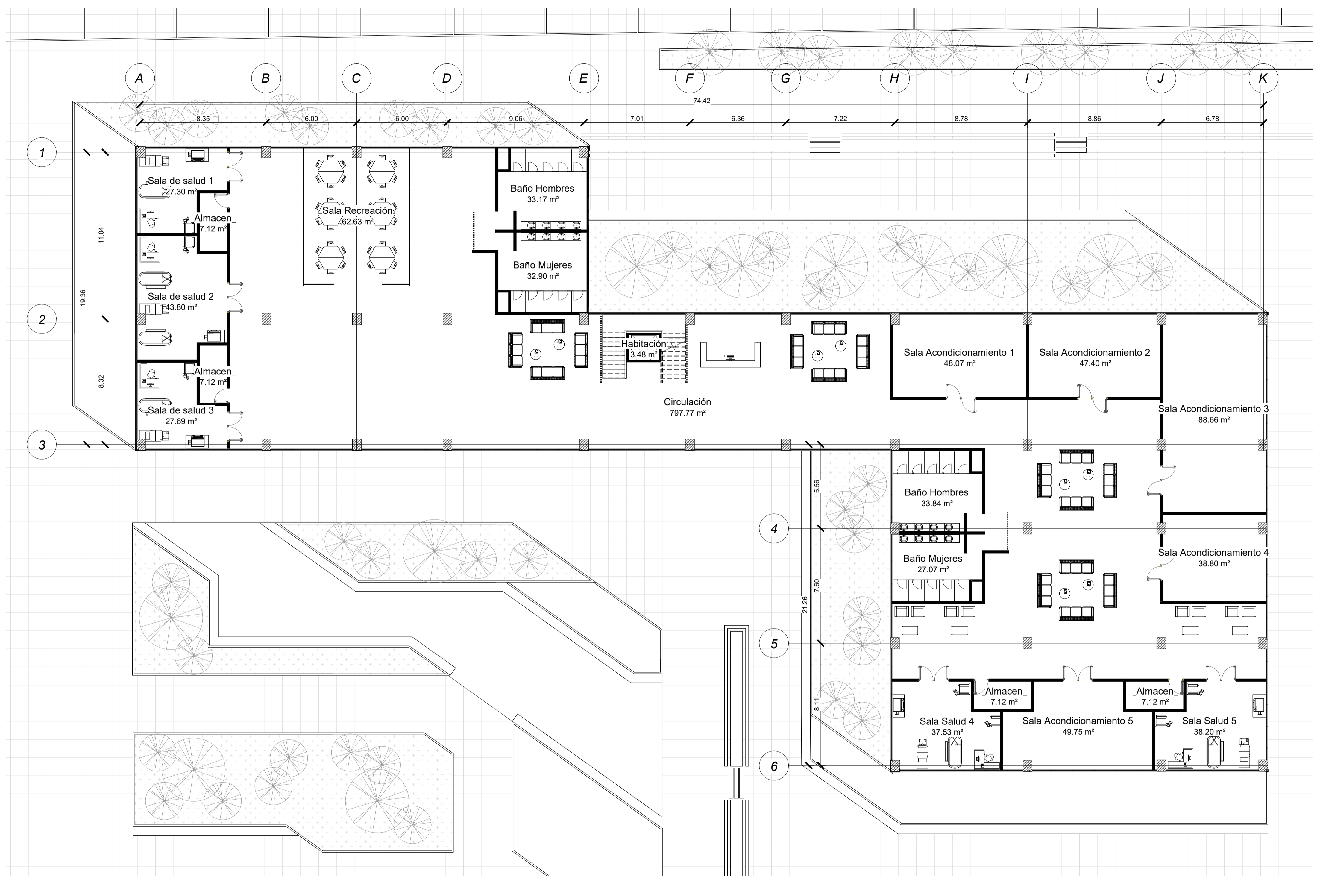
1 Nivel 1 - Salud A102 | 1 : 150
