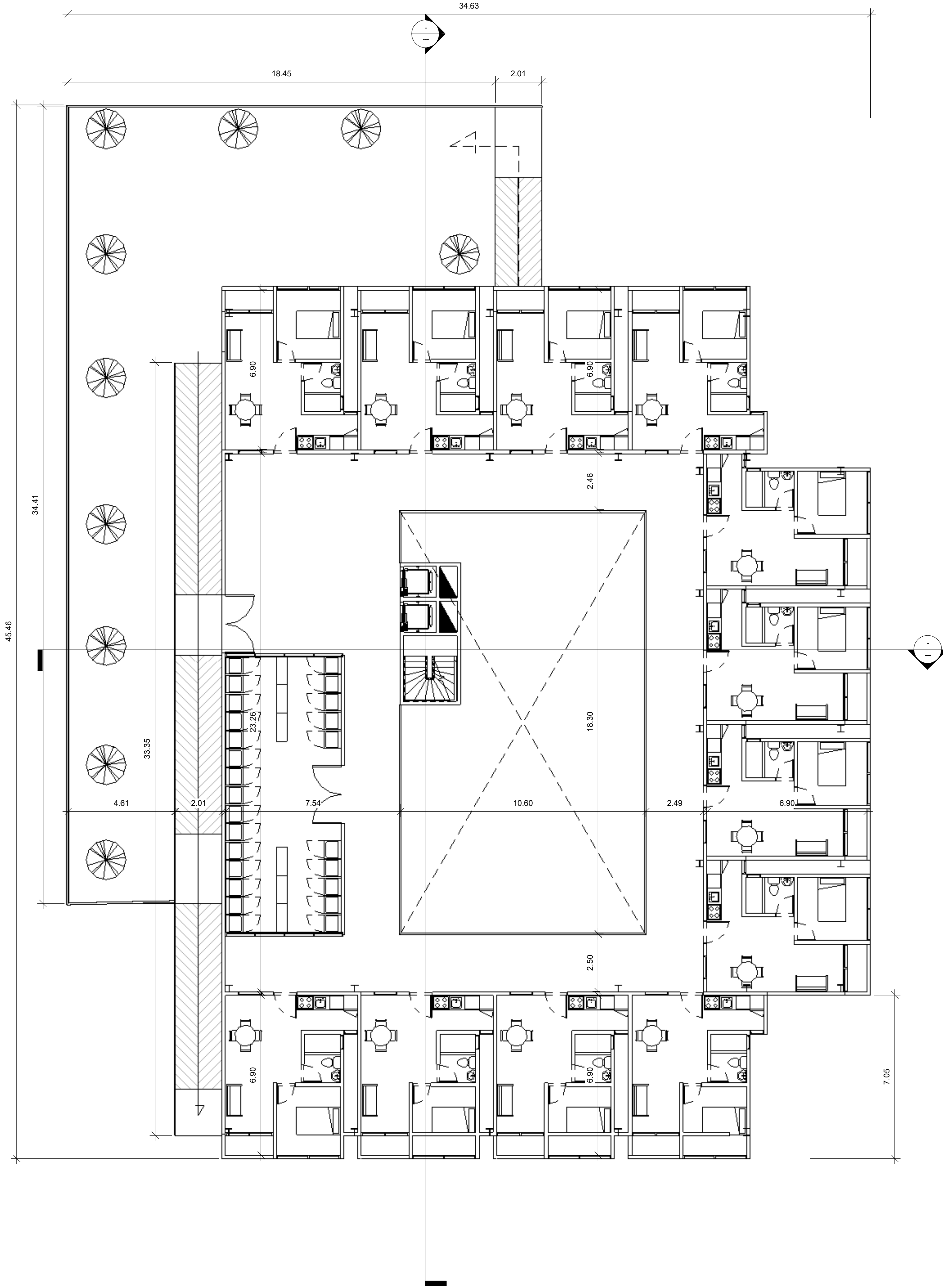
3 Nivel 10 1 : 100
