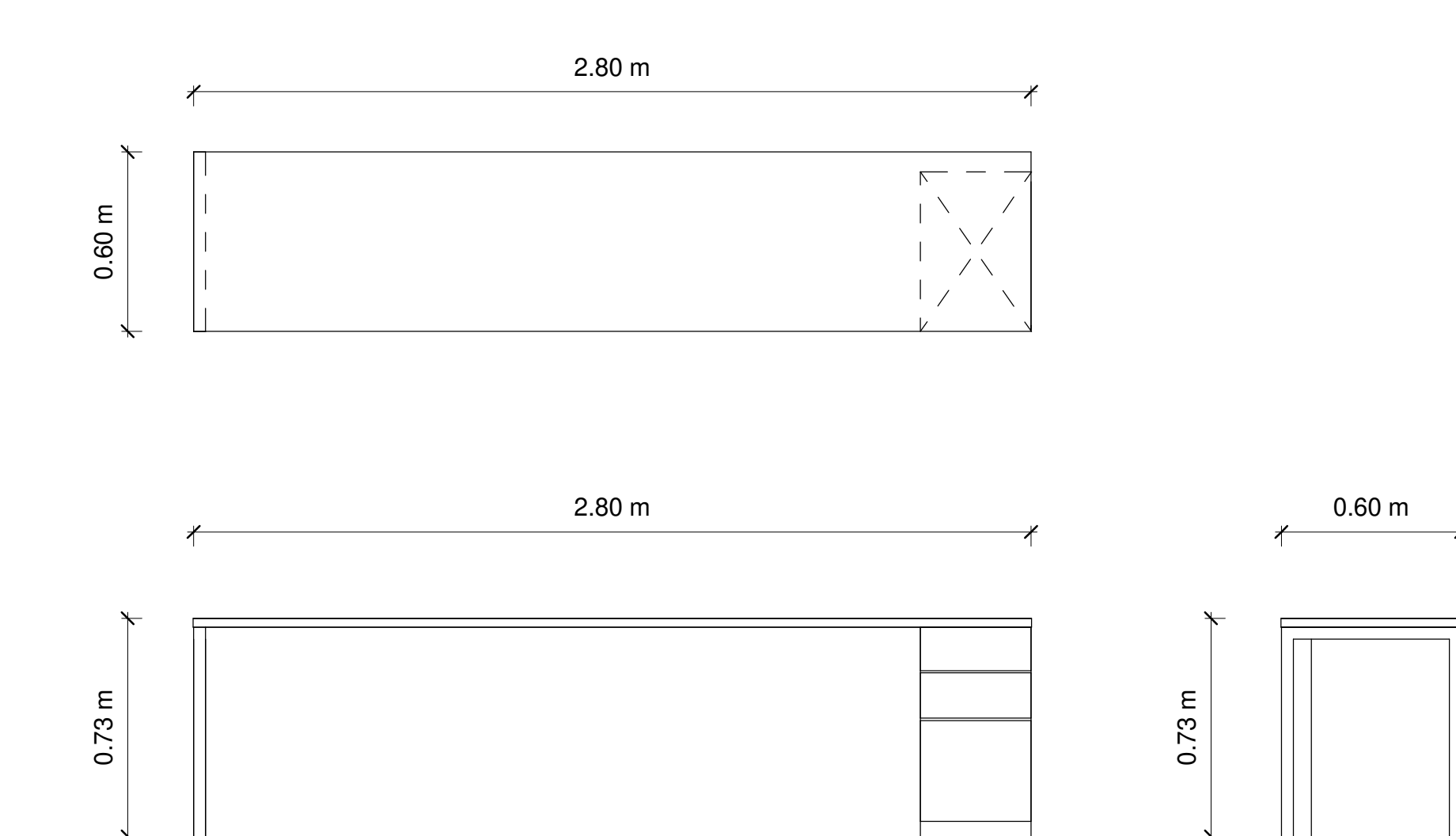
M-5 1 : 20
