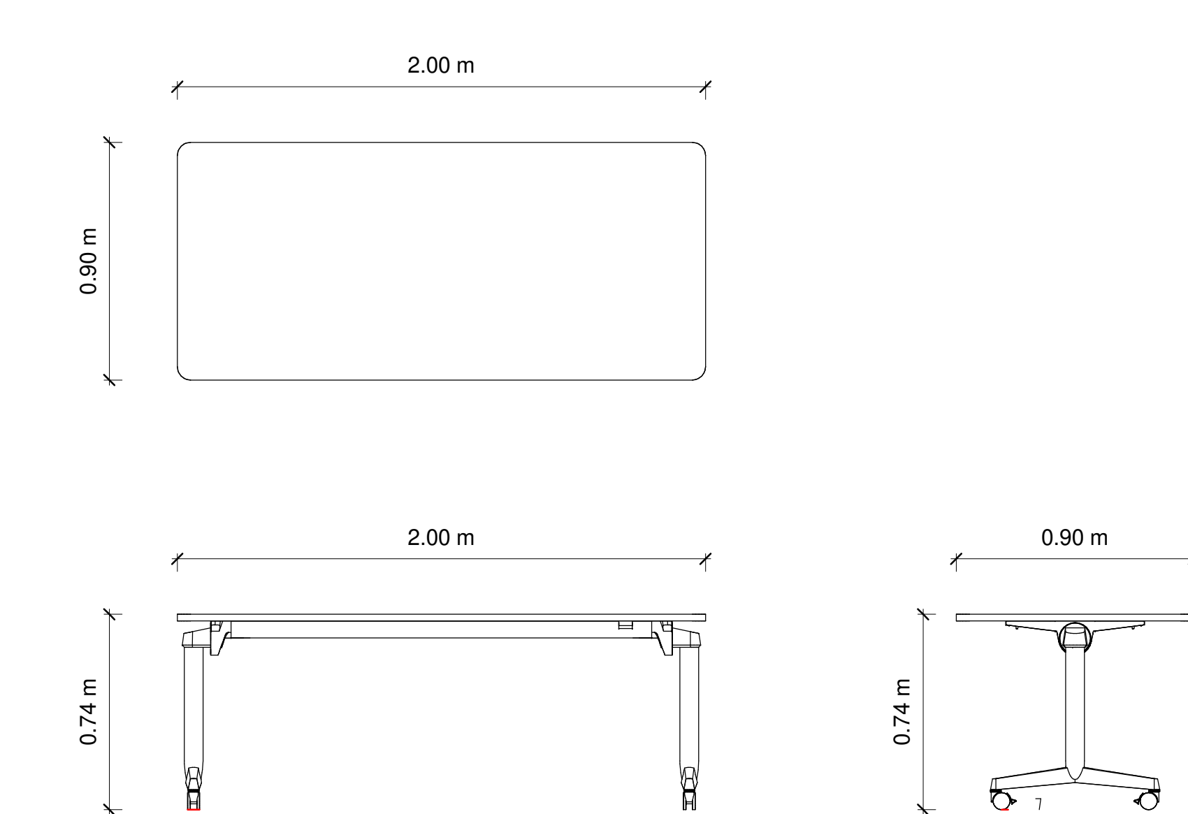
M-1 1 : 20
