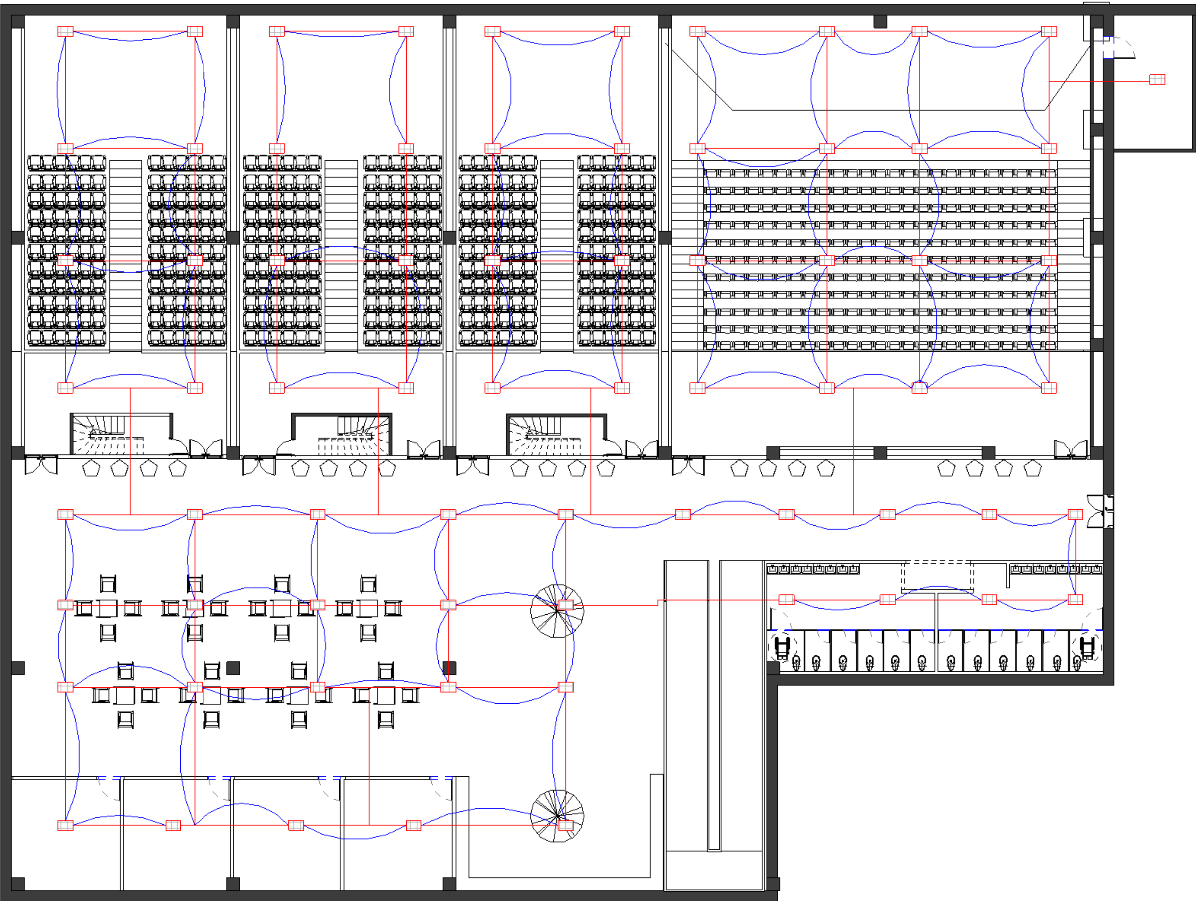
1 Nivel -2 ILUMINACION 1 : 100
