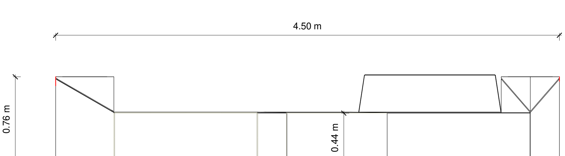
M-15 1 : 20
