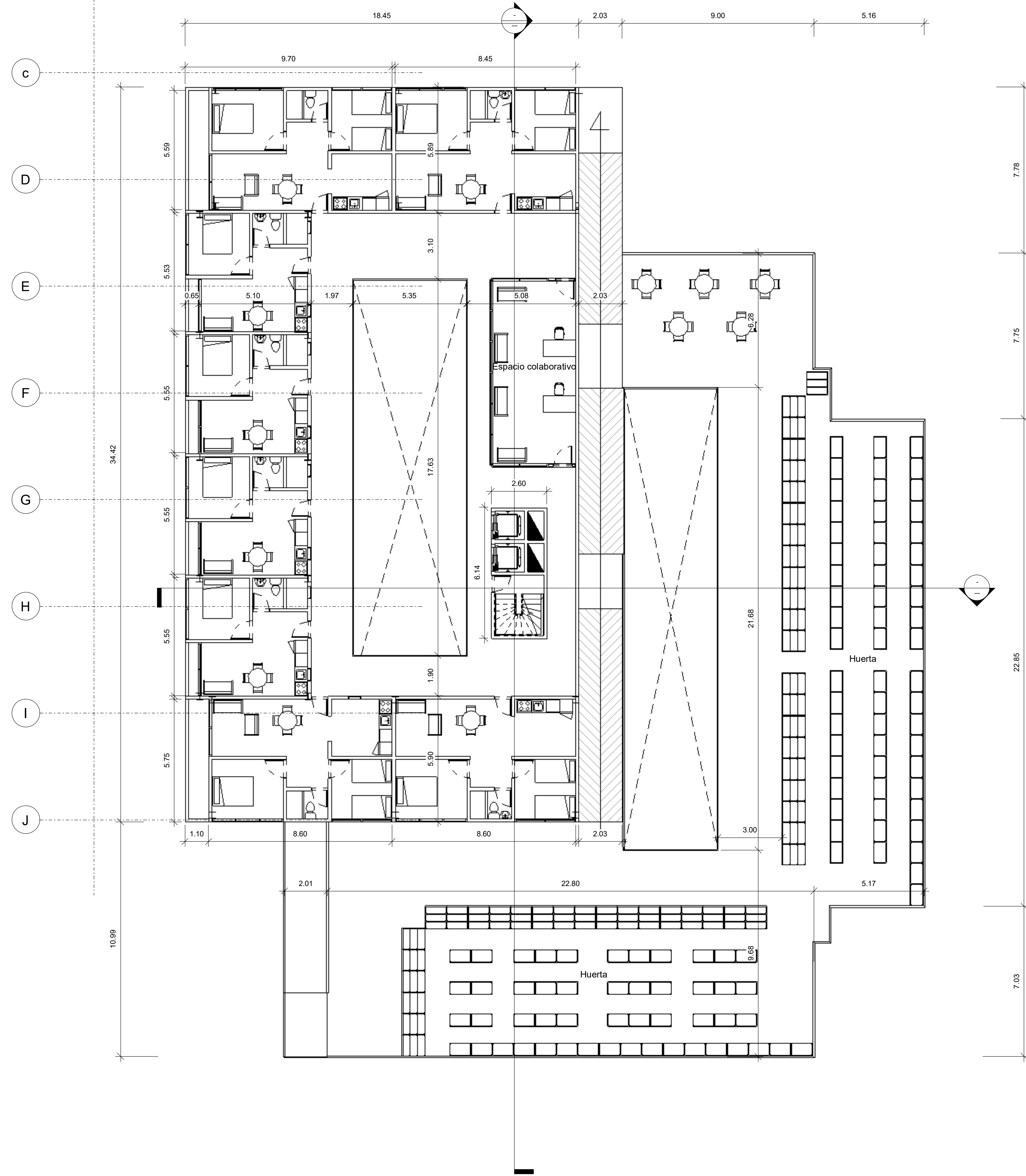
2 Nivel 7 1 : 100
