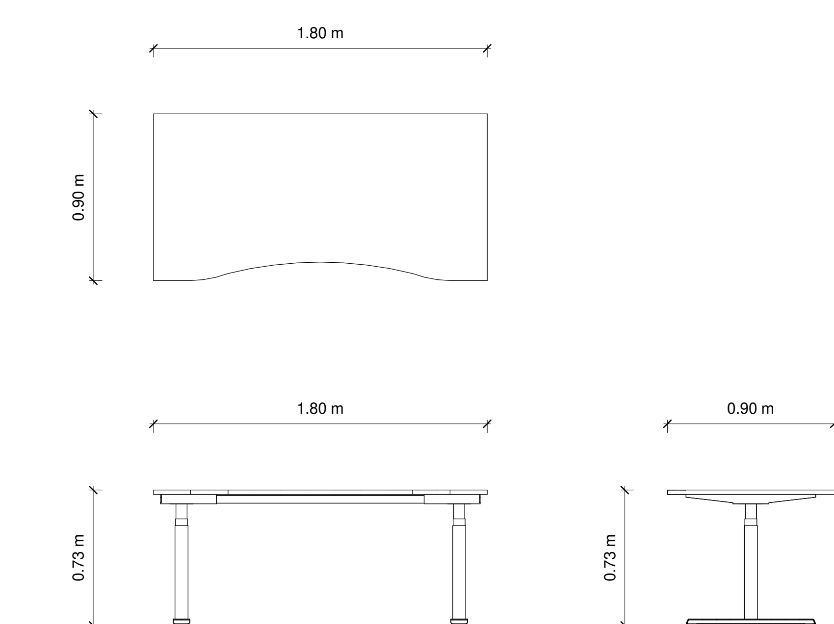
M-9 1 : 20
