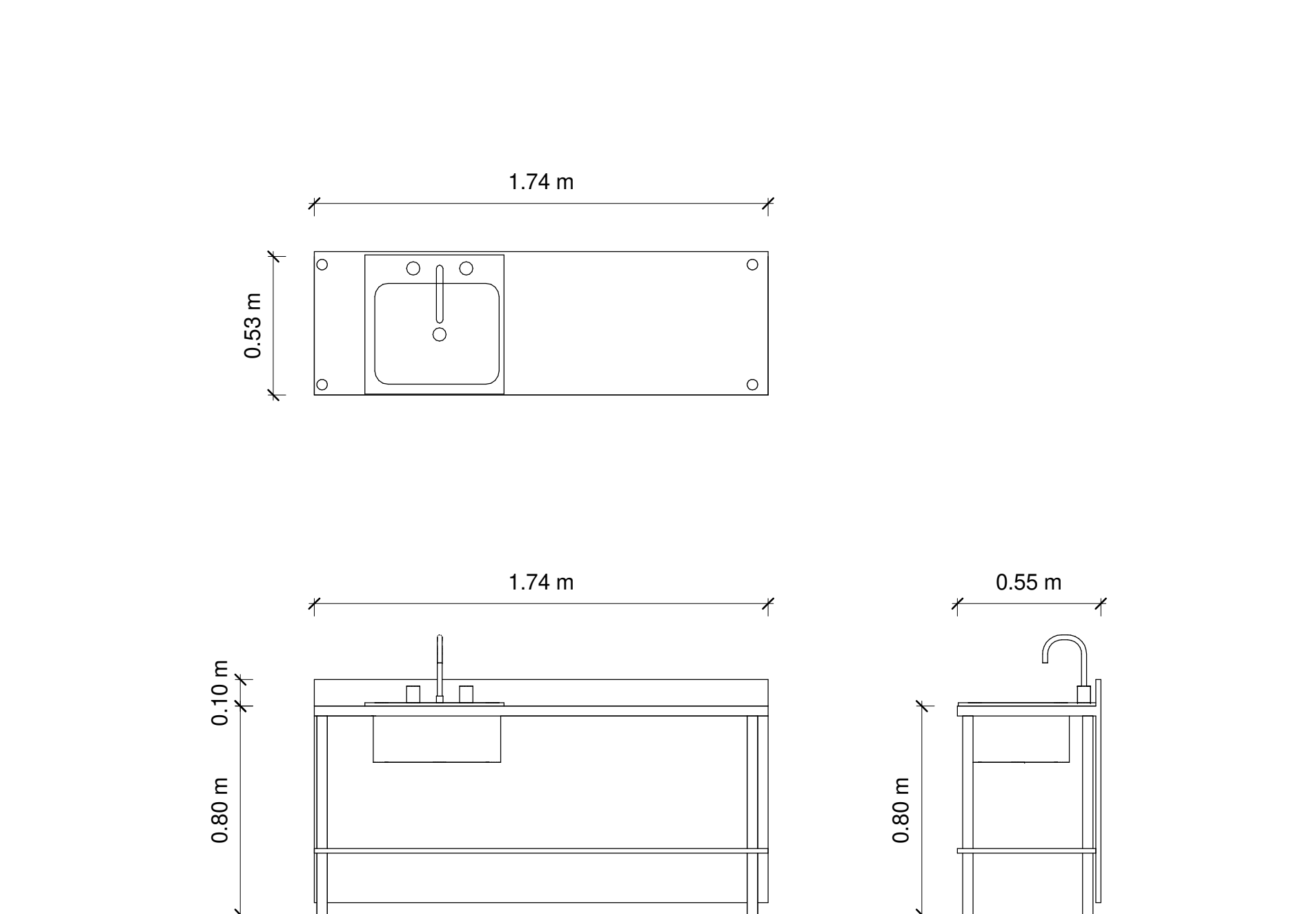
M-10 1 : 20
