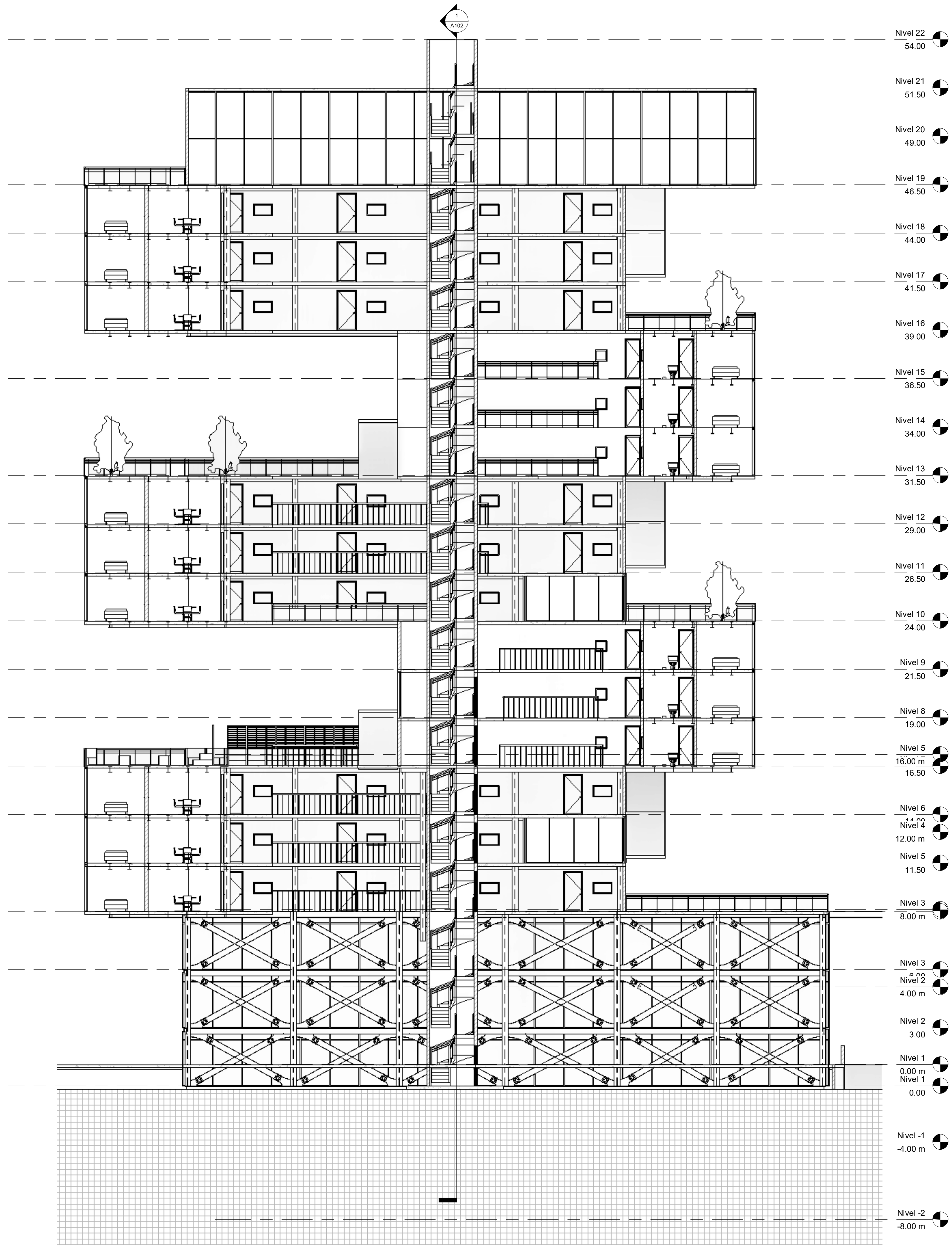
2 Sección 2 1 : 100
