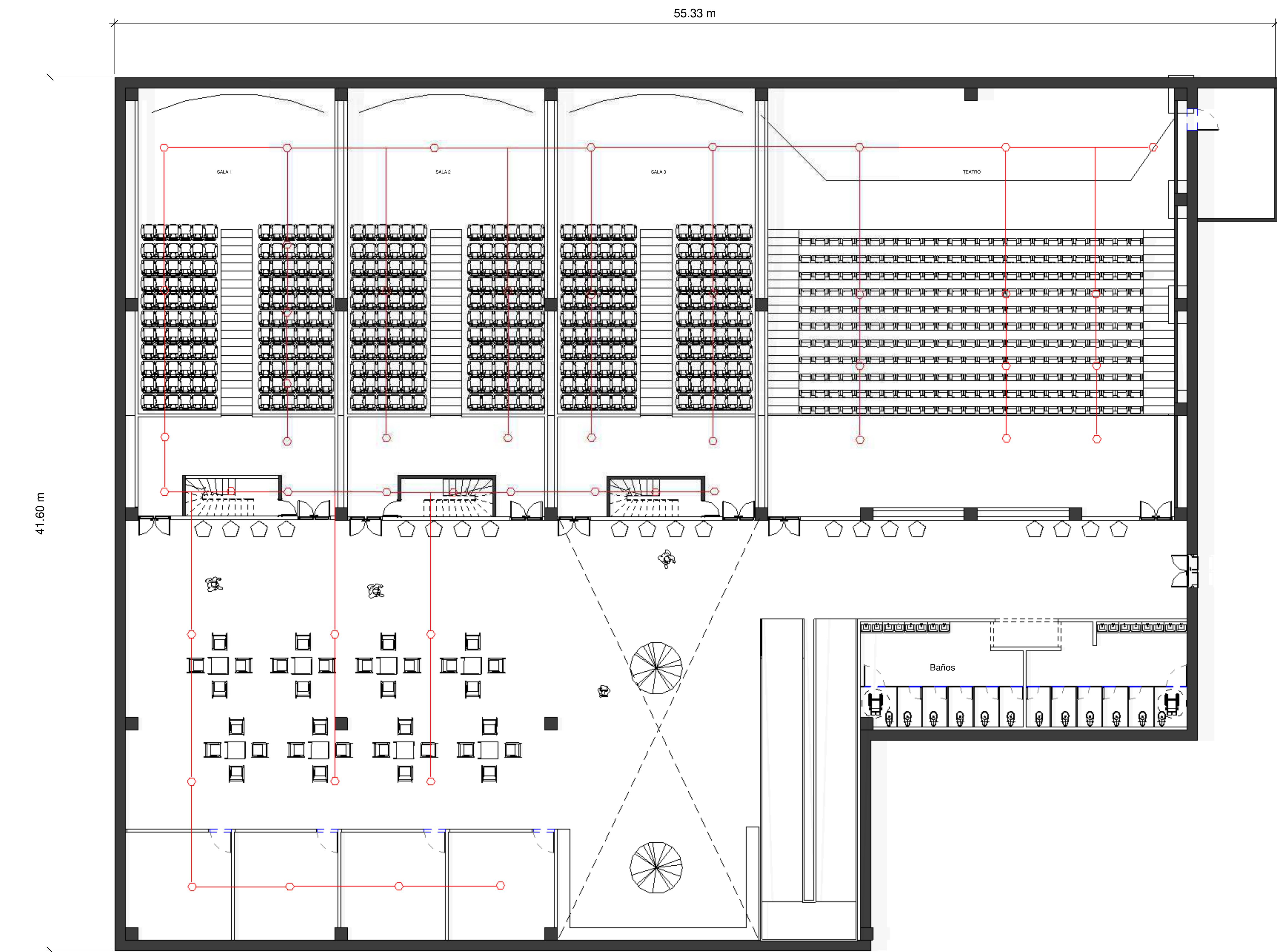
1 Nivel -2 CONTRA INCENDIOS 1 : 100
