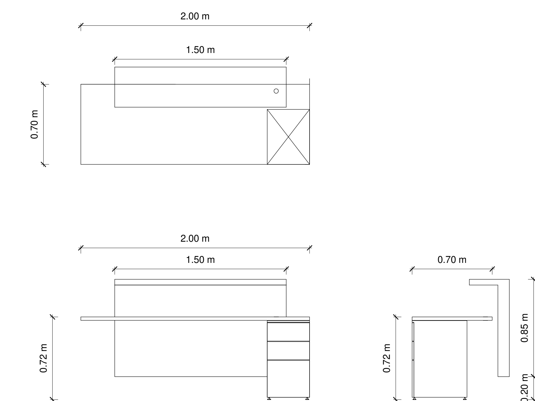
M-8 1 : 20
