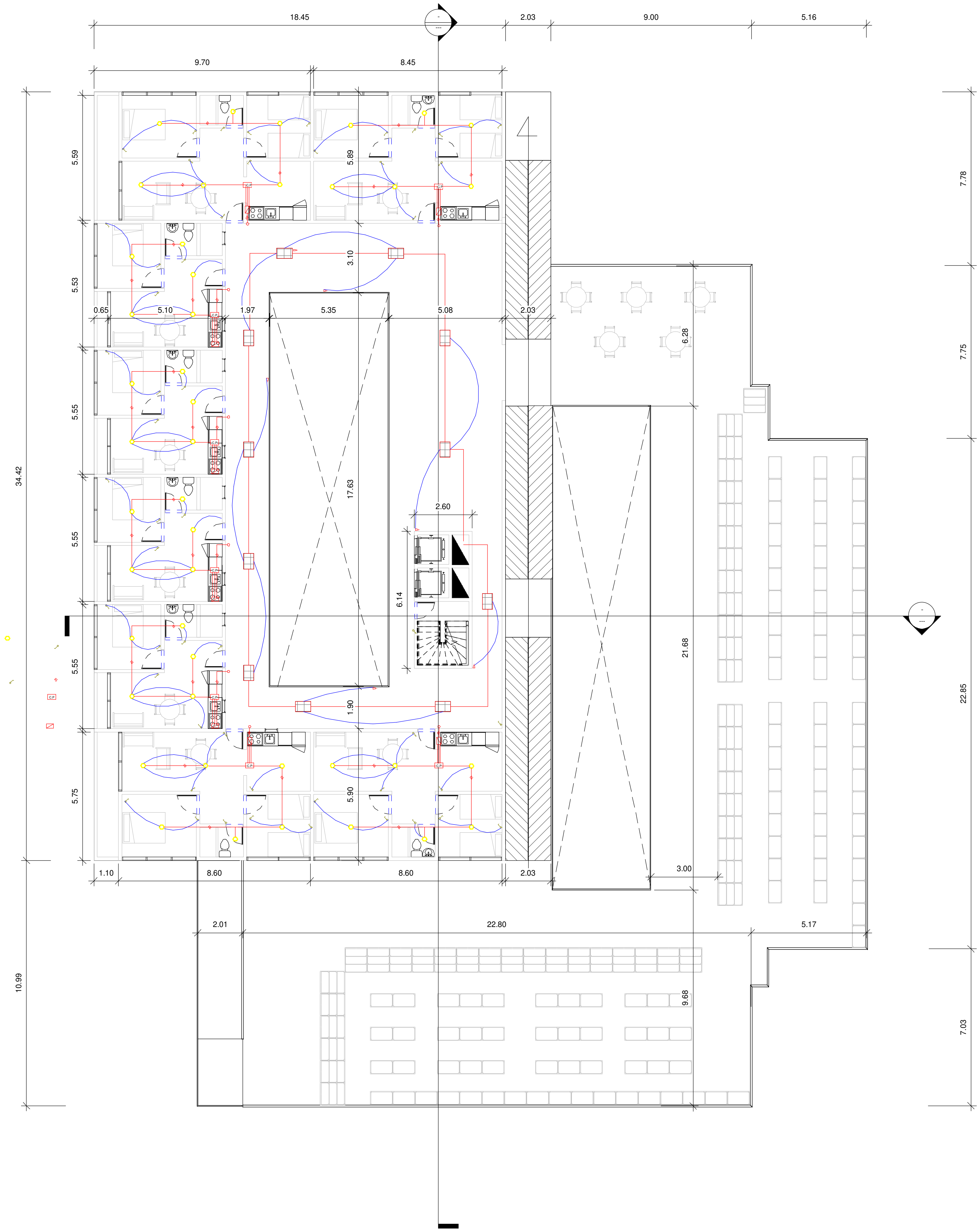
2 Nivel 7 ILUMINACION 1 : 100
