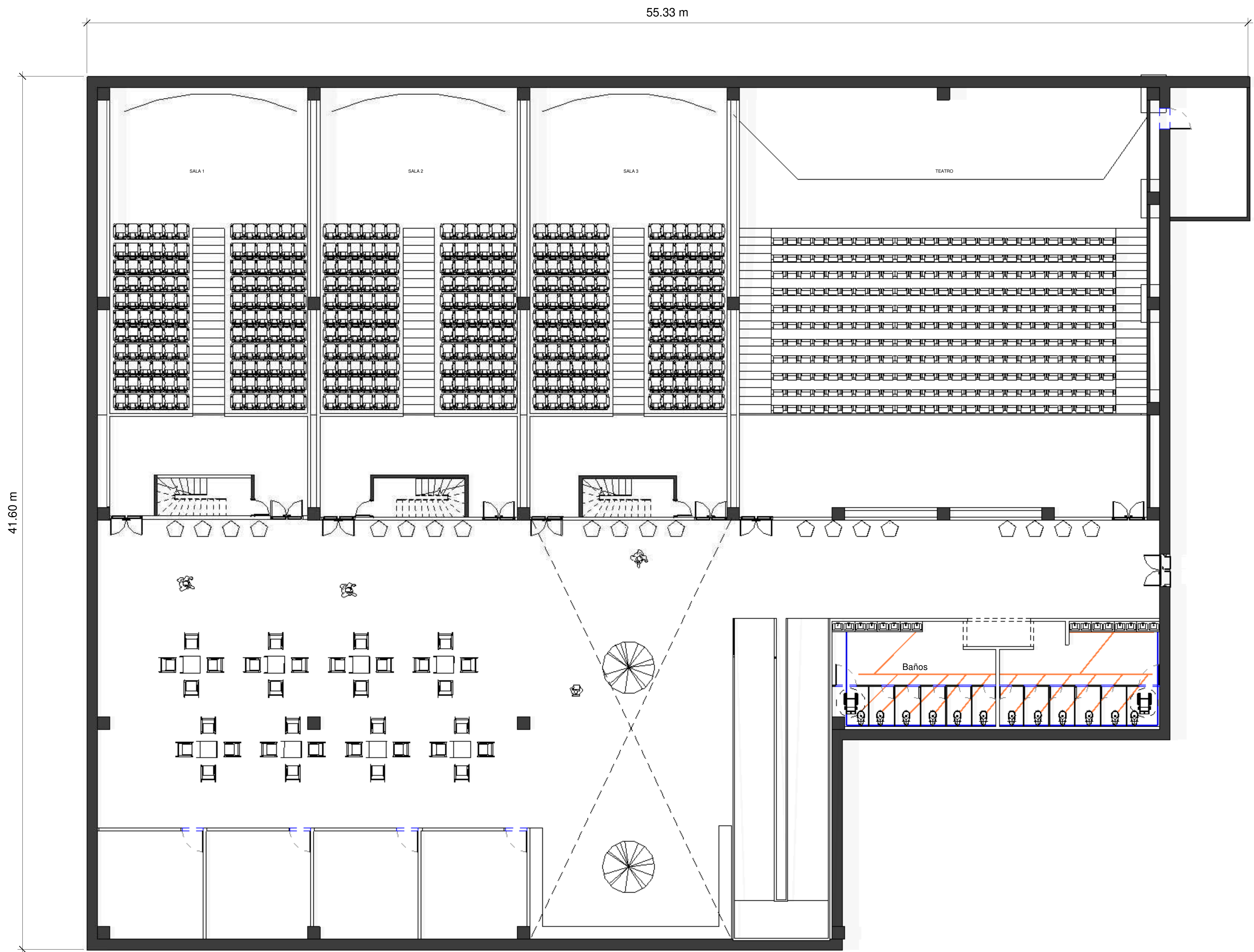
1 Nivel -2 HIDRAULICO 1 : 100
