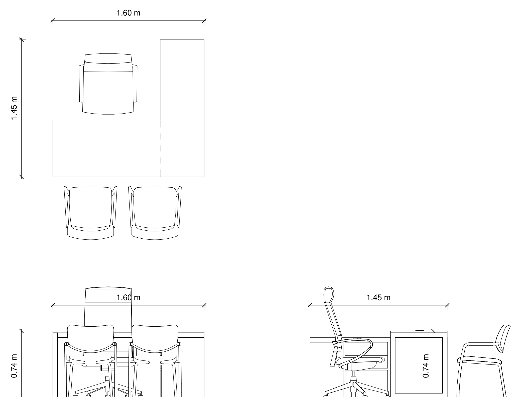
M-4 1 : 20
