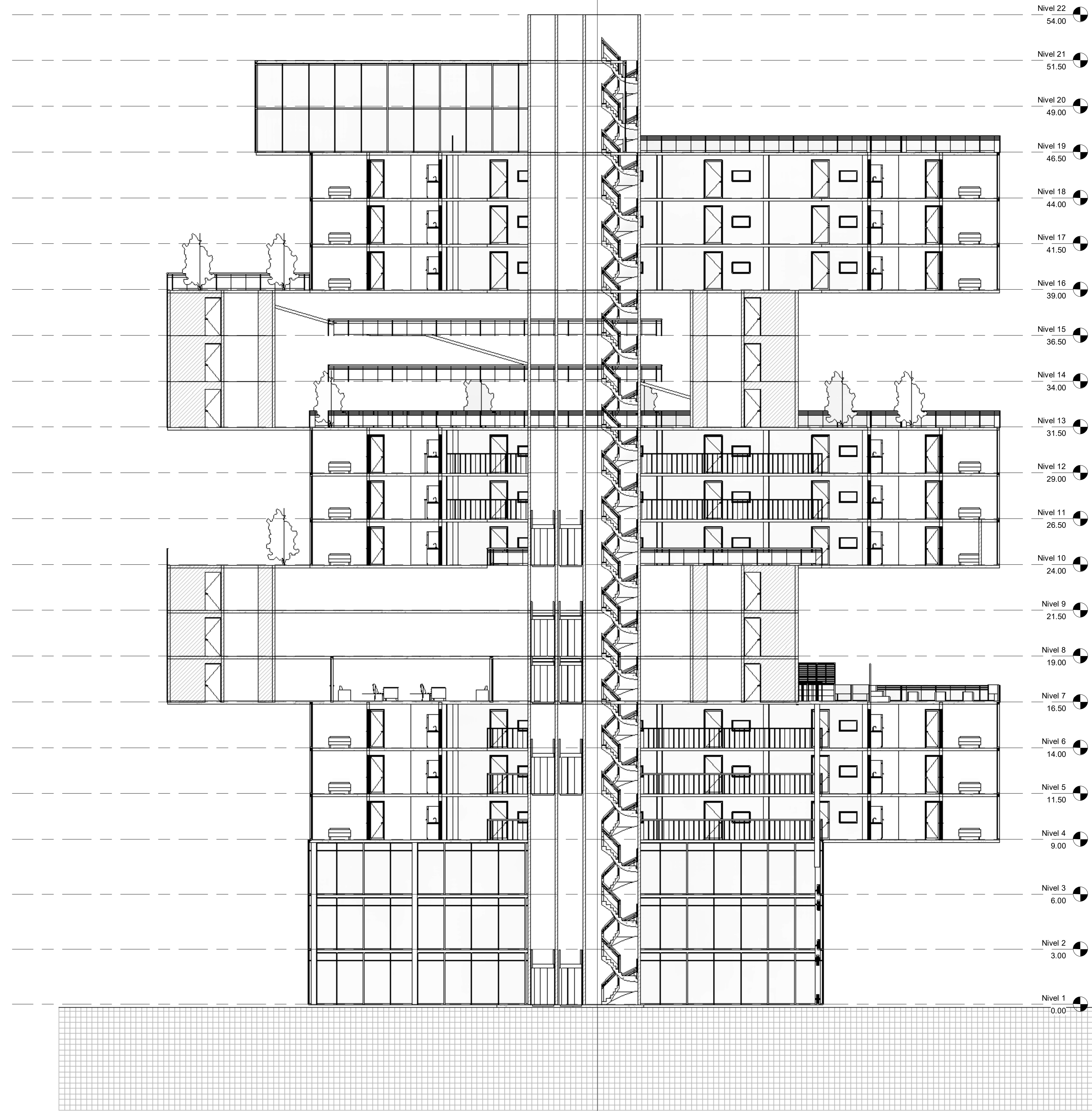
1 Sección 1 1 : 100
