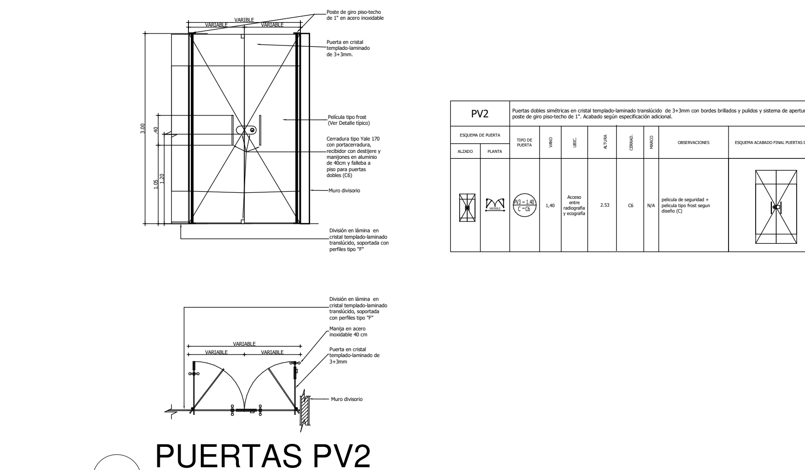
M-18 1 : 20
