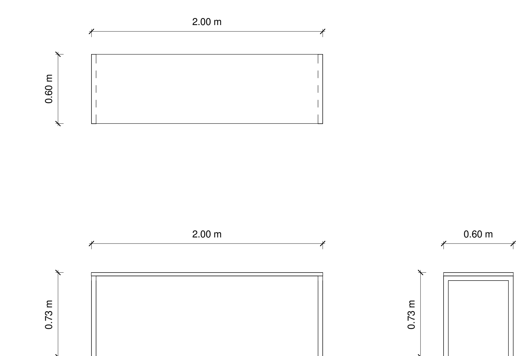
M-7 1 : 20
