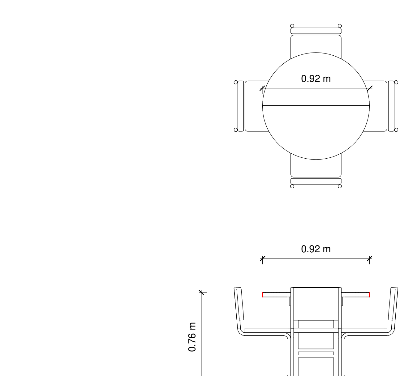
M-6 1 : 20
