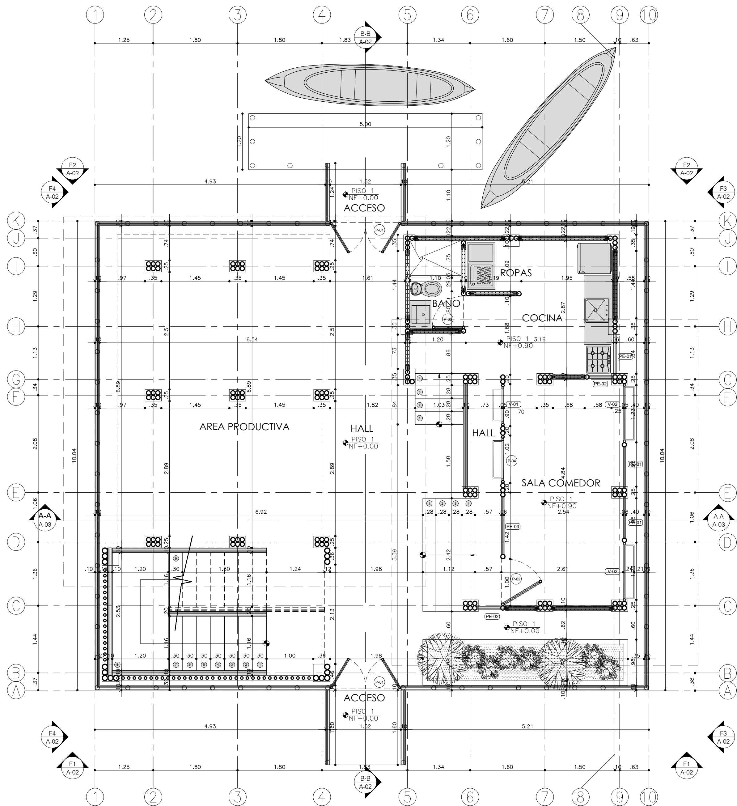
PROPUESTA ARQUITECTONICA PLANTA PRIMER PISO ESC 1:50 A-01
