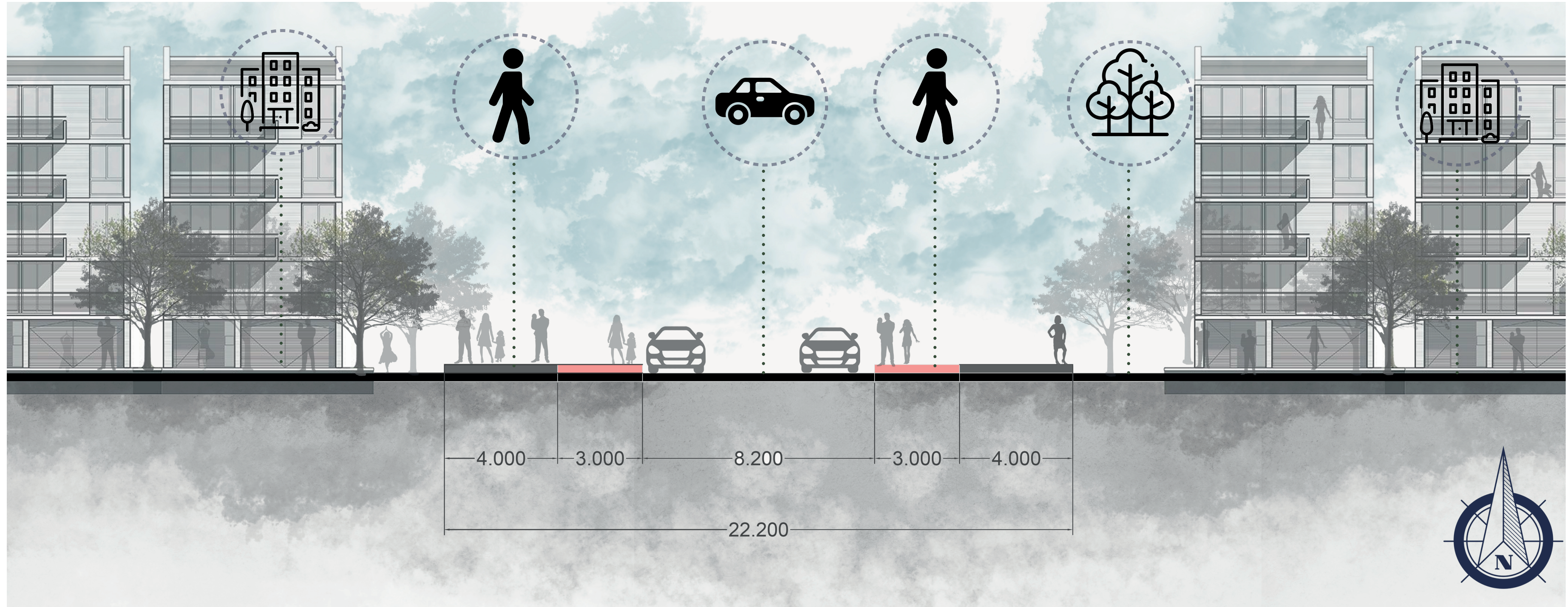
»PERFIL VIAL CALLE 12
