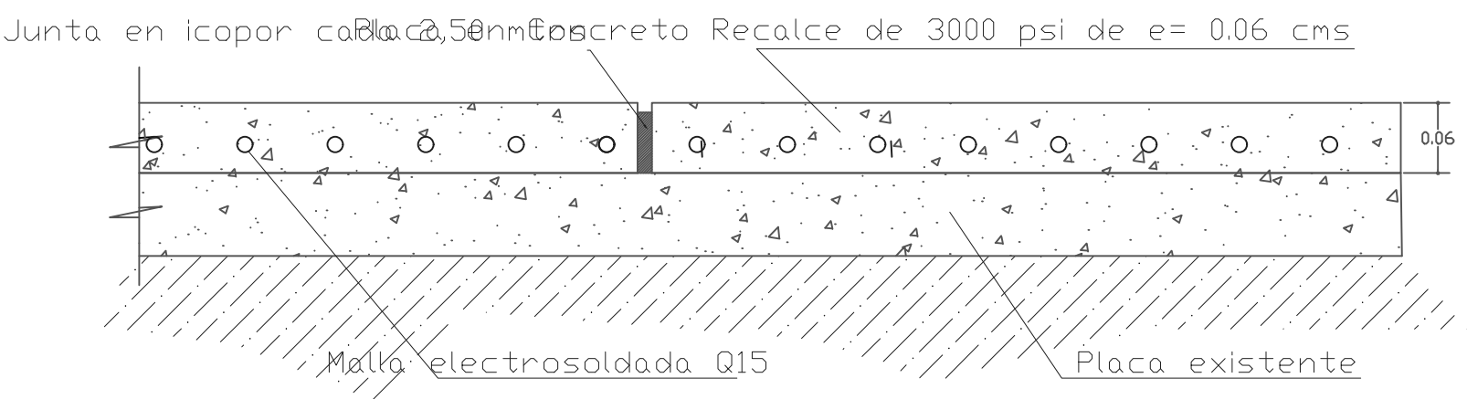
CORTE DE PLACA DE PISO
