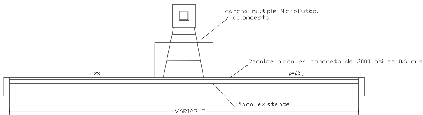
CORTE TRANSVERSAL A- A' ESC: 1:100
