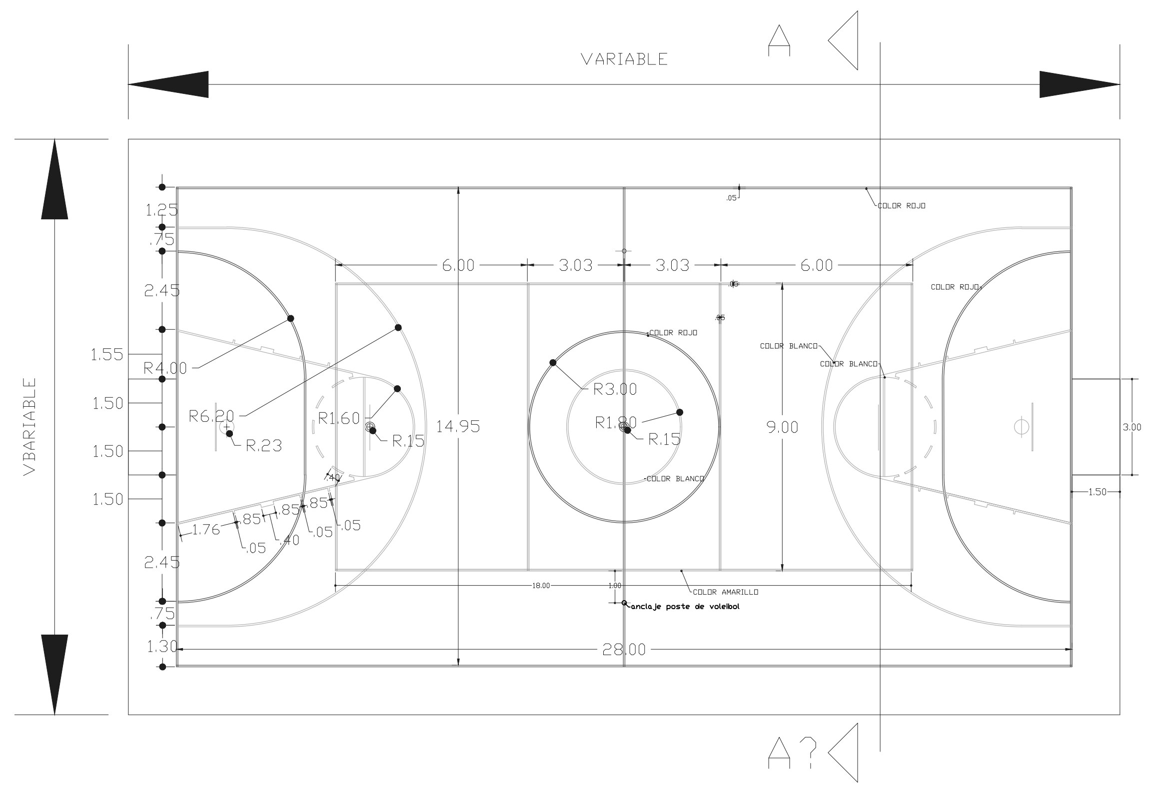
CANCHA MULTIFUNCIONAL BALONCESTO, MICROFUTBOL Y VOLEIBOL ESCALA 1:100
