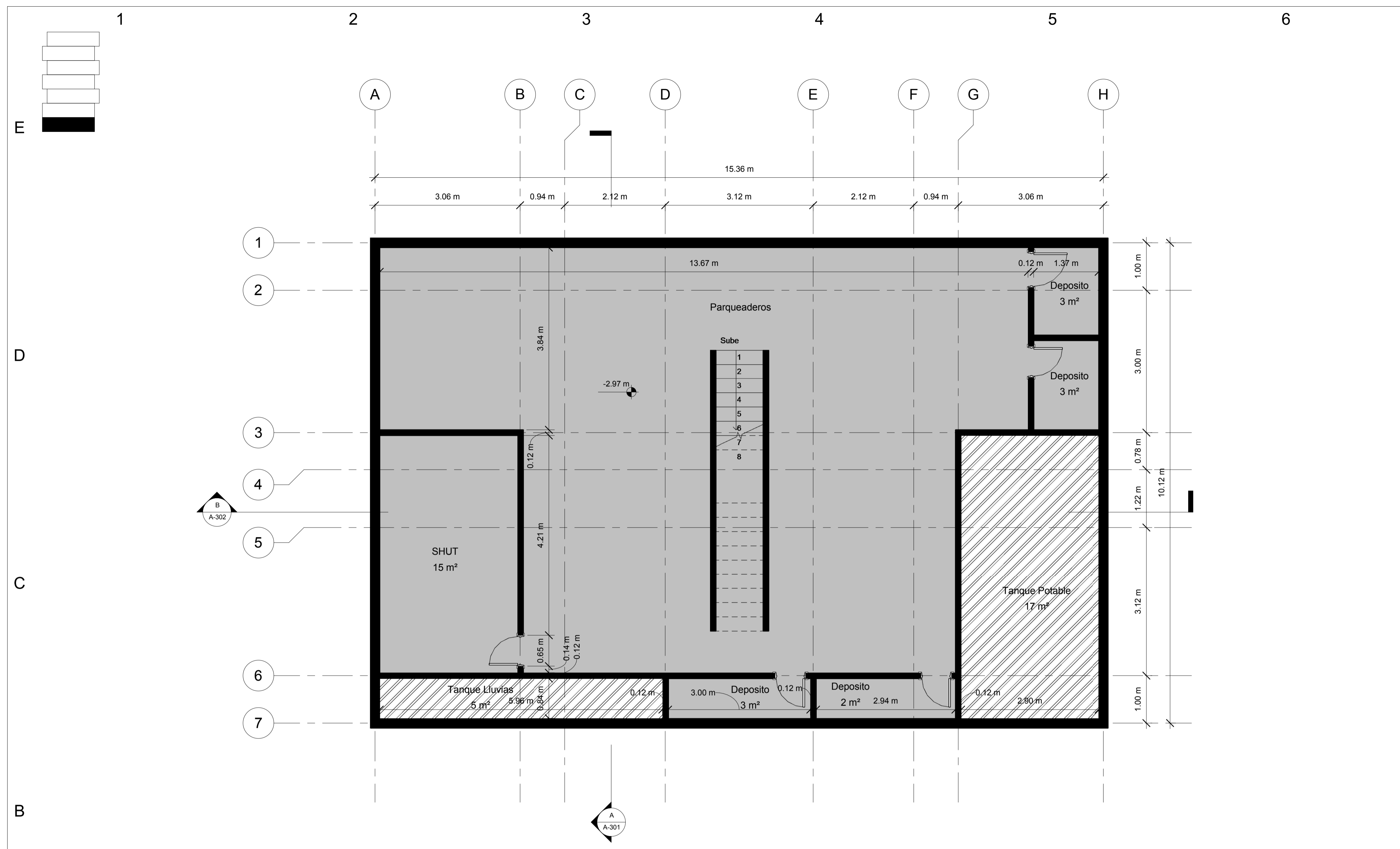
2 Semisotano Bloque 54 1 : 50
