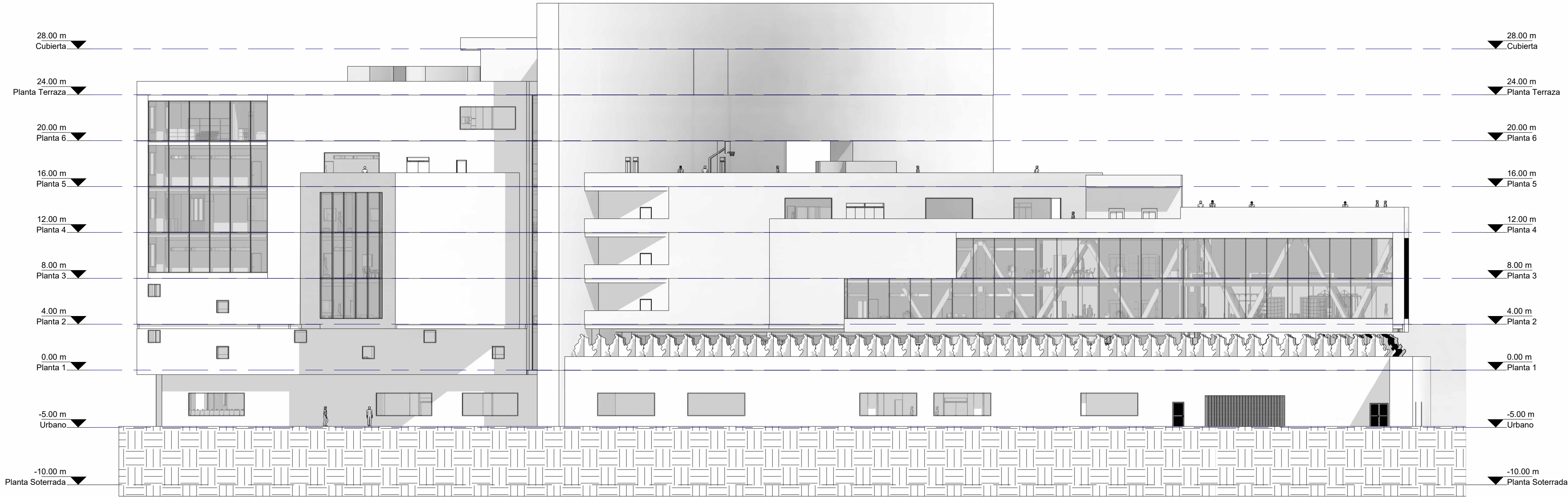
1 Fachada Norte I : 250
