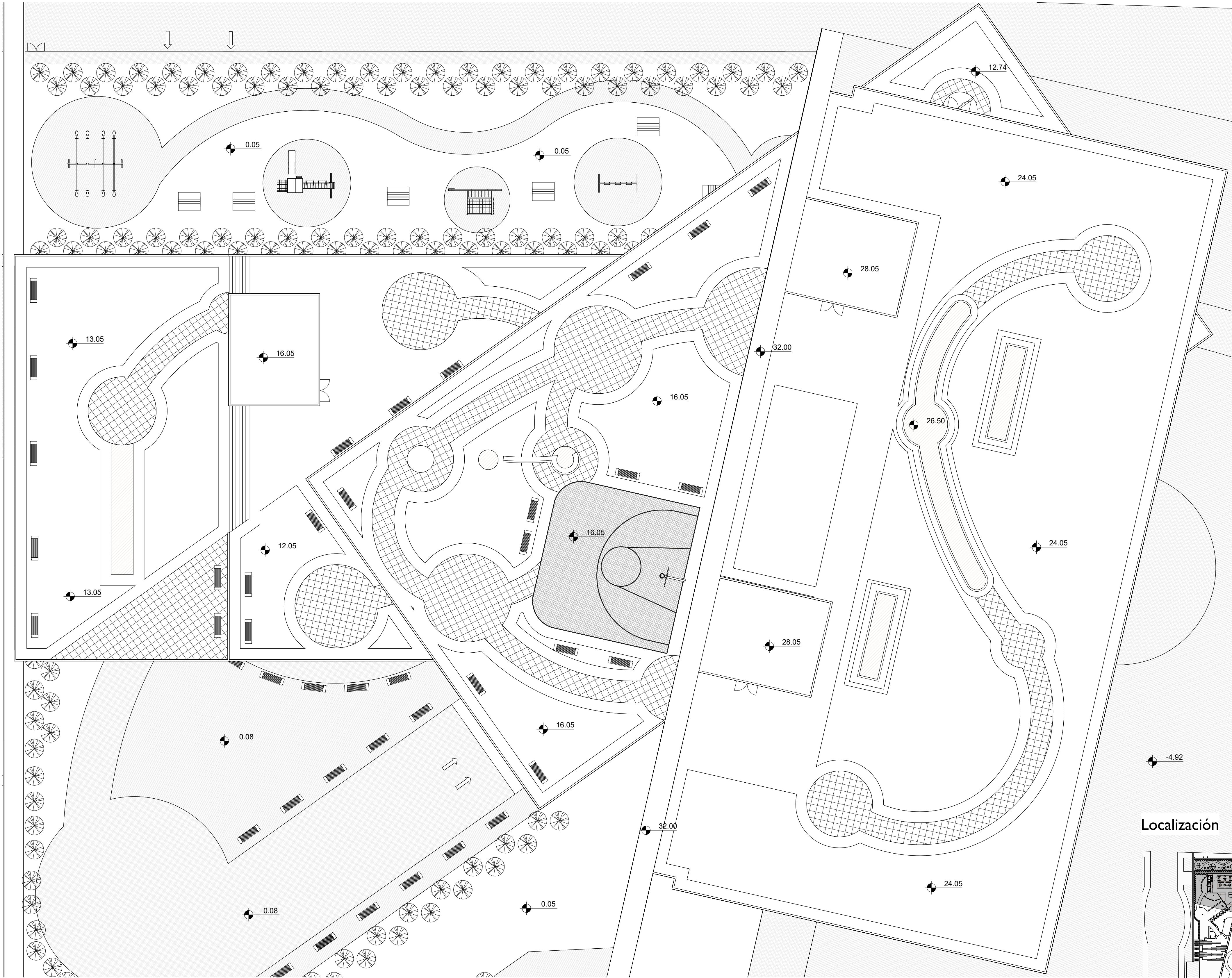
1 Planta de Cubierta General 1 : 200
