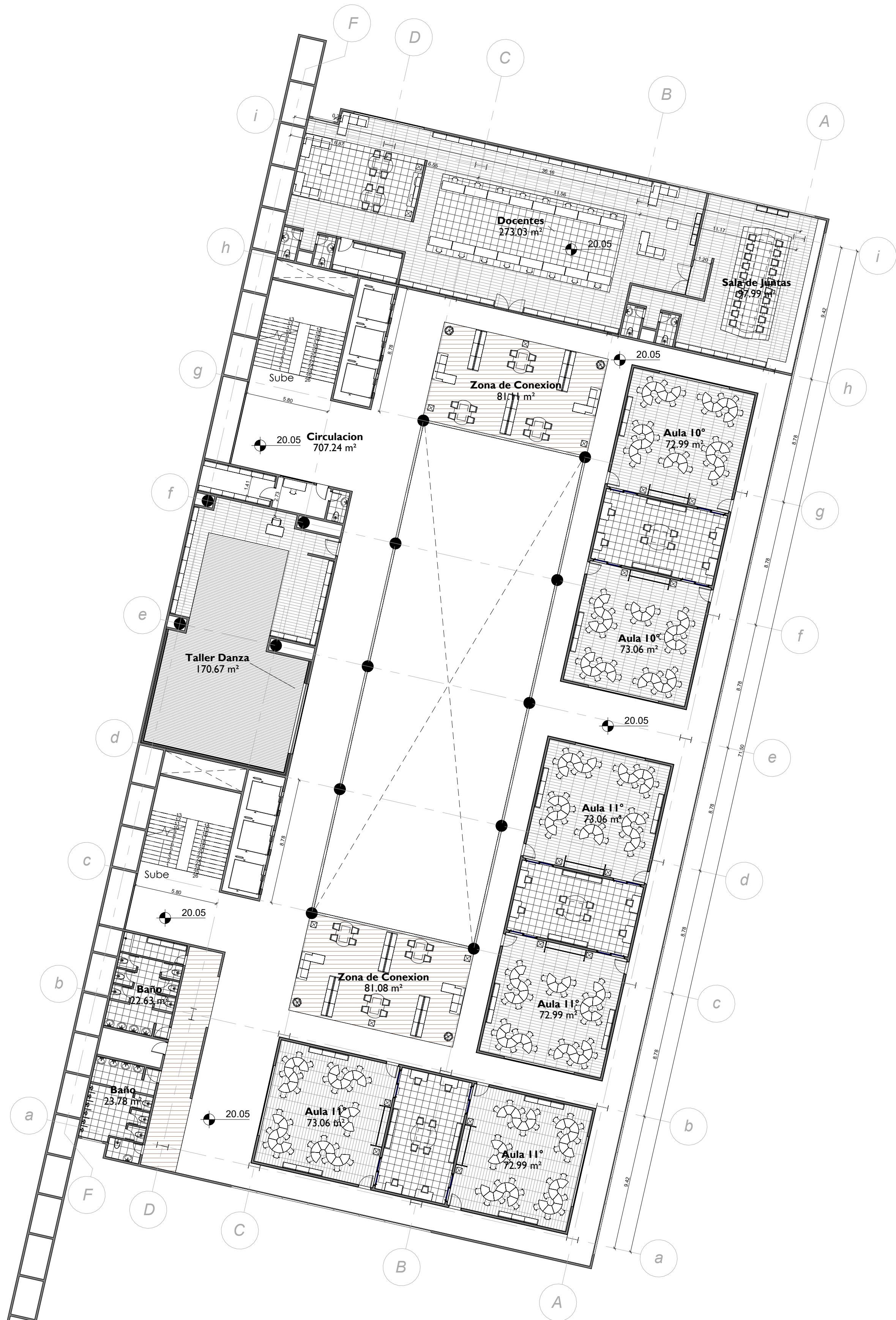
1 Planta 6 1 : 200
