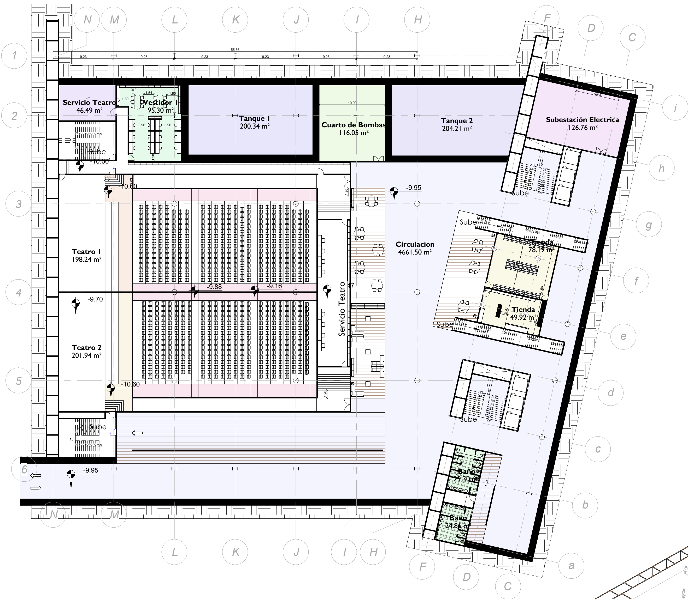
1 Uso cultural planta soterrada I : 300
