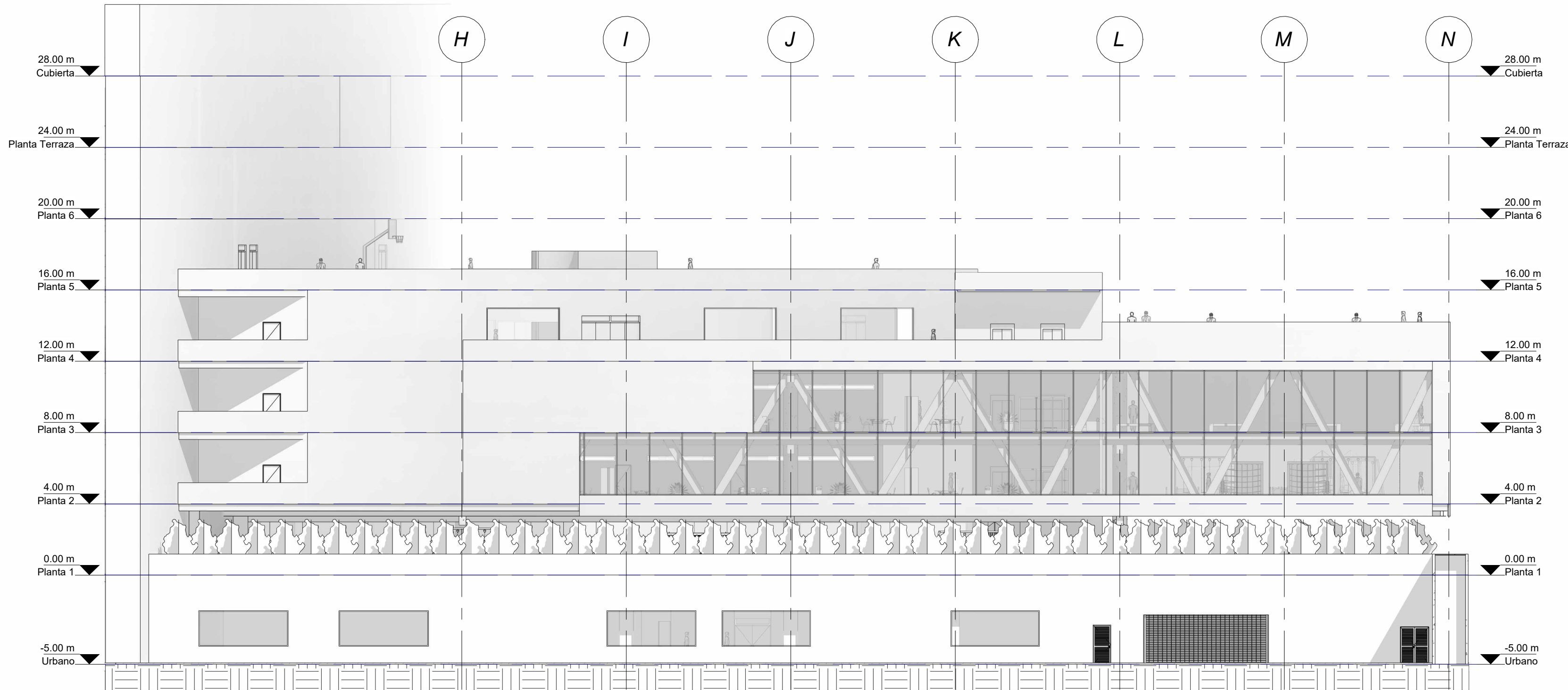
4 Fachada 7 I : 200
