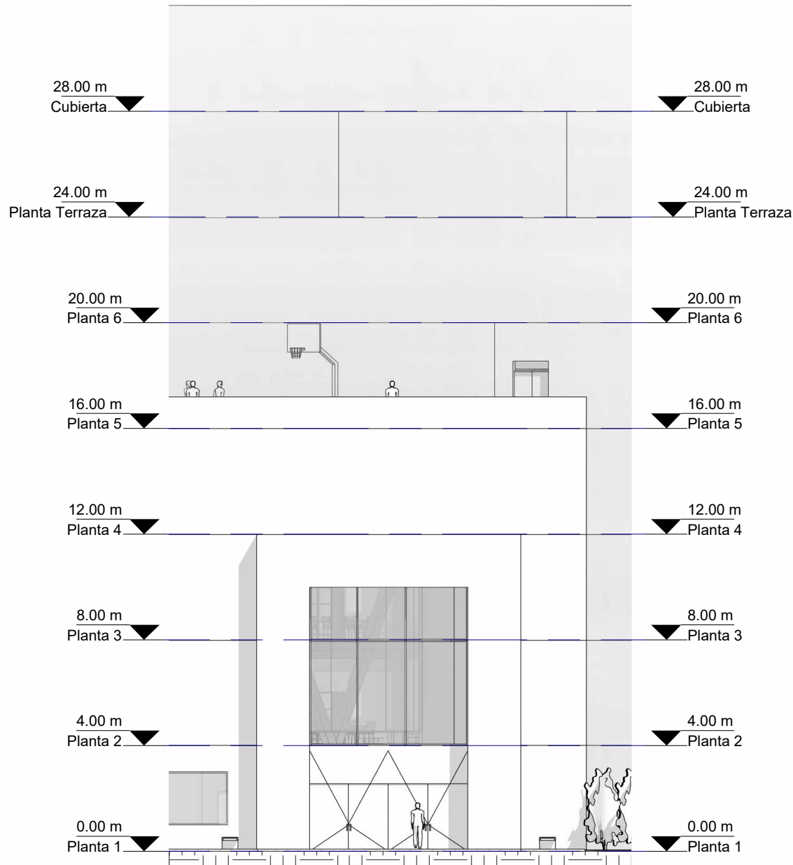
3 Fachada 4 I : 200
