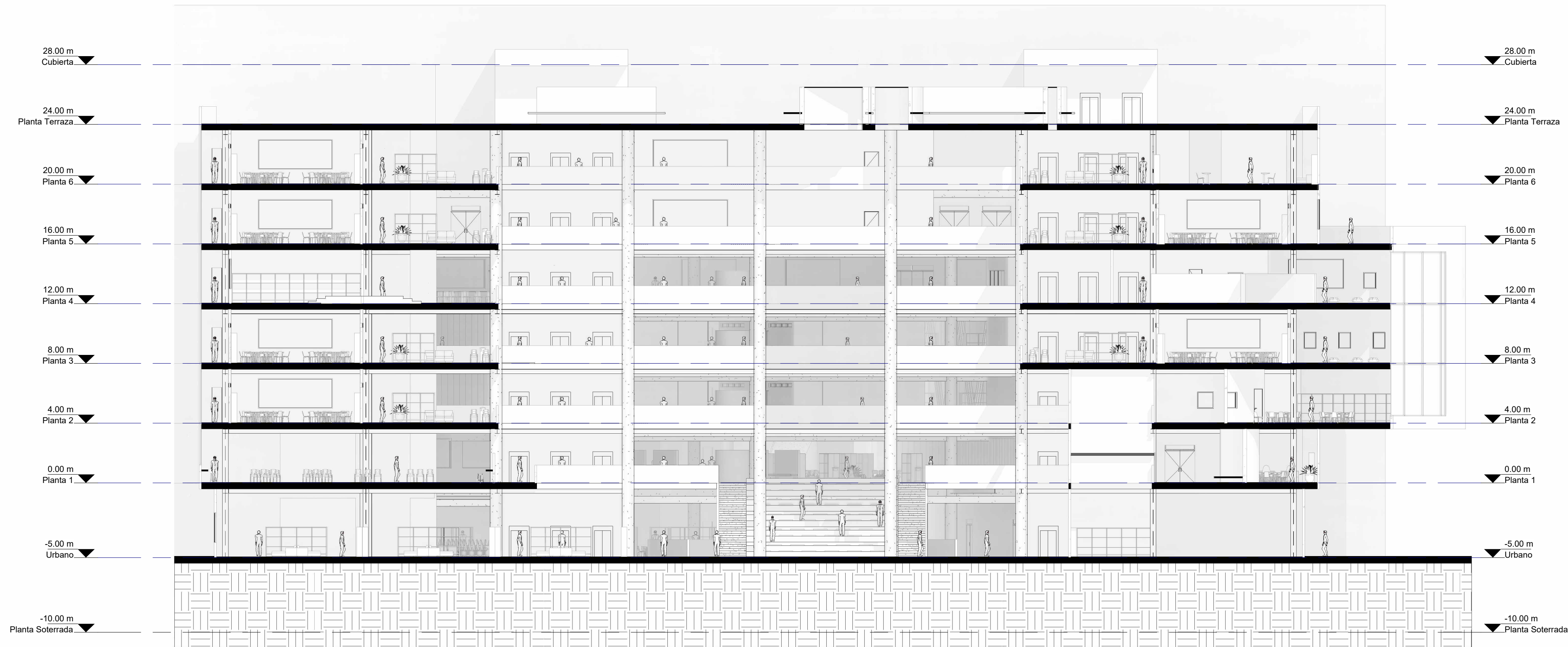
2 CORTE TRANSVERSAL 2 1 : 200
