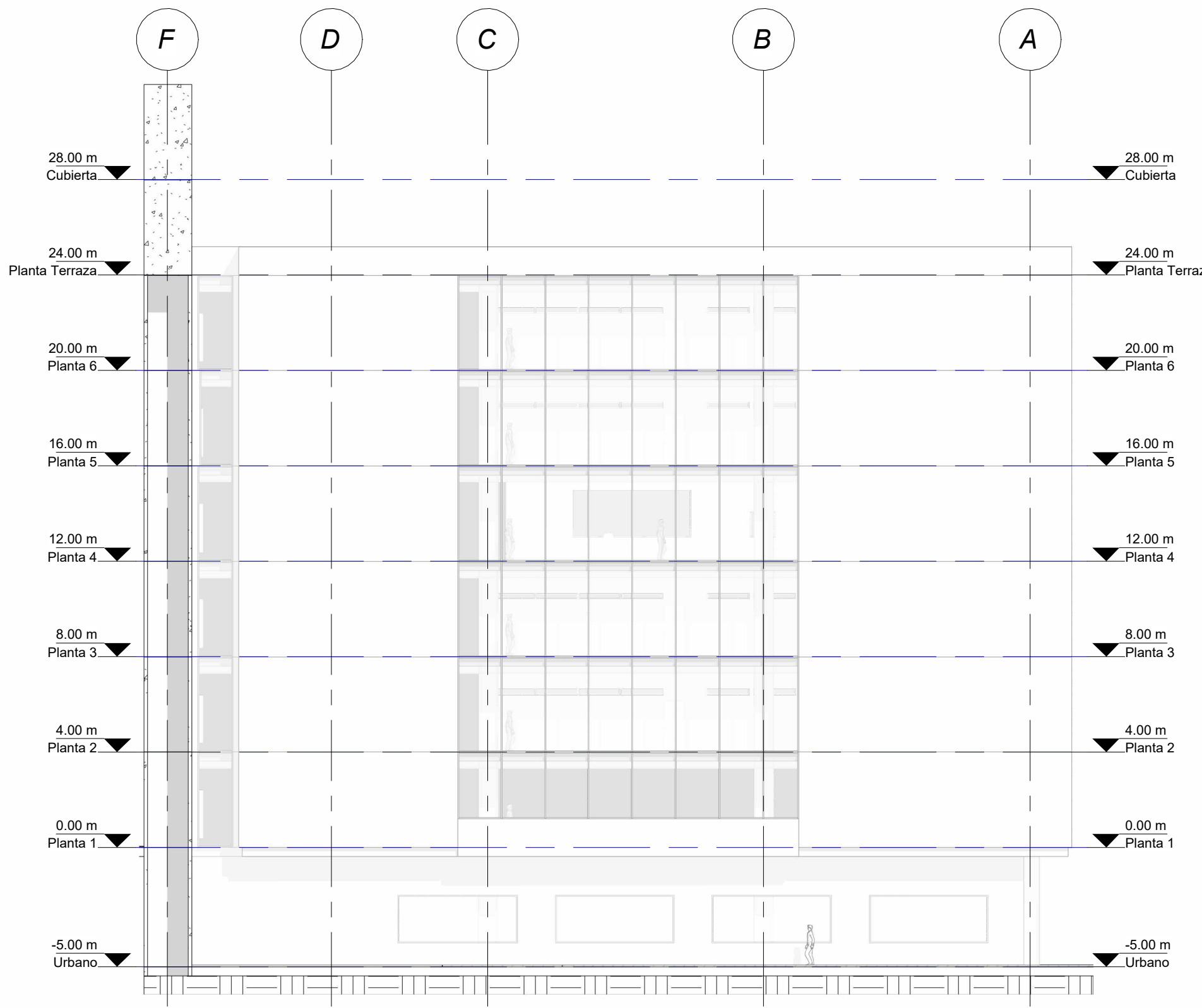
2 Fachada 2 I : 200
