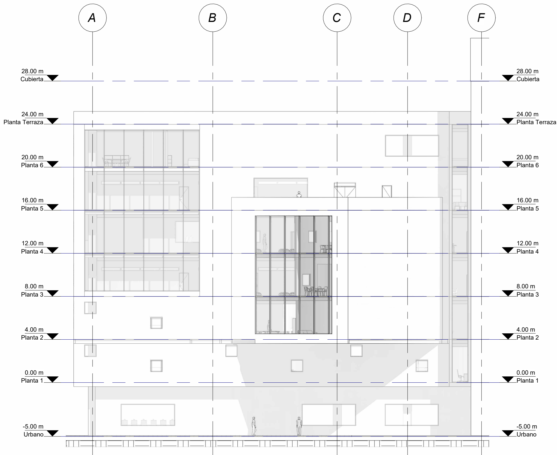
1 Fachada 1 I : 200
