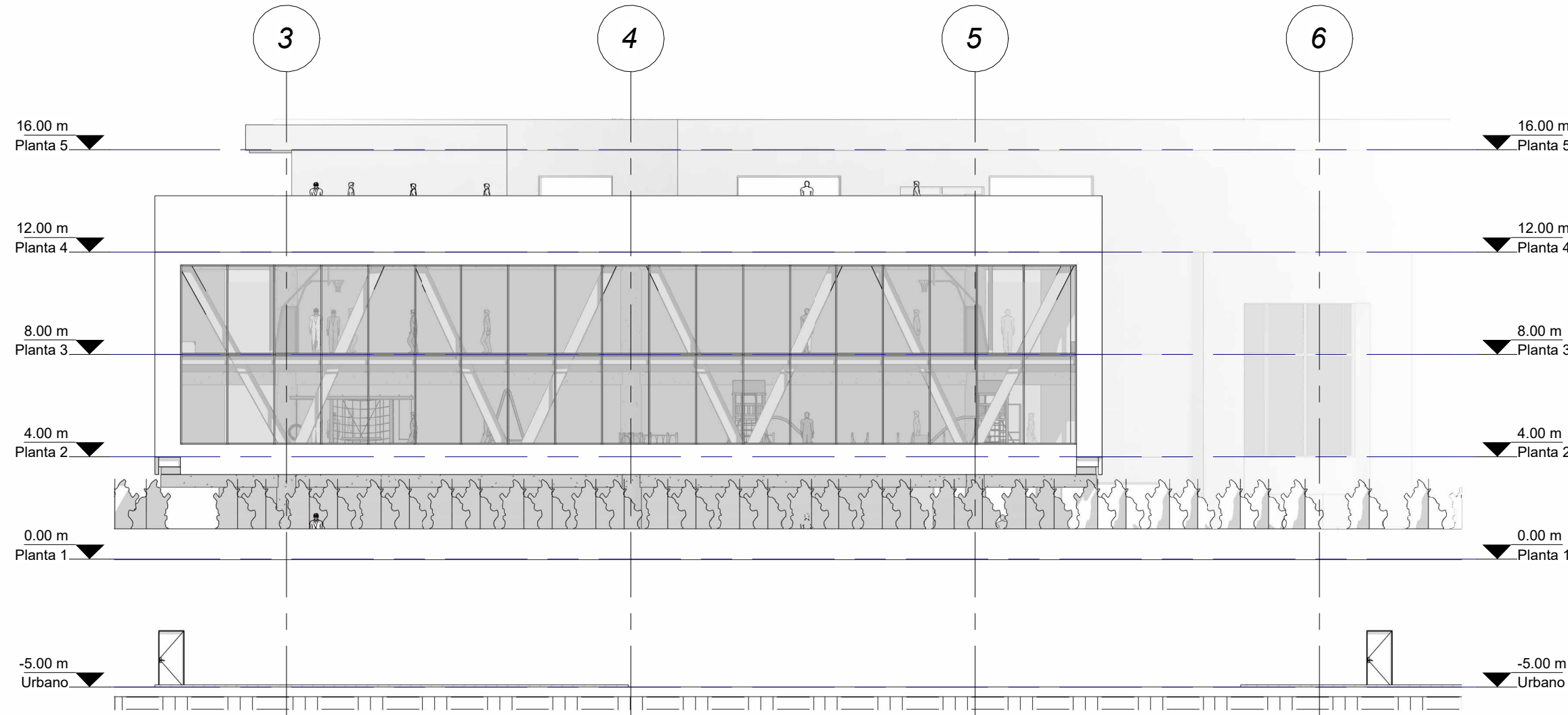
2 Fachada 6 I : 200
