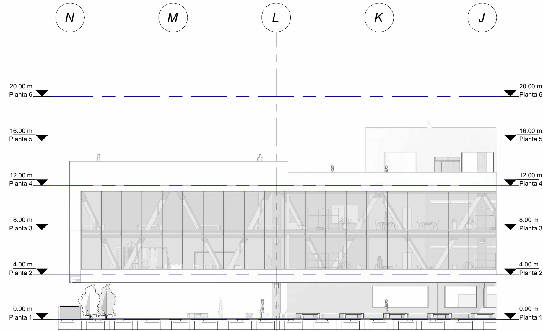
1 Fachada 5 I : 200
