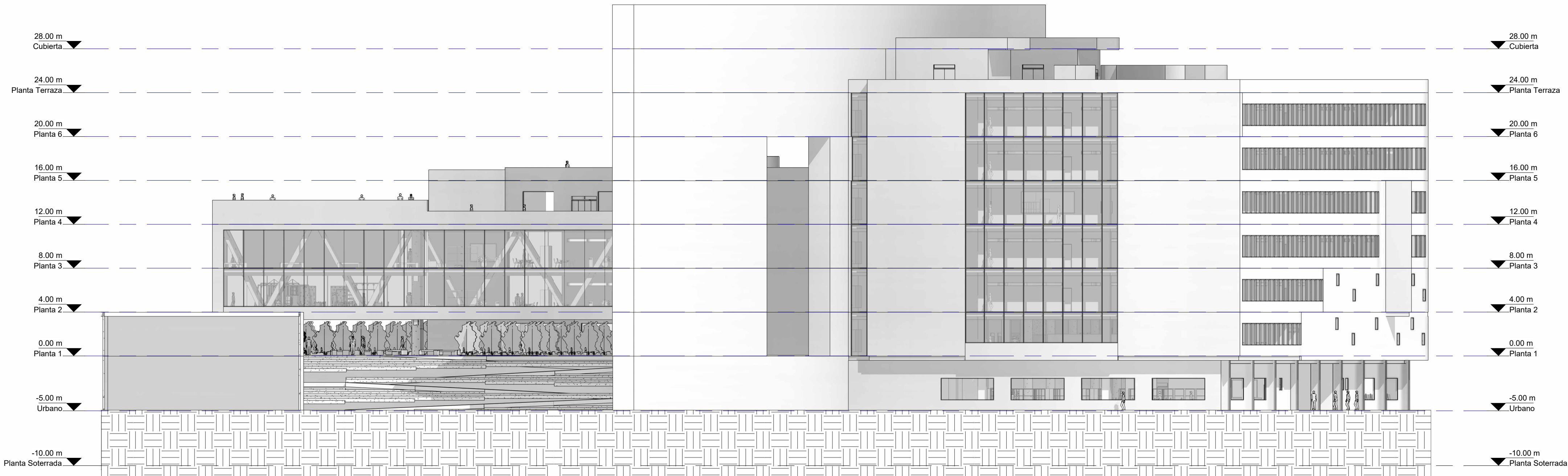
2 Fachada Sur I : 250
