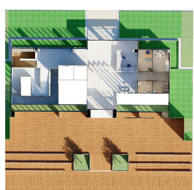
PLANTA ILUSTRATIVA
