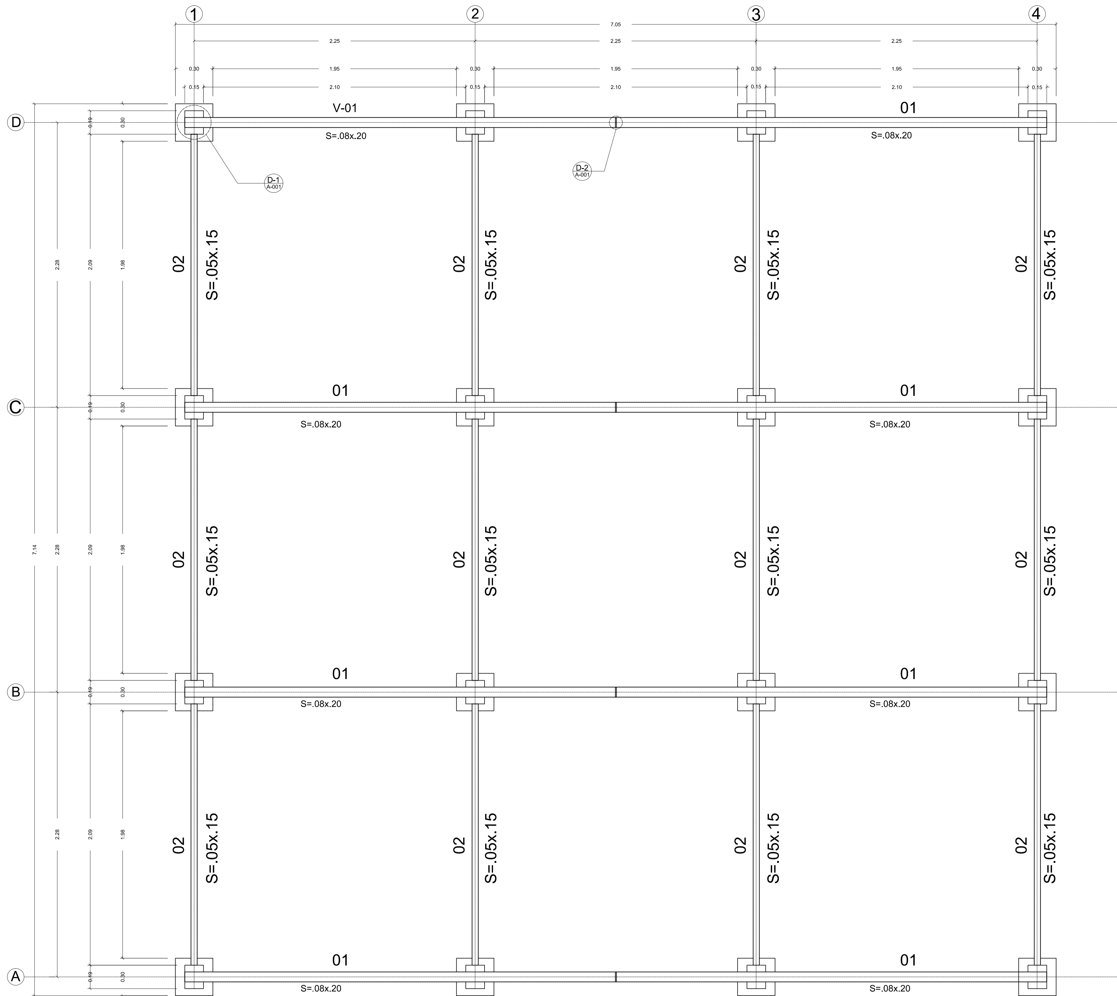
E Planta de cimentacion ESC 1:50
