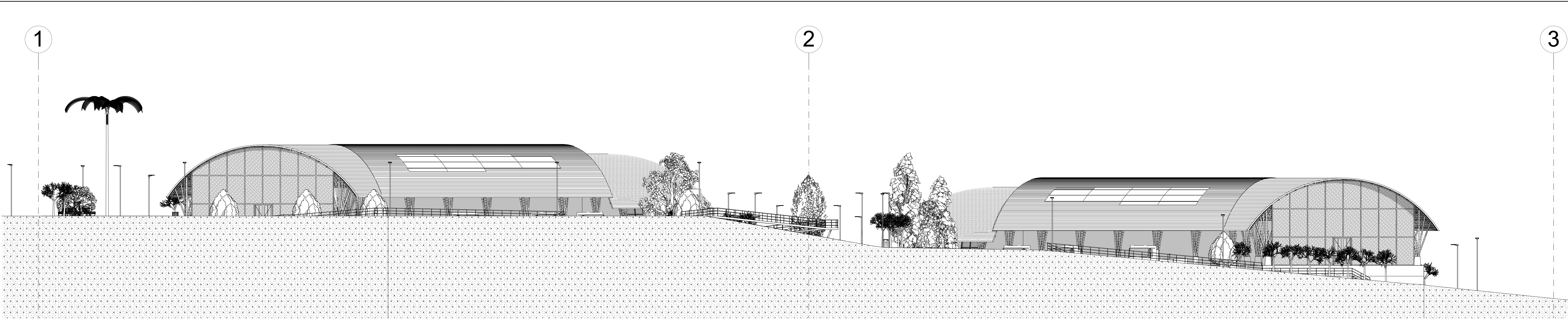
Sección Longitudinal
