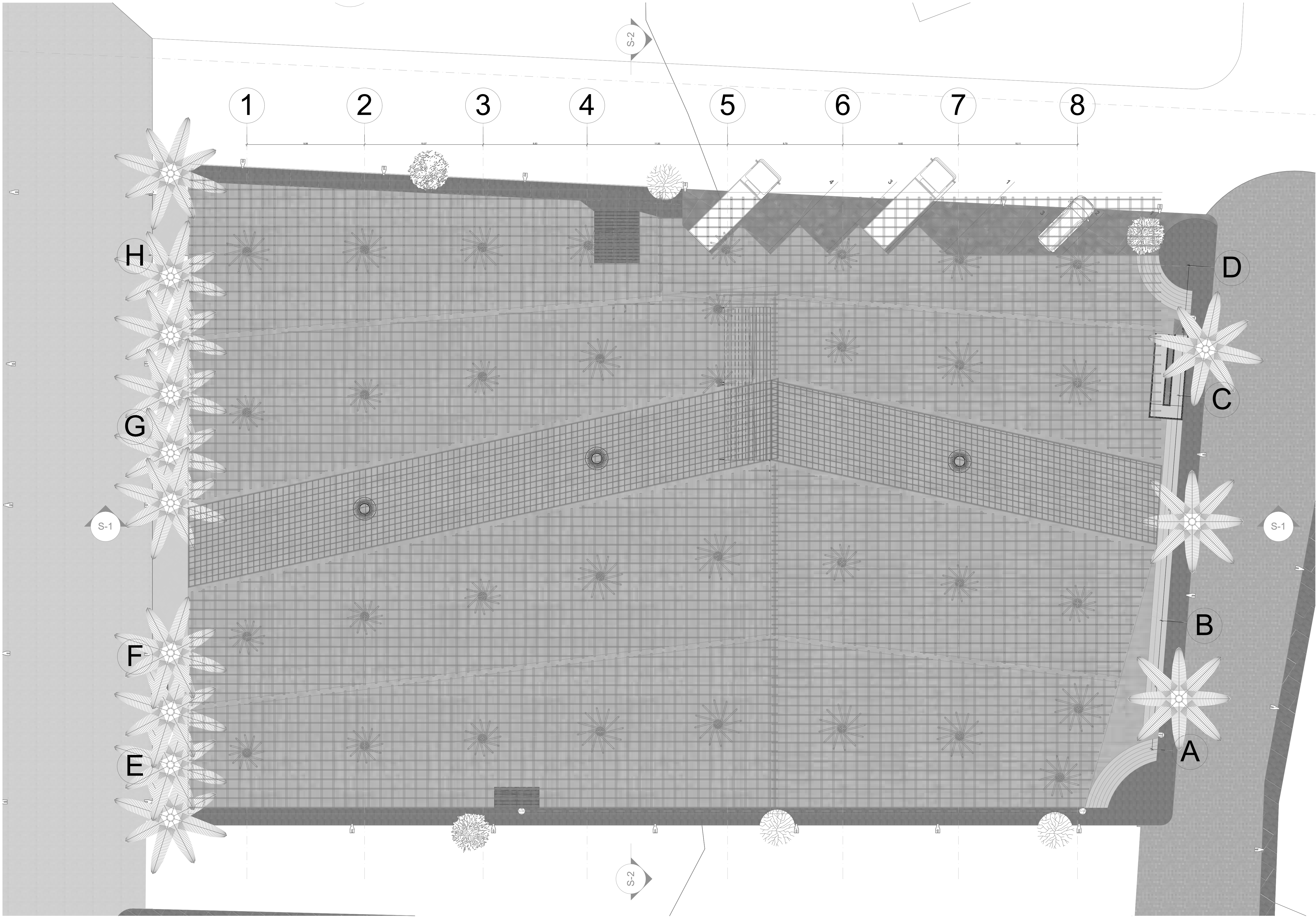
Planta Estructural - Cubierta
