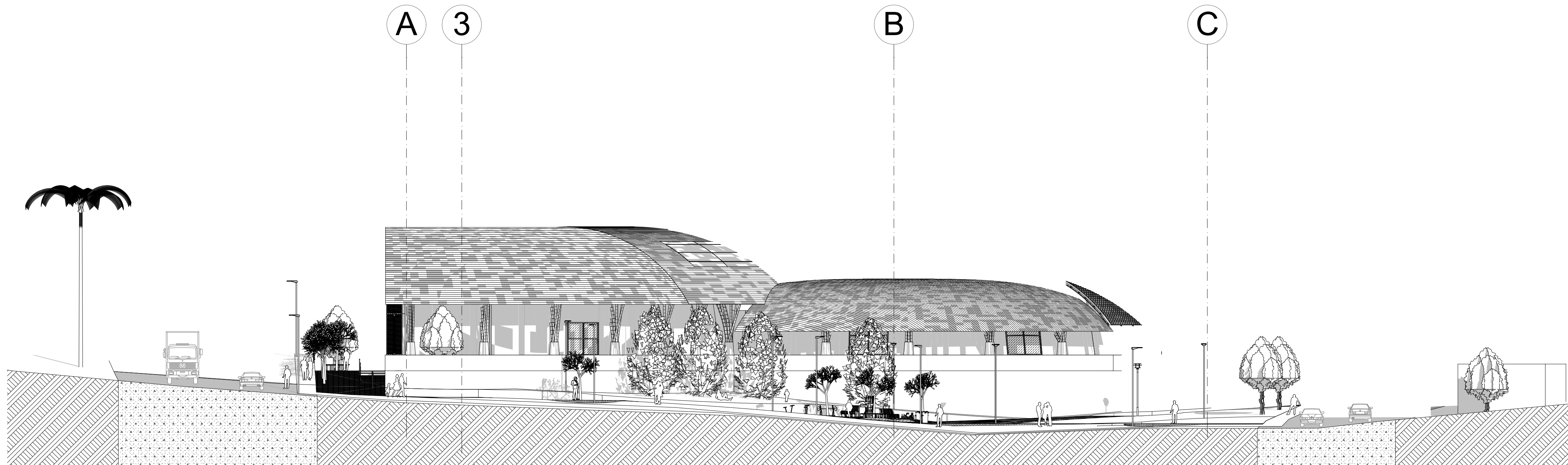
S-6 Sección Transversal 1:200
