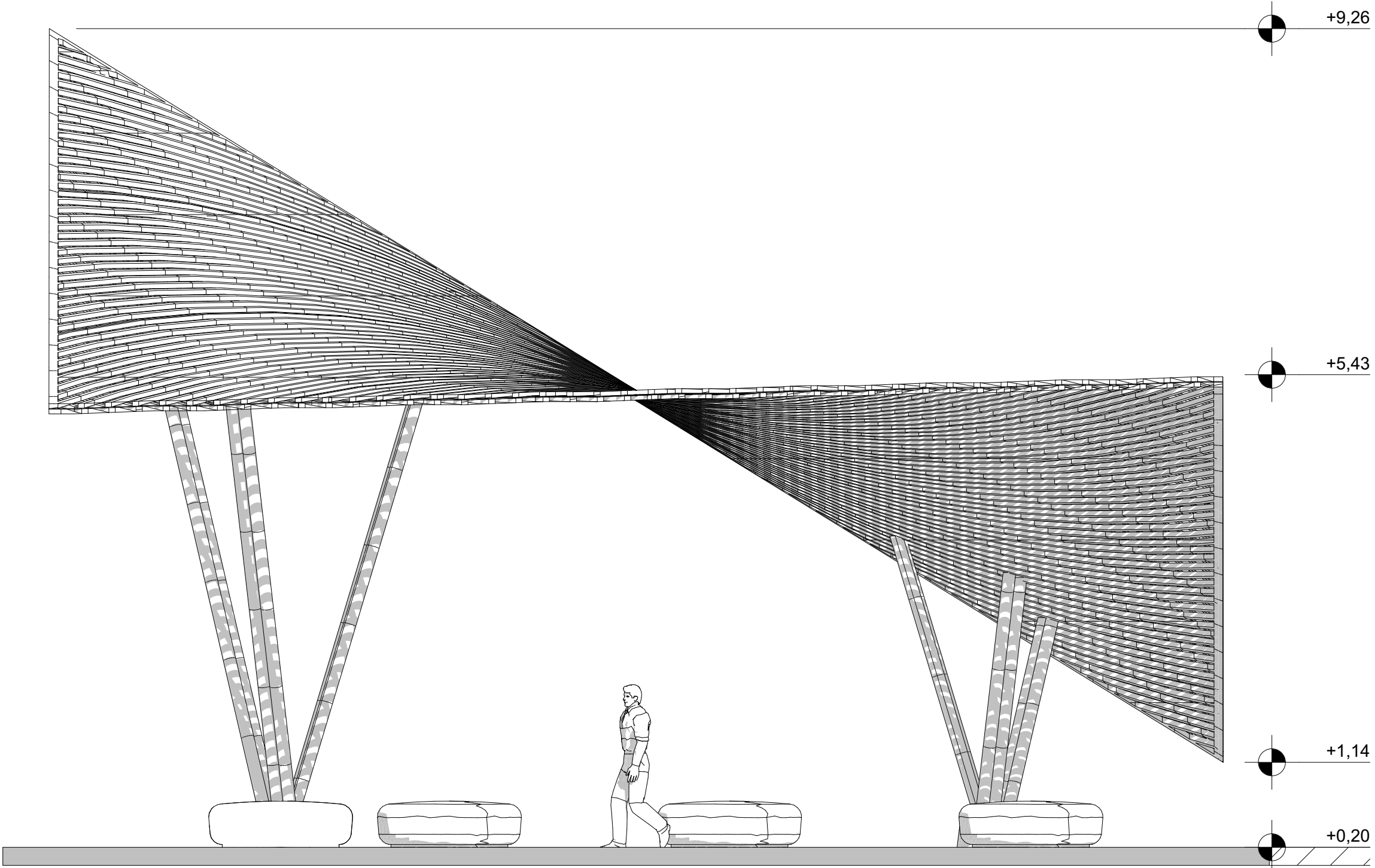
SD-02 Sección Transversal 1:50
