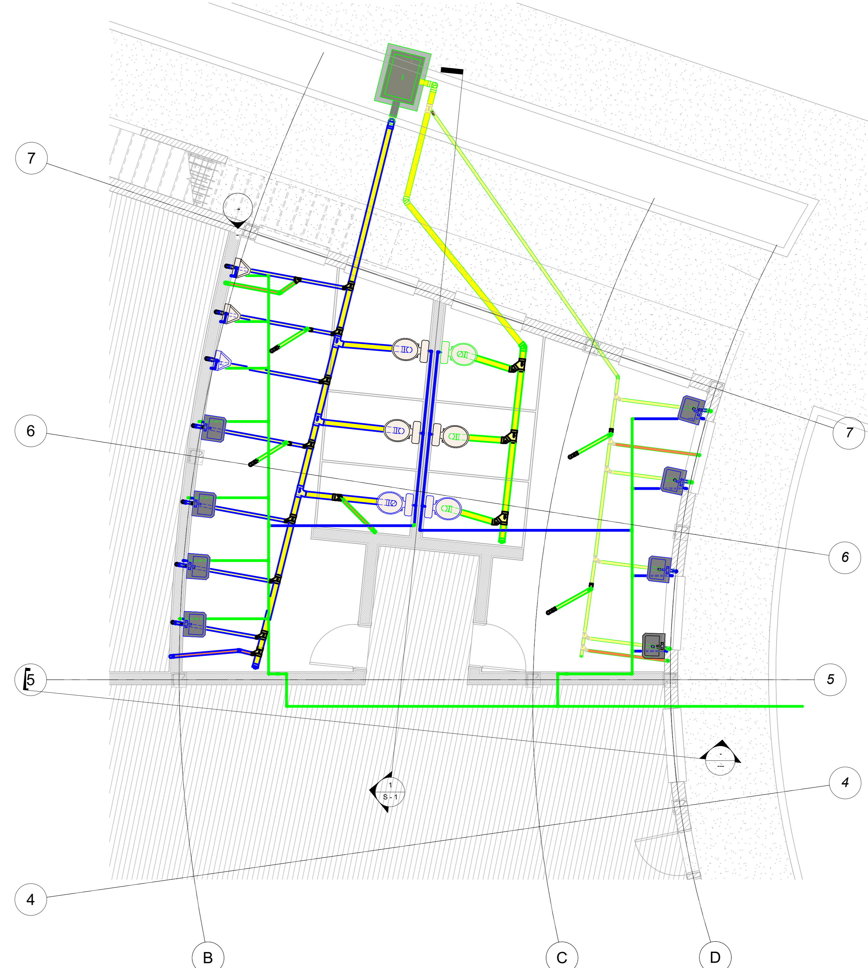
3 01_CIMENTACIÓN 1:50
