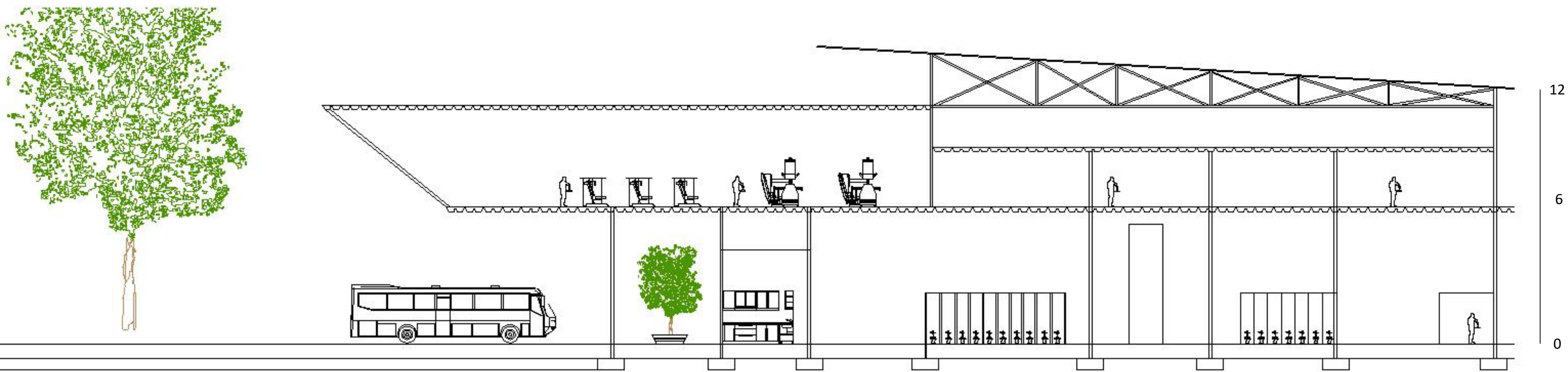
Sección de la terminal
