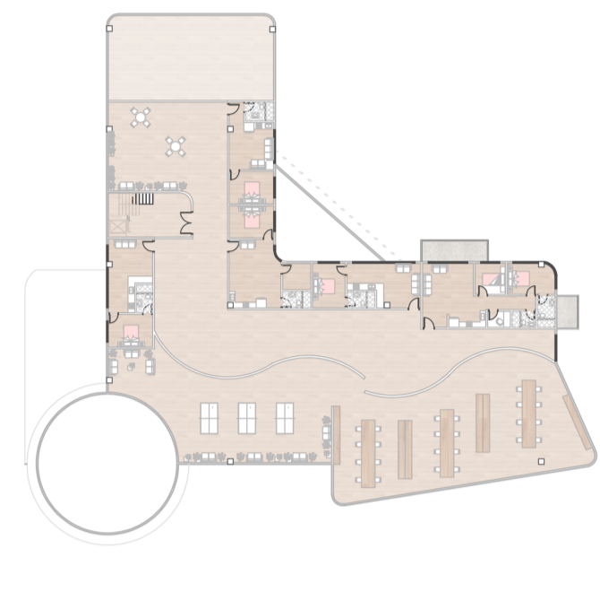
PLANTA PISO 3,5
