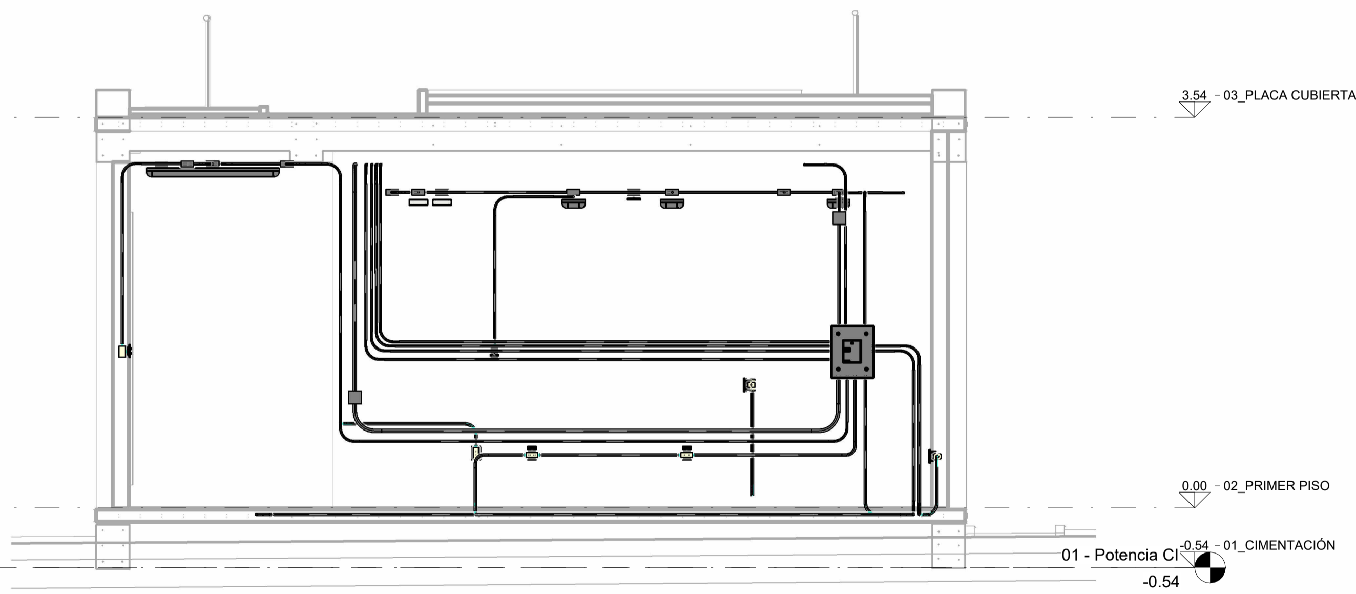
3 Sección 3 1 : 35
