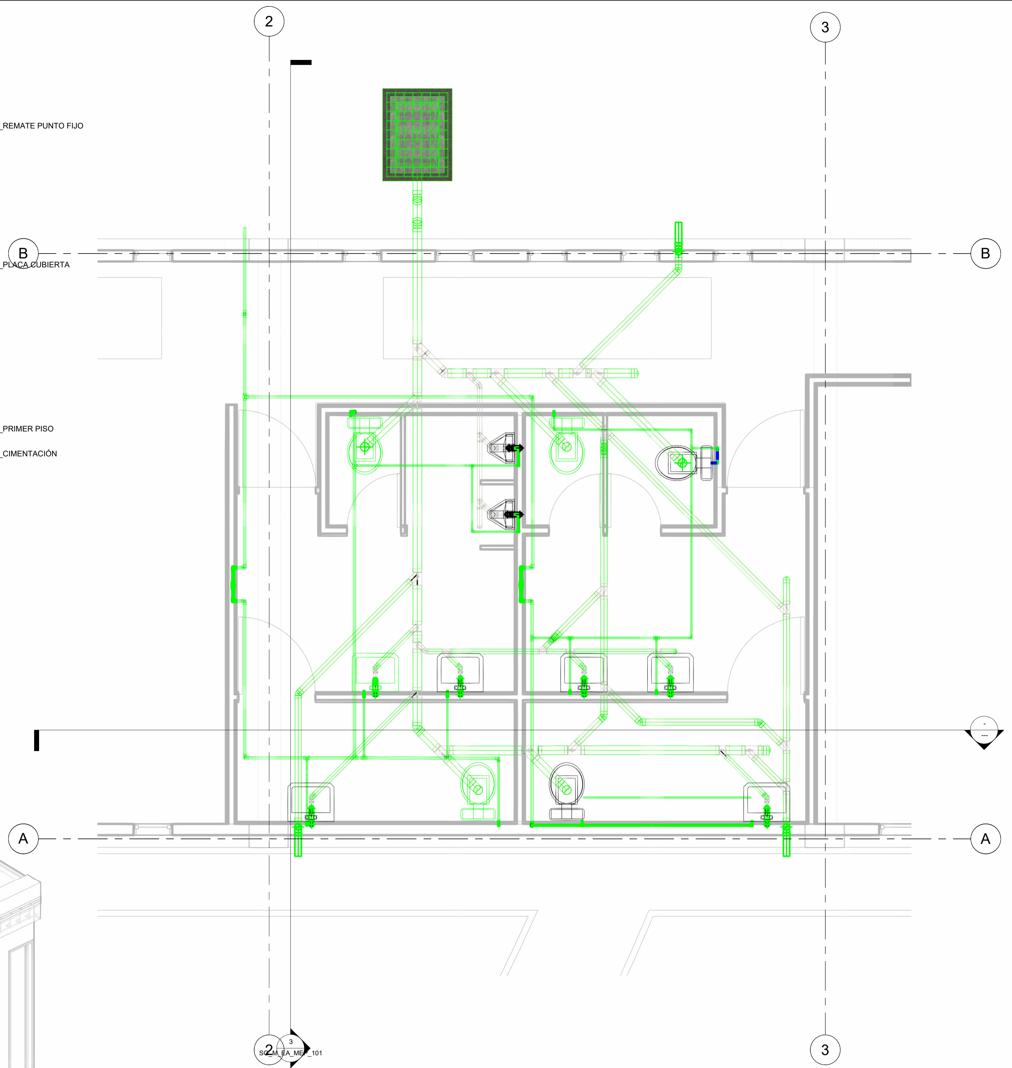
1 02_PRIMER PISO 1:30
