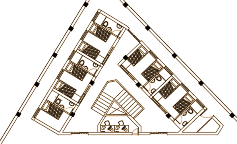
PLANTA DE SEGUNDO NIVEL Y PISO TIPO
