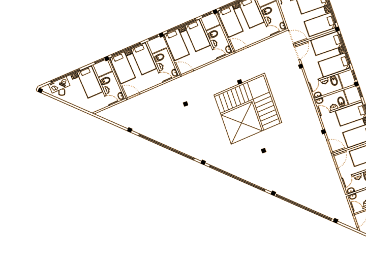
PLANTA SEGUNDO NIVEL Y PISO TIPO
