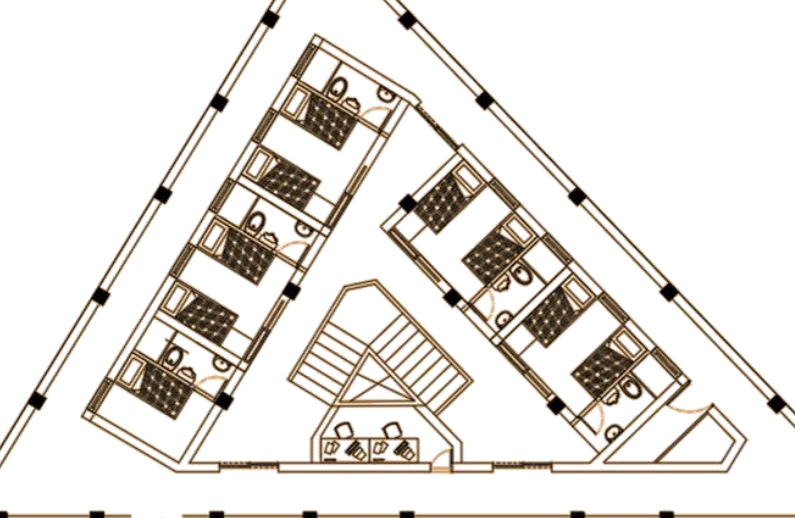
PLANTA DE SEGUNDO NIVEL Y PISO TIPO
