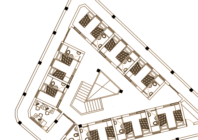
PLANTA DE SEGUNDO NIVEL Y PISO TIPO
