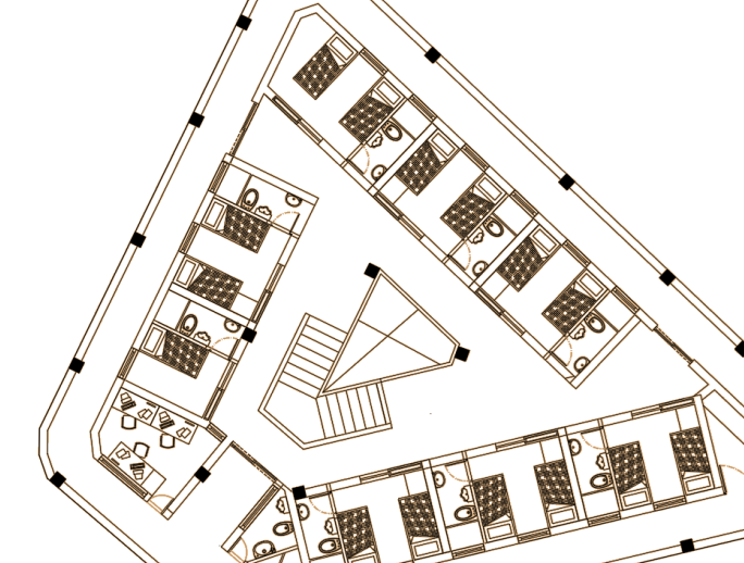
PLANTA DE SEGUNDO NIVEL Y PISO TIPO
