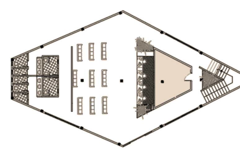
PLANTA PISO TIPO NIVEL 2 Y 3
