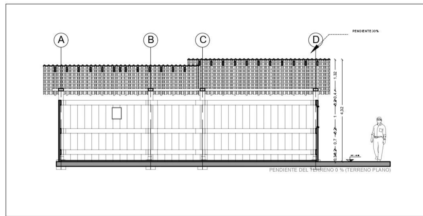
P1 CORTE LONGITUDINAL ESCALA 1:100
