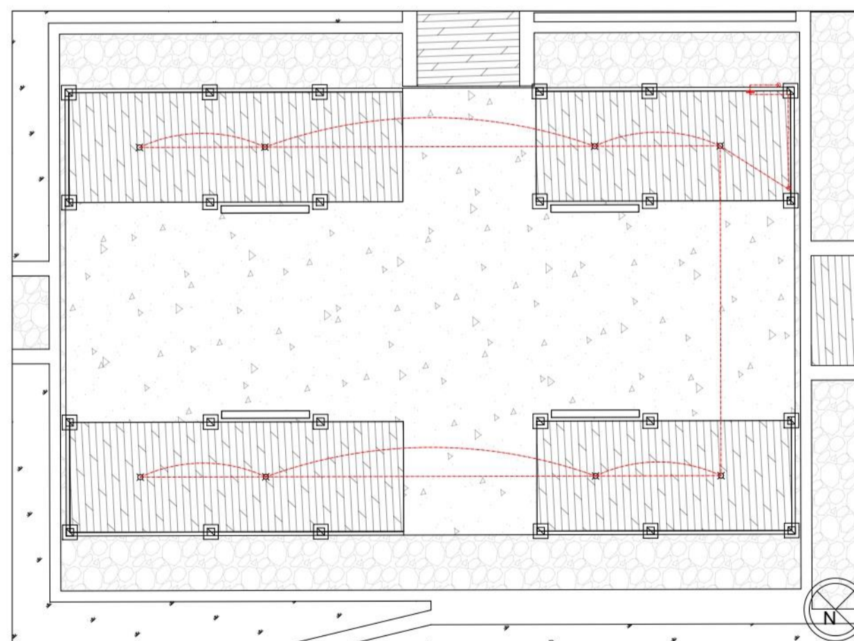
P2 INSTALACION ELECTRICA ESCALA 1:200
