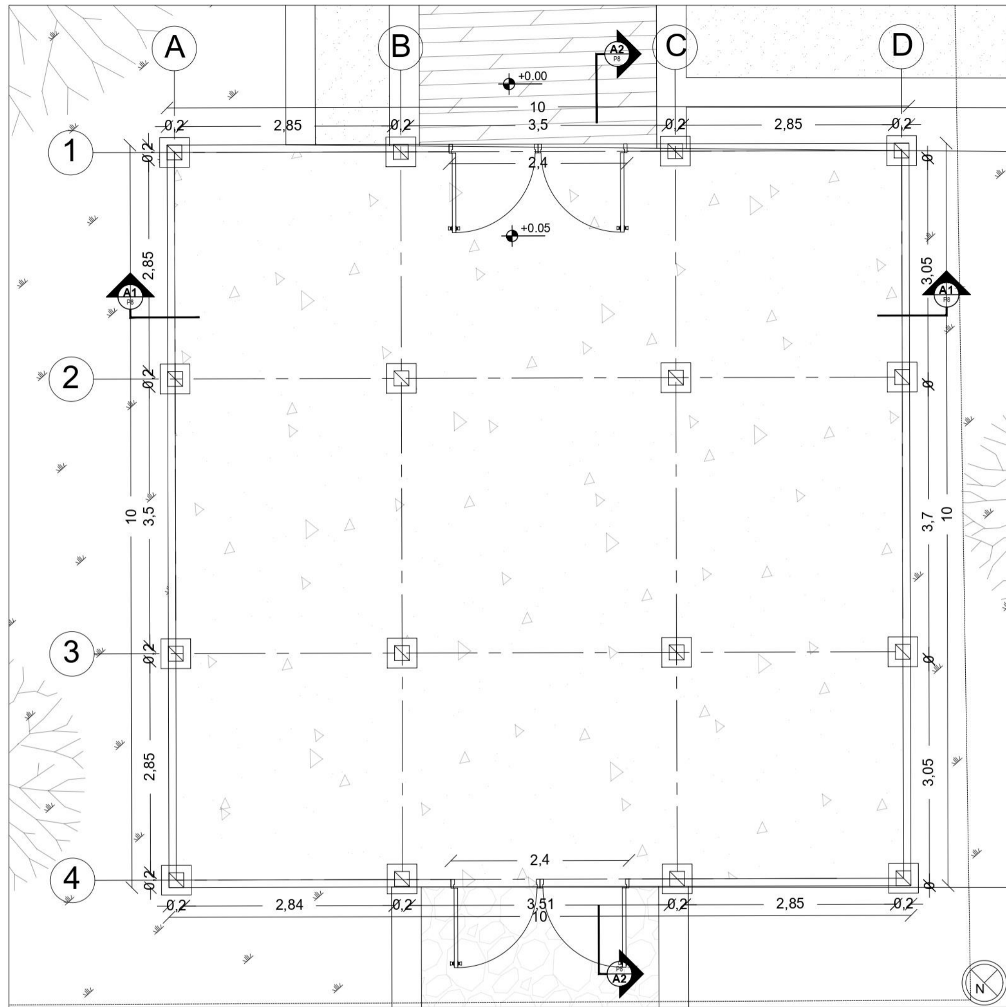
P1 PLANTA TIPO PARA BODEGA Y TALLERES CONSTRUCCION ESCALA 1:50
