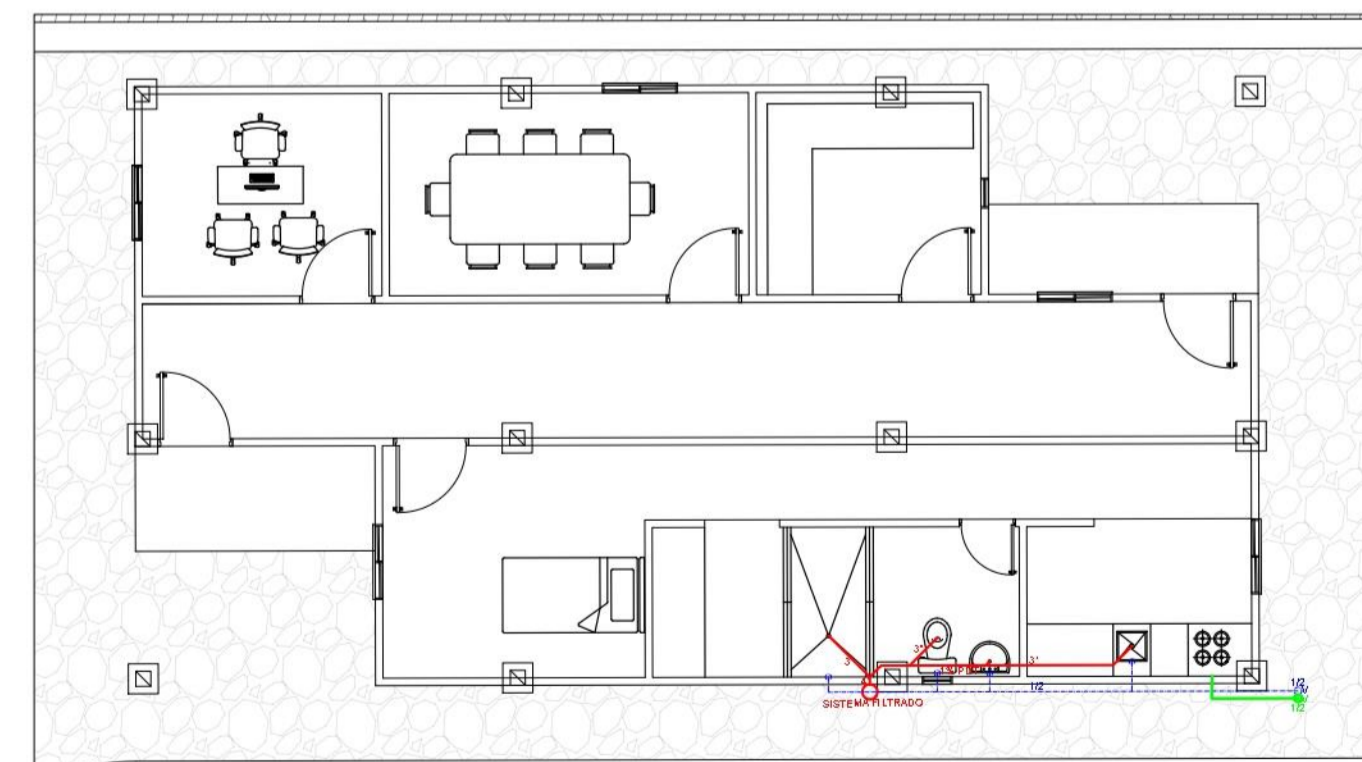
P6 INSTALACIONES HIDROSANITARIAS Y GAS ESCALA 1:100
