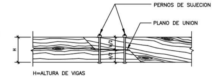
UNION VIGAS LONGITUDINALES
