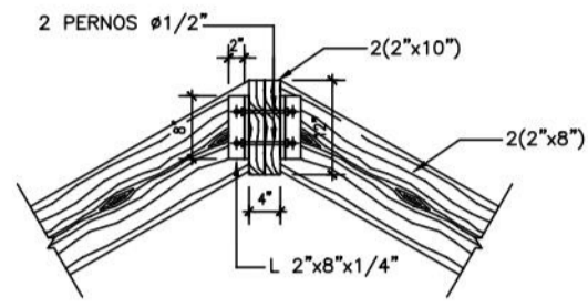
DETALLE CABALLETE (SECCION)
