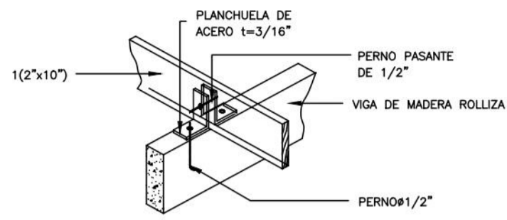
UNION DE VIGA MADERA
