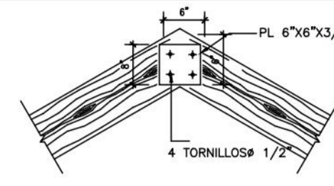
SECCION CABALLETE
