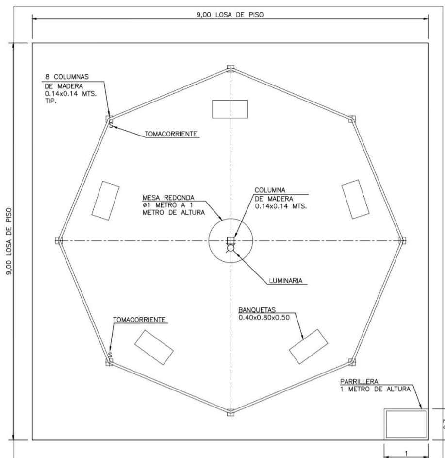
VISTA DE PLANTA NIVEL ±0.00
