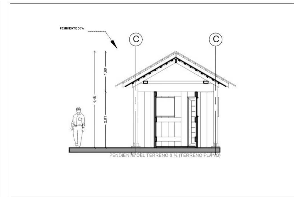
P1 CORTE TRANSVERSAL ESCALA 1:100
