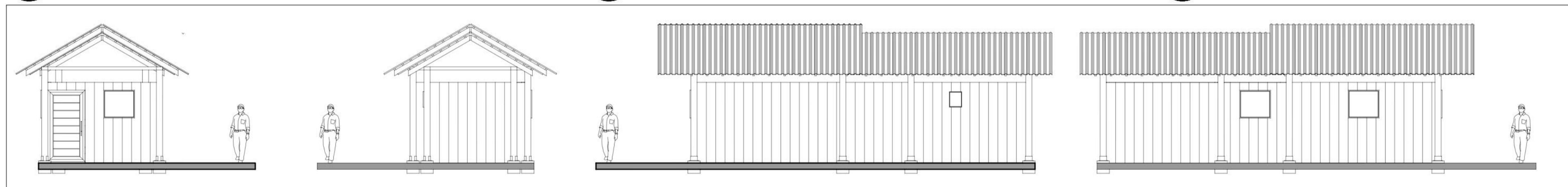
P1 FACHADAS FRONTAL - TRASERA - DERECHA - IZQUIERDA ESCALA 1:100
