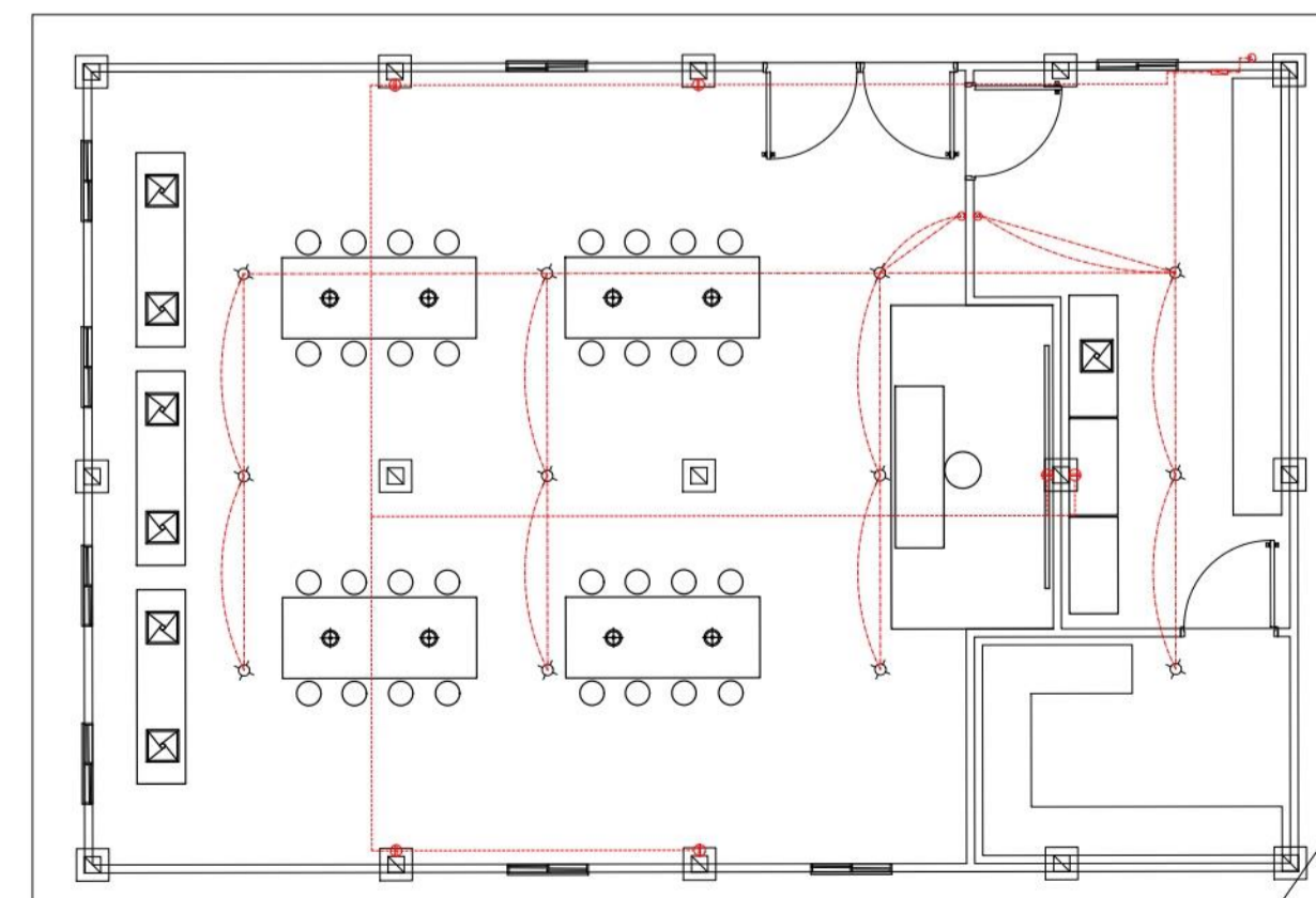
P5 INSTALACION ELECTRICA ESCALA 1:100
