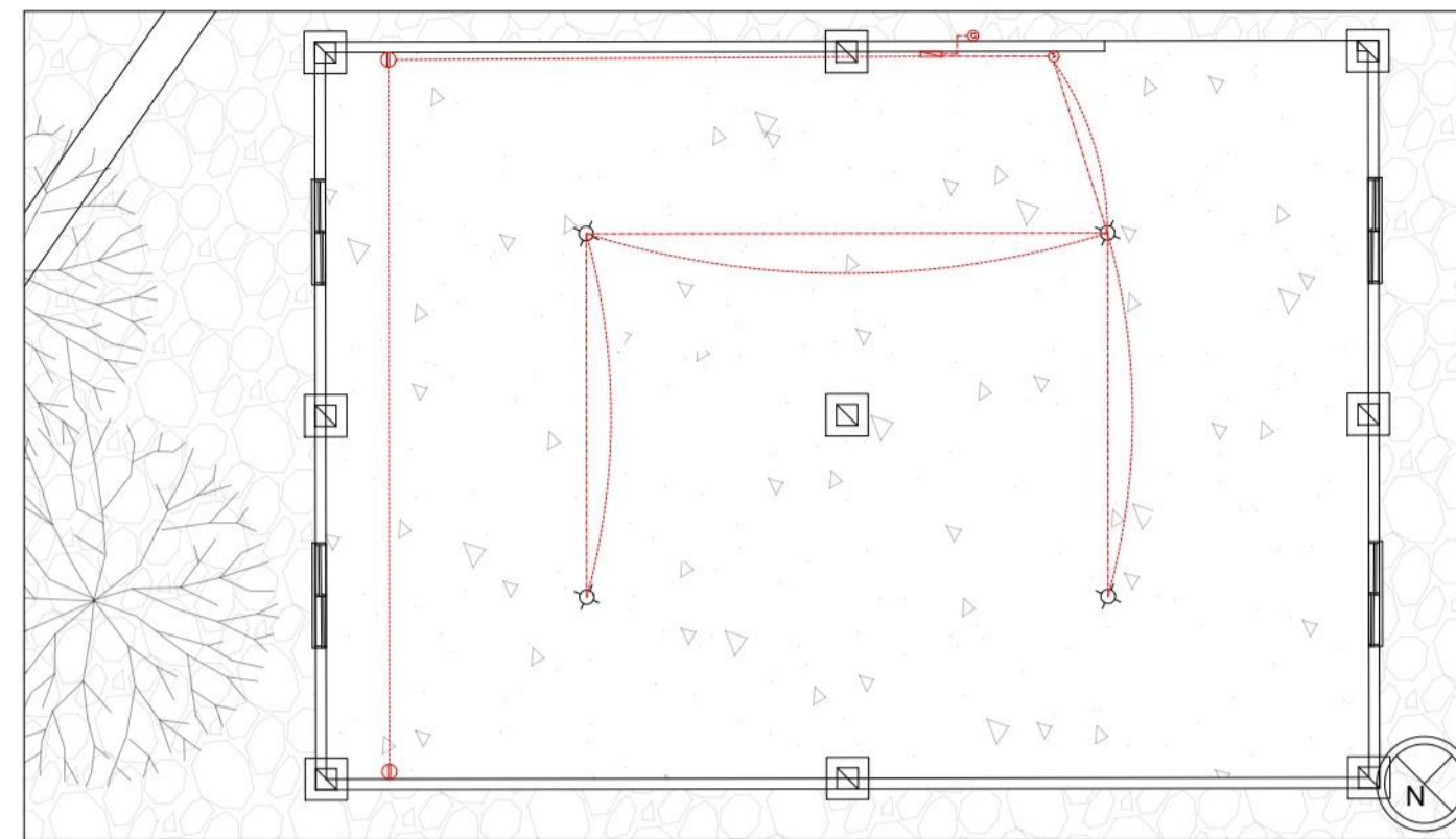
P4 INSTALACIONES ELECTRICAS ESCALA 1:75
