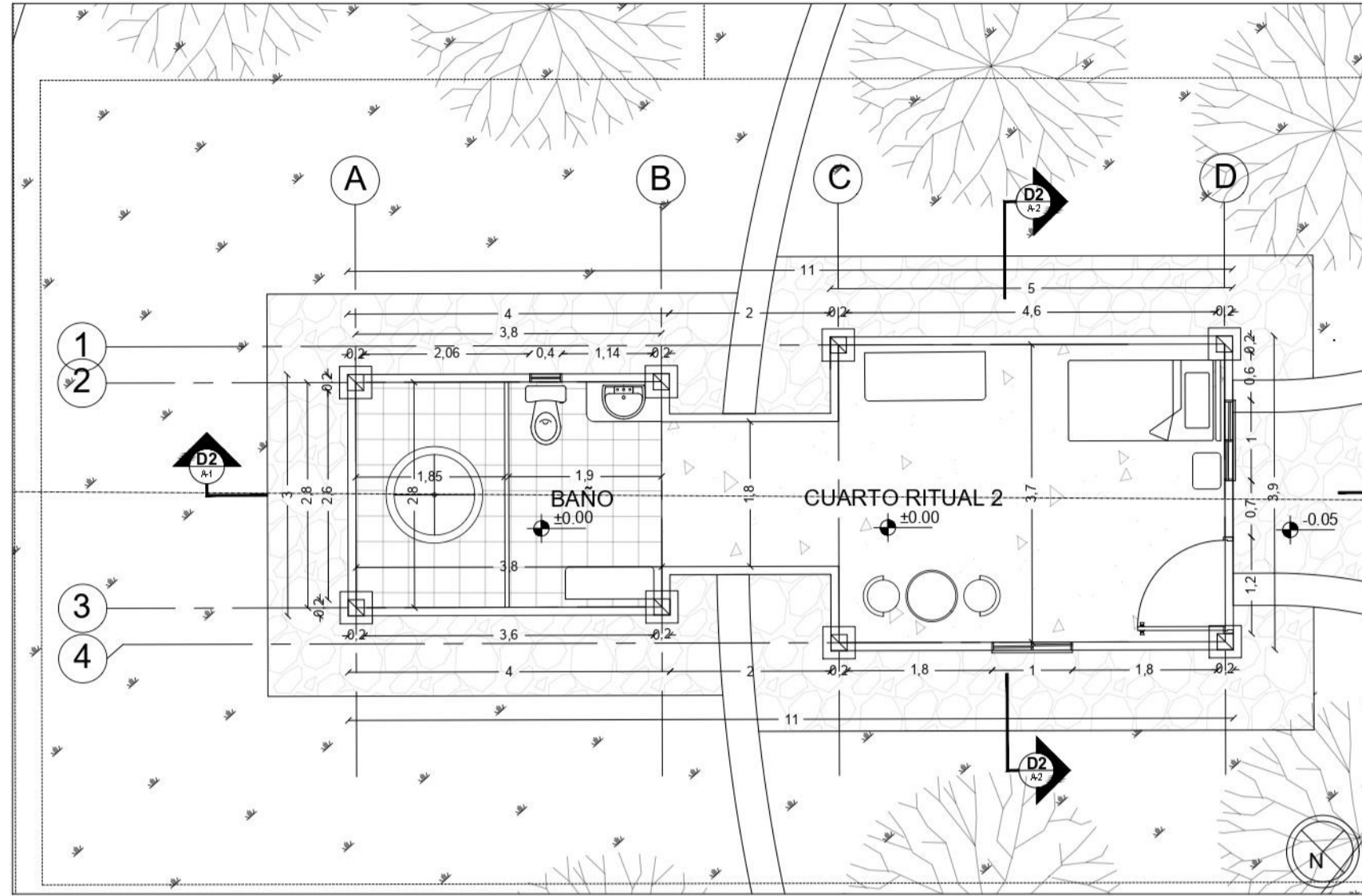
P1 PLANTA CLAUSTRO ESCALA 1:75
