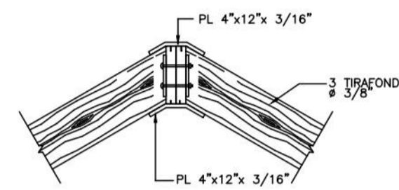
SECCION CABALLETE
