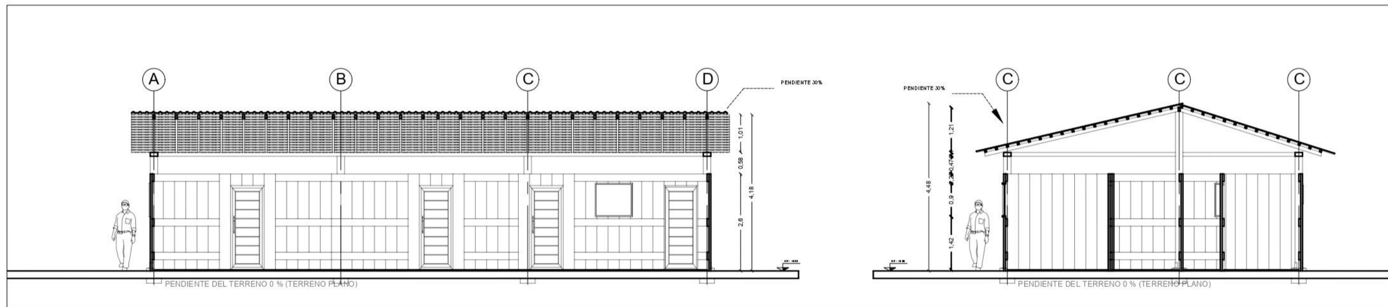
P6 CORTE LONGITUDINAL Y TRANSVERSAL ESCALA 1:100
