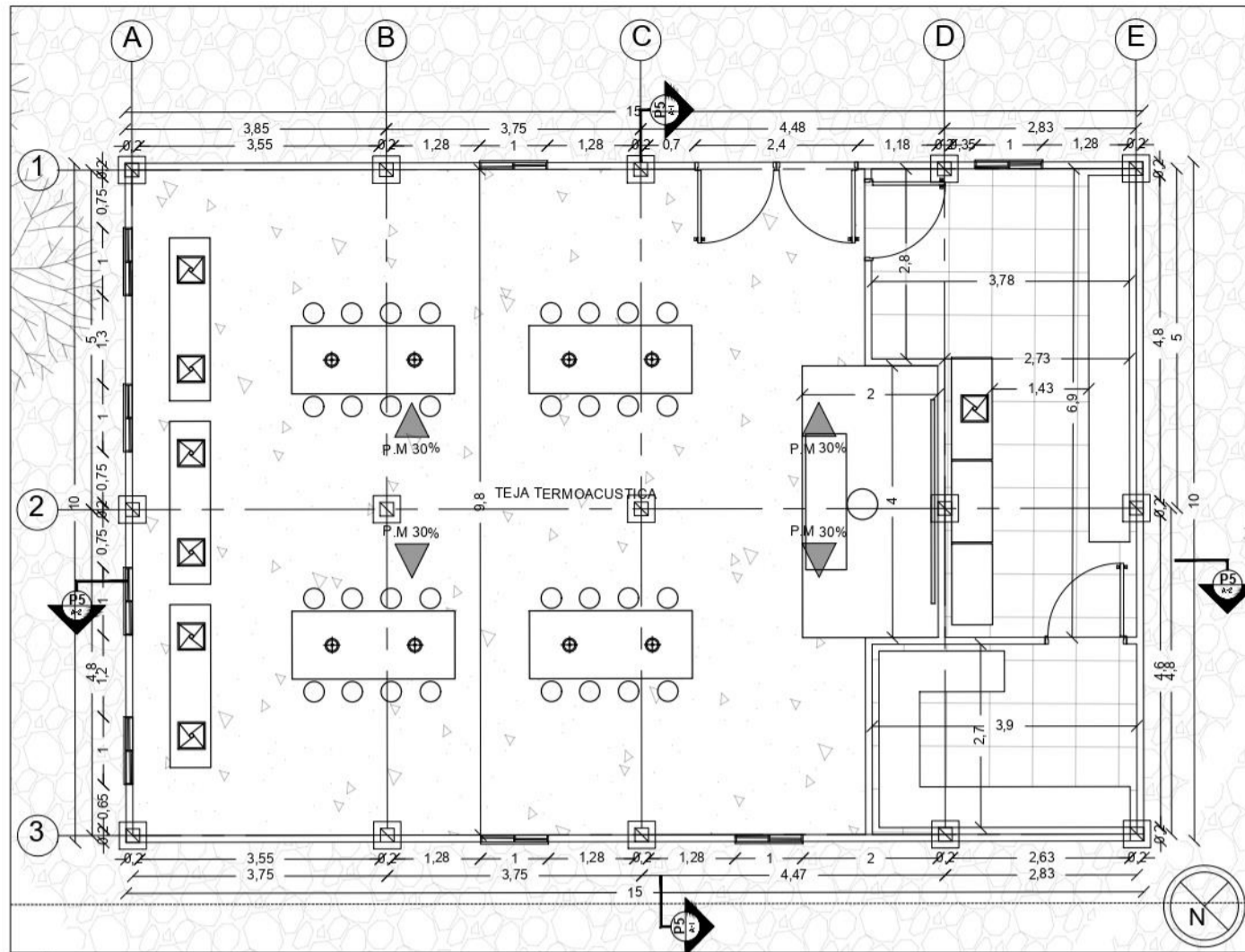
P5 PLANTA LABORATORIO ETNOEDUCATIVO ESCALA 1:100
