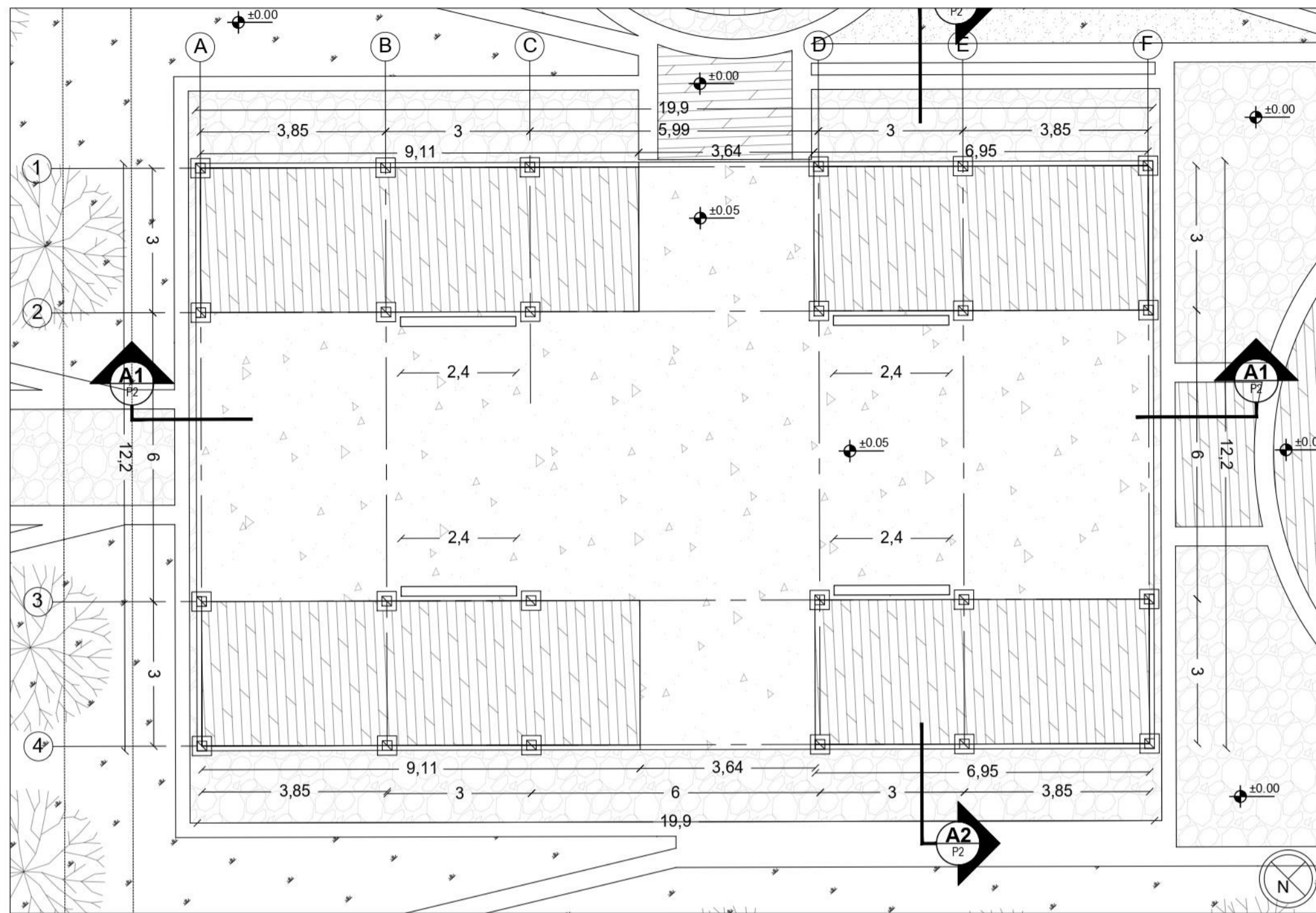
P2 MALOCA TICUNA ESCALA 1:100
