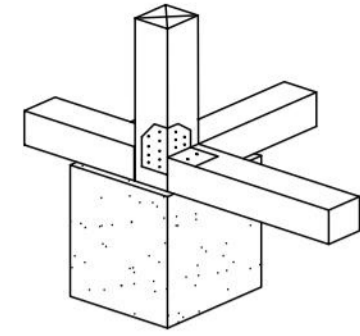
ANCLAJES TIPO ANGULO
