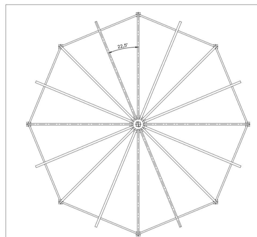
VISTA DE PLANTA NIVEL ±0.00
