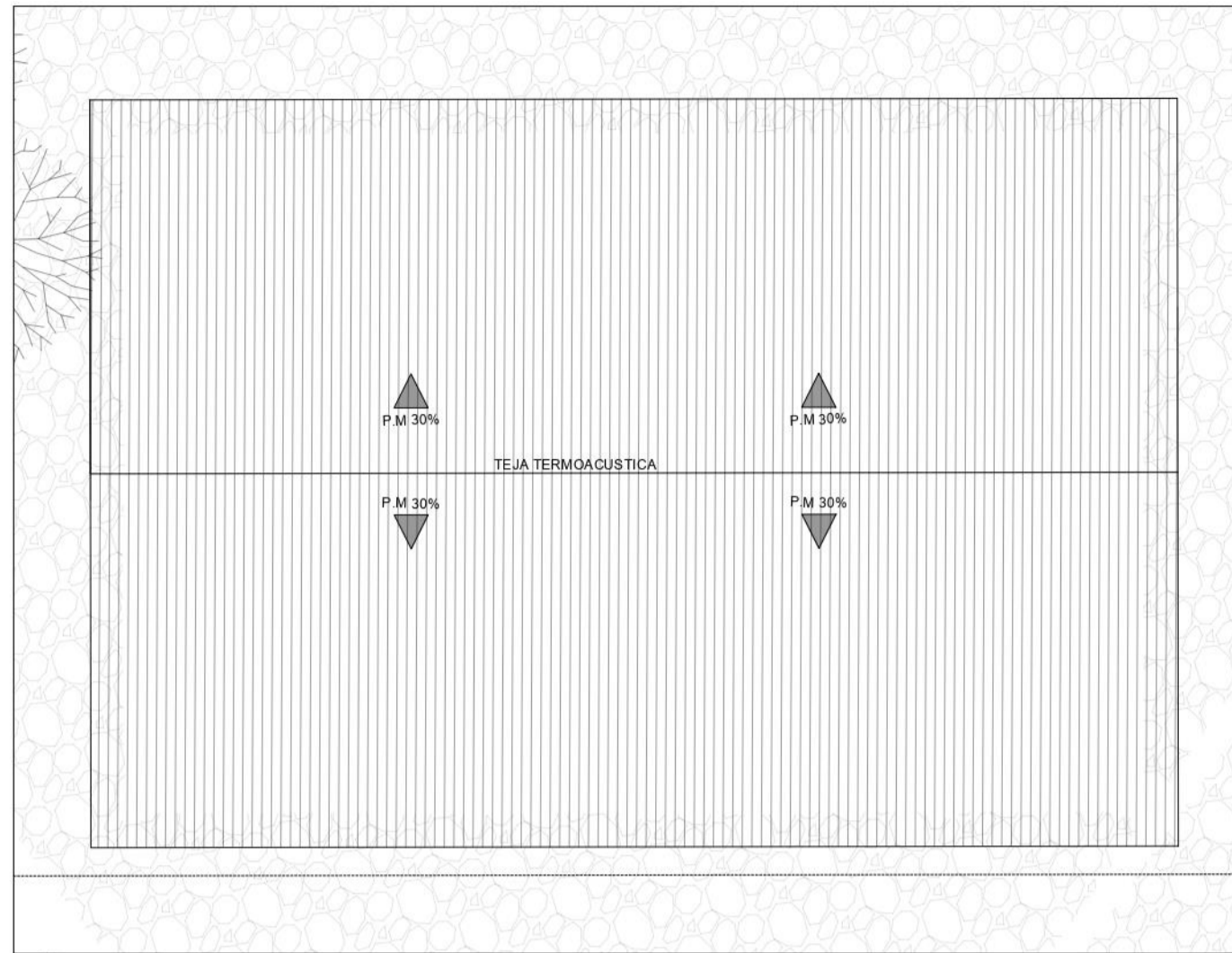
P5 PLANO CUBIERTA ESCALA 1:100
