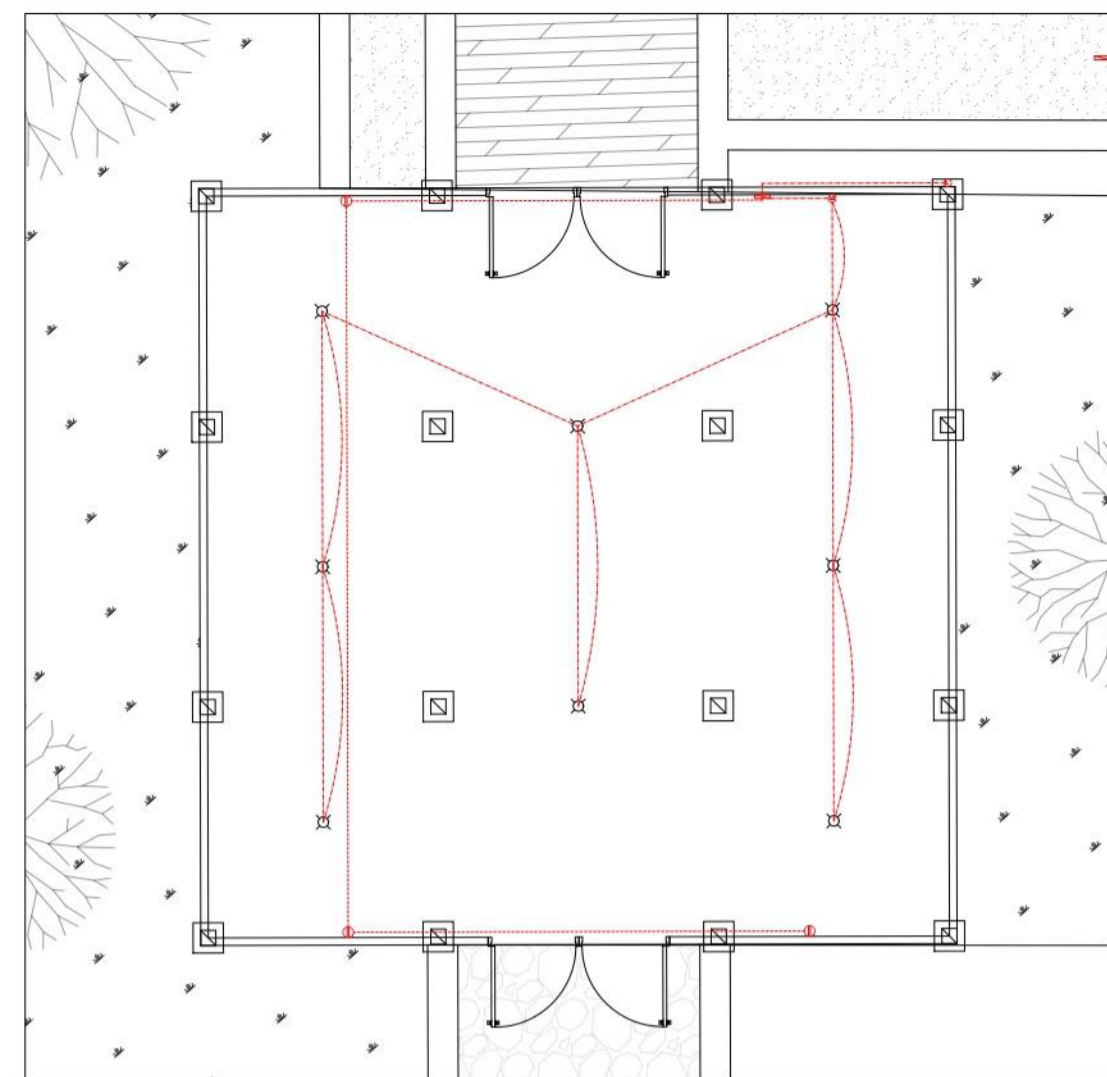
P8 INSTALACIONES ELECTRICAS ESCALA 1:100
