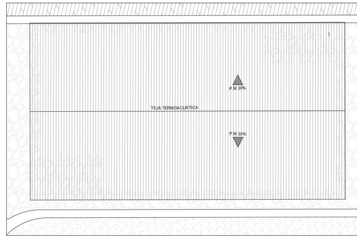
P6 CUBIERTAS AREA ADMINISTRATIVA COMPLEJO EDUCATIVO ESCALA 1:100
