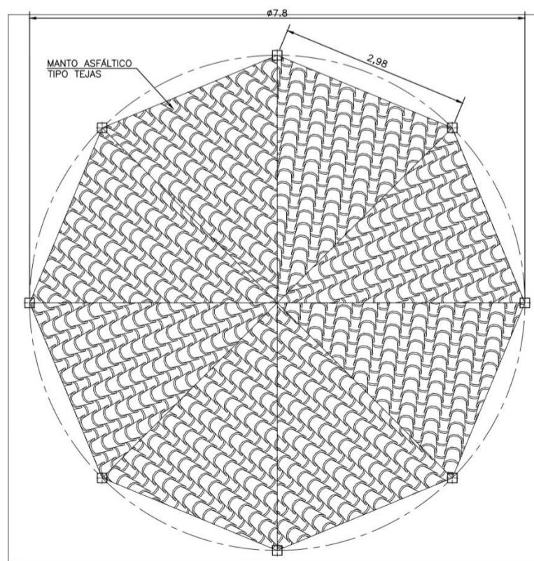
VISTA DE PLANTA TEOHO NIVEL ±4.18
