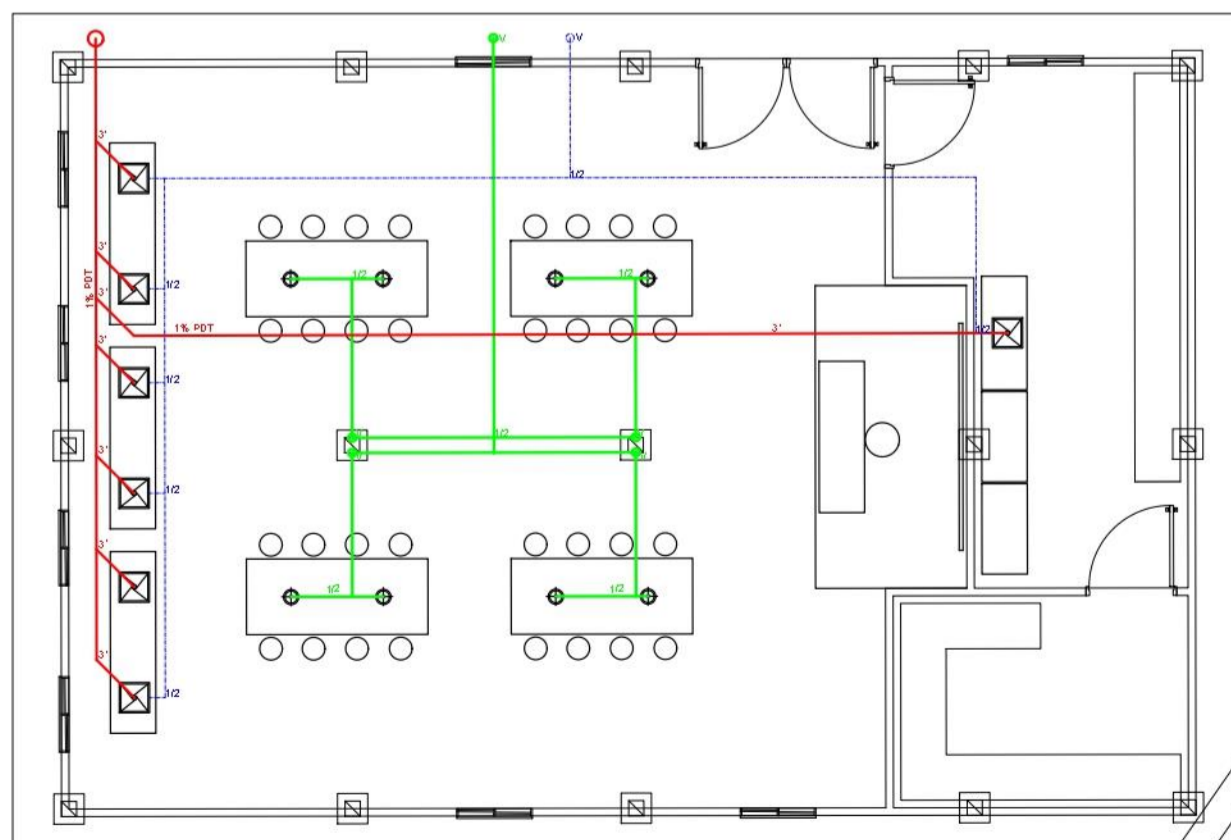
P5 INSTALACIONES HIDROSANITARIAS Y GAS ESCALA 1:100
