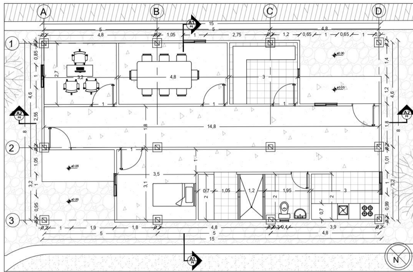
P6 PLANTA AREA ADMINISTRATIVA COMPLEJO EDUCATIVO ESCALA 1:100
