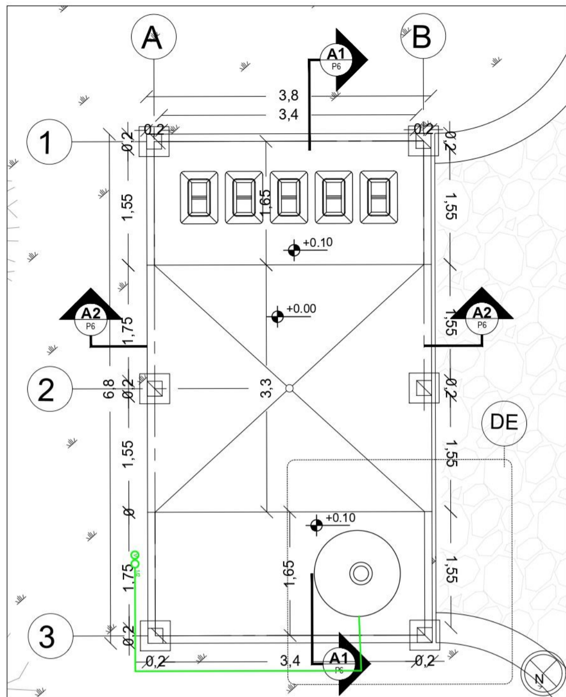
P7 PLANTA ZONA BASURAS Y BIODIGESTOR ESCALA 1:50
