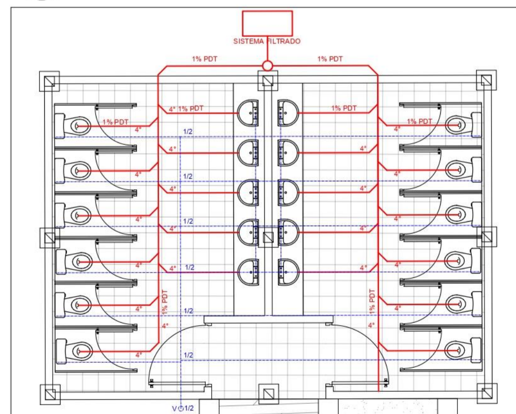
P3 INSTALACION HIDROSANITARIA ESCALA 1:75
