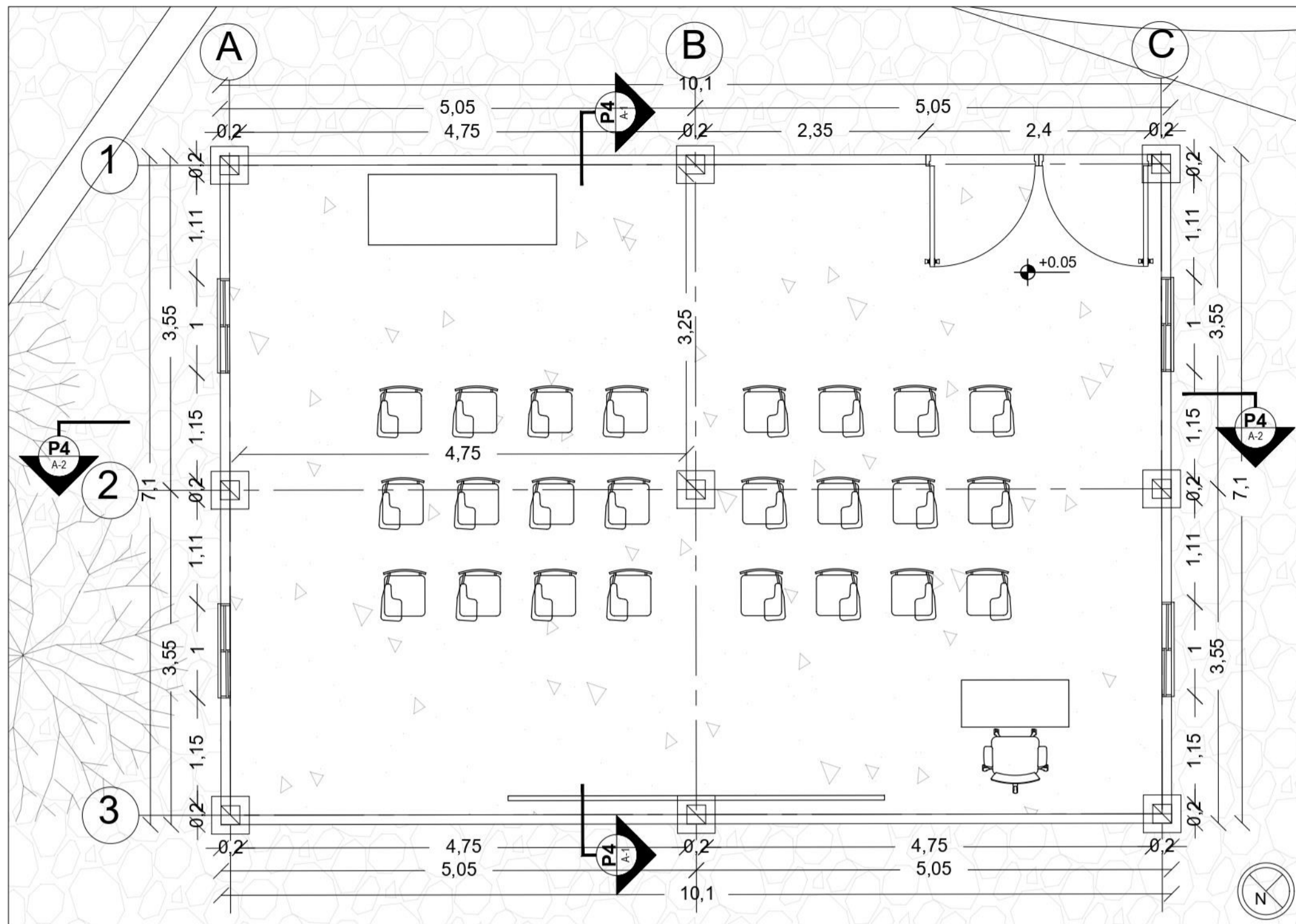
P4 PLANTA TIPO AULAS DE CLASE ESCALA 1:50
