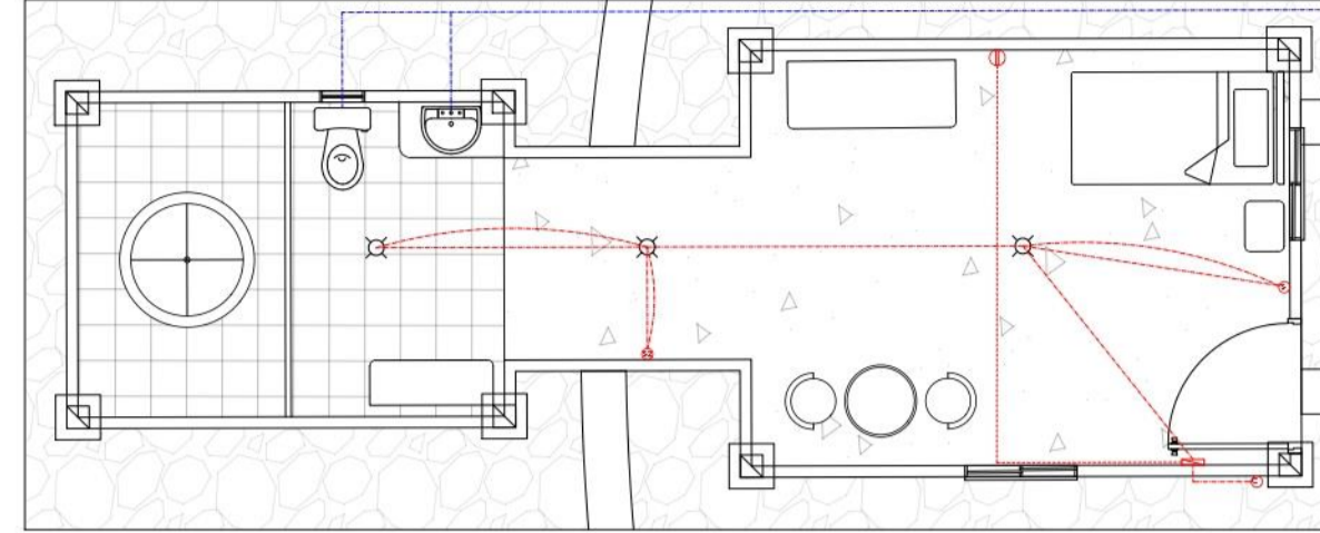
P1 INSTALACION ELECTRICA ESCALA 1:100
