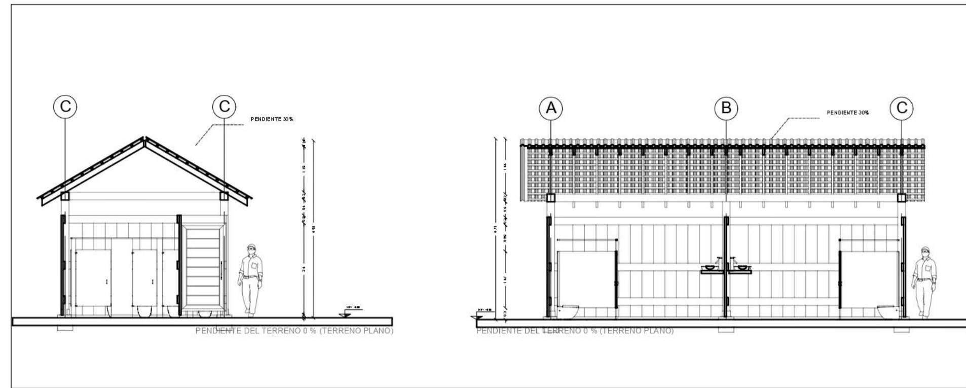
P3 CORTE TRANSVERSAL Y LONGITUDINAL ESCALA 1:100
