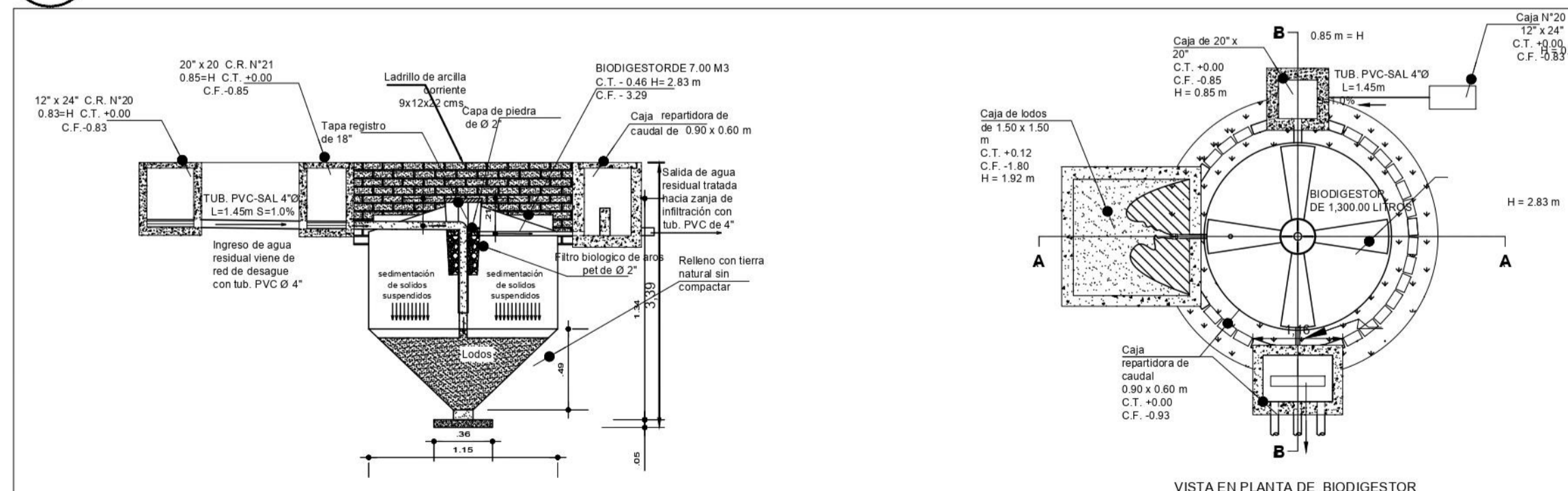
DE DETALLE ESPECIFICO BIODIGESTOR ESCALA 1:50
