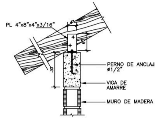
DETALLE ANCLAJES A MADERA
