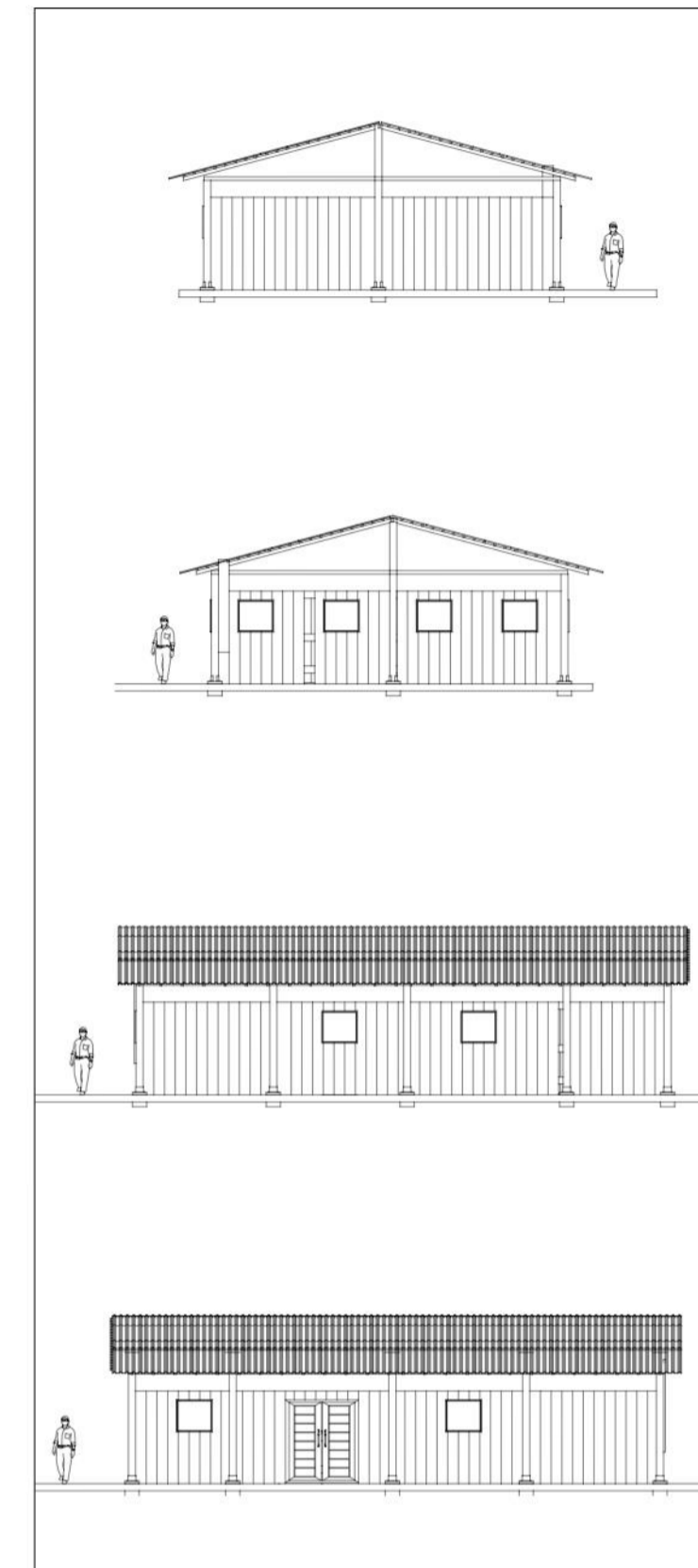
P5 FACHADAS IZQ - DER - TSR - FRT ESCALA 1:200
