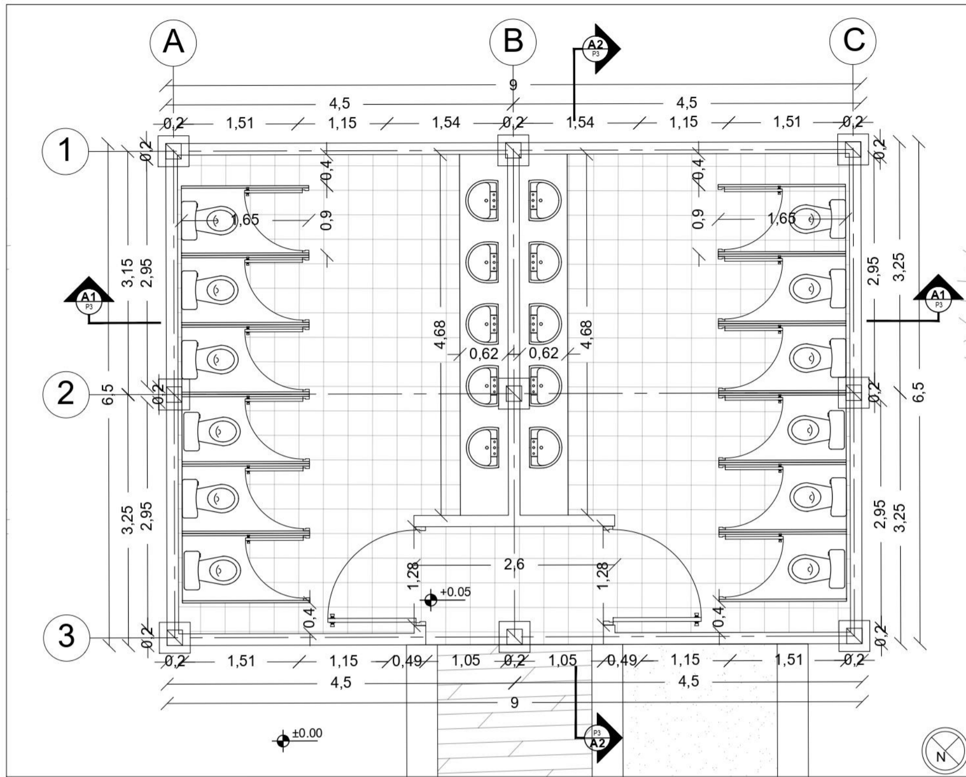
P3 BAÑO TIPO 1 ESCALA 1:50
