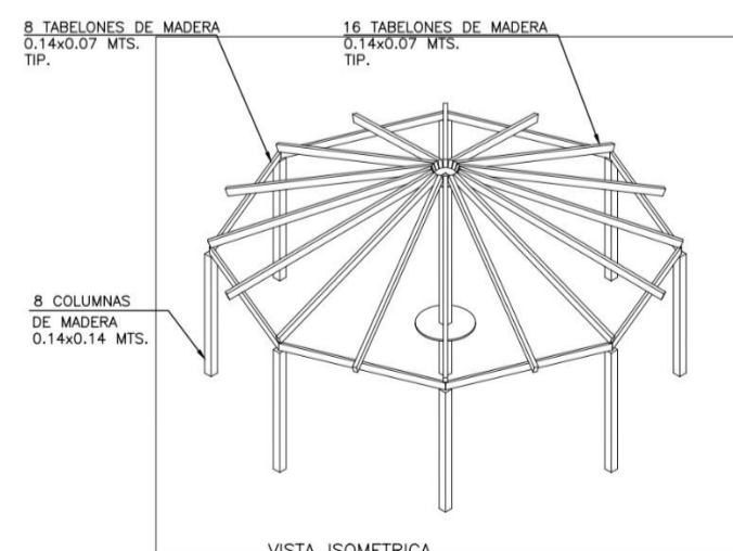
VISTA ISOMETRICA
