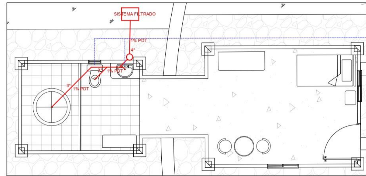
P1 INSTALACION HIDROSANITARIA ESCALA 1:100
