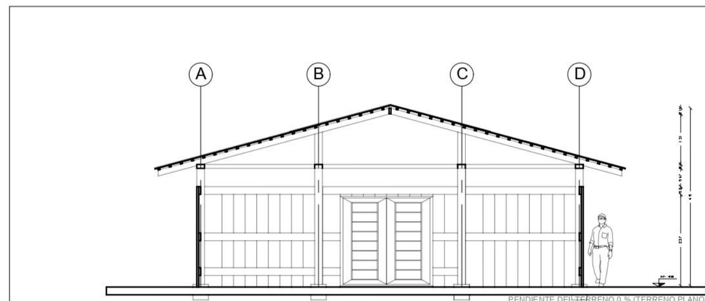
P1 CORTES TRANSVERSAL Y LONGITUDINAL ESCALA 1:100
