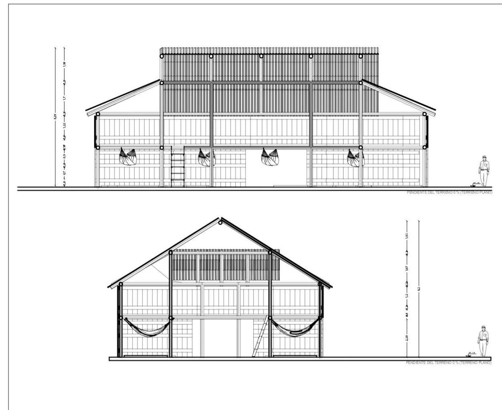
P2 CORTES TRANSVERSALES Y LONGITUDINALES ESCALA 1:100
