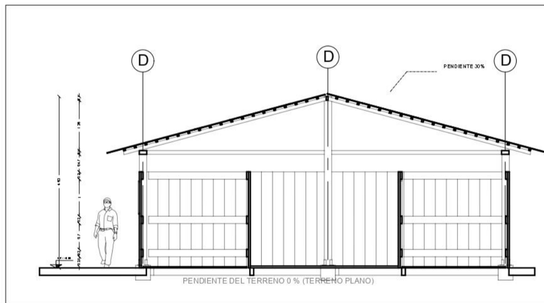
P5 CORTES TRANSVERSAL Y LONGITUDINAL ESCALA 1:100
