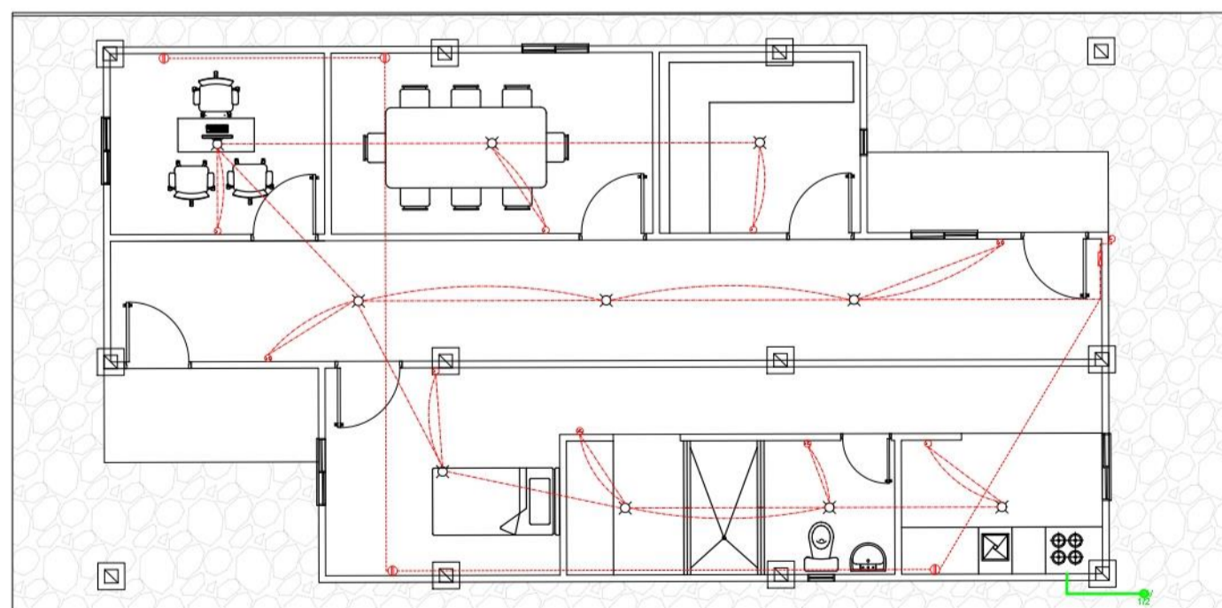
P6 INSTALACIONES ELECTRICAS ESCALA 1:100
