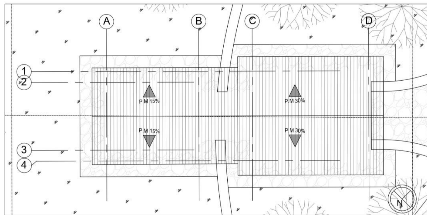
P1 PLANO CUBIERTA CLAUSTRO ESCALA 1:100
