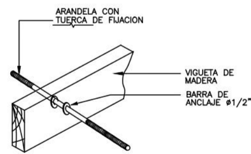
PERPECTIVA ESCALA 1:20
