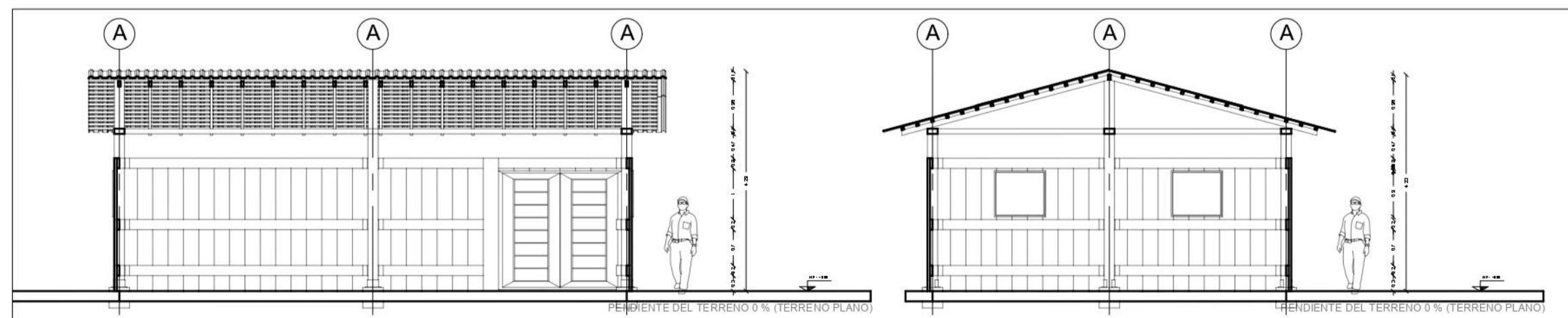
P4 CORTE TRANSVERSAL LONGITUDINAL ESCALA 1:100
