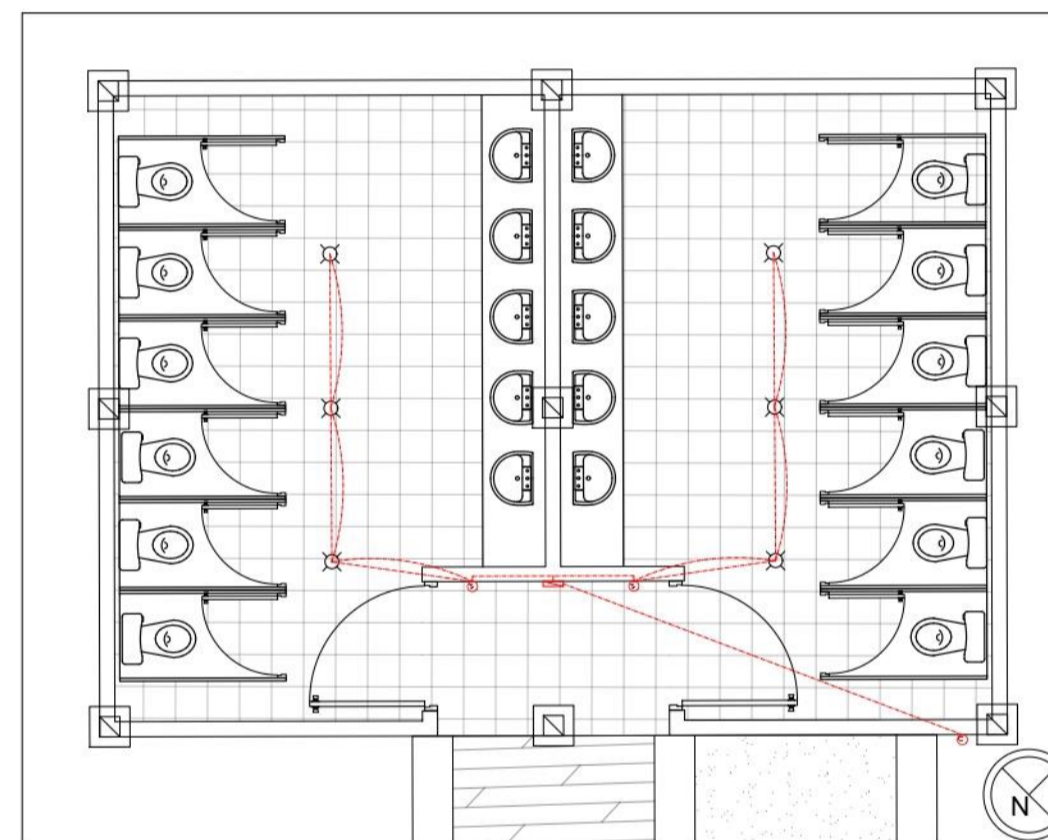
P3 INSTALACION ELECTRICA ESCALA 1:75
