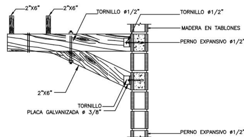
DETALLE 1 SV-3
