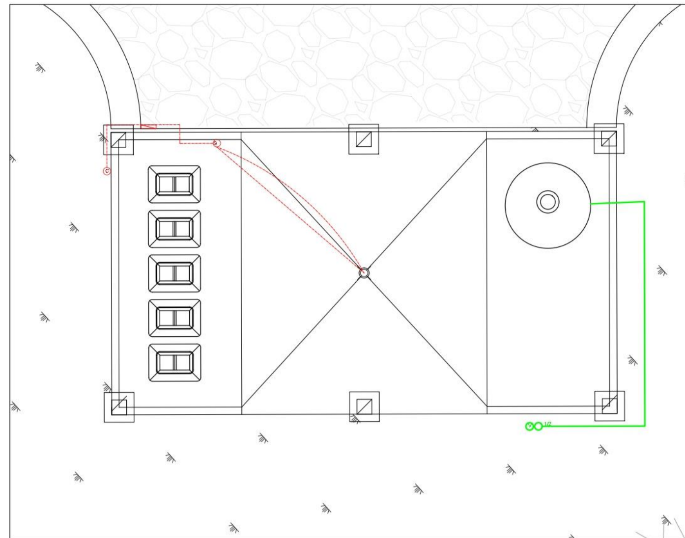
P7 INSTALACION ELECTRICA Y SALIDA DE GAS ESCALA 1:50
