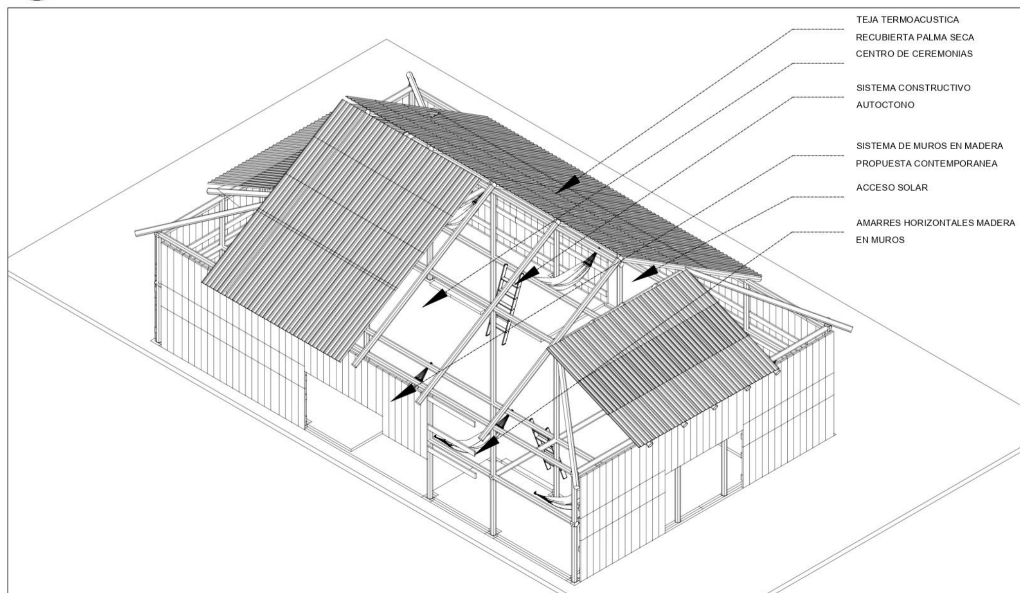
P2 AXONOMETRIA Y SISTEMA CONSTRUCTIVO MALOCA TICUNA ESCALA 1:100
