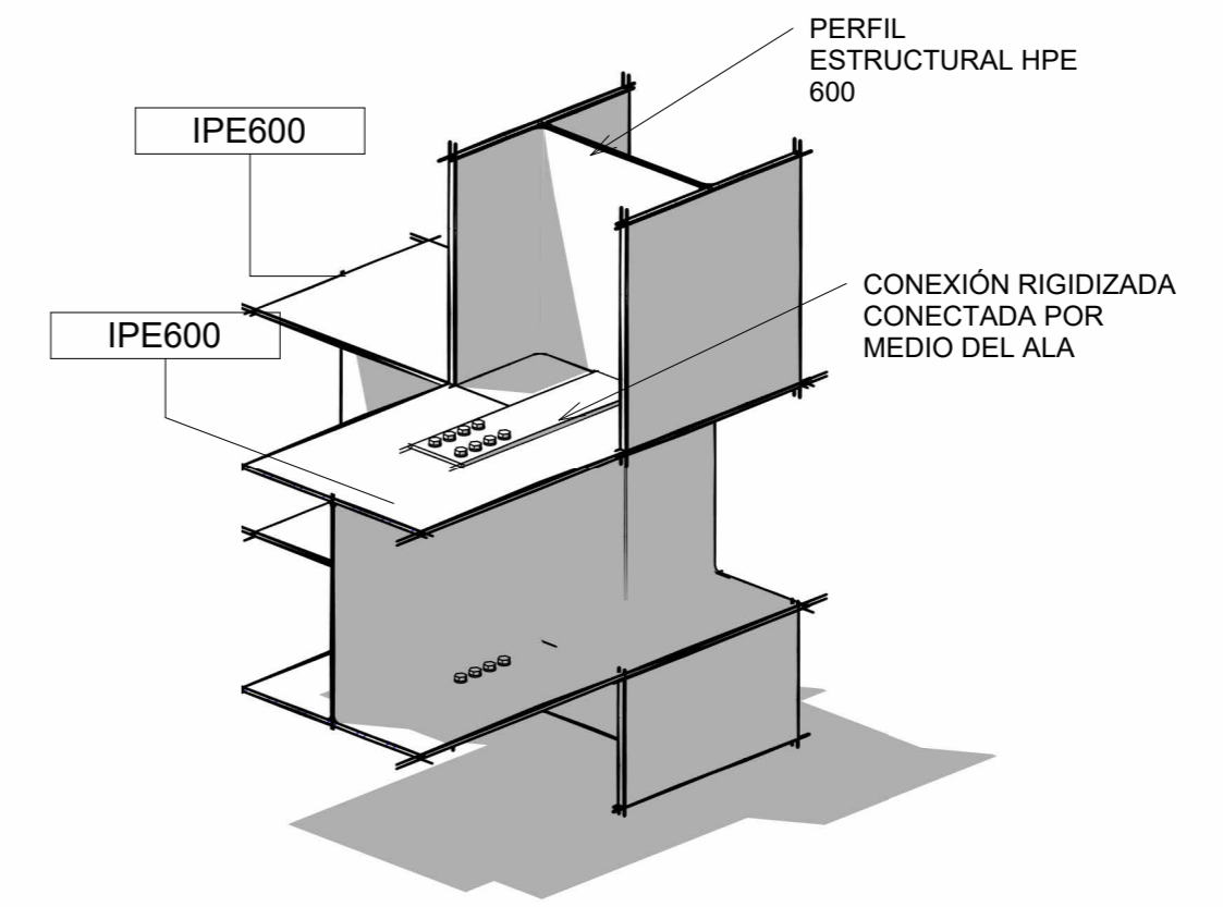
4 DETALLE CONEXIÓN VIGA VIERENDEEL A115
