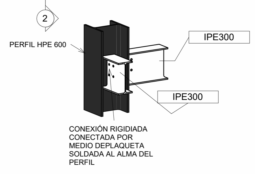
3 DETALLE CONEXIÓN A115
