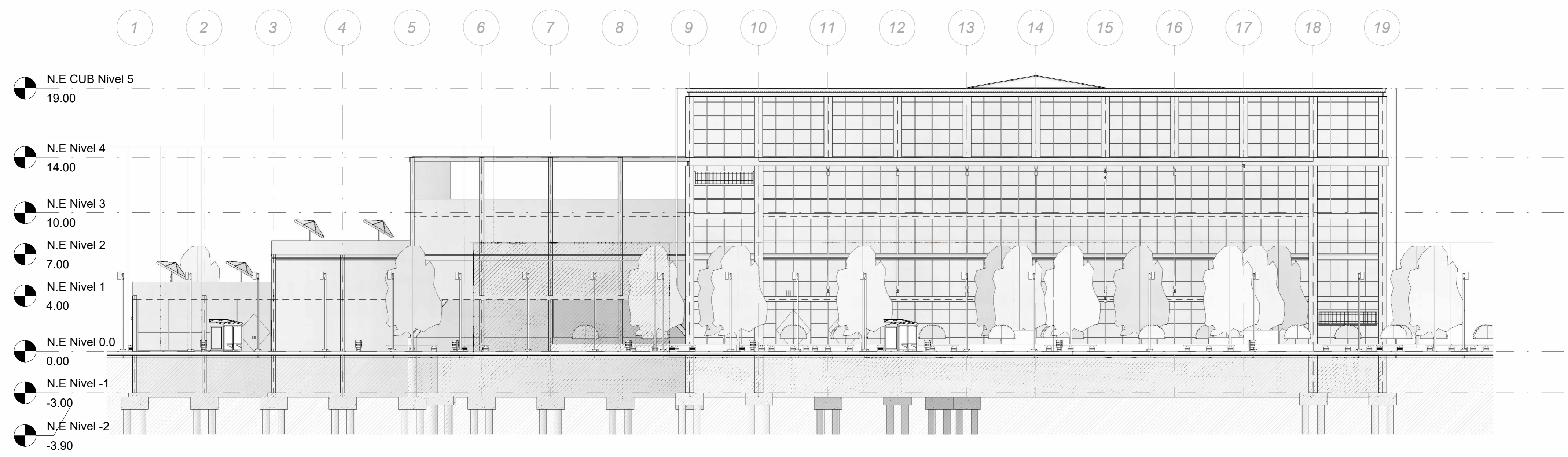
1 FACHADA PRINCIPAL 1 : 200
