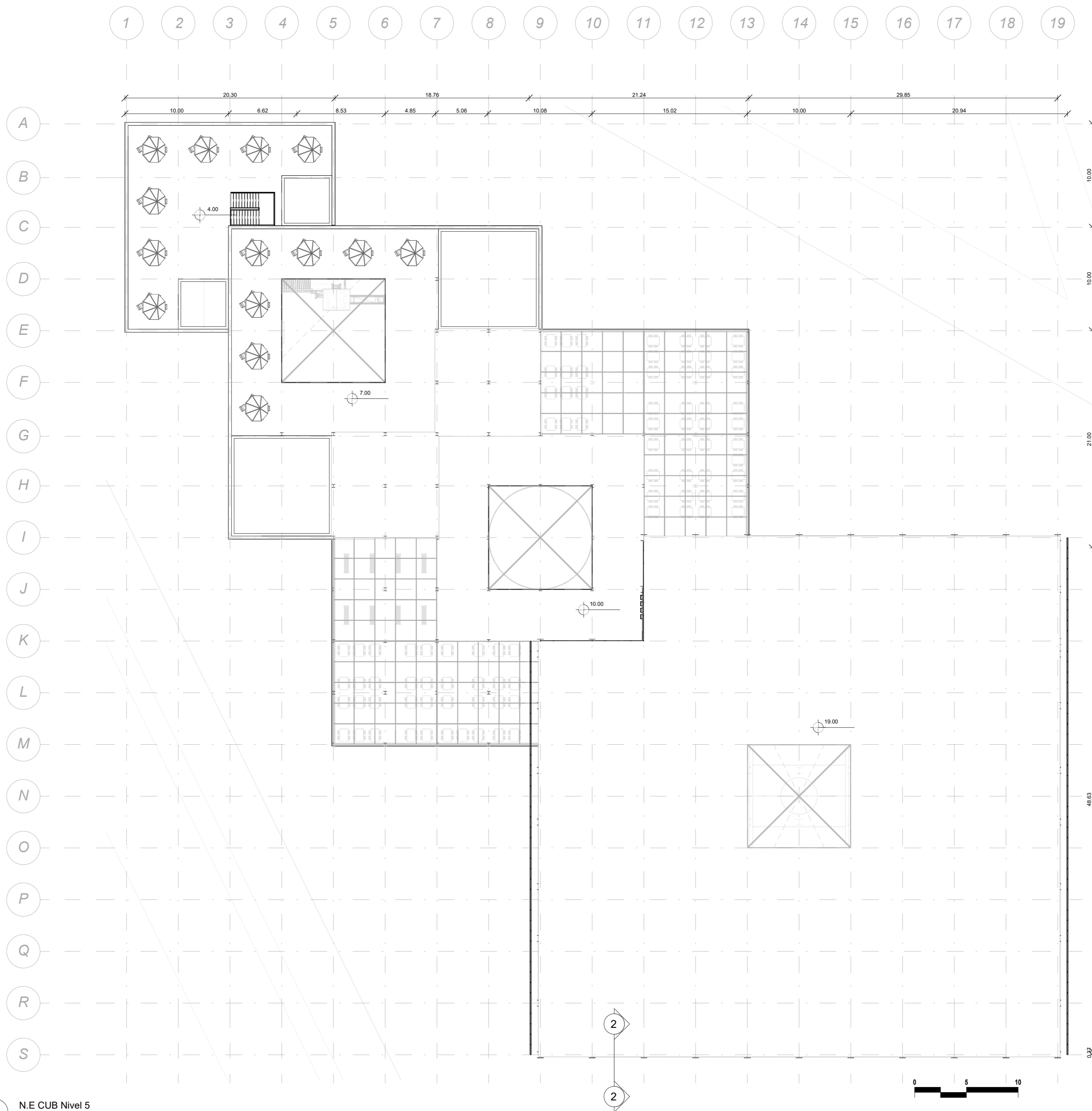
1 N.E CUB Nivel 5 A108 1 : 250
