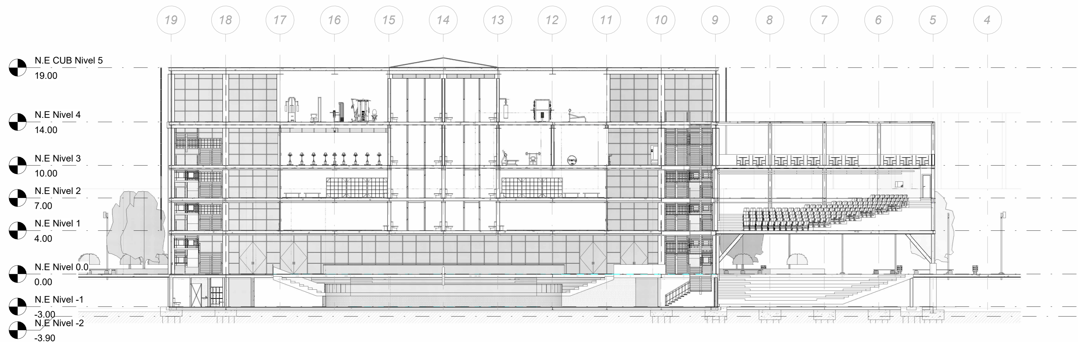
2 CORTE TRANSVERSAL A109 1:200
