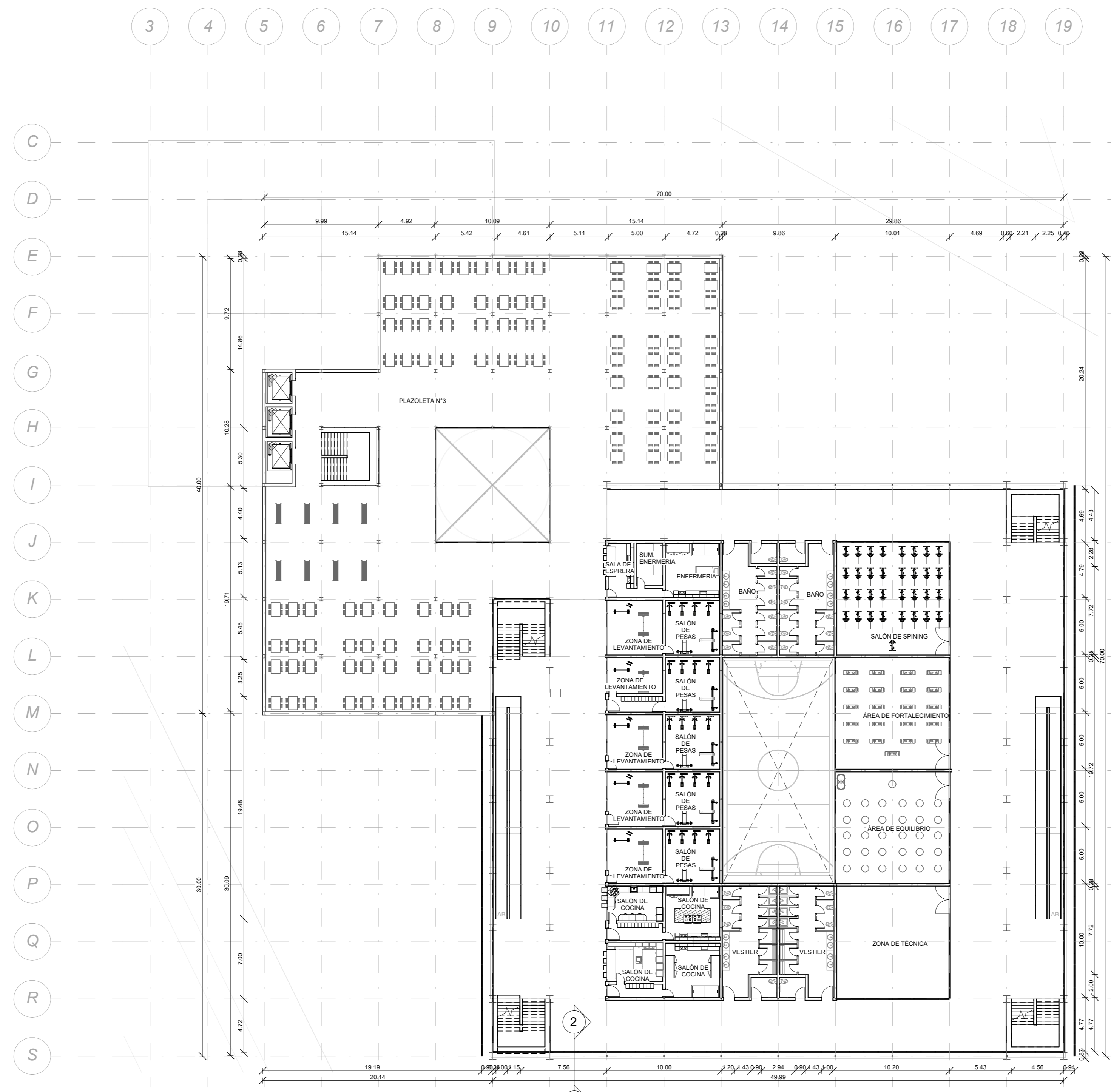
1 N.E Nivel 3 A106 1: 250
