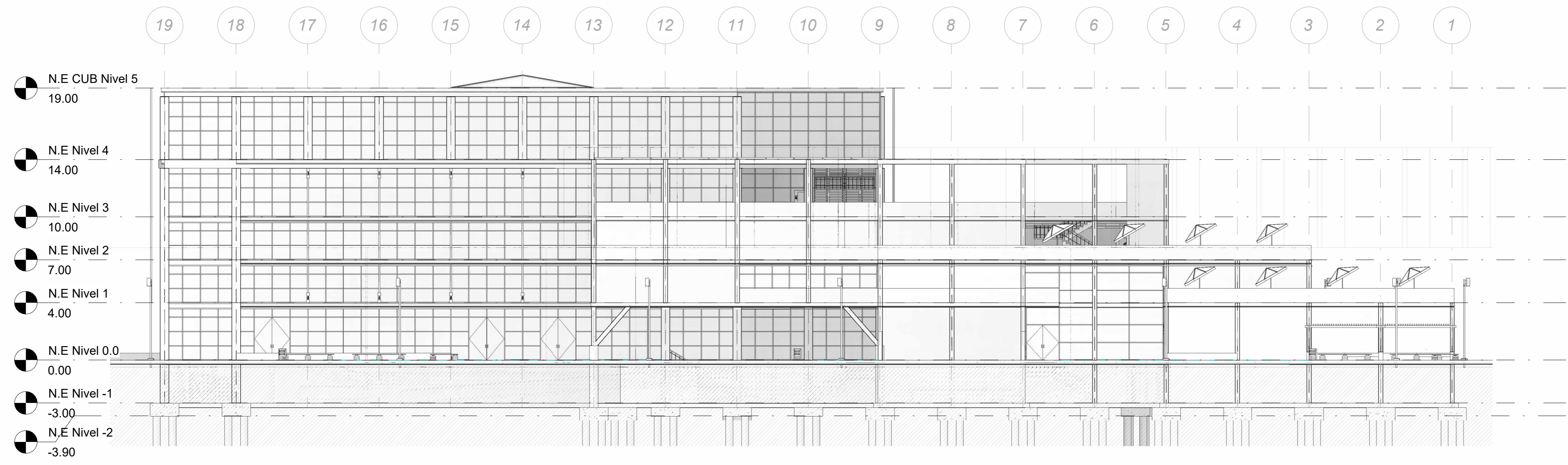
2 FACHADA POSTERIOR 1 : 200
