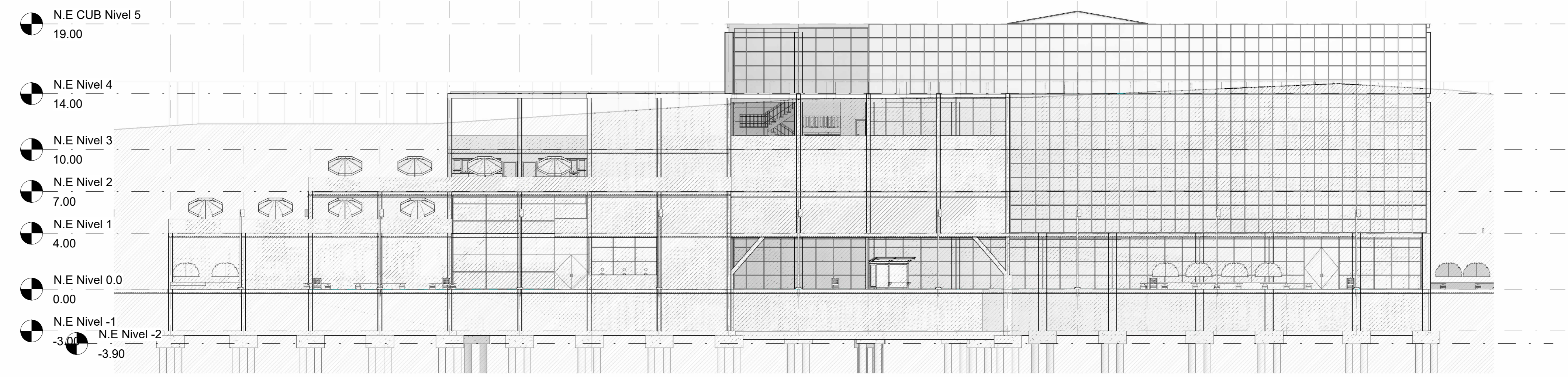
2 A118 FACHADA LATERAL IZQUIERDA 1:200
