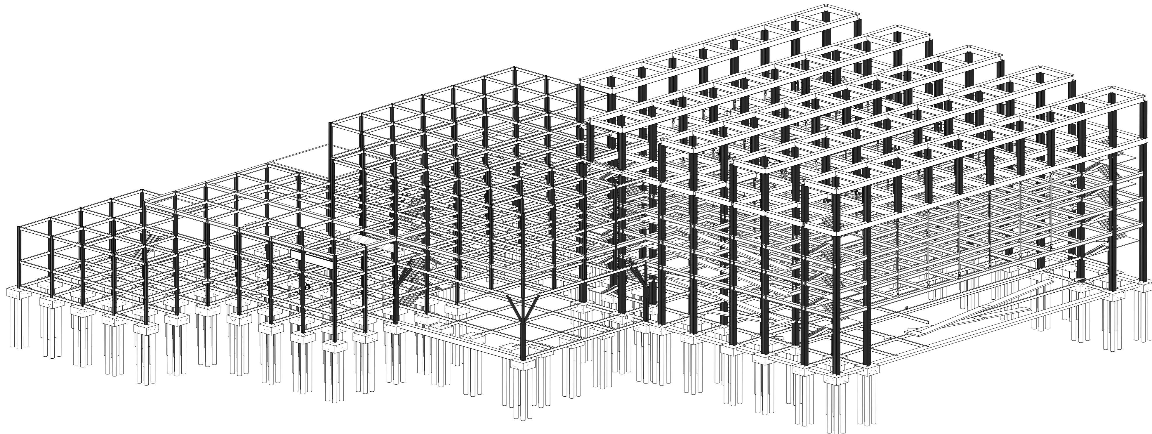
1 A119 ISOMETRIA - ESTRUCTURA
