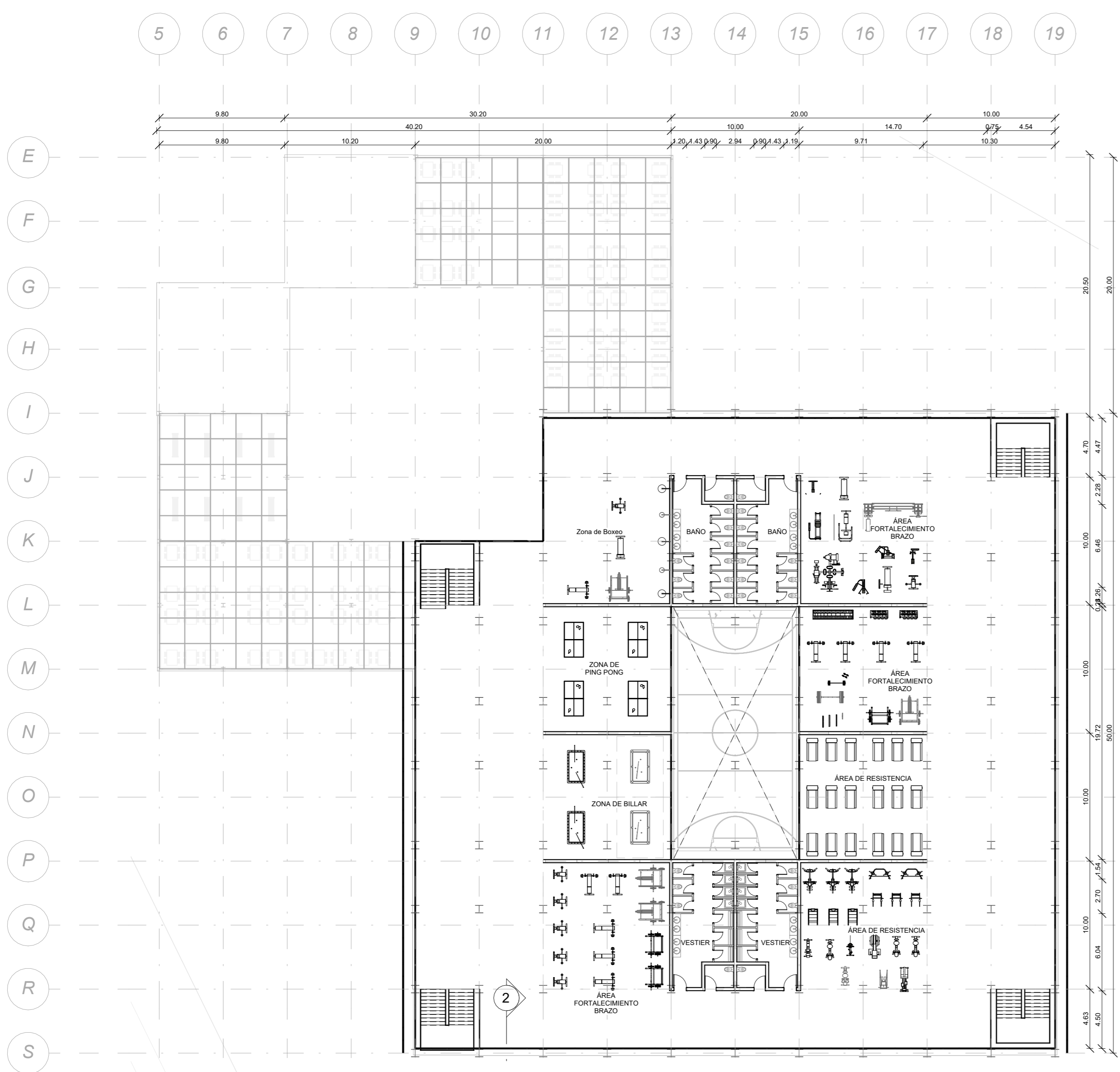
1 N.E Nivel 4 A107 1:250
