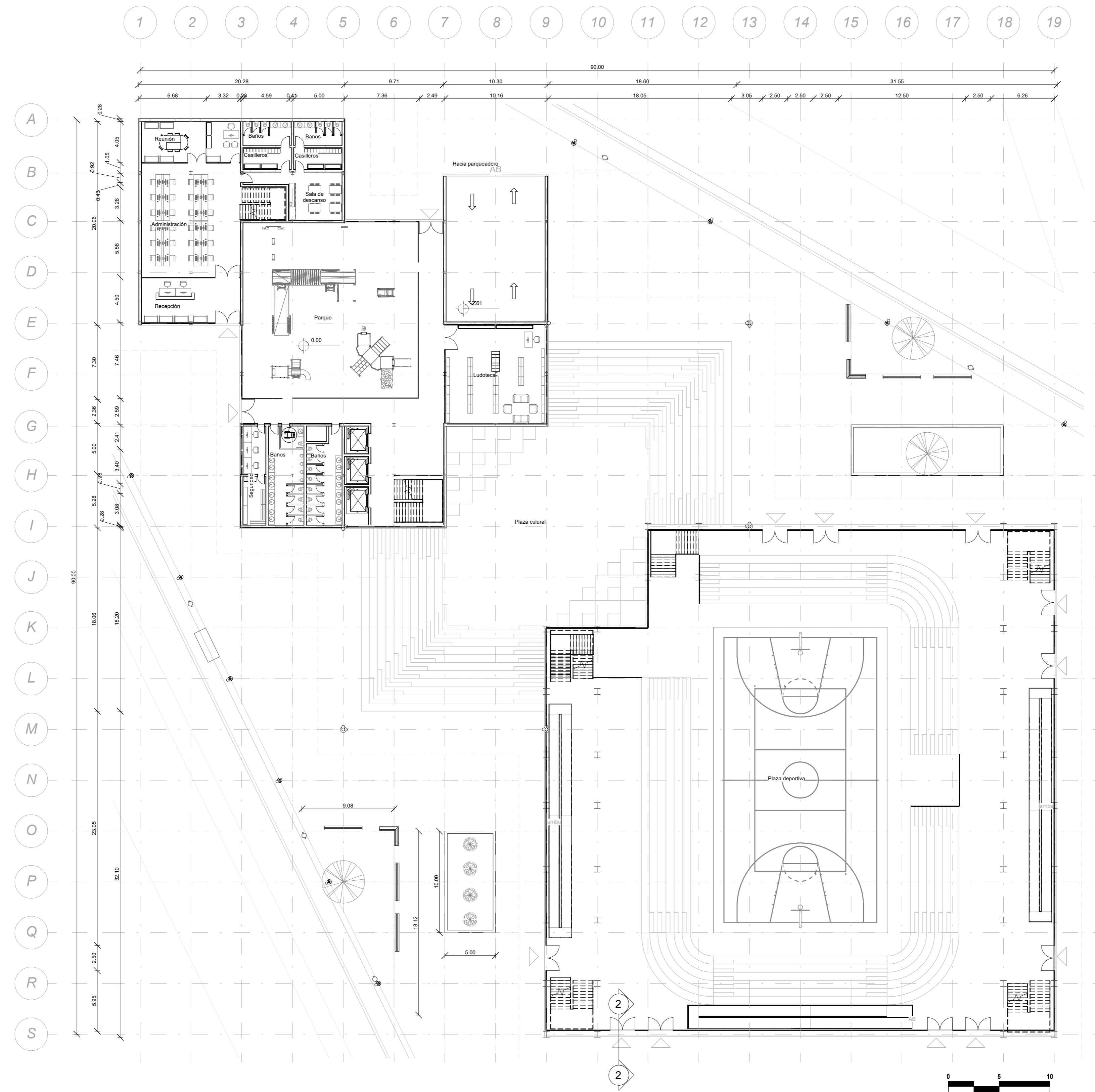
1 N.E Nivel 0.0. A103 1 : 250
