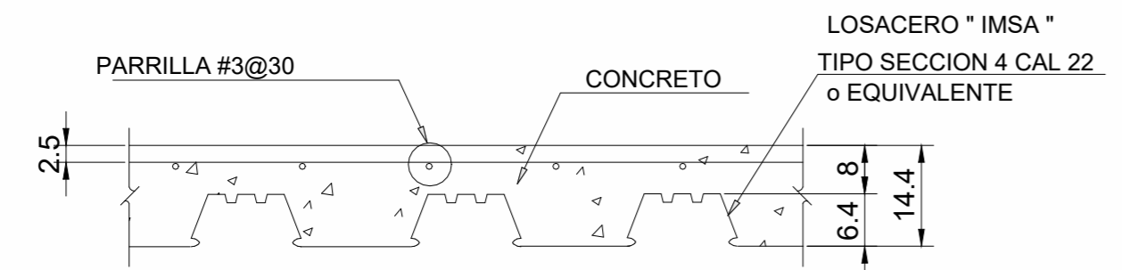
DETALLE ENTREPISO 1:150
