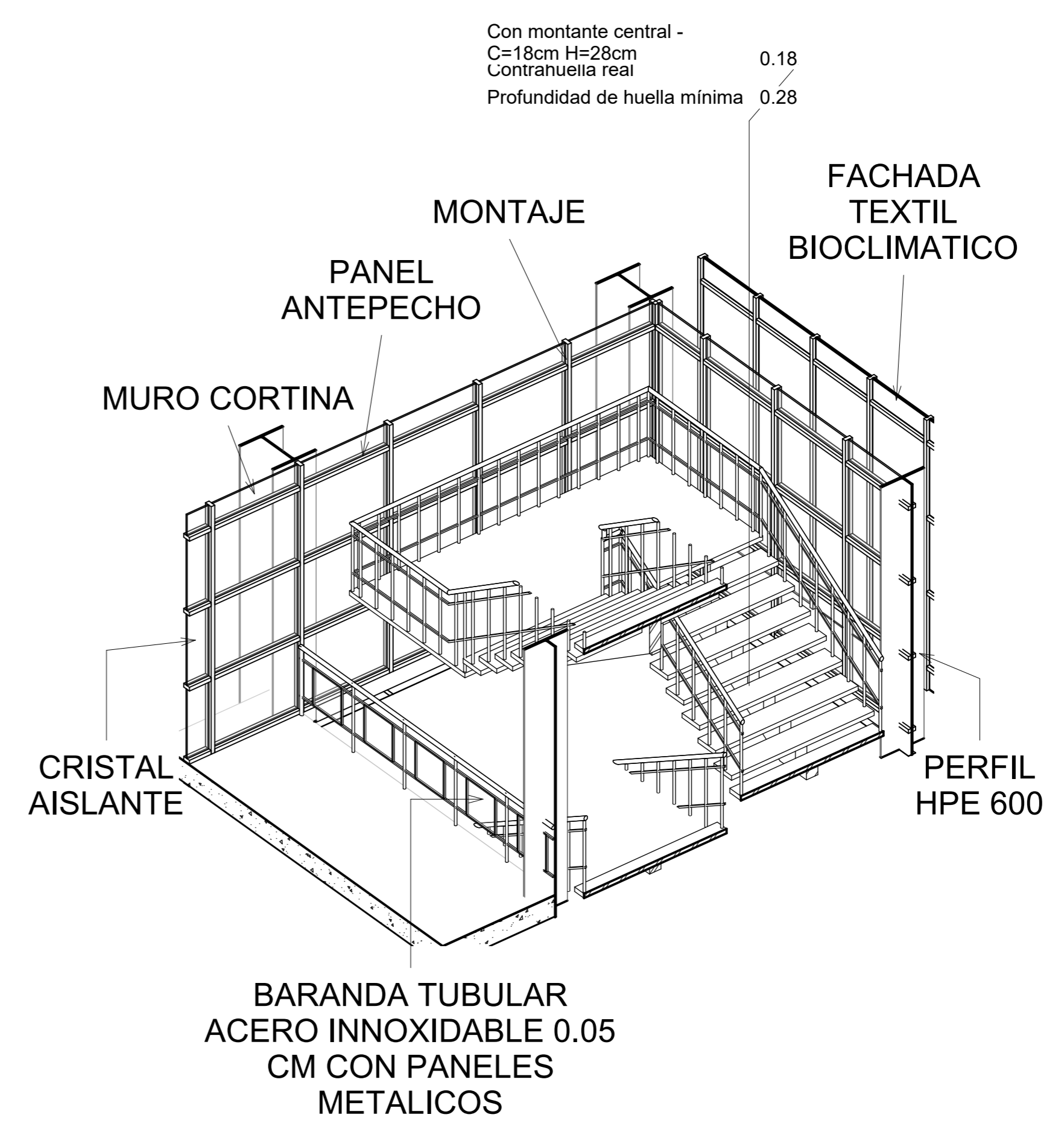
2 DETALLE ESCALERA A107
