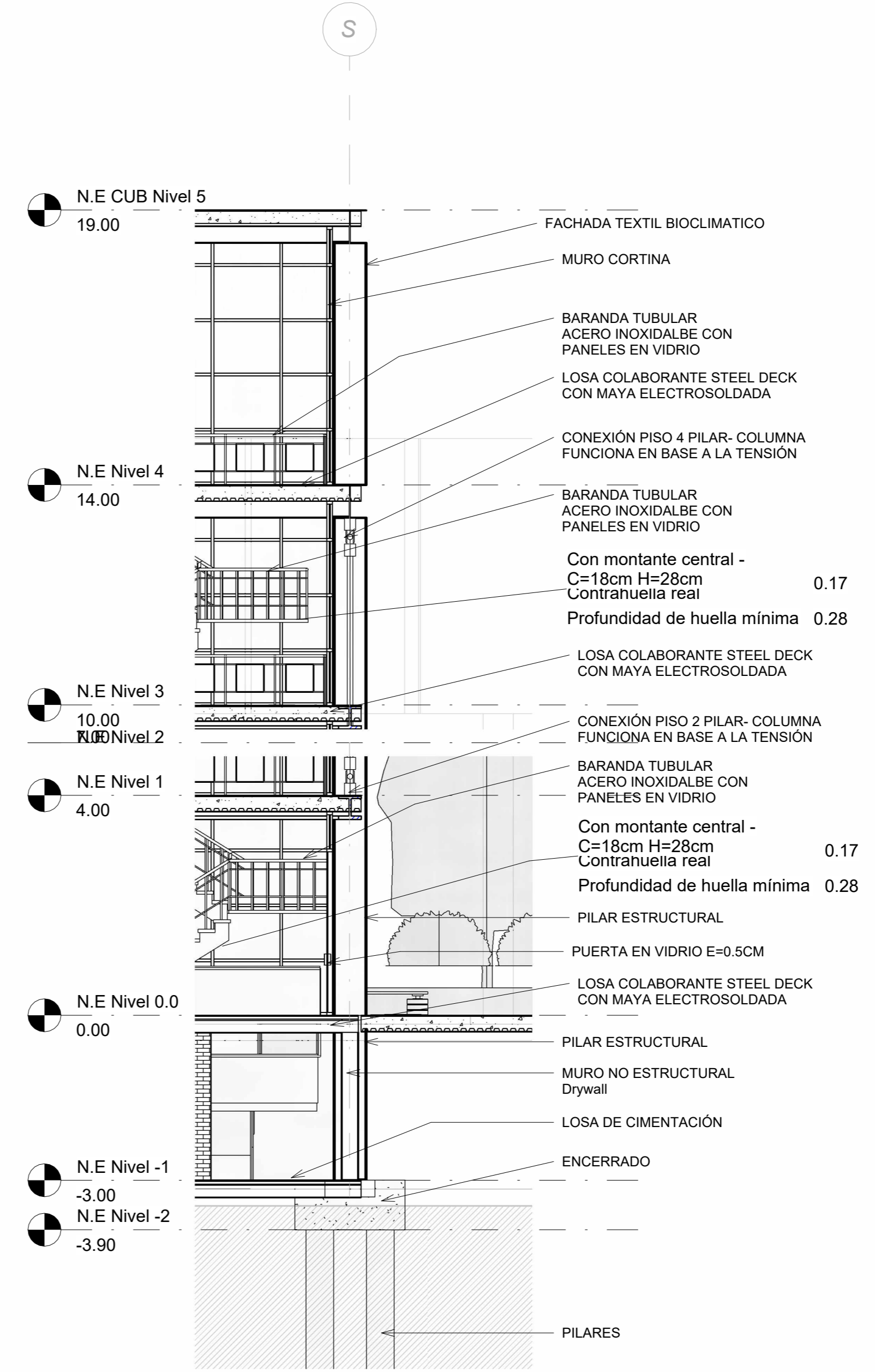
2 CORTE FACHADA A116 1:75
