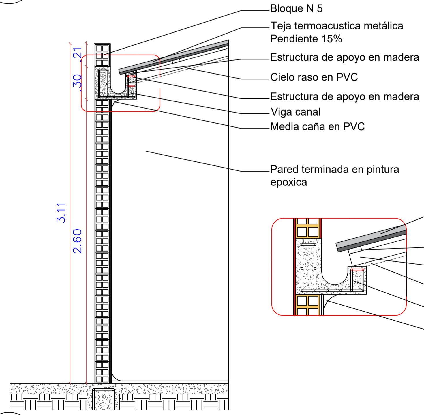
P17 DETALLE ZONA DE PRODUCCIÓN ESCALA: 1:20
