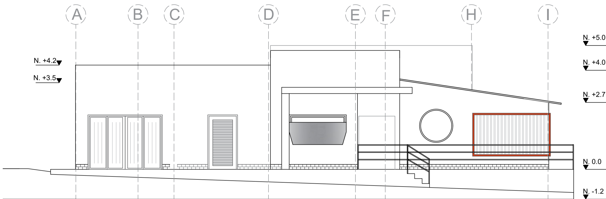
P8 FACHADA ORIENTAL ESCALA: 1:75
