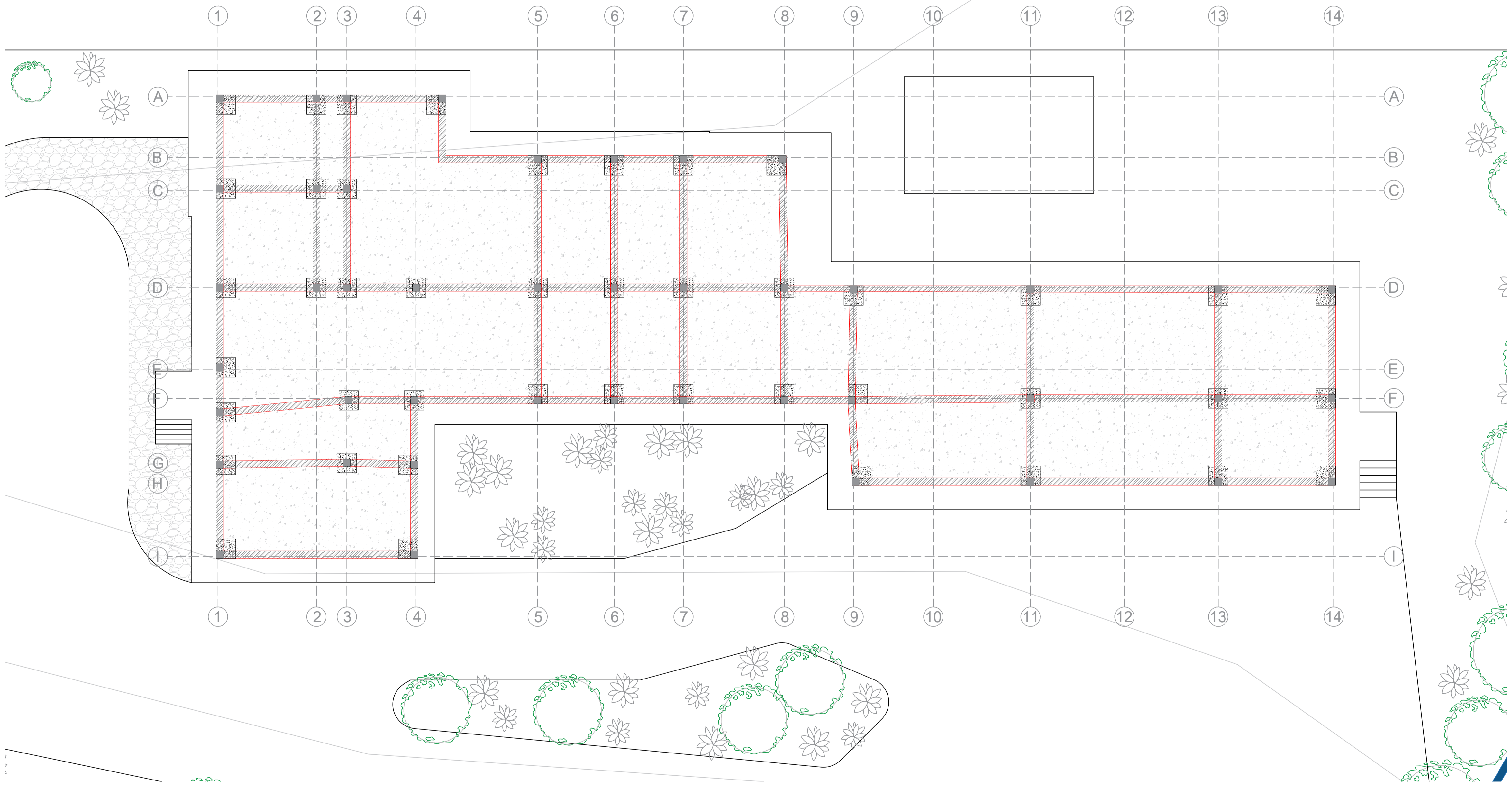
P29 PLANO DE CIMENTACIÓN ESCALA: 1:100
