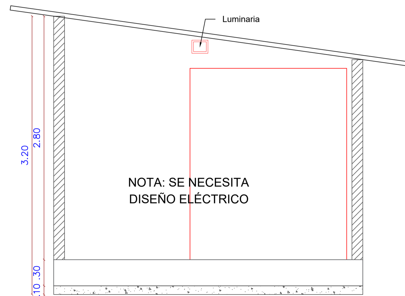
P6 CORTE A-A SUBESTACIÓN ELÉCTRICA ESCALA: 1:25
