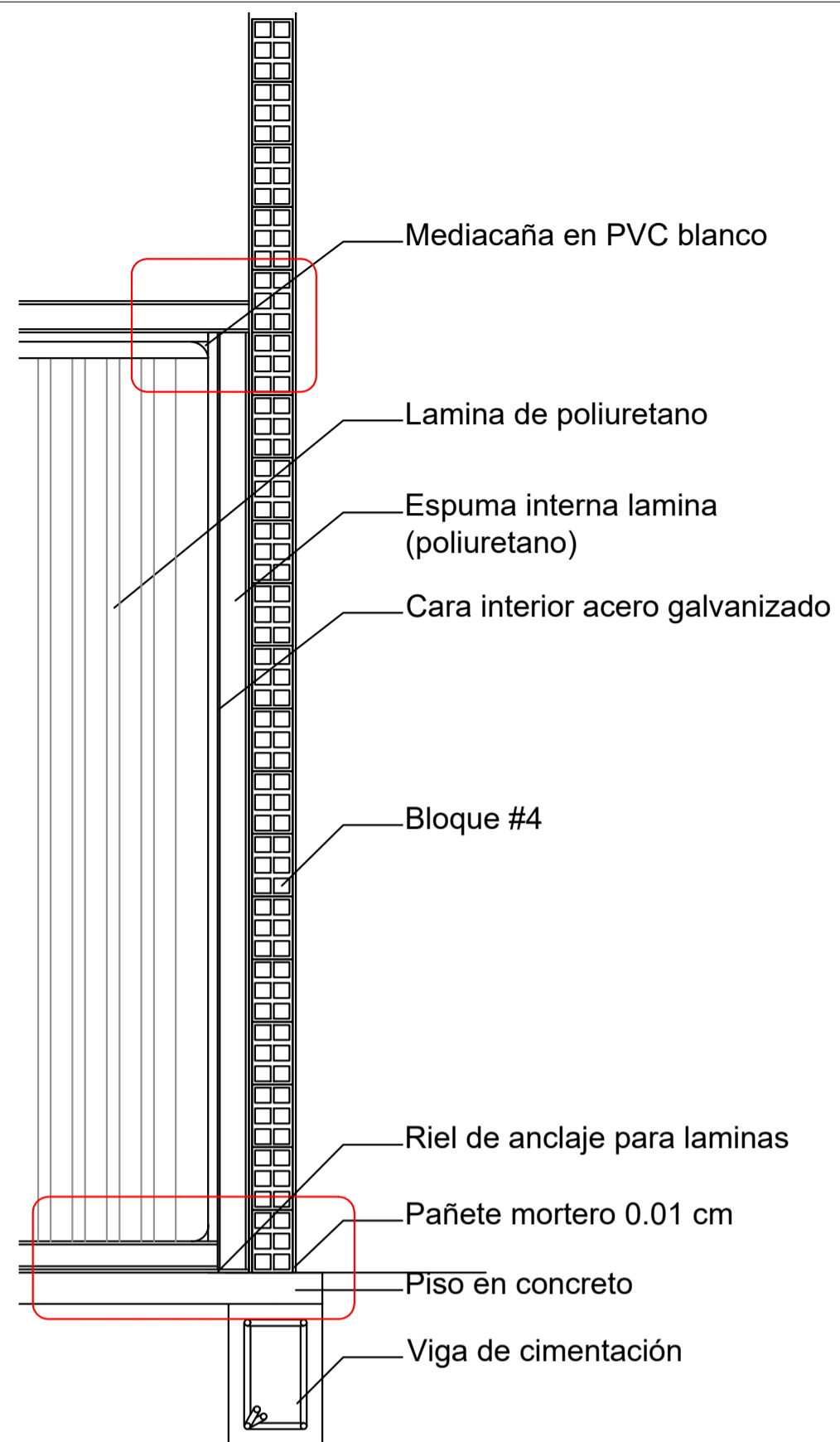
P16 DETALLE CUARTO FRIO - POLIURETANO ESCALA: 1:20
