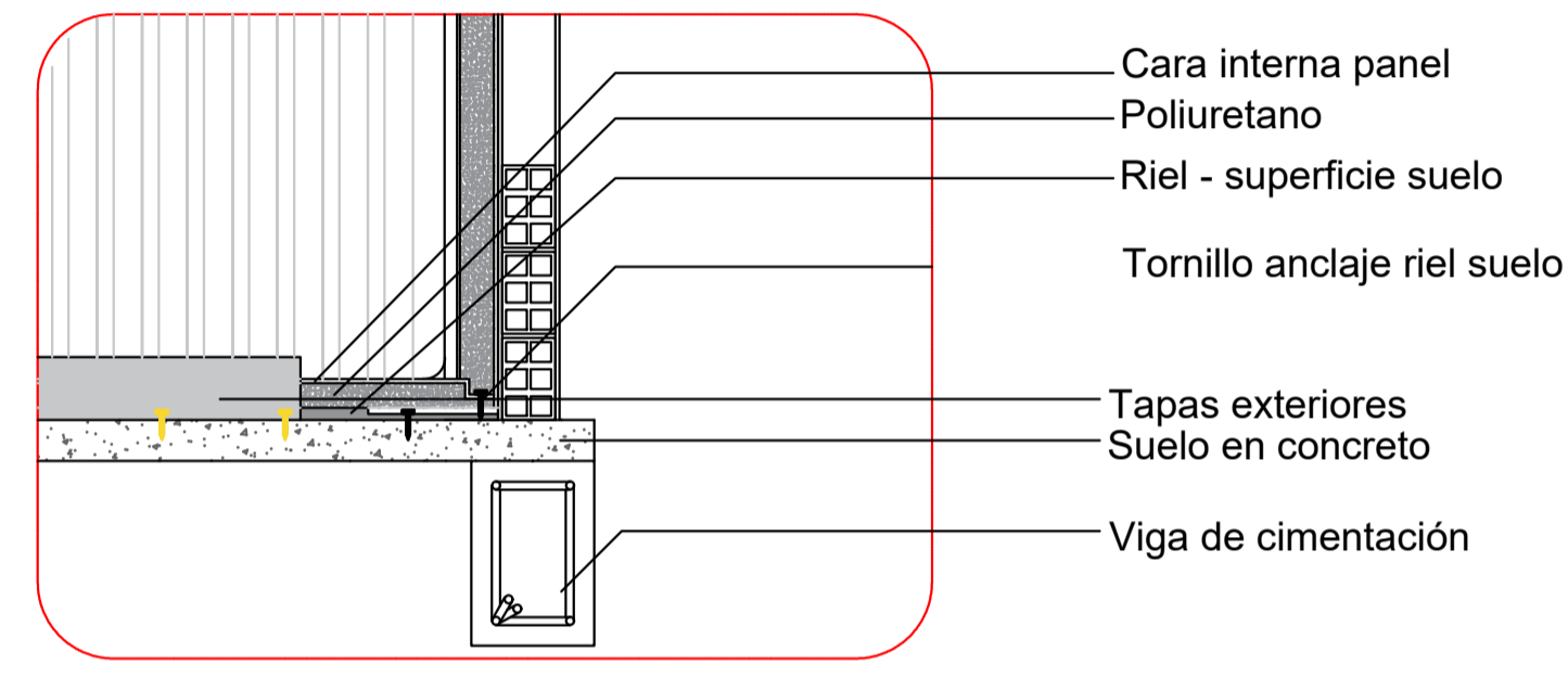
P16 DETALLE CUARTO FRIO - POLIURETANO ESCALA: 1:20
