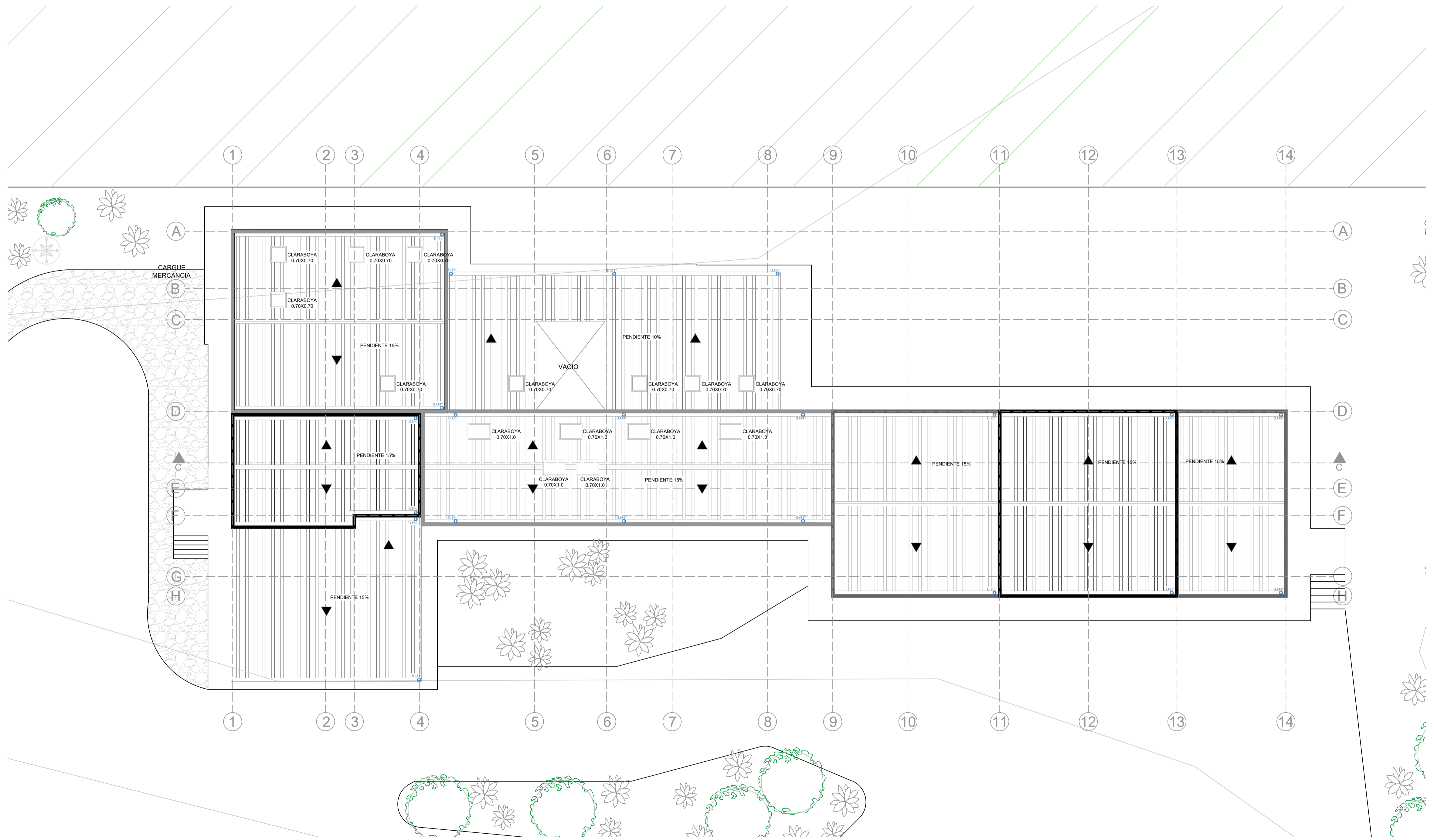
P26 PLANTA CUBIERTAS ESCALA: 1:100
