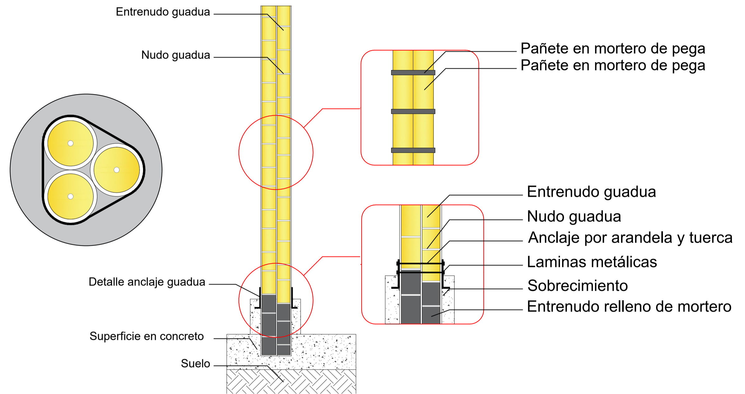
P21 DETALLE COLUMNA EN GUADUA ESCALA: 1:20
