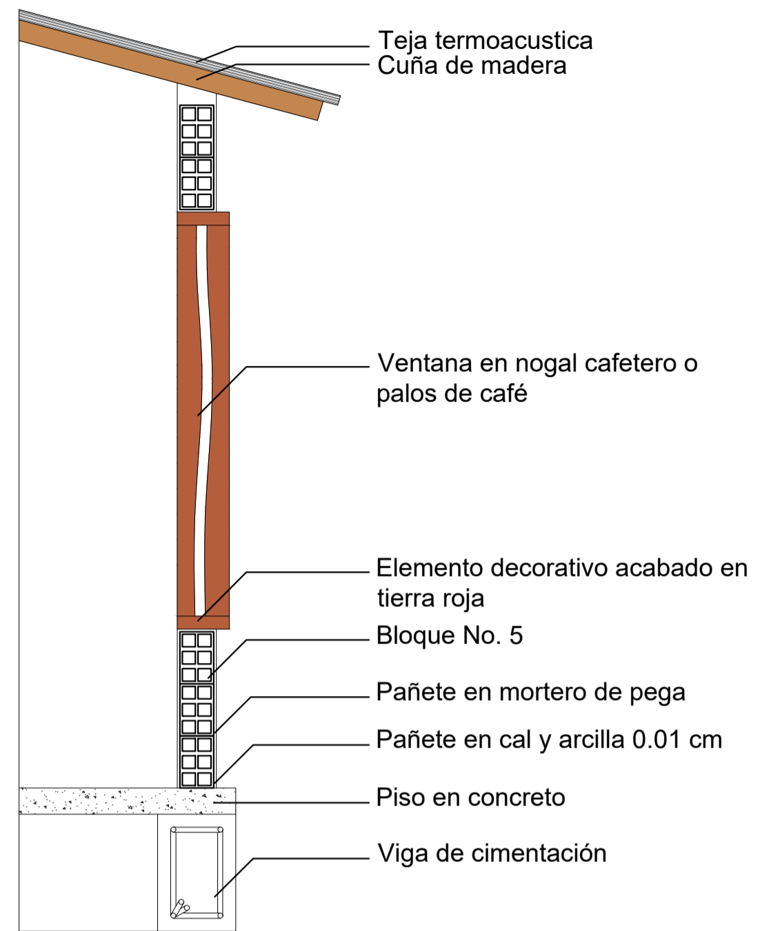
P20 DETALLE MURO COMEDOR ESCALA: 1:20
