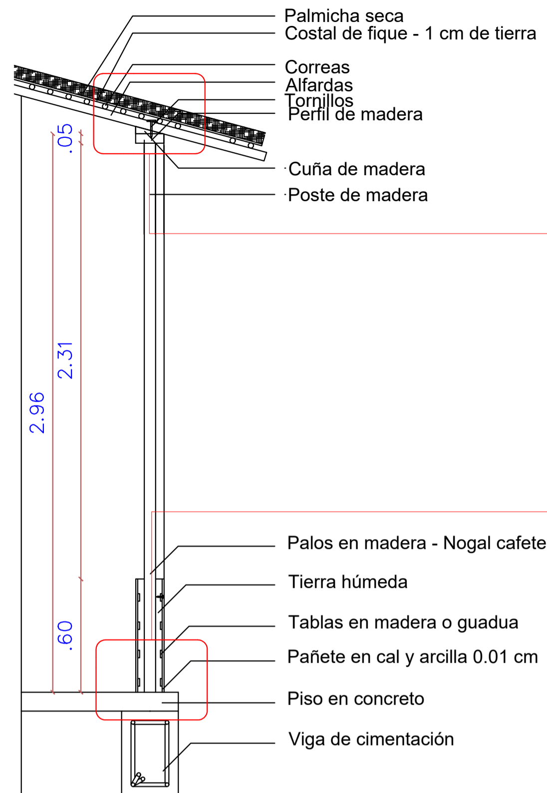
P18 DETALLE MURO EN BAHAREQUE ESCALA: 1:20
