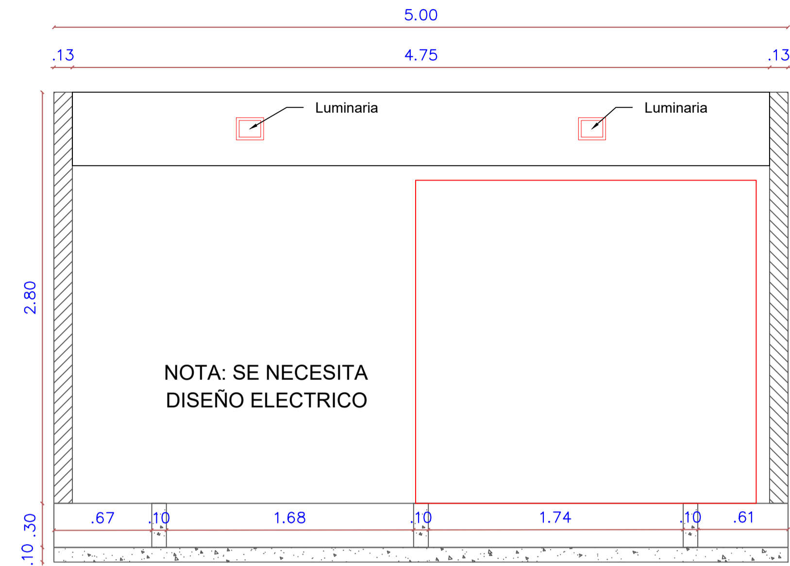
P5 CORTE B-B SUBESTACIÓN ELÉCTRICA ESCALA: 1:25
