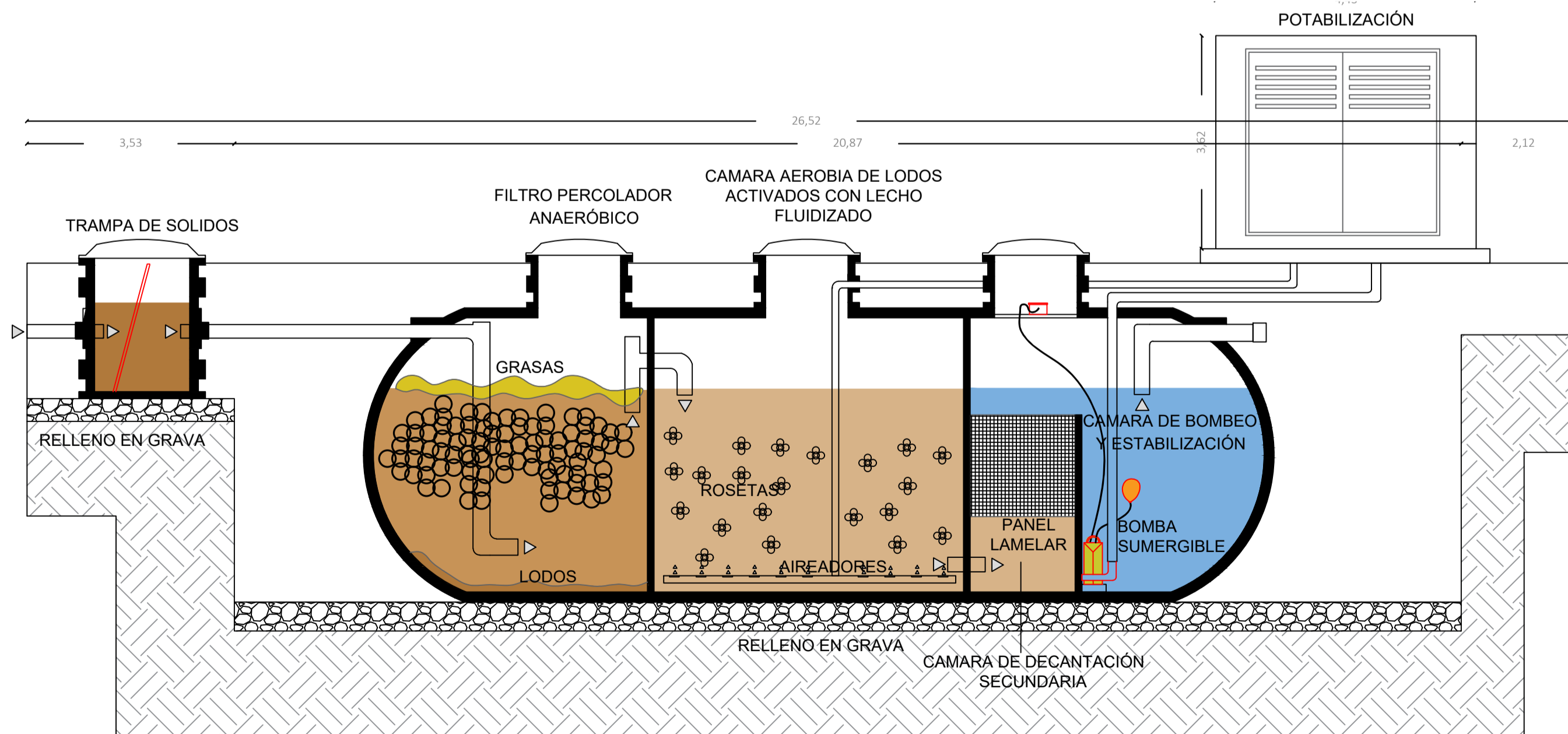
P13 DETALLE PTAR ESCALA: 1:75
