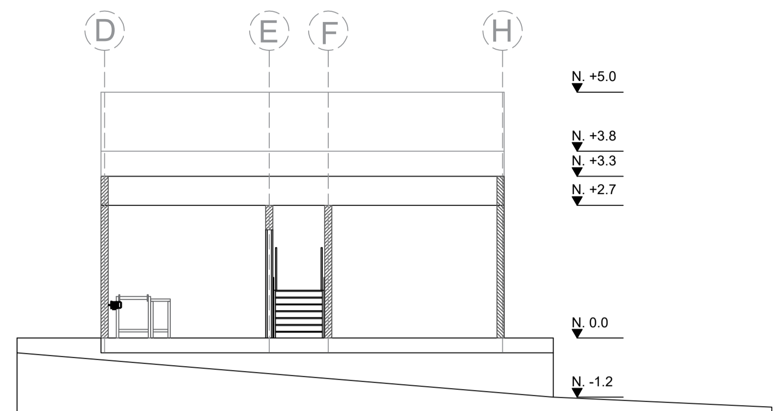
P9 CORTE TRANSVERSAL ESCALA: 1:75
