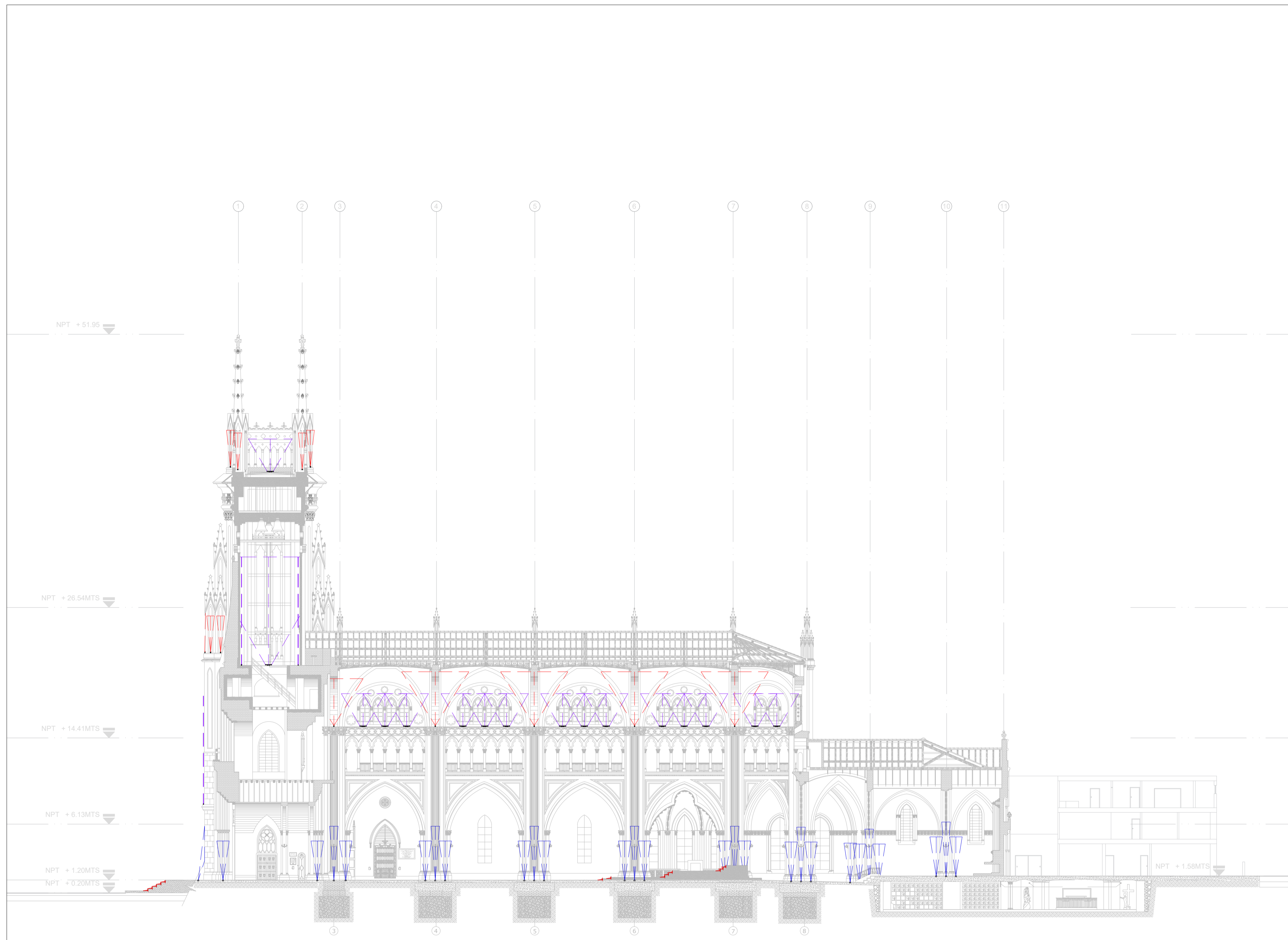
AA Corte longitudinal A - A ESCALA 1:220
