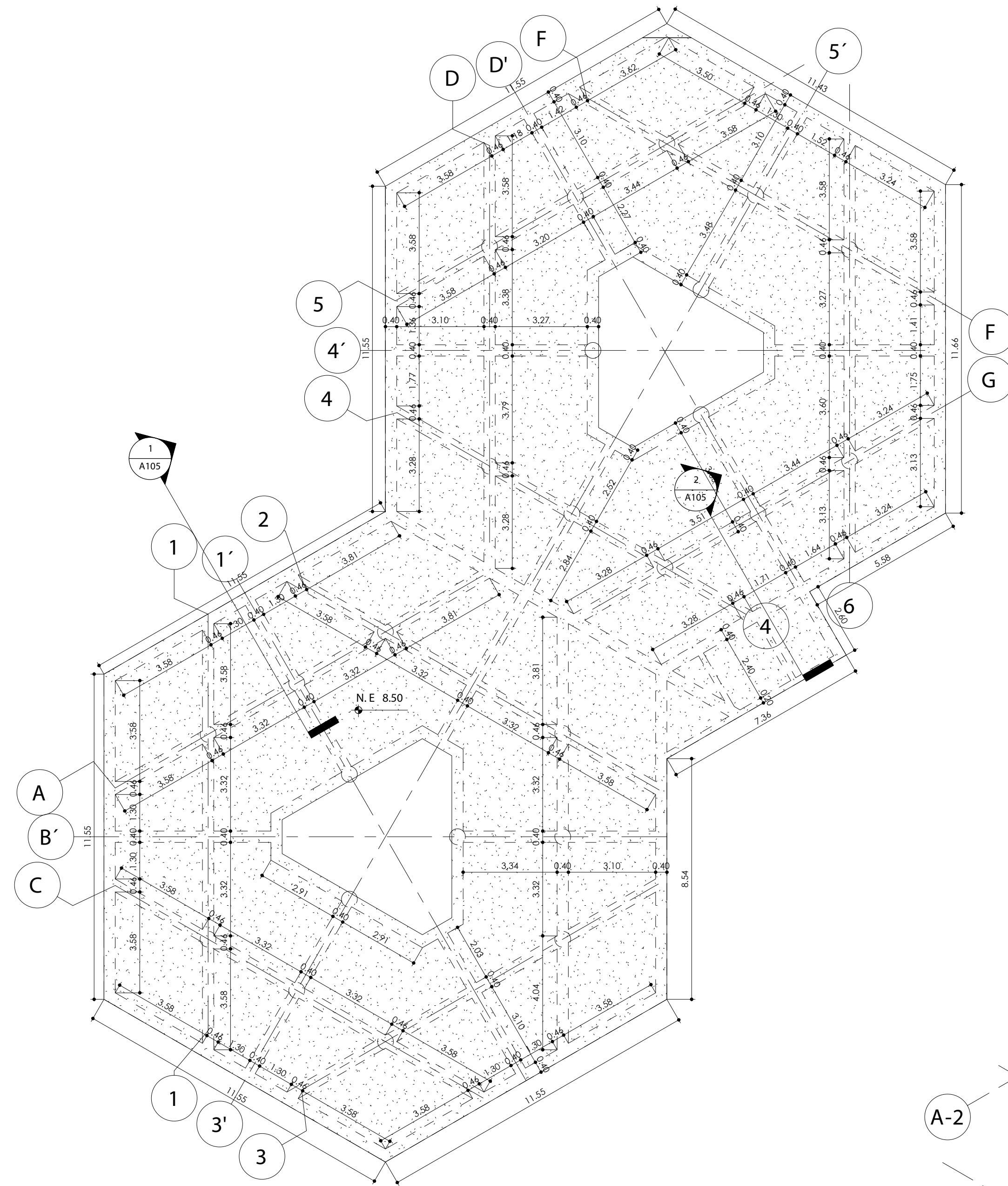
PLANTA NIVEL +8.50 1:125
