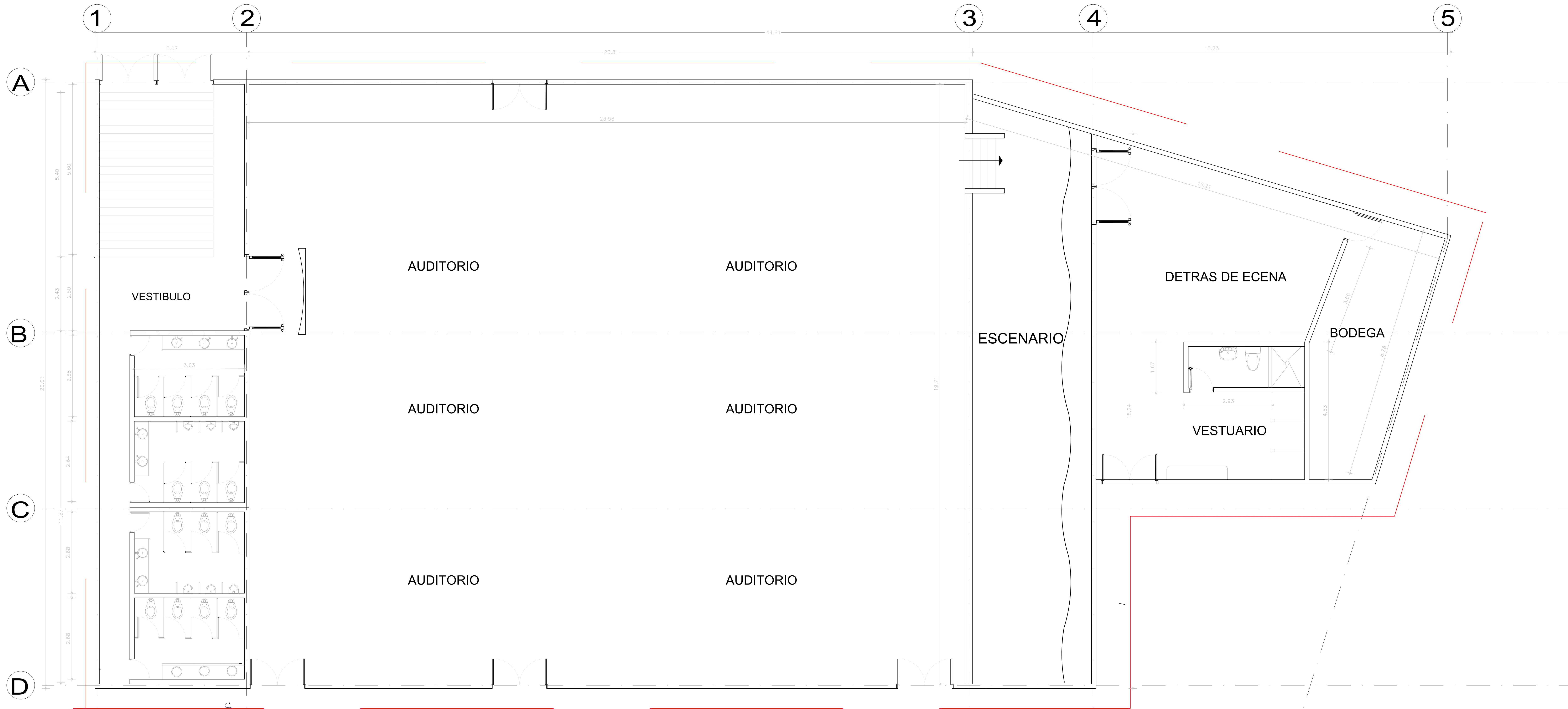
A1 PRIMER NIVEL MODULO 7 ESCALA 1:GRAFICA
