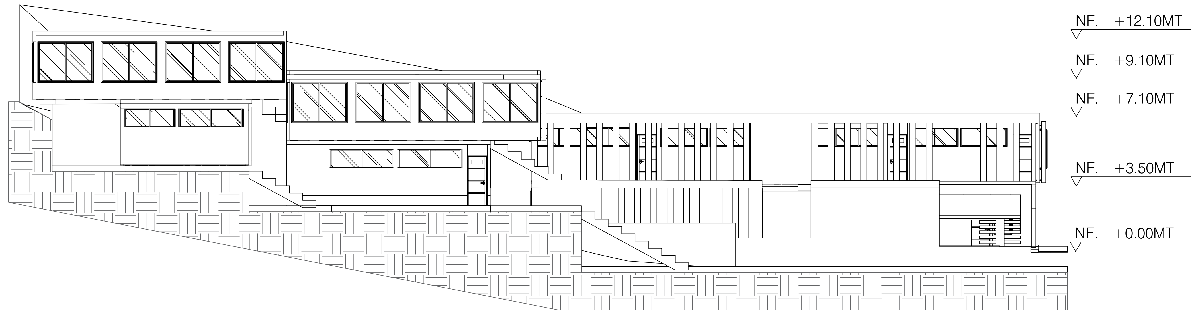
F FACHADA LATERAL DERECHA ESCALA 1:200
