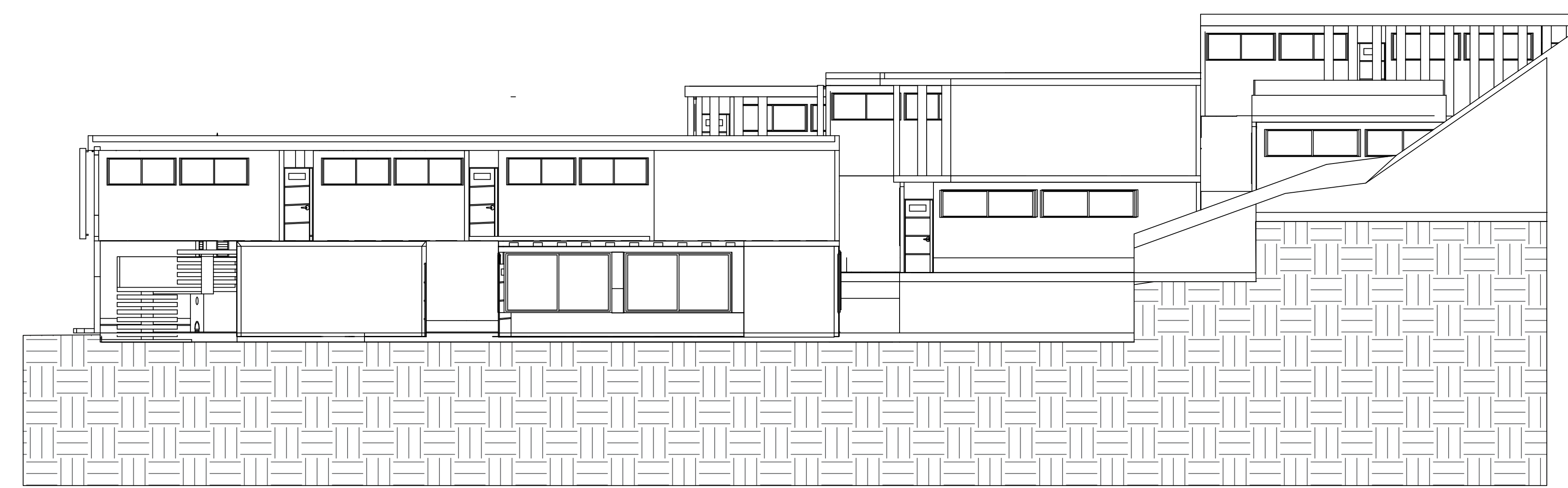
F FACHADA LATERAL IZQUIERDA ESCALA 1:200
