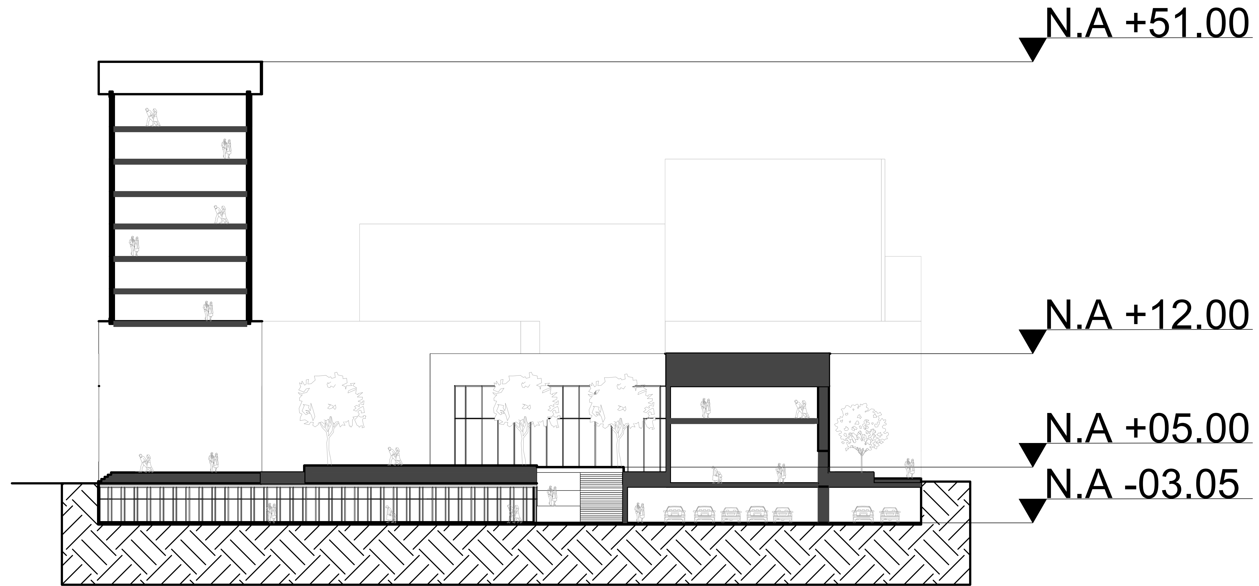
A1 CORTE C-C ESC 1:200
