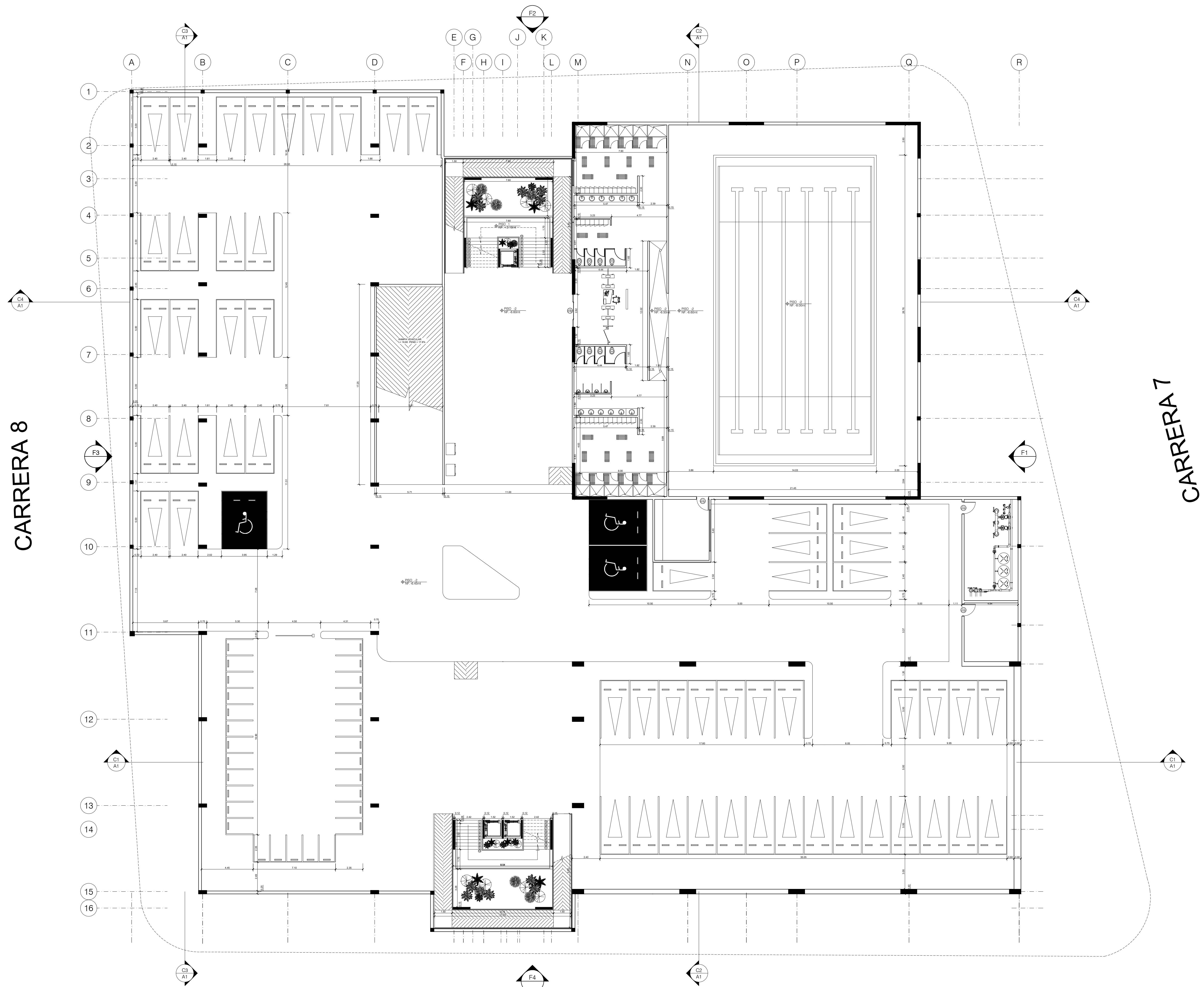
A PLANTA SOTANO 2 ESCALA 1:150 CALLE 18
