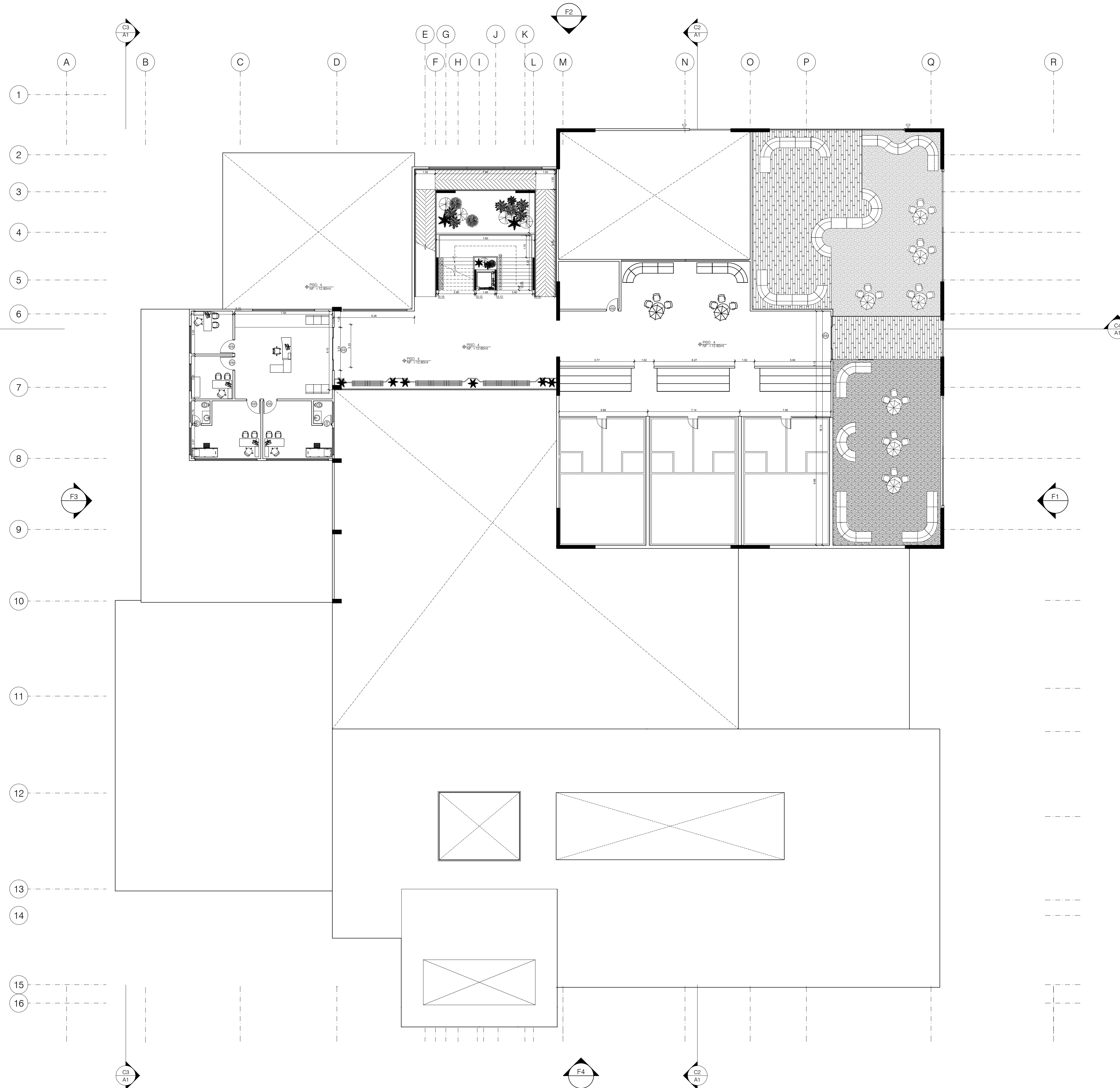
A PLANTA CUARTO PISO ESCALA 1:150 CALLE 18
