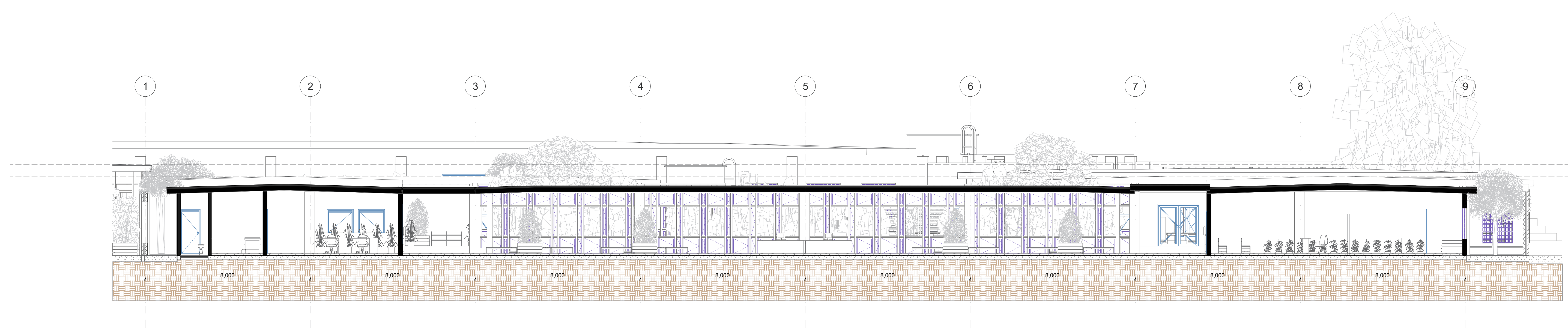
C1 CORTE LONGITUDINAL C1 esc 1:100
