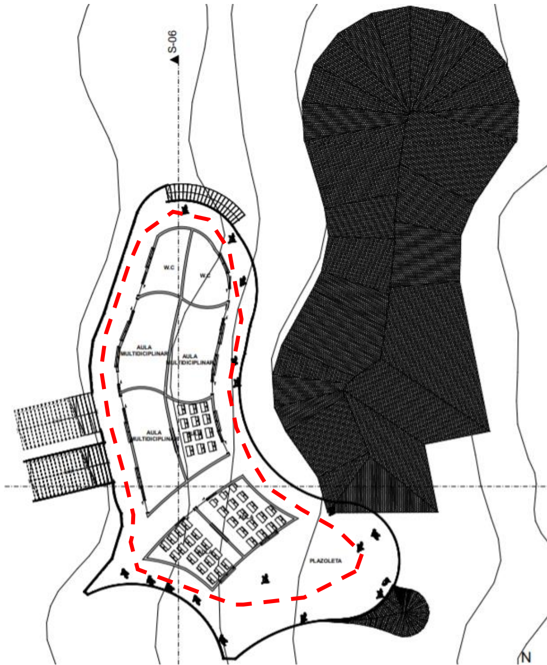
Figura 48 Circulación 3 piso
