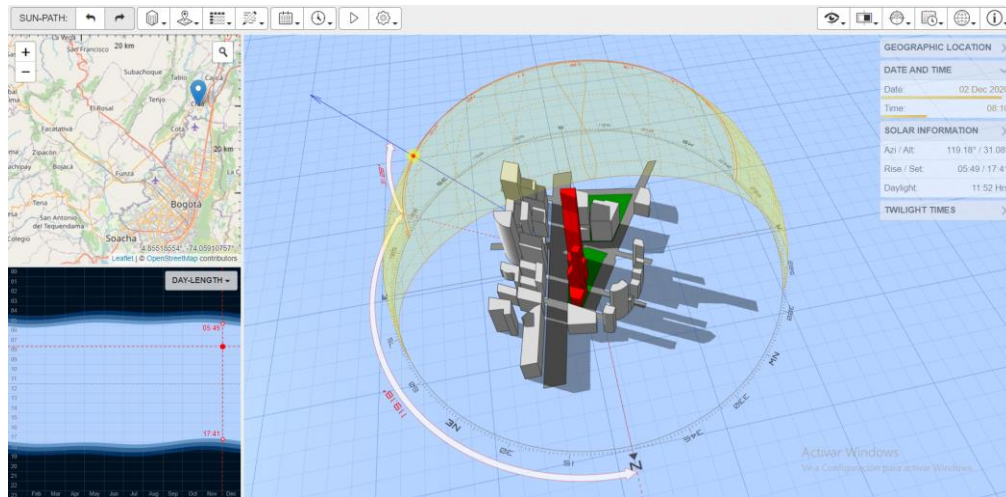
Figura 45 Análisis asolación
