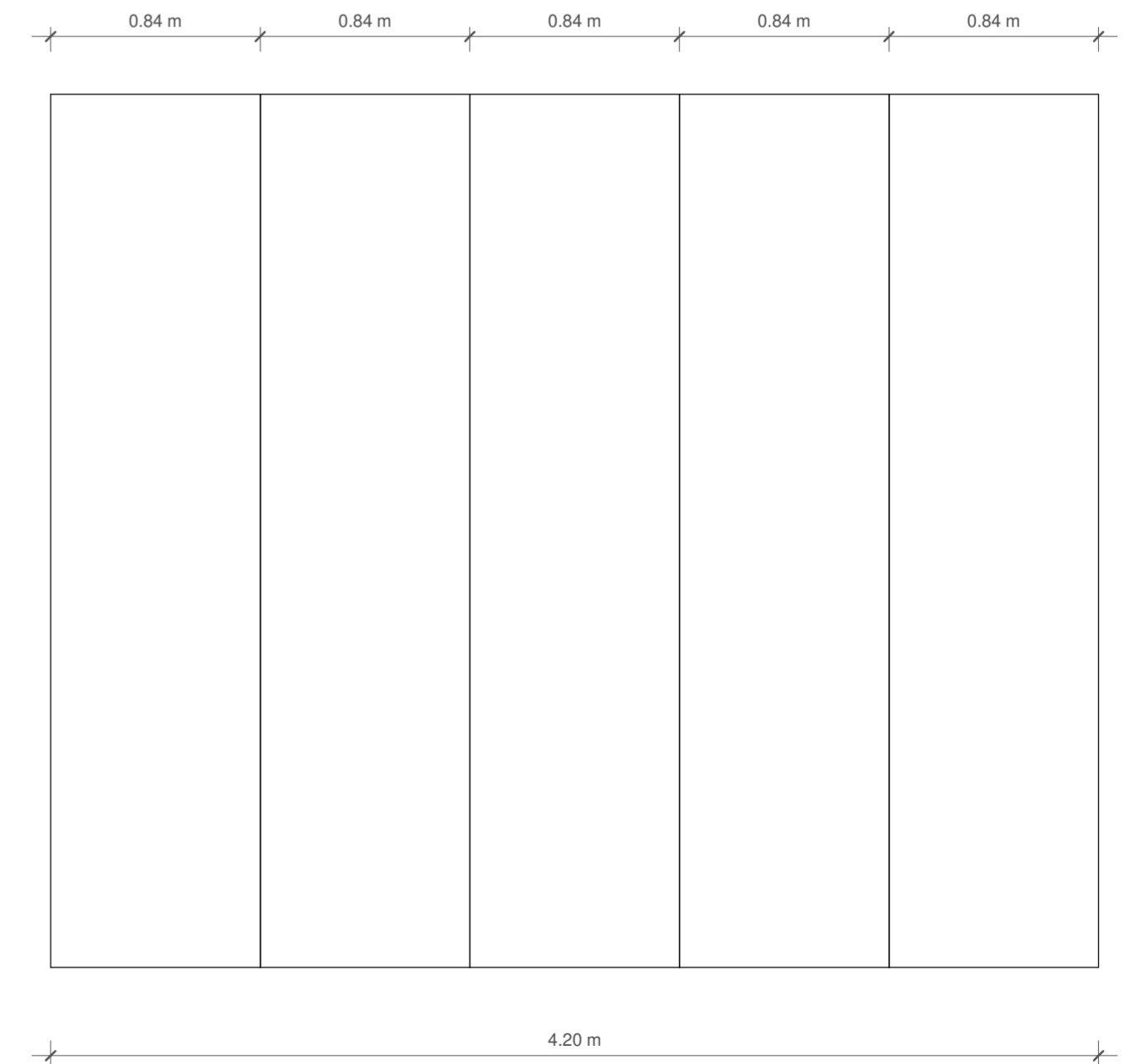
9 Section 37 1 : 25
