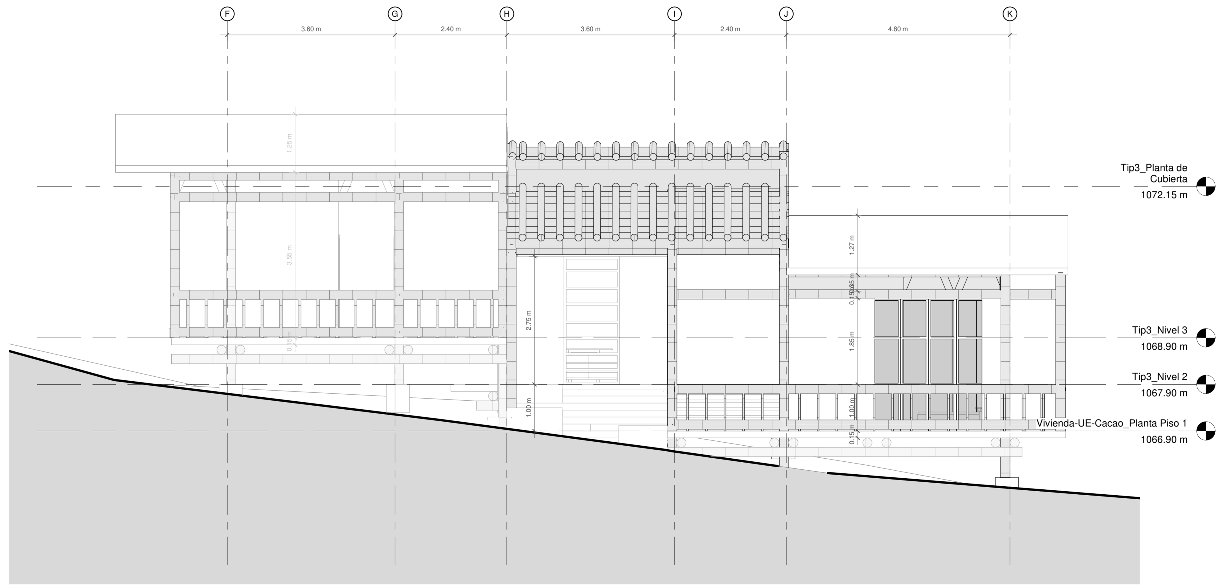
1 Fachada Acceso 1 : 50
