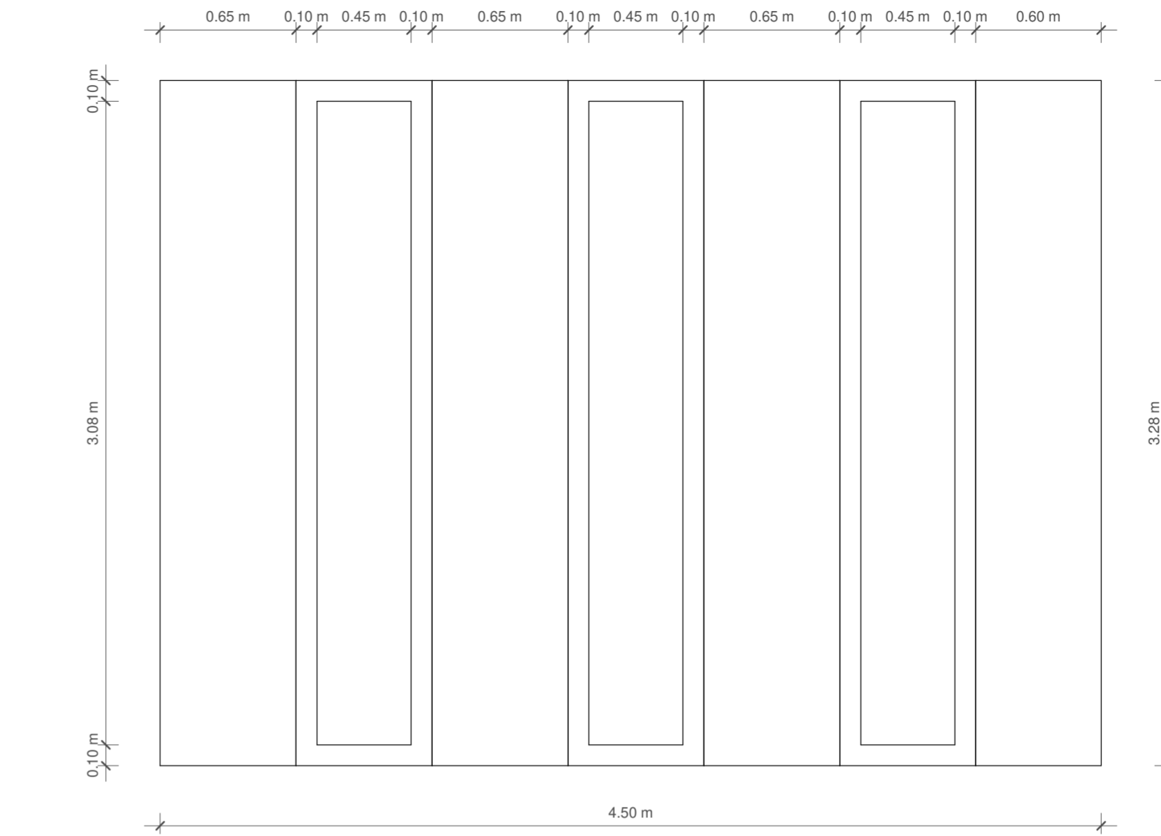
6 Section 34 1 : 25
