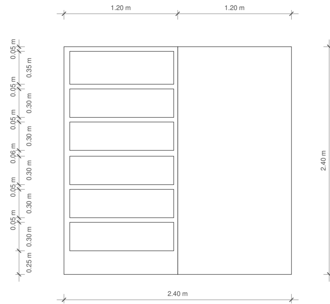
1 Section 1 1 : 25
