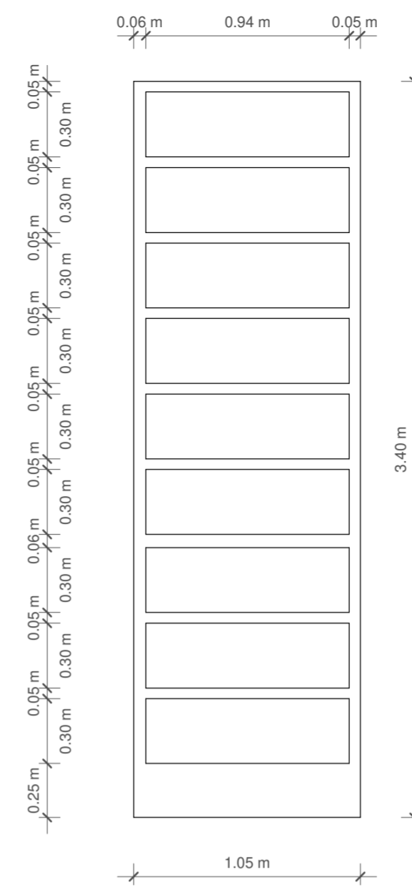
4 Section 13 1 : 25
