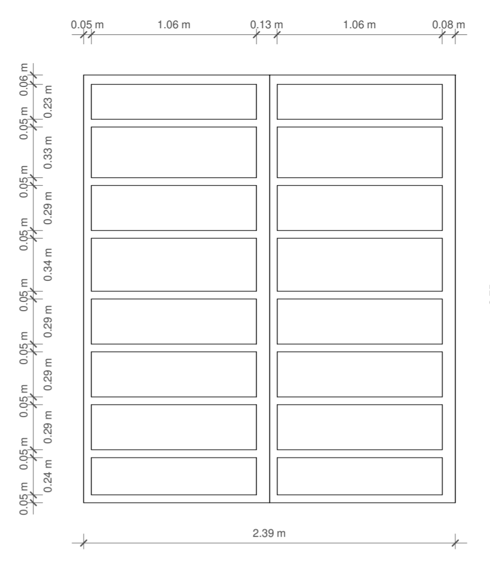
6 Section 24 1 : 25
