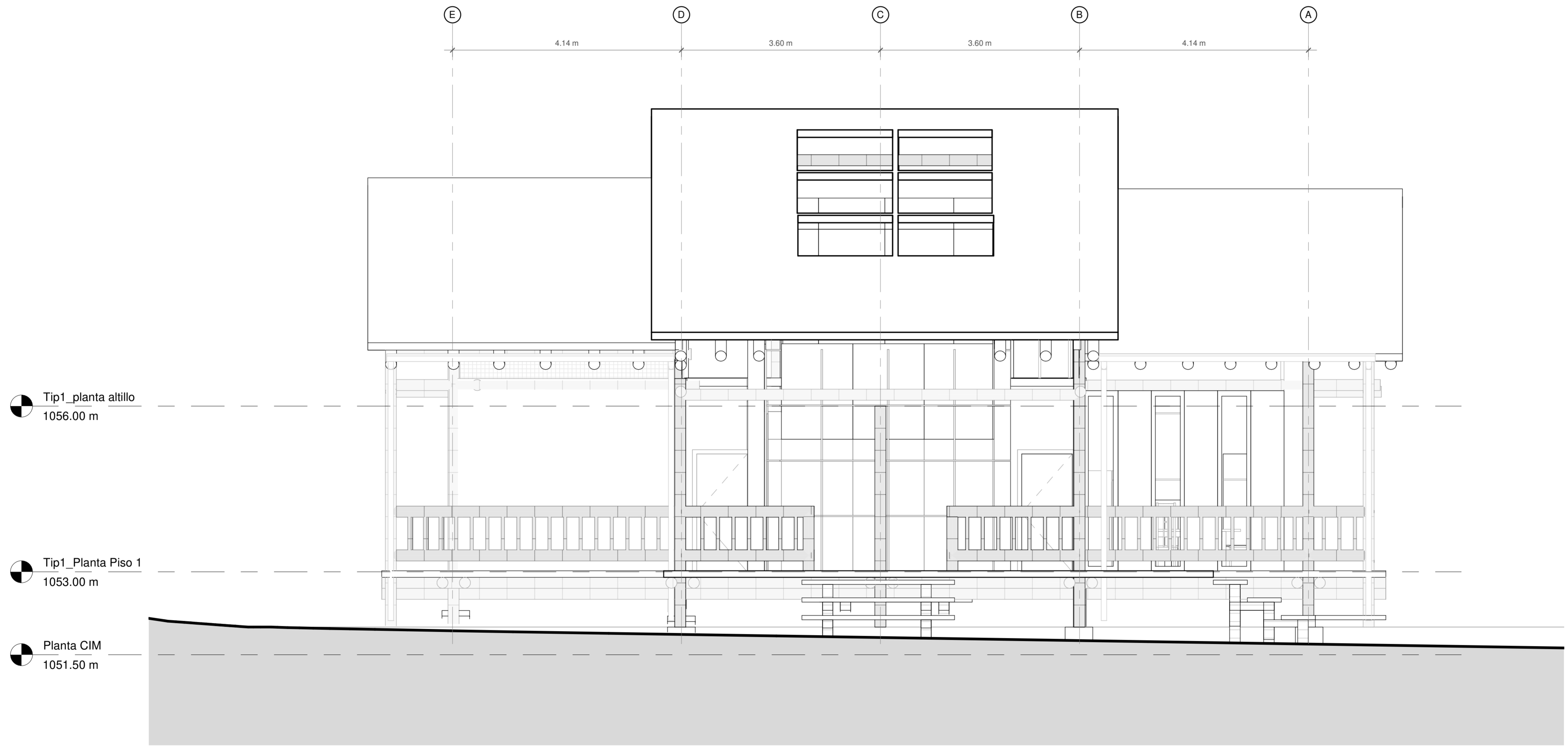
1 Fachada Oriente 1 : 50
