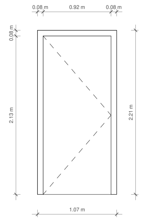
10 Section 28 1 : 25
