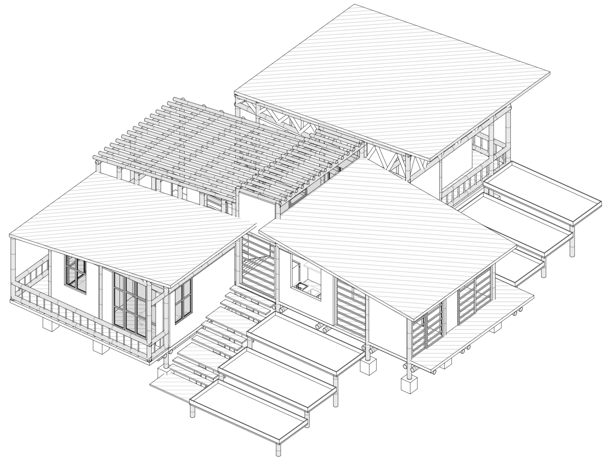
3 Vivienda-UE-Cacao_ISOMETRICO GENERAL
