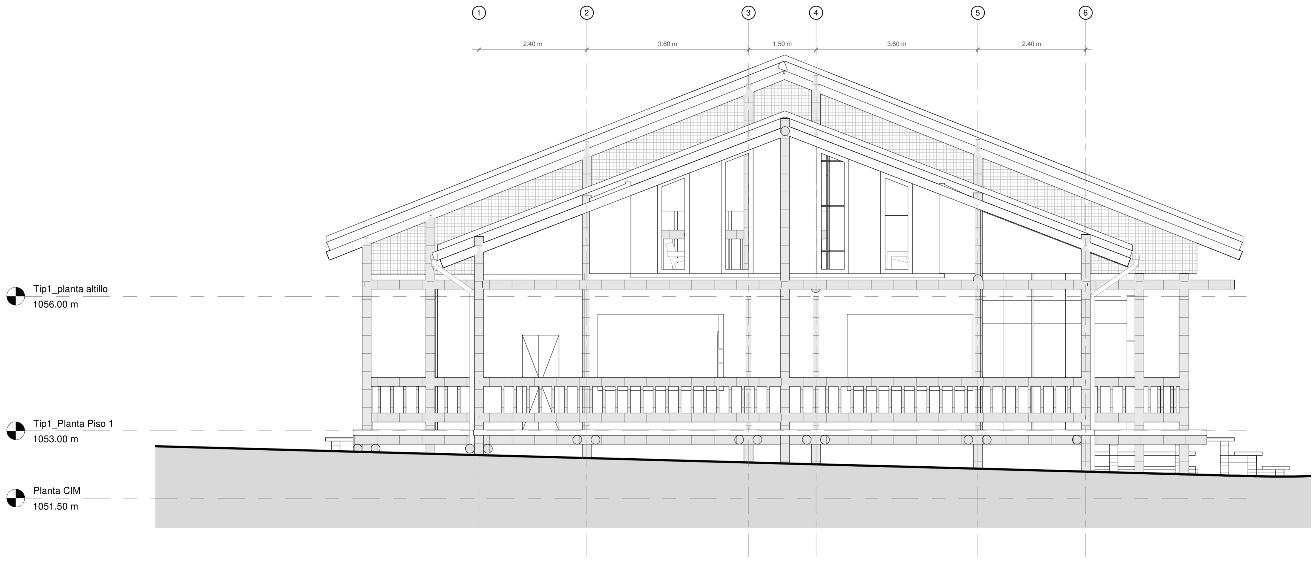
1 Fachada Sur 1 : 50
