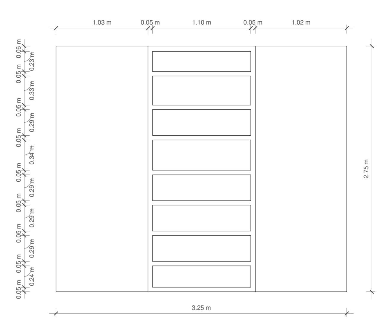
9 Section 27 1 : 25
