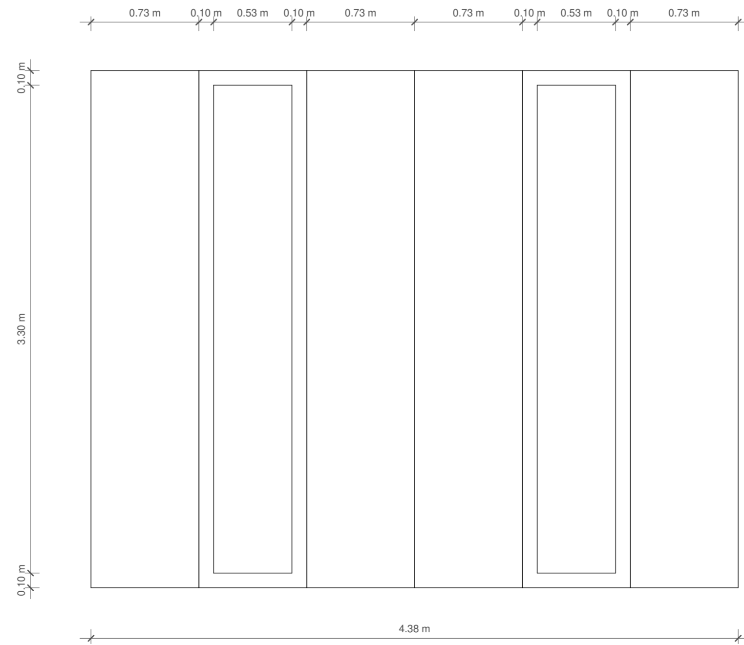
7 Section 35 1 : 25
