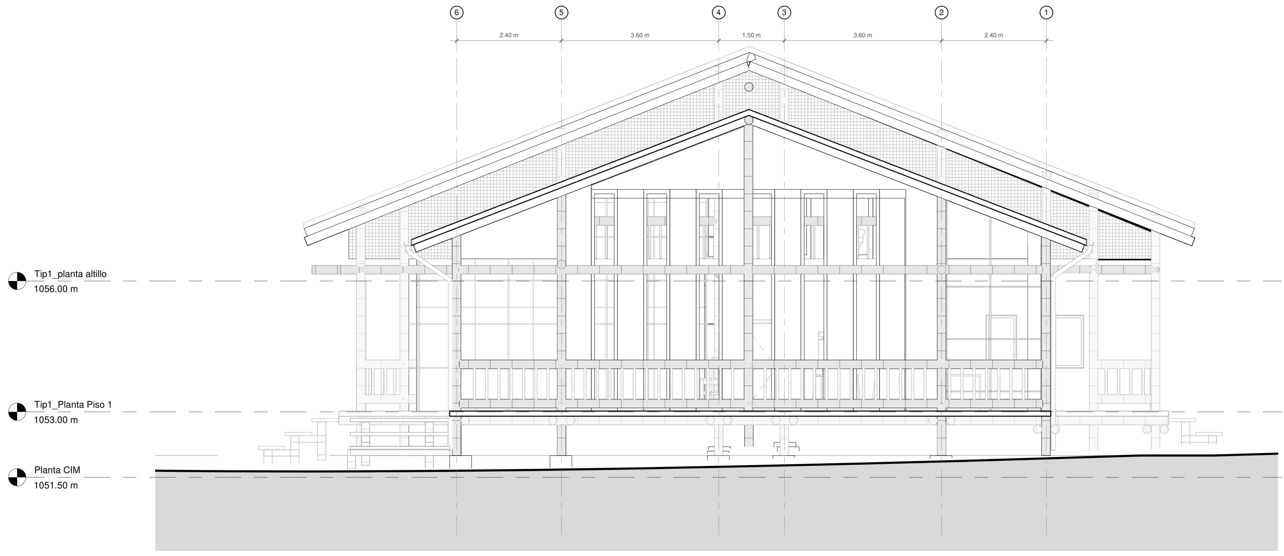
2 Fachada Norte 1 : 50
