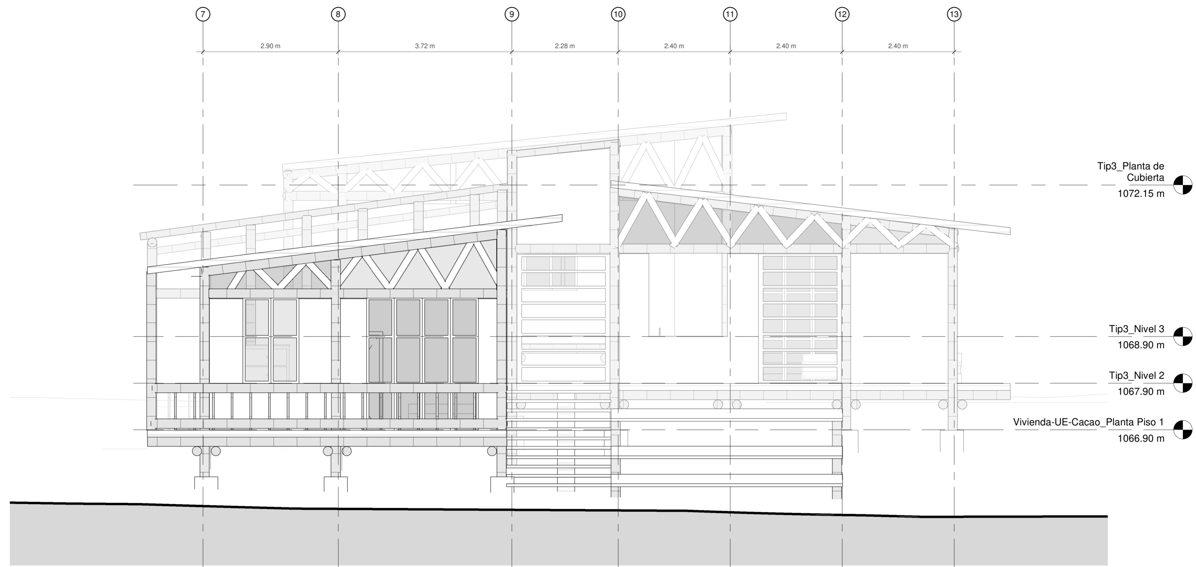
1 Fachada principal 1 : 50
