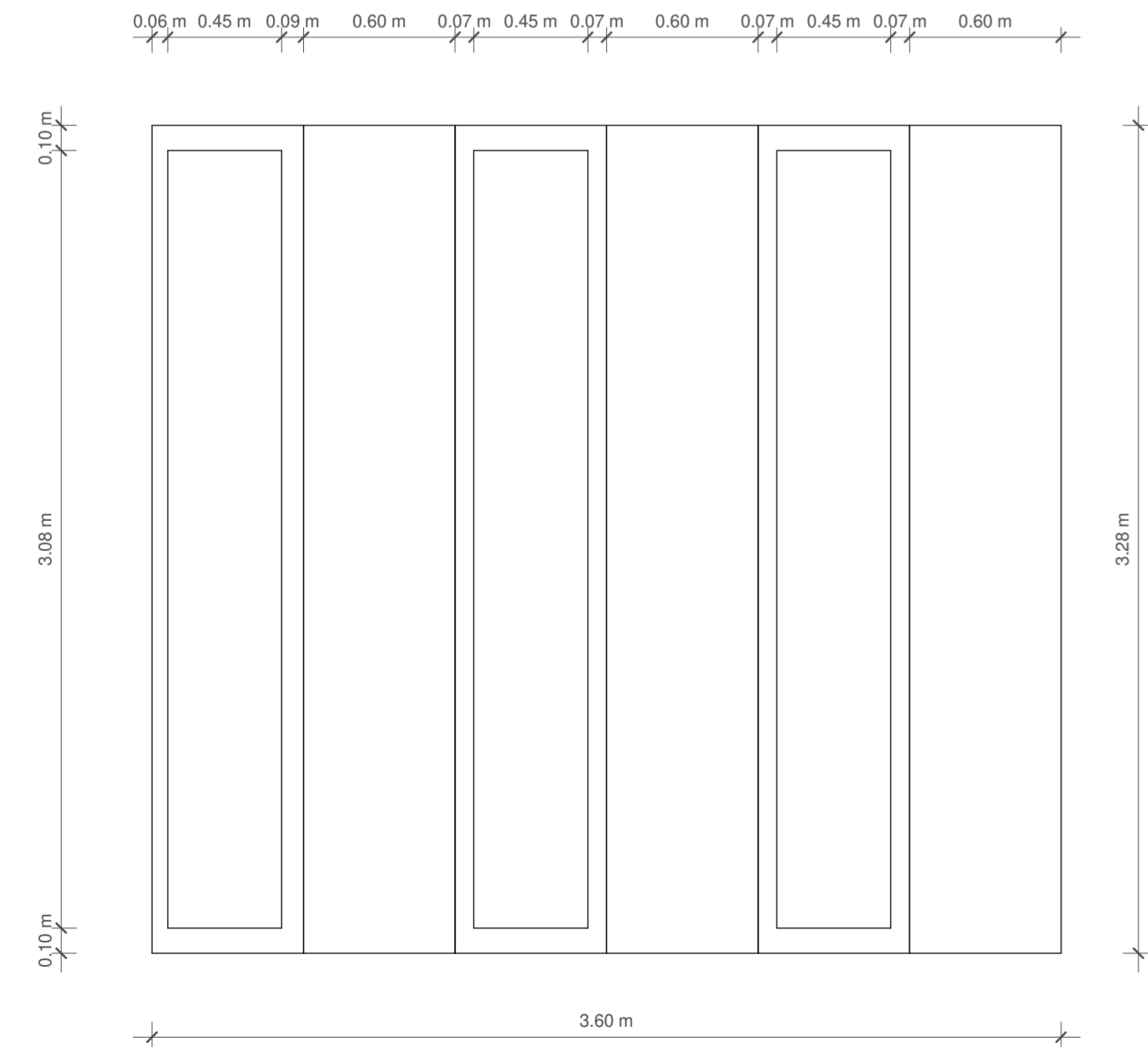
2 Section 30 1 : 25
