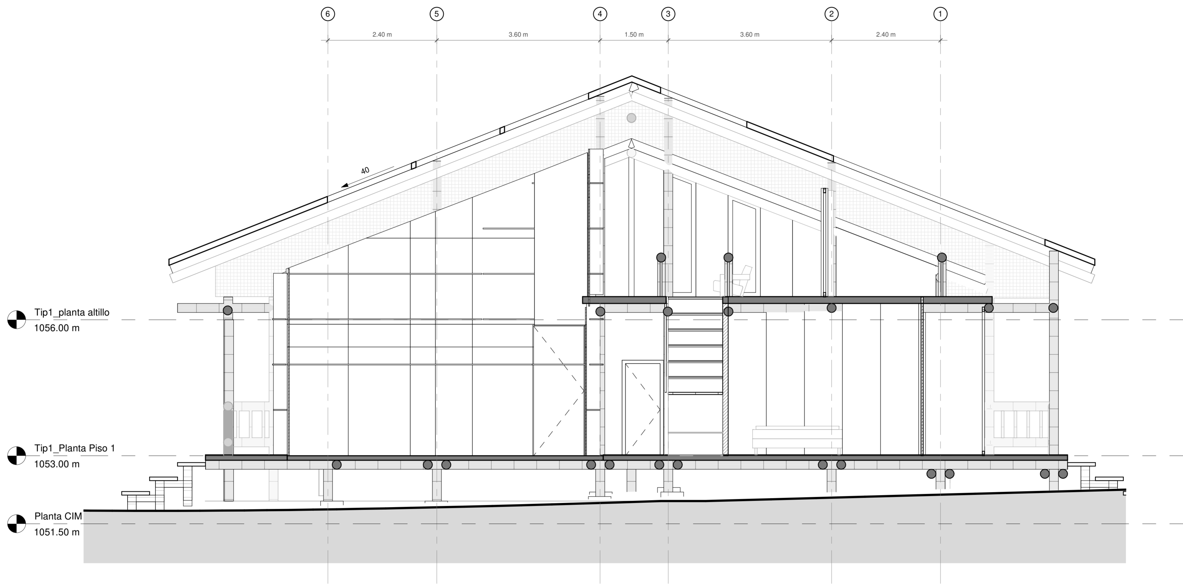
1 Corte A 1 : 50
