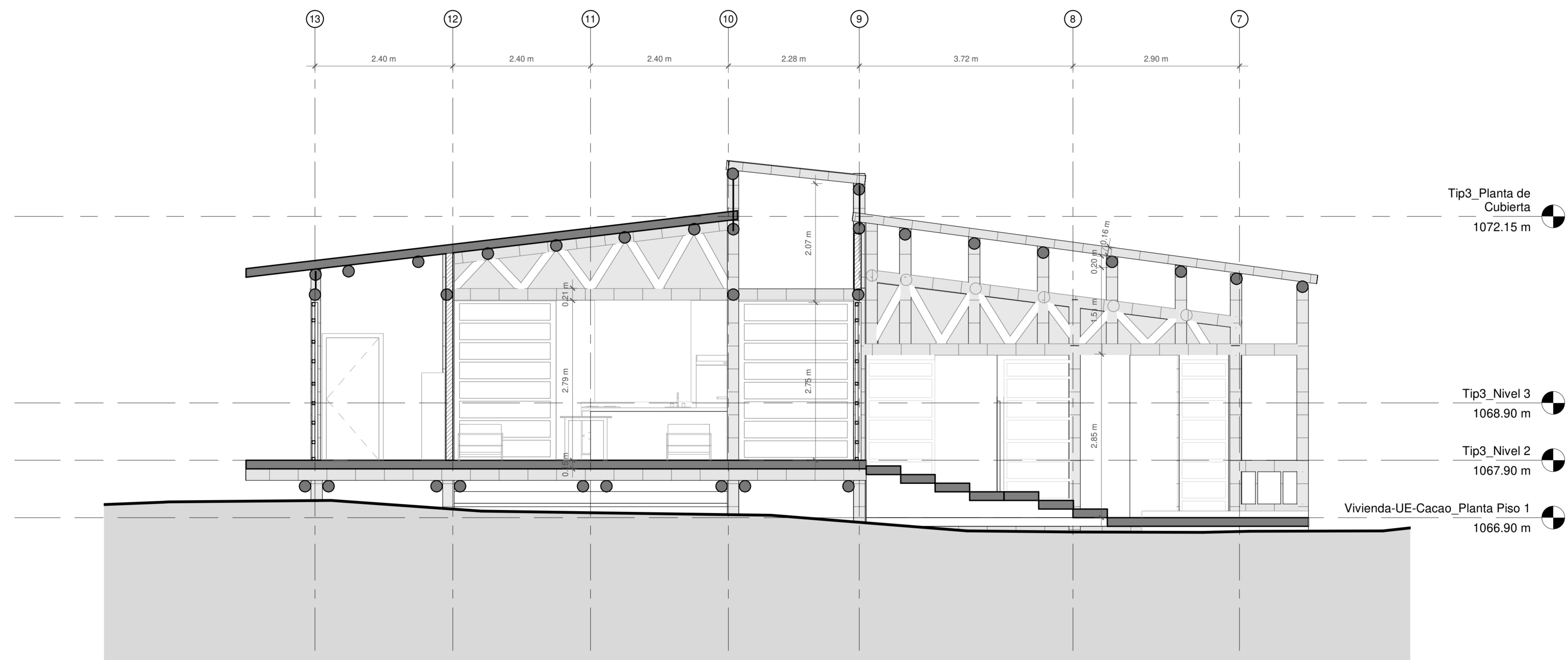
1 Corte A-A 1 : 50
