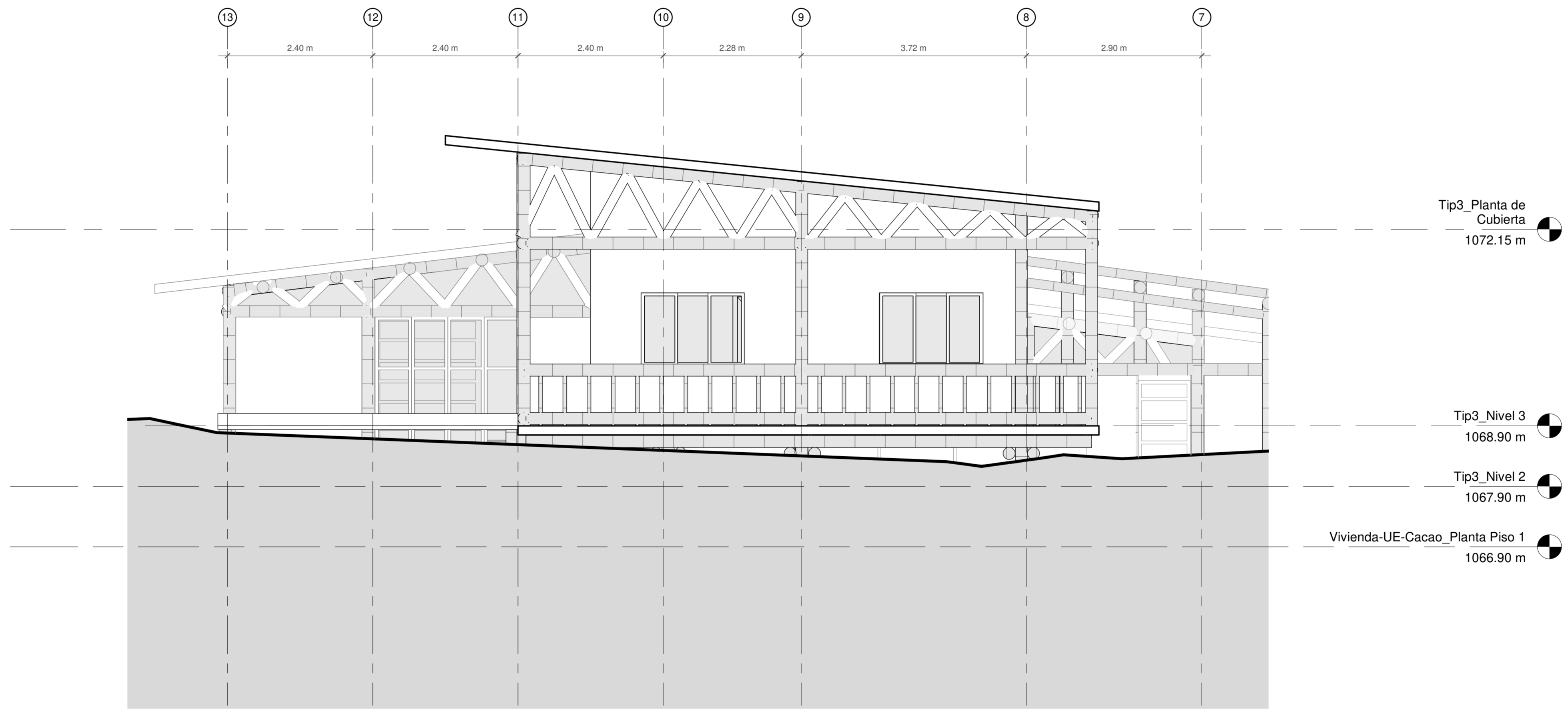
1 Fachada Posterior 1 : 50
