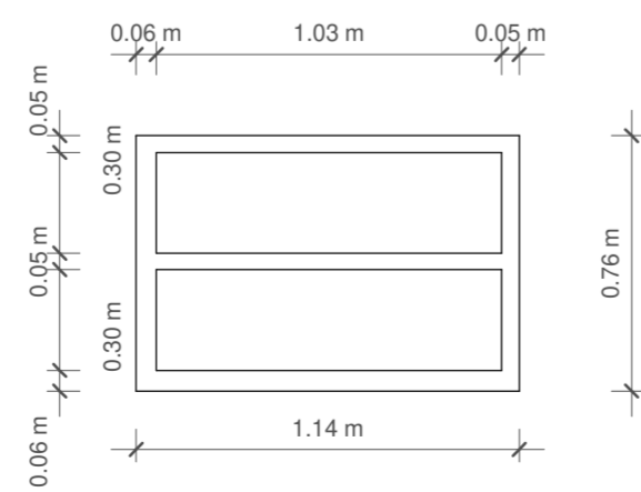
7 Section 16 1 : 25
