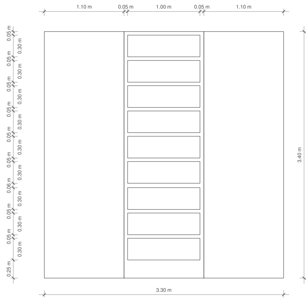
3 Section 12 1 : 25
