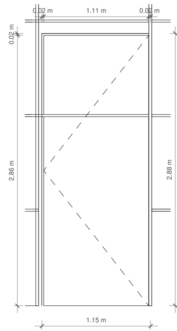
3 Section 33 1 : 25
