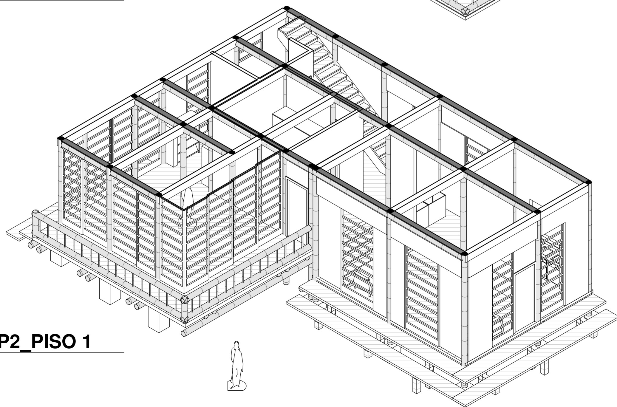
2 TIP2_PISO 2
