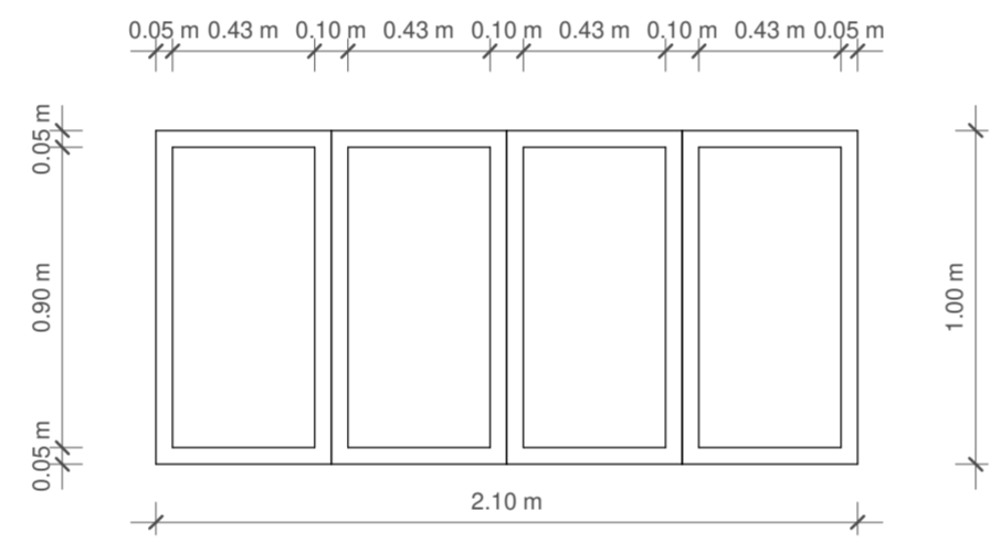
9 Section 18 1 : 25
