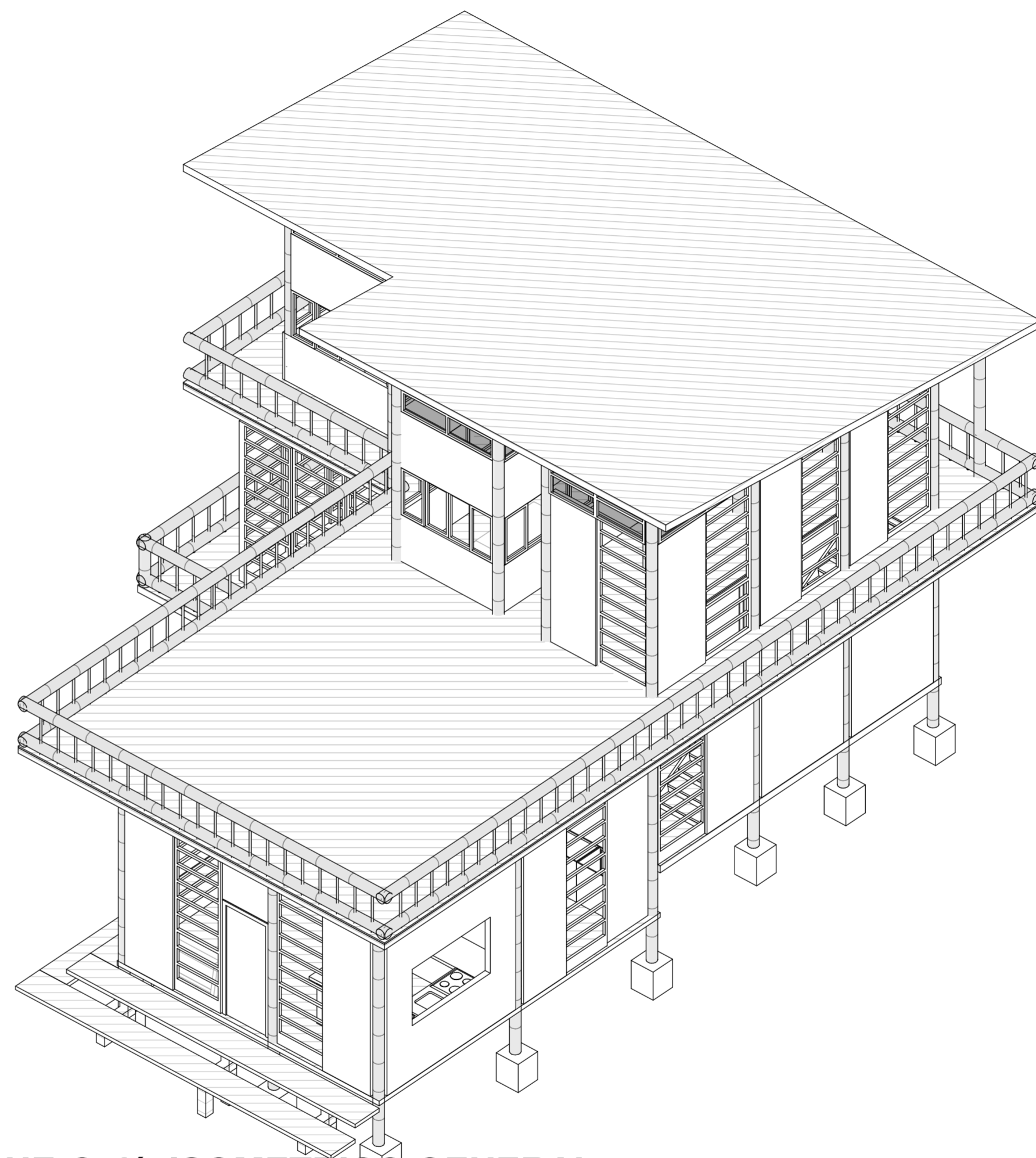
1 Vivienda-UE-Café_ISOMETRICO GENERAL
