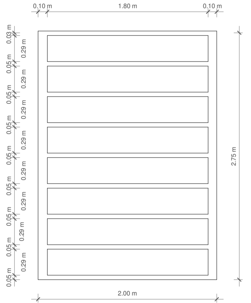
4 Section 22 1 : 25
