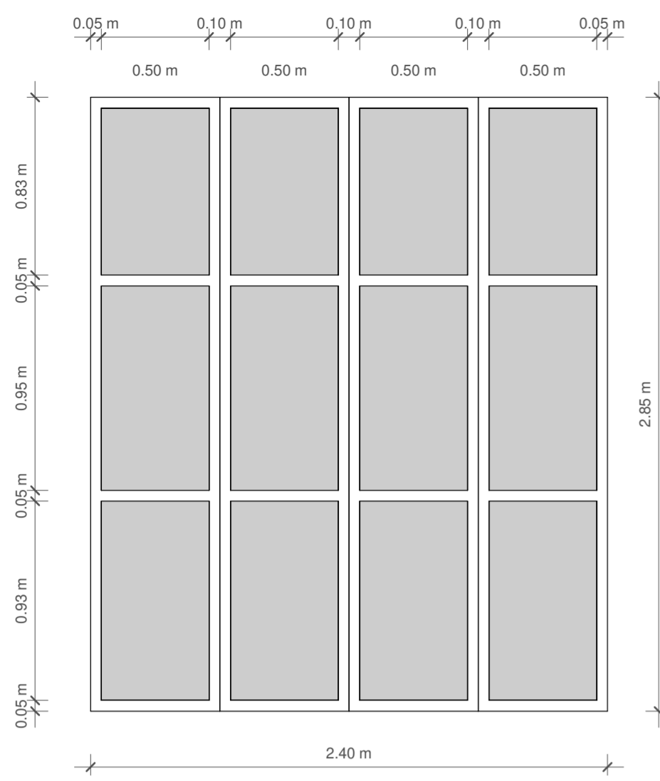
1 Section 19 1 : 25
