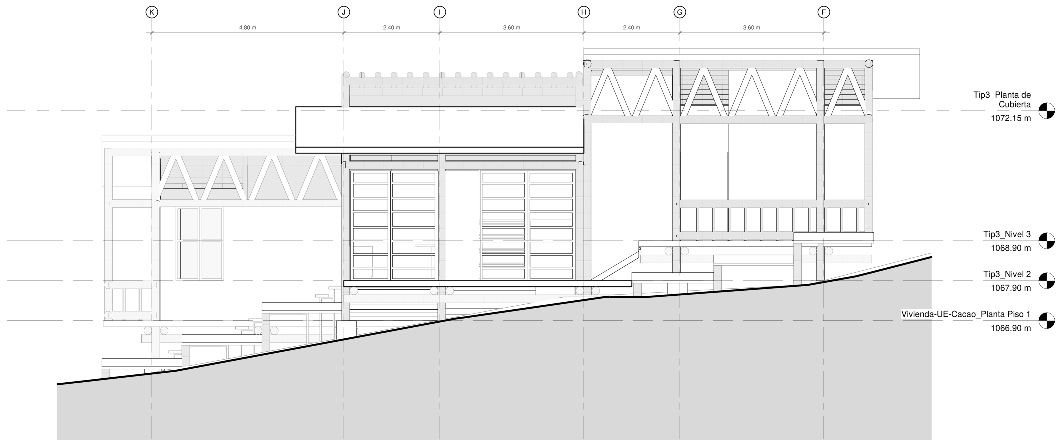
1 Fachada Bodega 1 : 50
