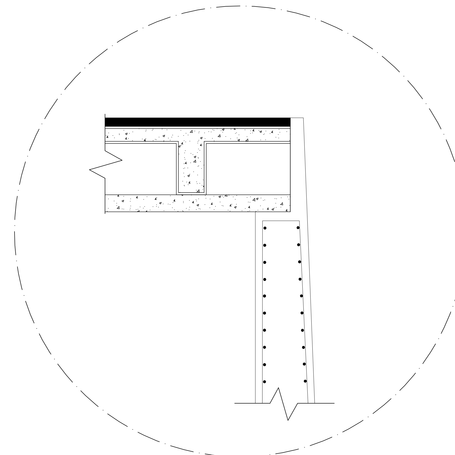
D2 DETALLE ANCLAJE MURO PANTALLA ESC: 1.150
