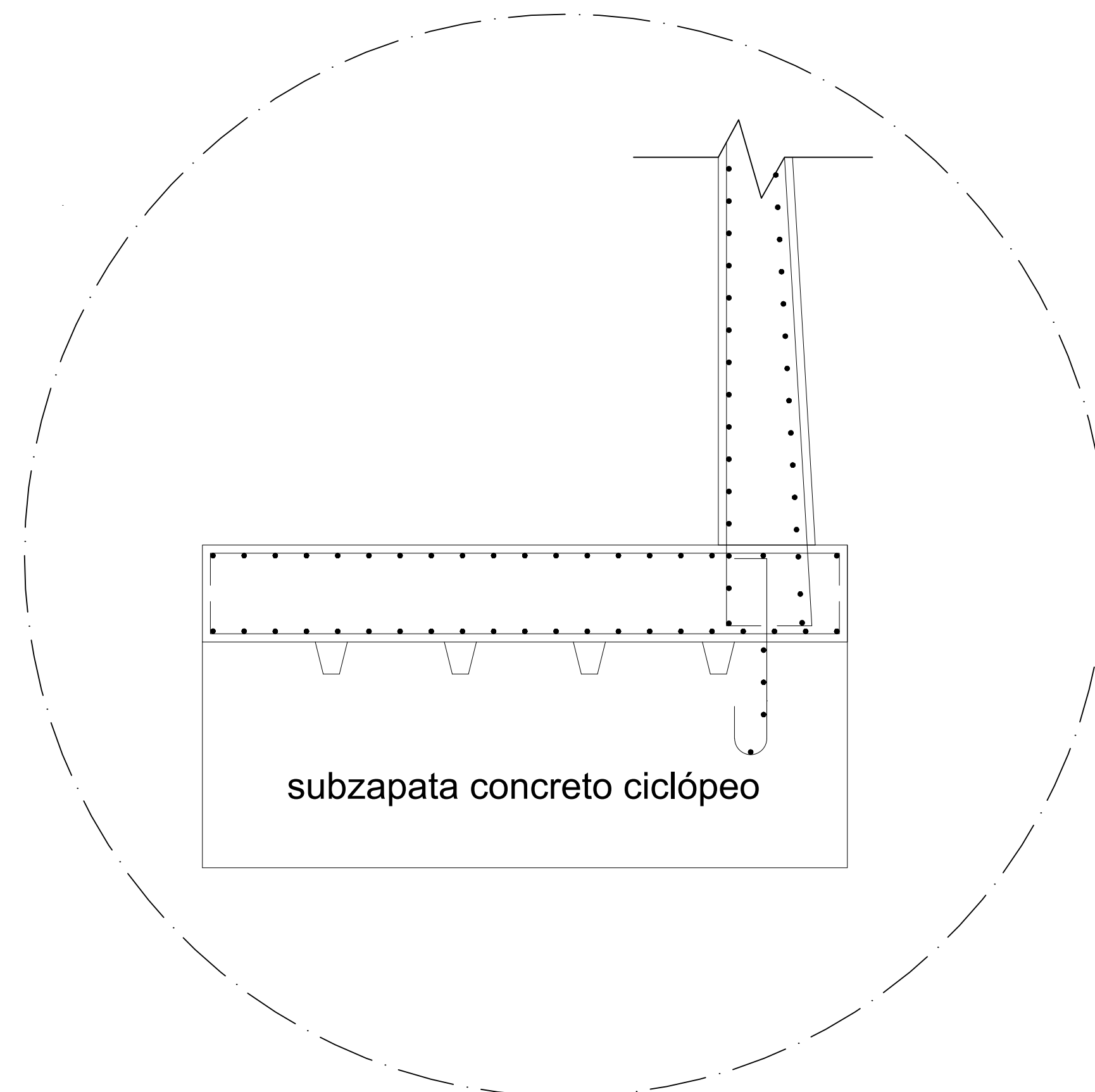
D1 DETALLE MURO PANTALLA ESC: 1.150
