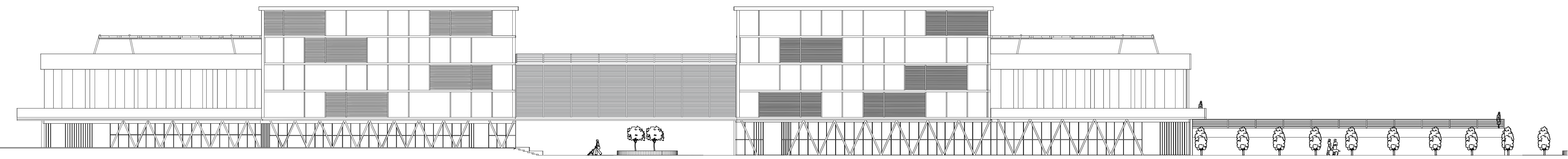
SECCIÓN 1 - C. OFICIOS TRADICIONALES ESC 1:200
