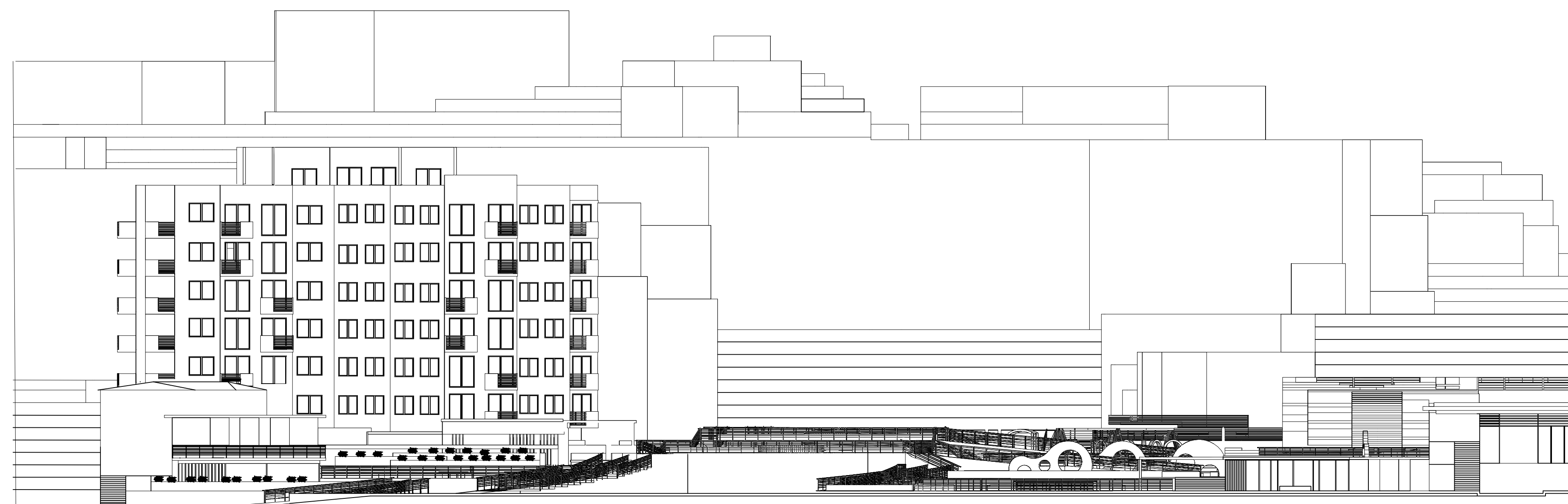
SECCIÓN 2 - PARQUE ESC 1: 250
