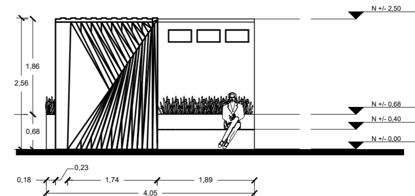
ALZADO FONTRAL TIPOLOGIA 1
