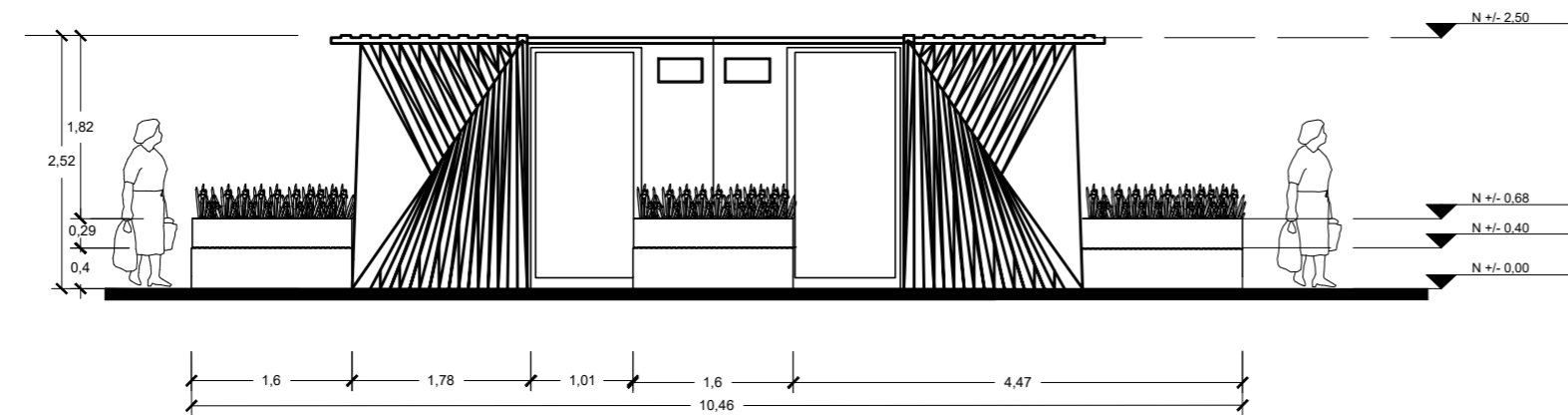
ALZADO FONTRAL TIPOLOGIA 3
