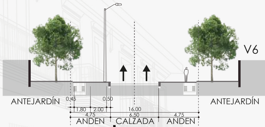
PERFIL VIAL PROPUESTO
