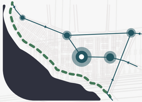
DEGRADACIÓN AMBIENTAL
