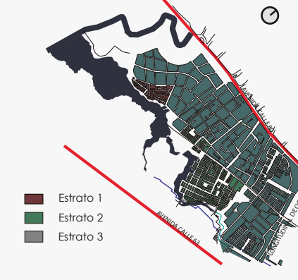
ESTRATIFICACIÓN
