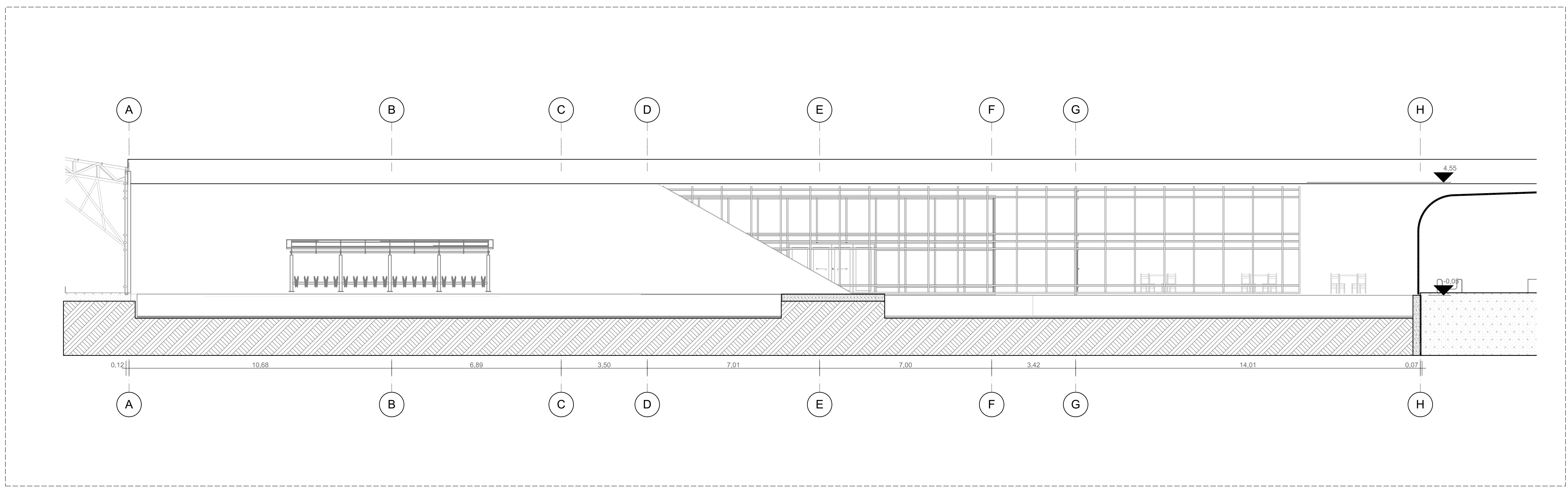
F 4 FACHADA CENTRO CAPACITACION 1:75
