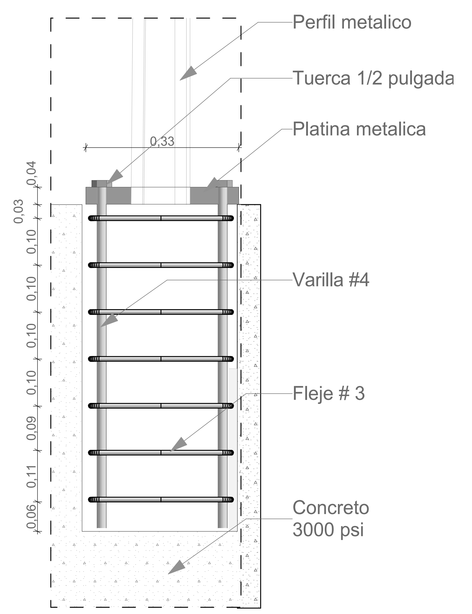
D-01 Detalle muro contención 1:5
