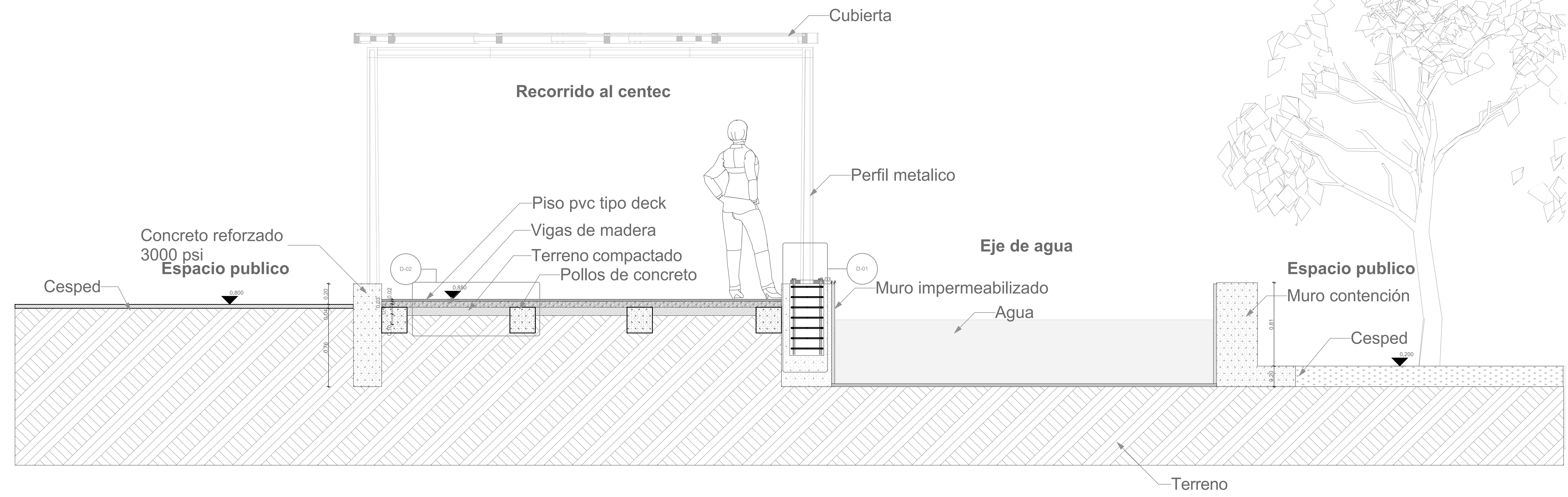
D-02 CORTE 1:20
