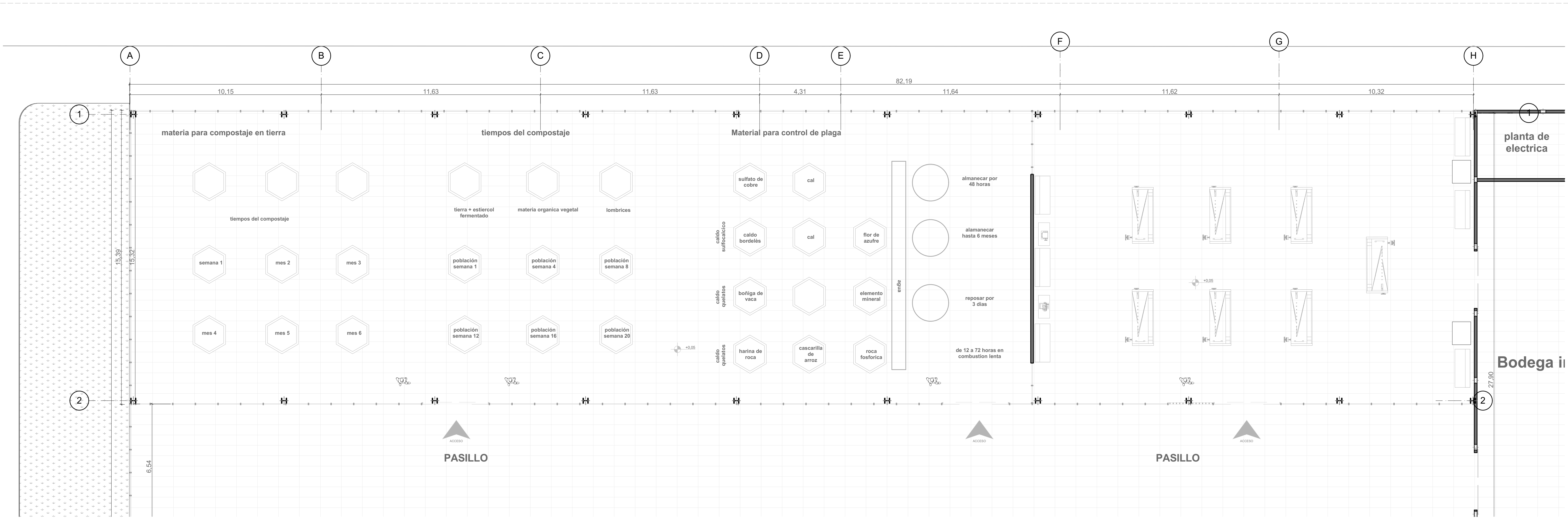
SECCION 1. ZONA COMPOSTAJE Y CARPINTERIA
