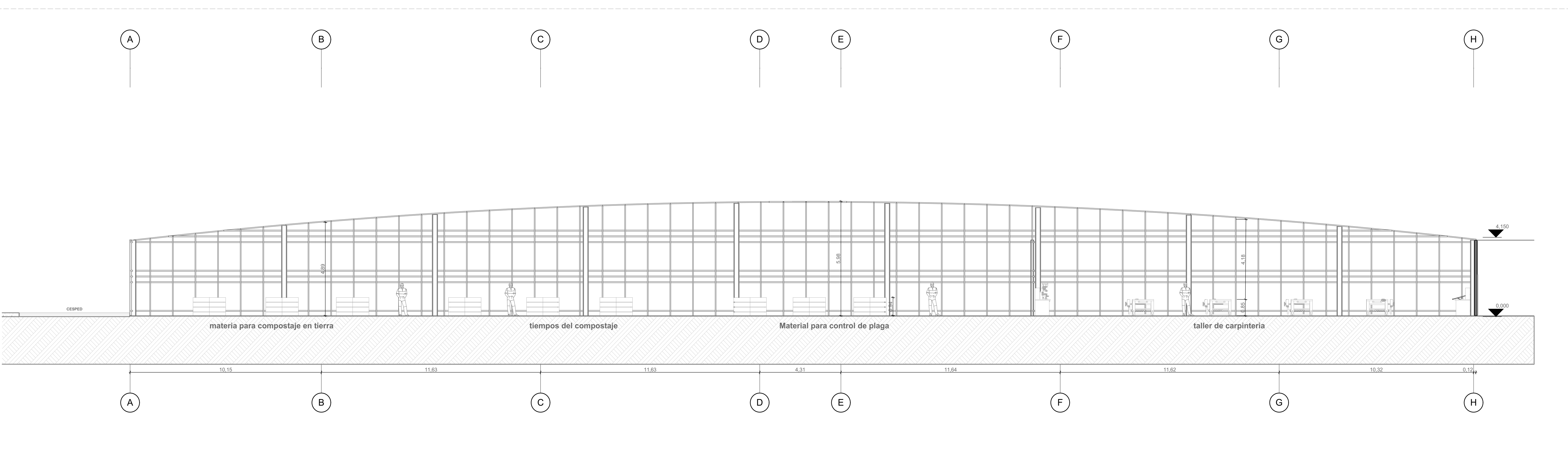
CORTE ZONA COMPOSTAJE
