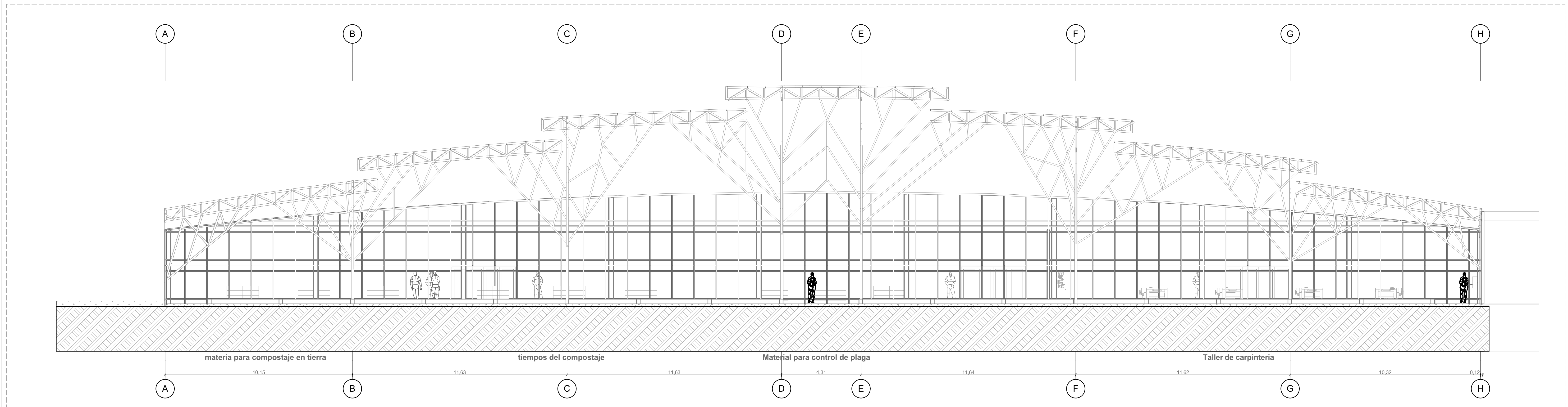
C-02 CORTE ZONA DE PRACTICAS 1:100
