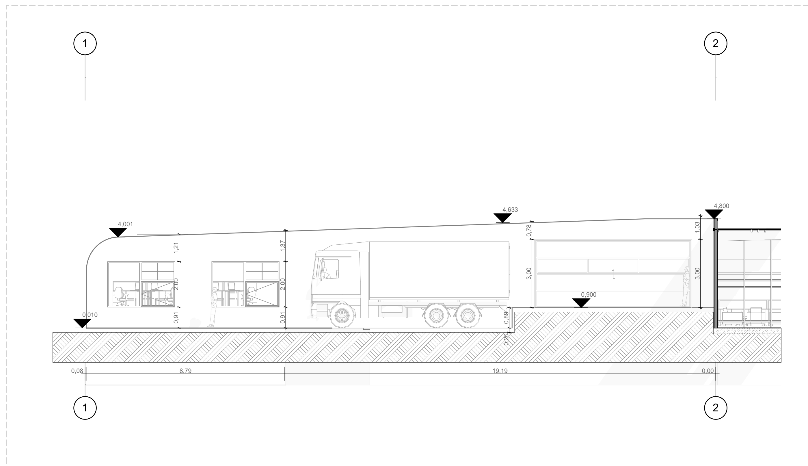
C-05 corte zona de carga pecuaria 1:100
