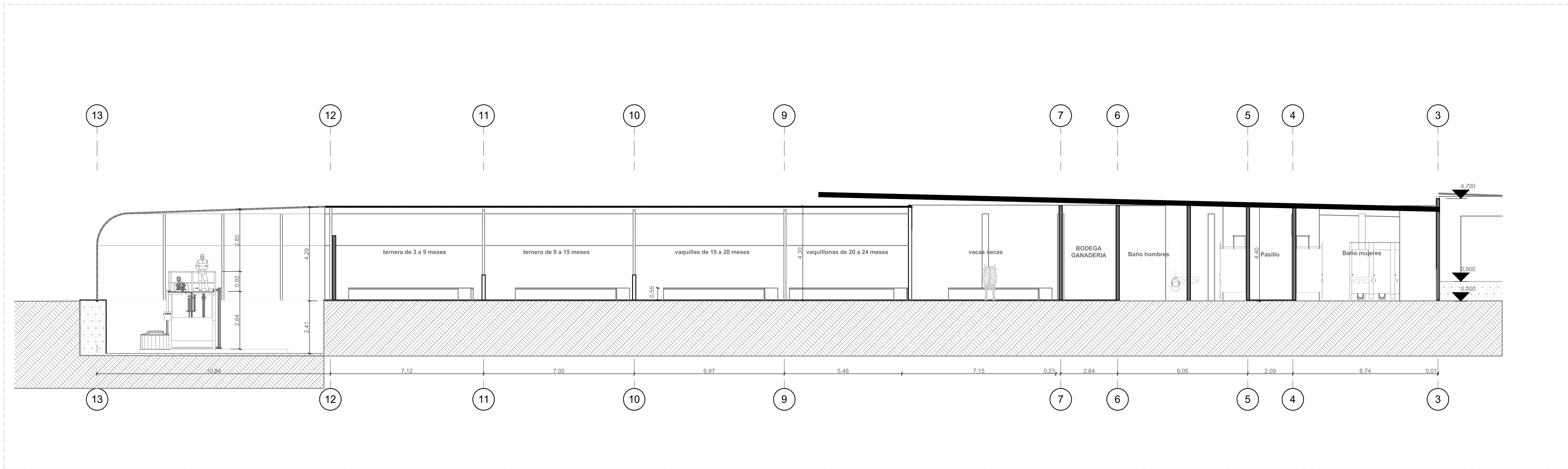
C-07 CORTE ZONA CORRALES 1:100
