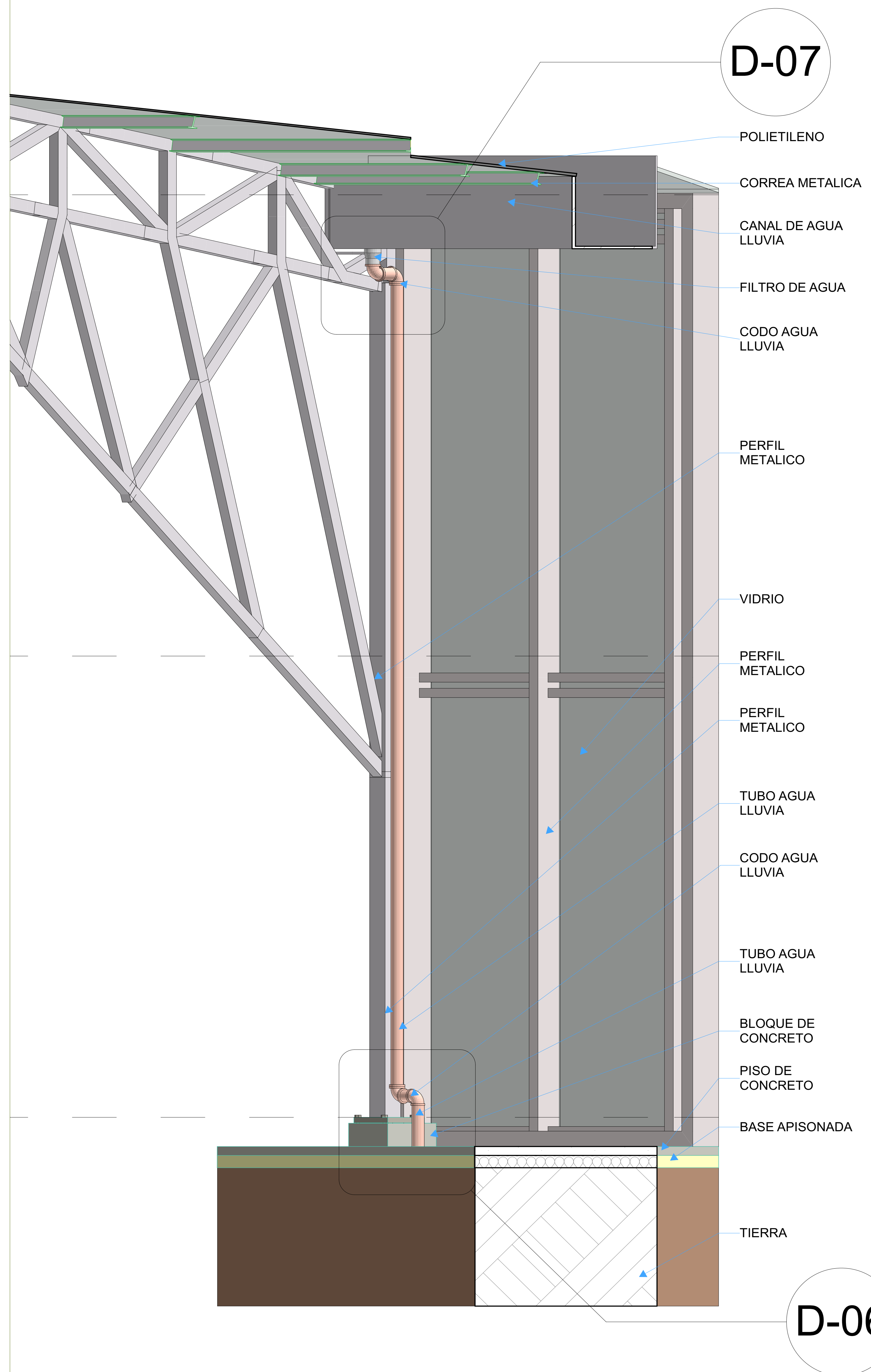
C-2 Sección Construcción
