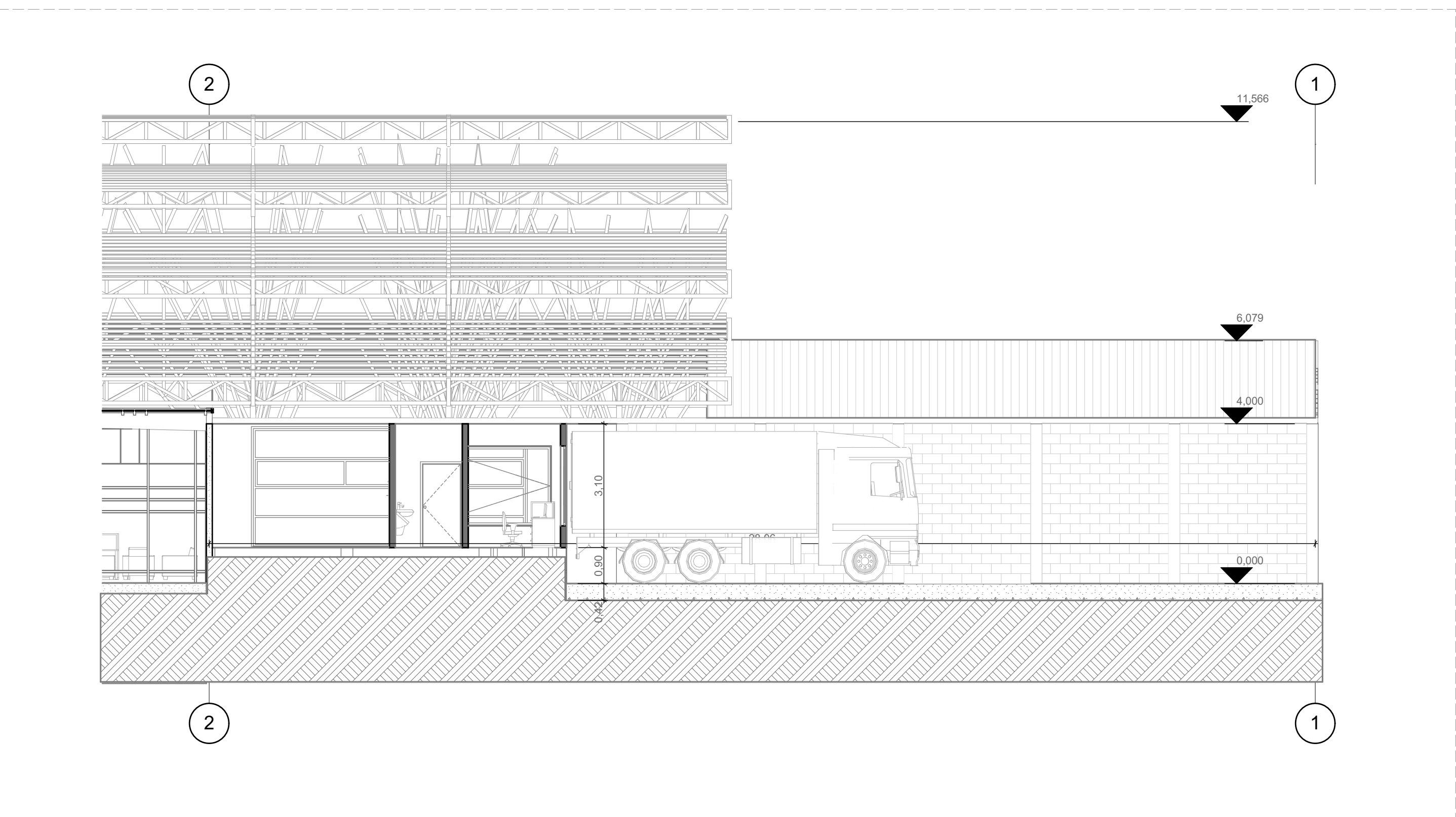
C-06 corte zona de carga invernadero 1:100
