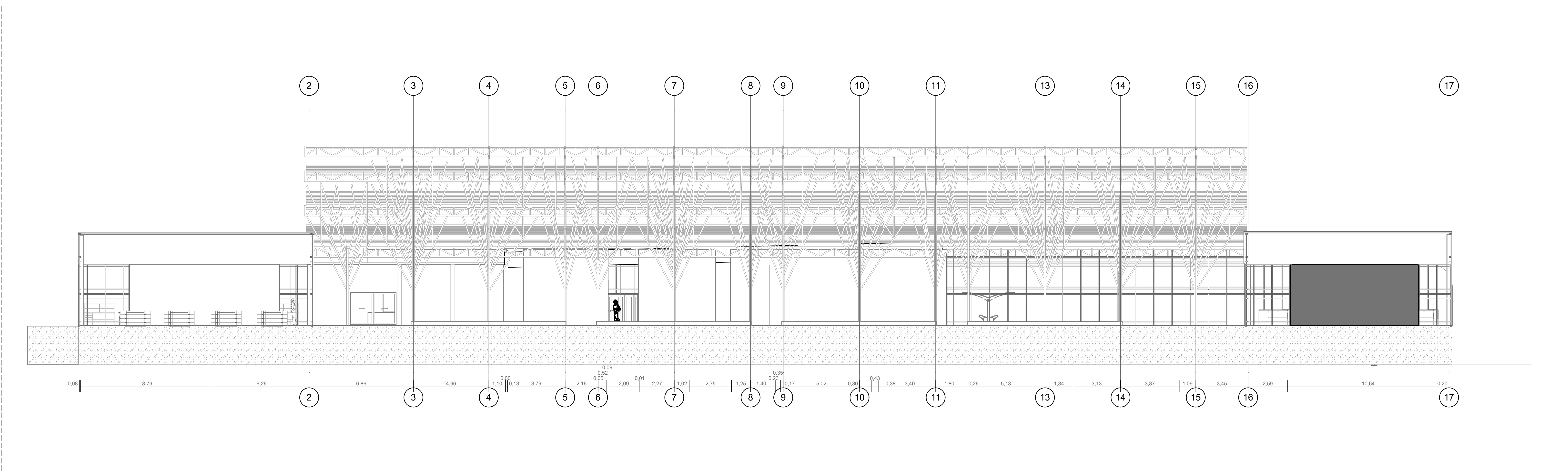
CT 1 CORTE TRANSVERSAL INVERNADERO 1:125
