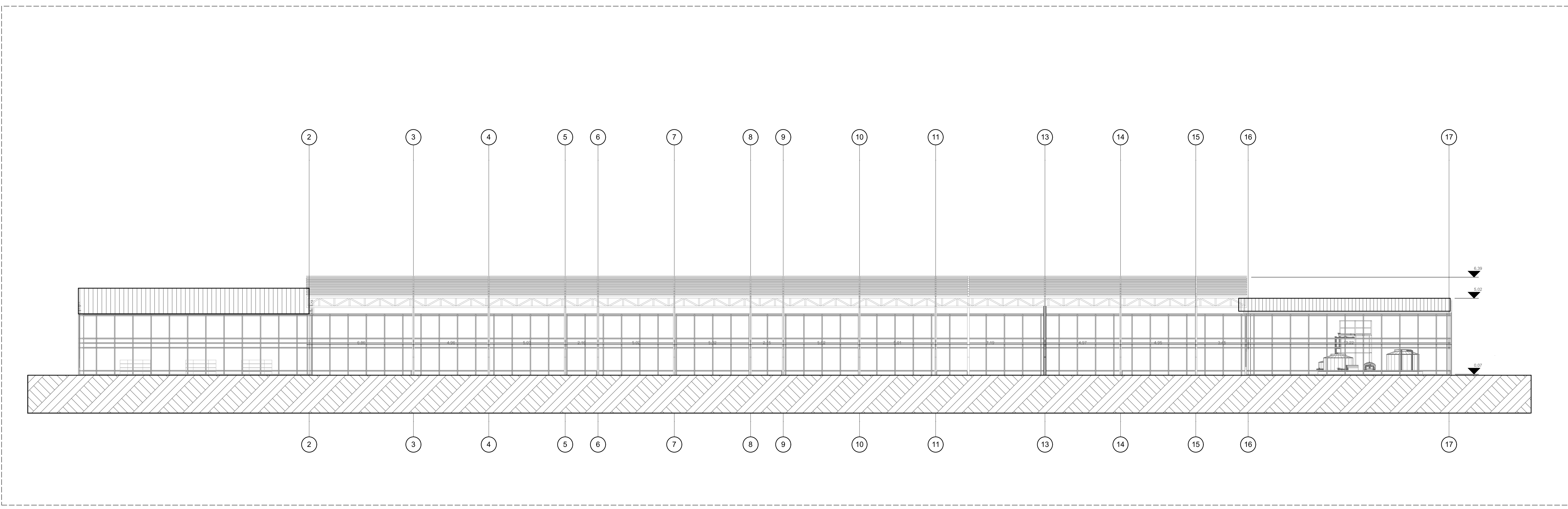
F 3 FACHADA LATERAL 1:125
