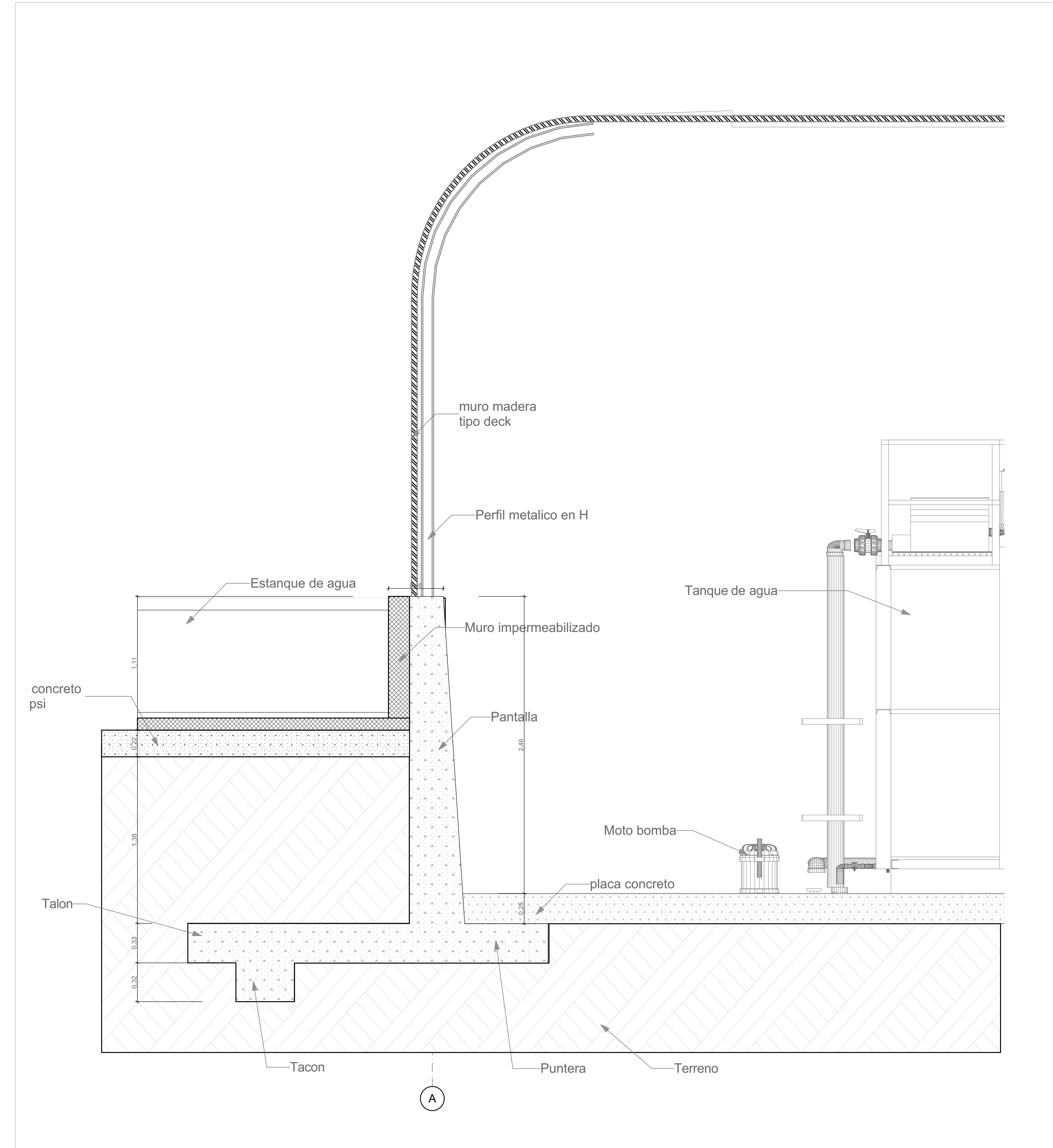
D-03 MURO CONTENCION AGUA 1:20
