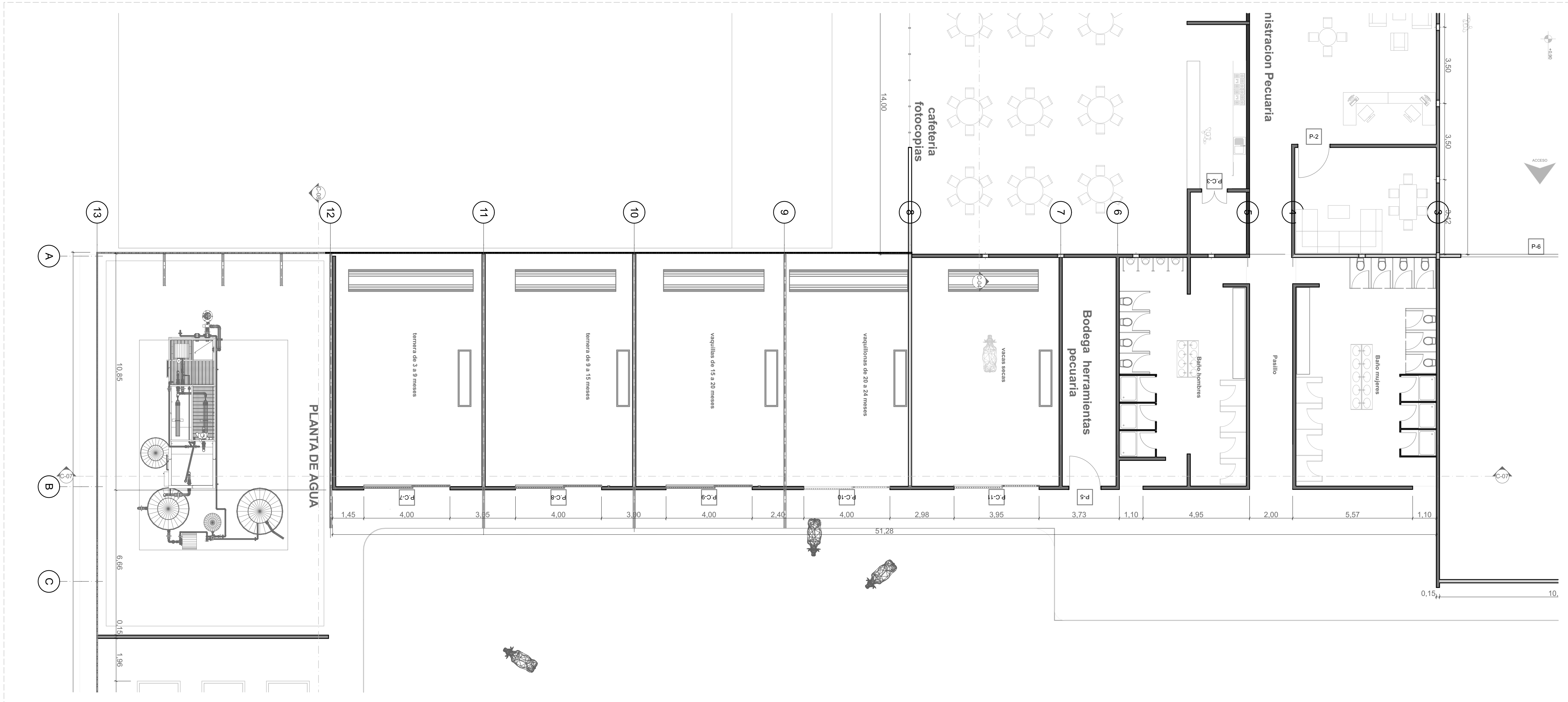
P.G SECCION 2. CORRALES 1:100
