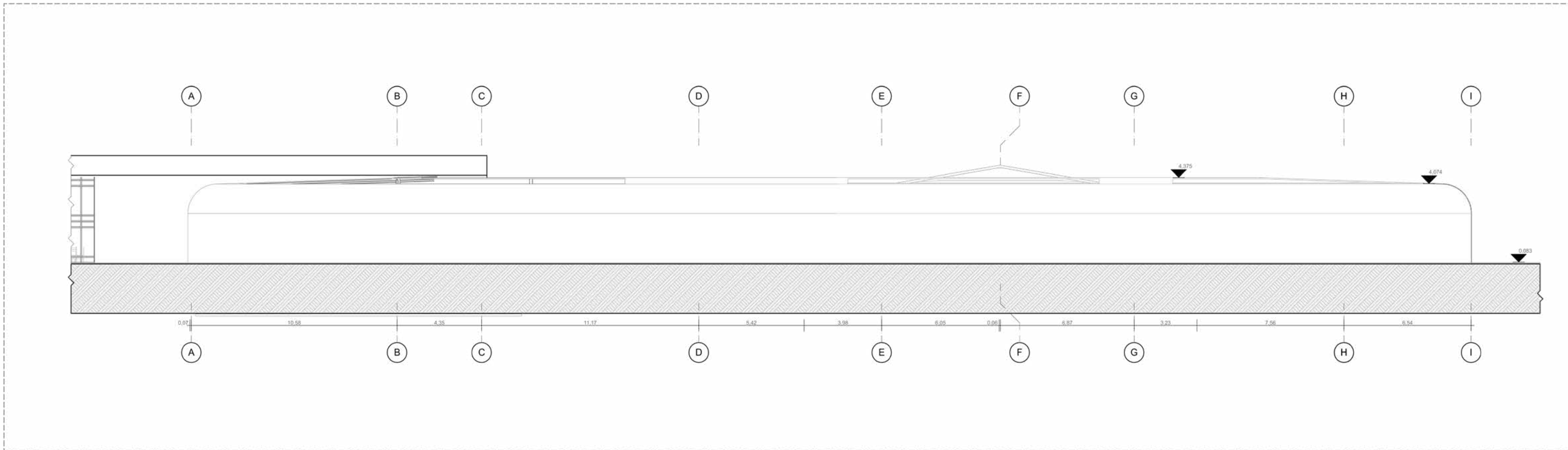
F 6 FACHADA PRINCIPAL GANADERIA 1:100
