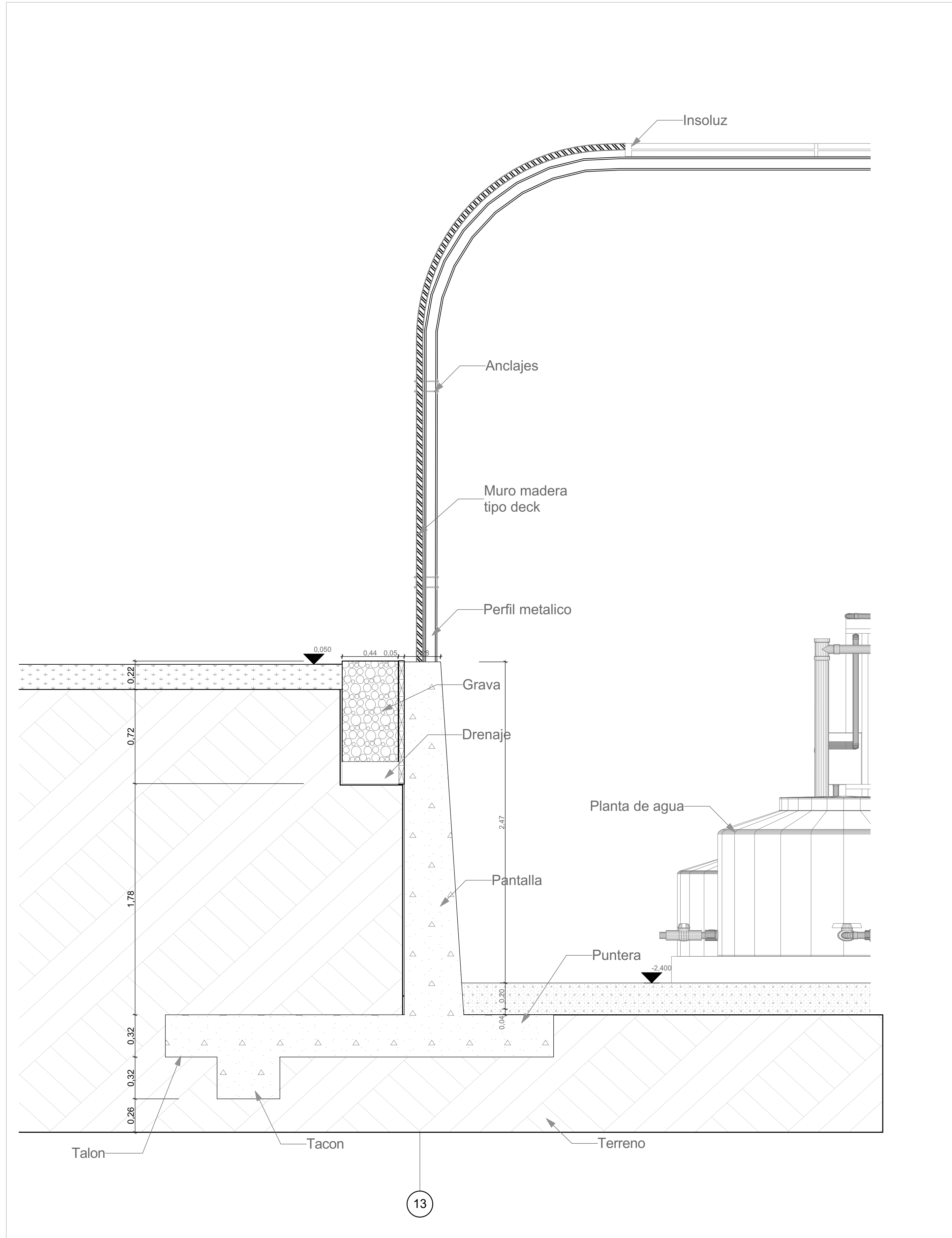
D-01 MURO CONTENCION GANADERIA 1:20
