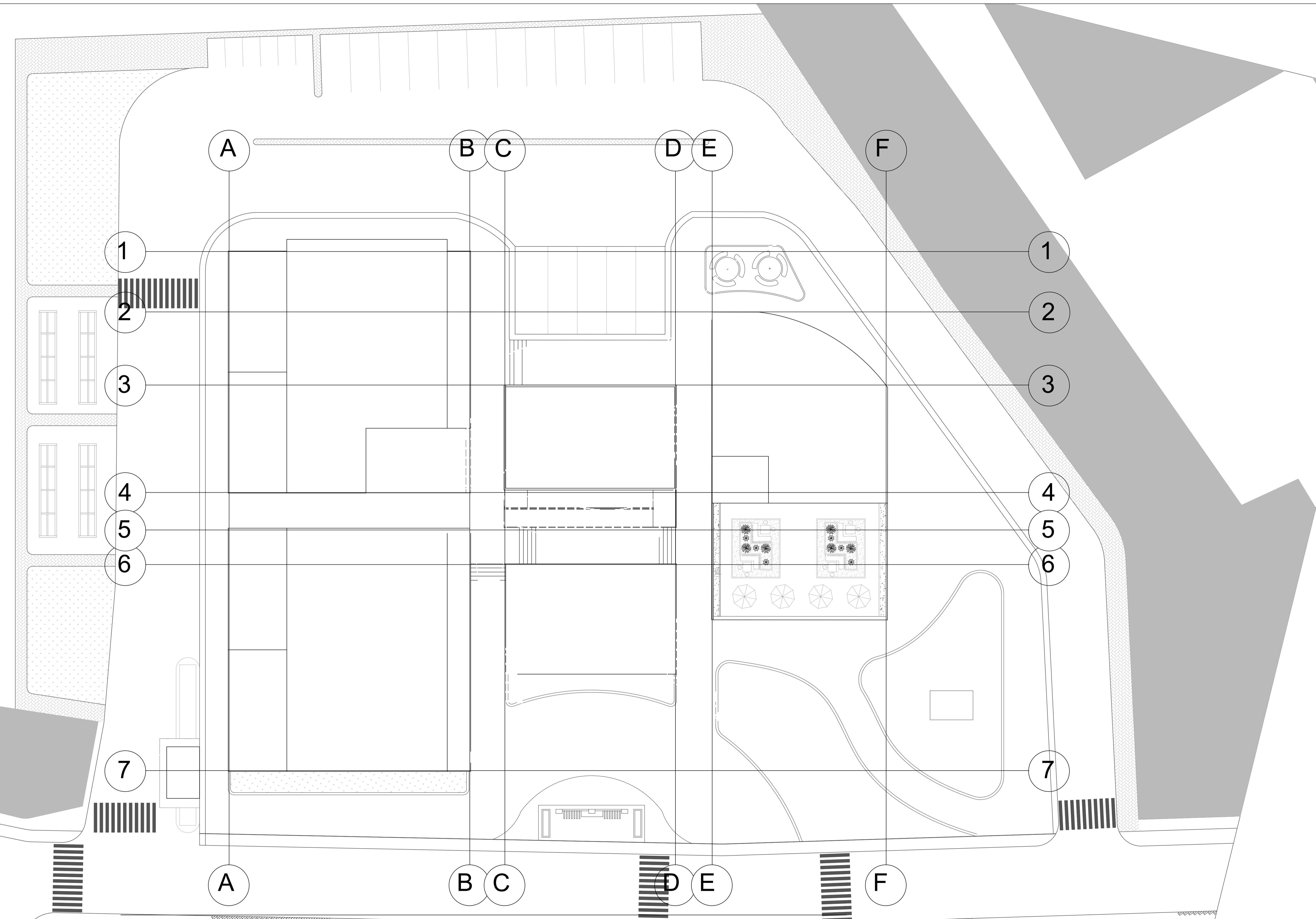
A PLANTA DE CUBIERTAS
