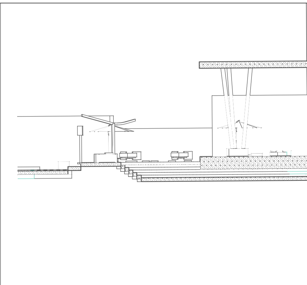
D-2 SECCIÓN PLAZOLETA PRINCIPAL 1: 200
