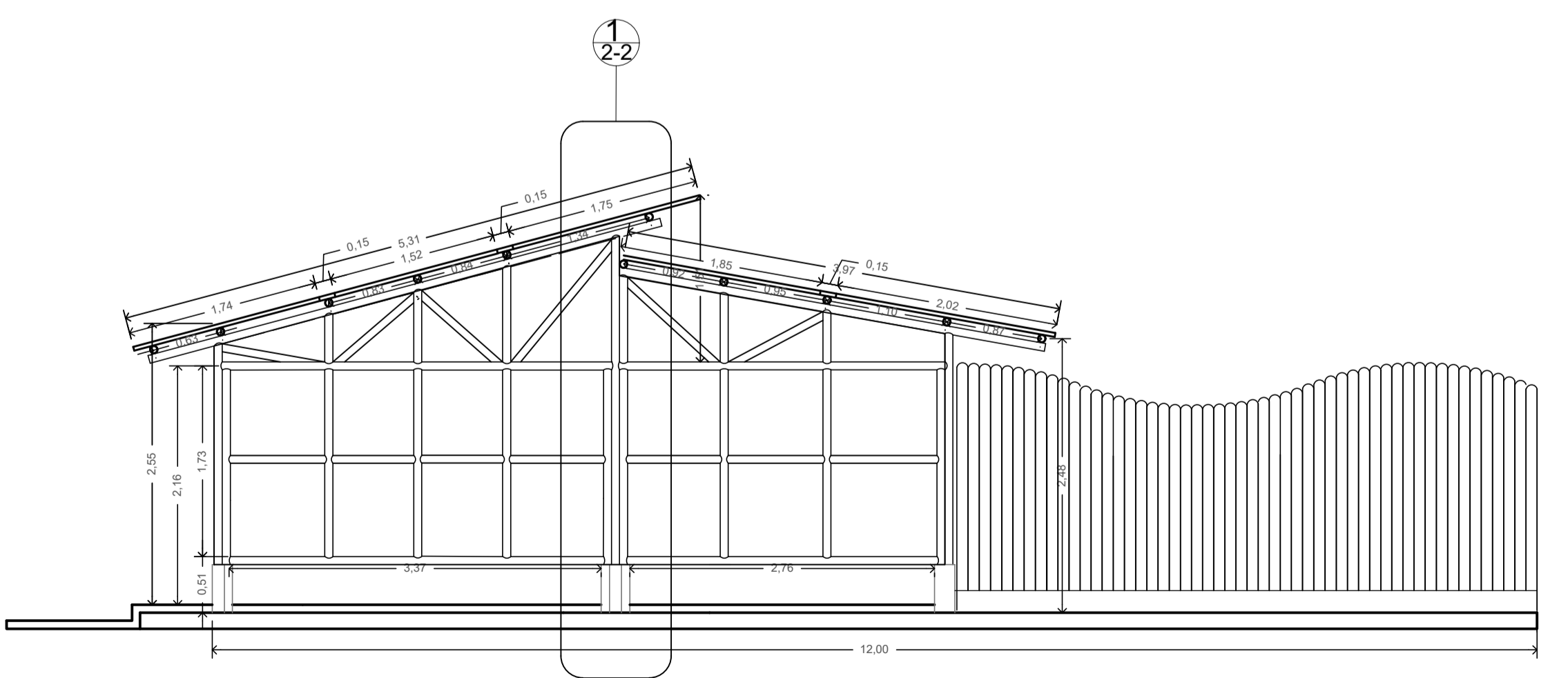
A CORTE LONGITUDINAL 1/30
