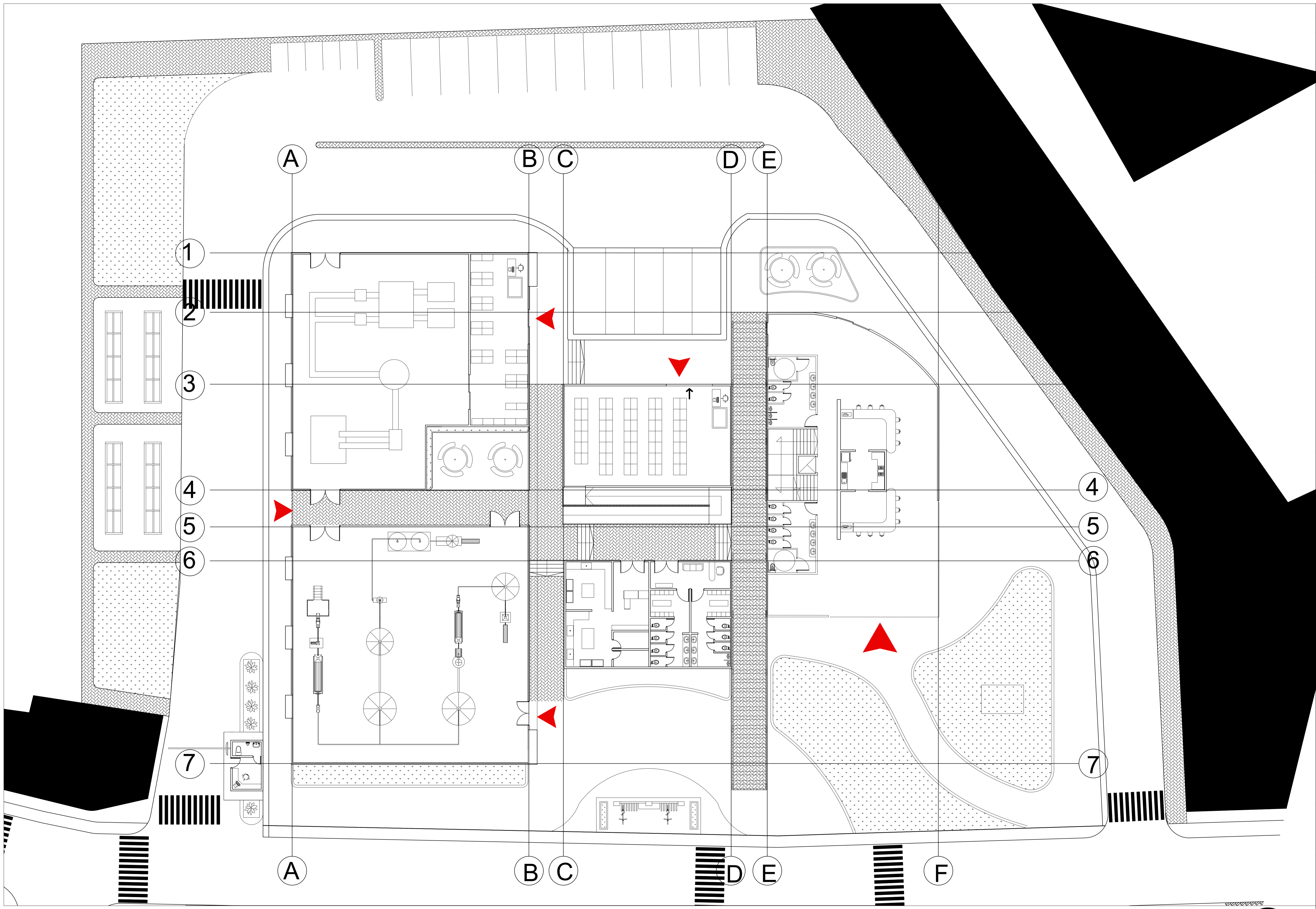
A PLANTA PRIMER NIVEL
