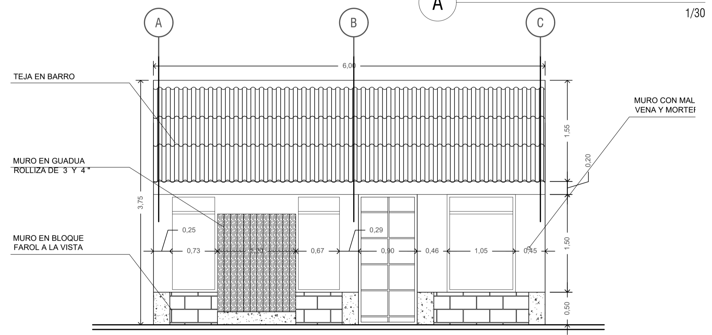
A FACHADA POSTERIOR 1/30
