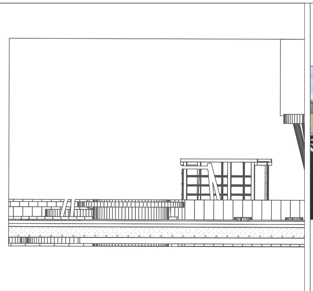
D-1 SECCIÓN PLAZOLETA DEPORTIVA 1: 200
