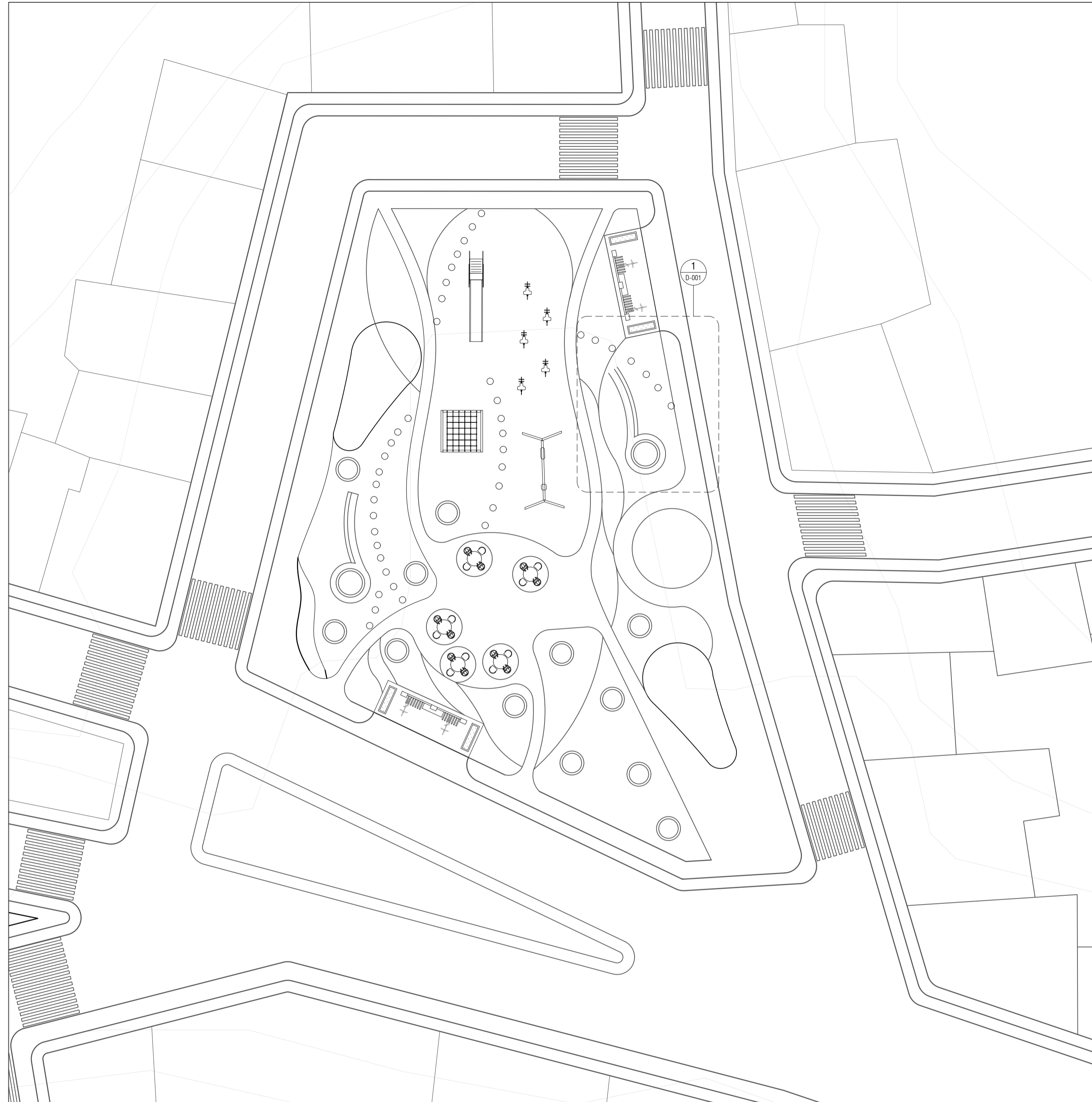
D-1 PLAZOLETA DEPORTIVA 1: 250
