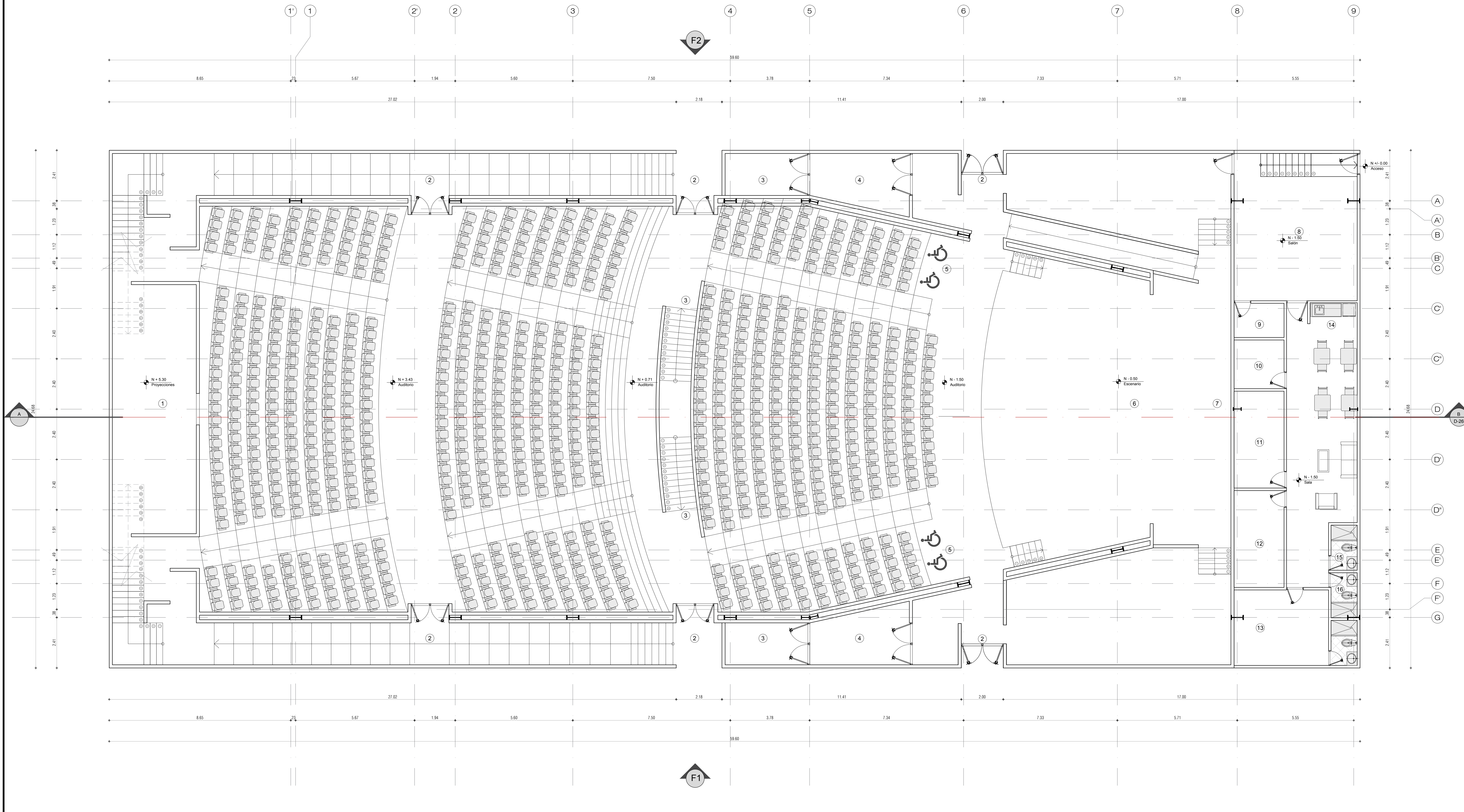
D1 PLANTA SEGUNDO NIVEL 1:75
