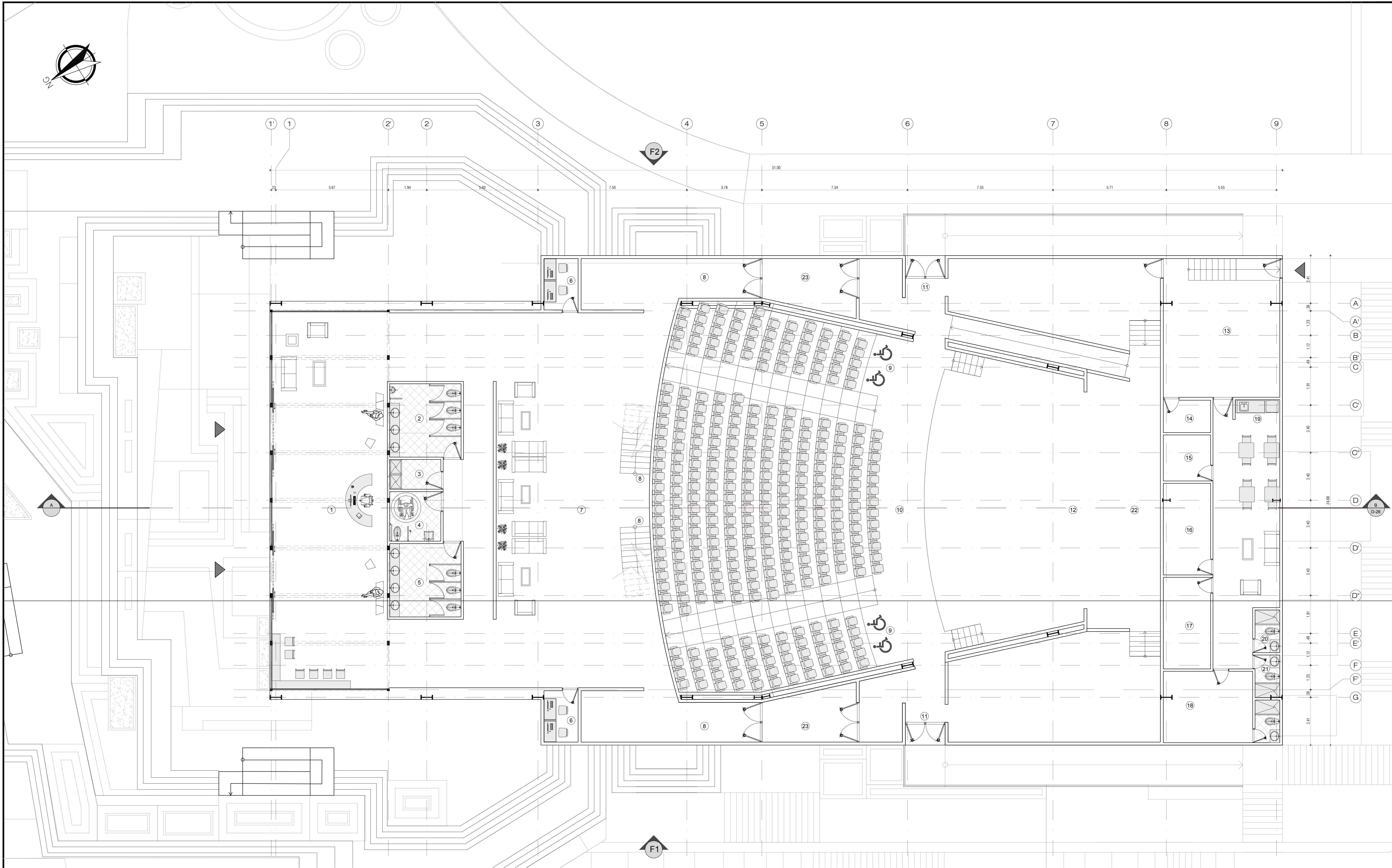
D1 PLANTA PRIMER NIVEL 1:75
