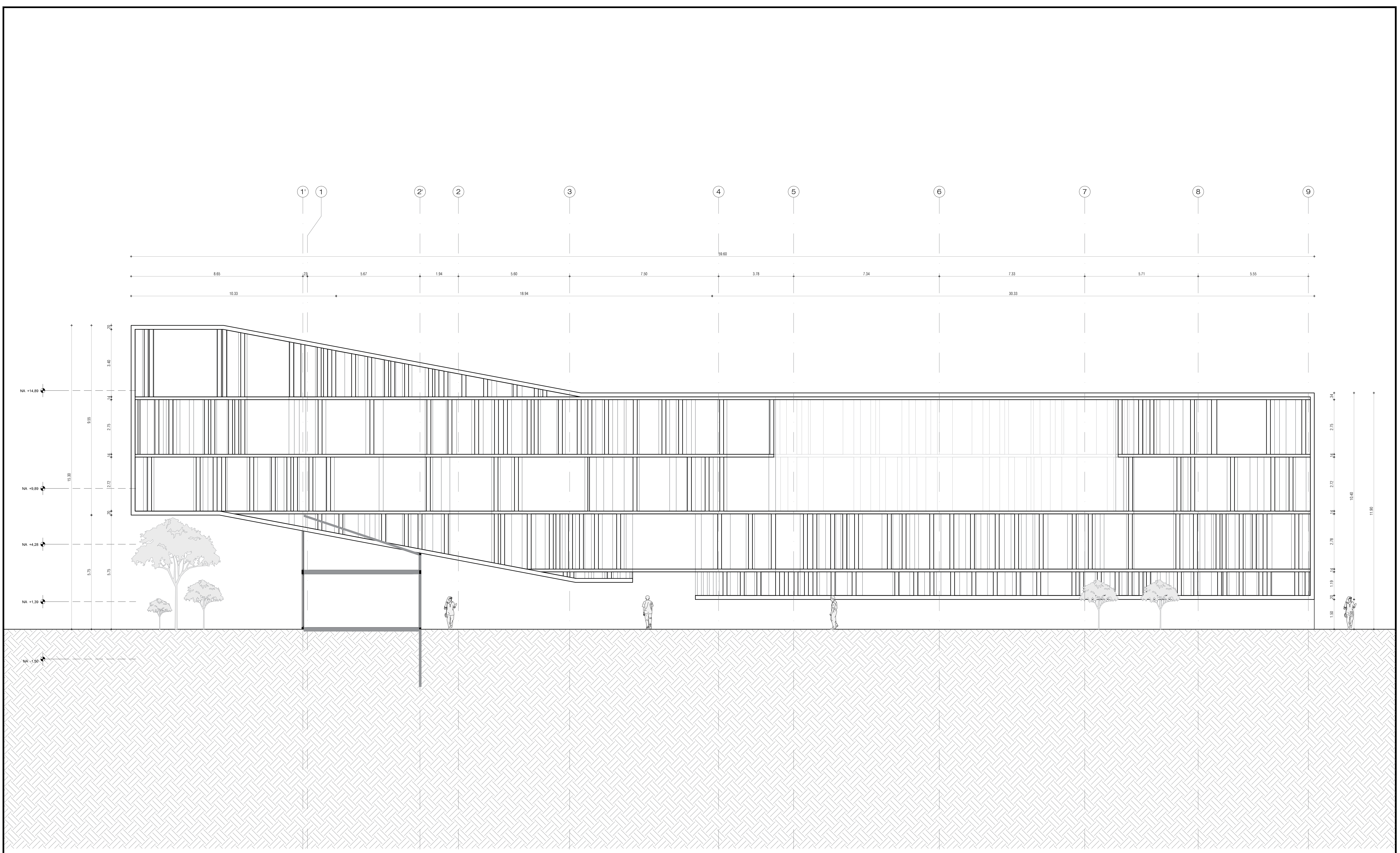
D1 F1 - FACHADA NOROCCIDENTE 1:75
