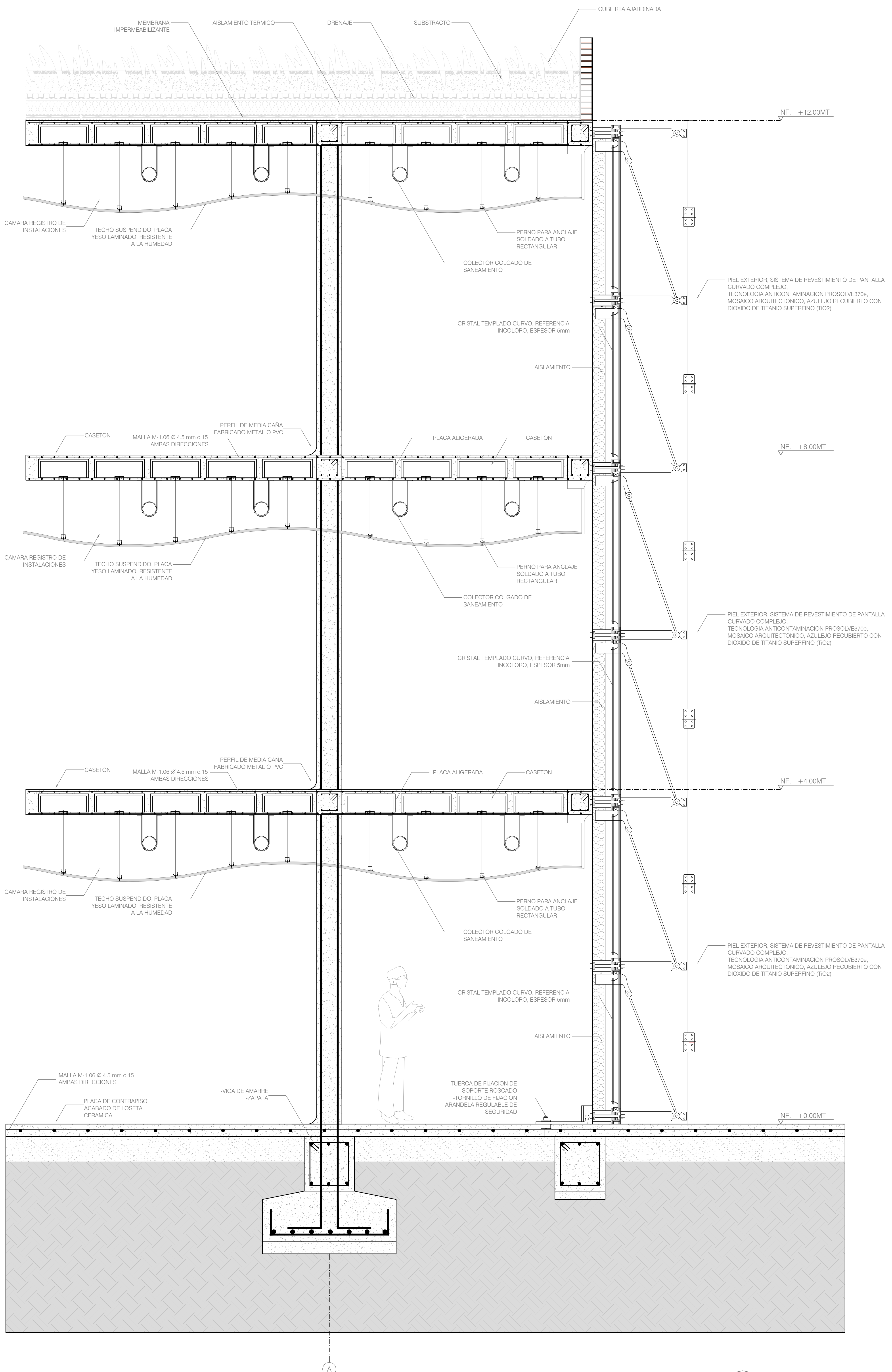
C1 CORTE FACHADA ESCALA 1:20
